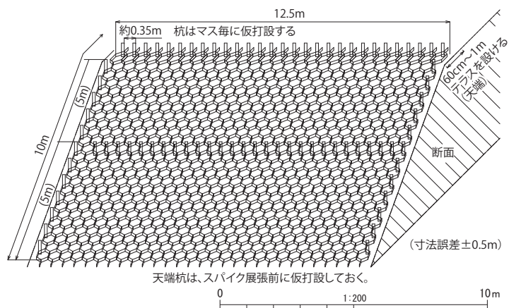
第 26 図 地盤補強材止杭打ち参考図
