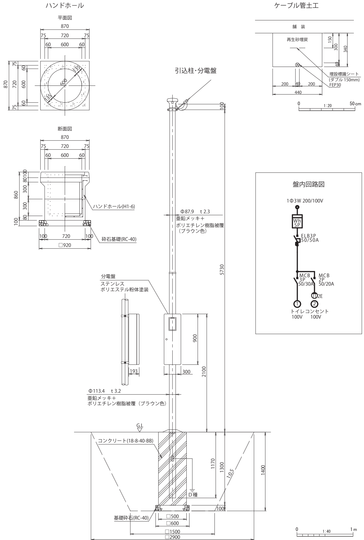
第 59 図 電気設備工詳細図
