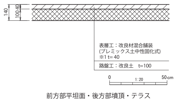
第62図 土質舗装 A 工標準断面図
