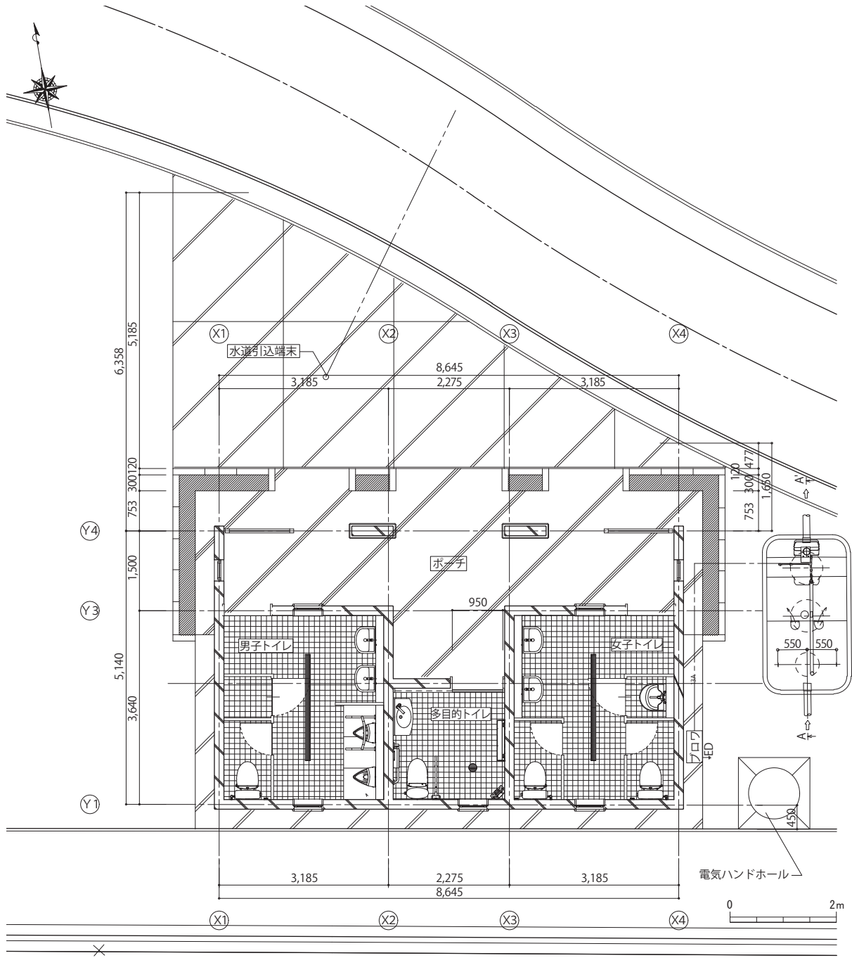
第 80 図 トイレ全体平面図
