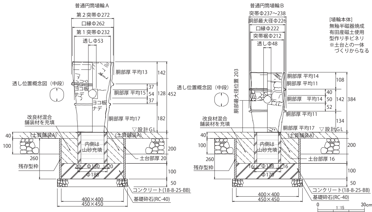
第52図 埴輪工（普通円筒形埴輪）の標準断面
