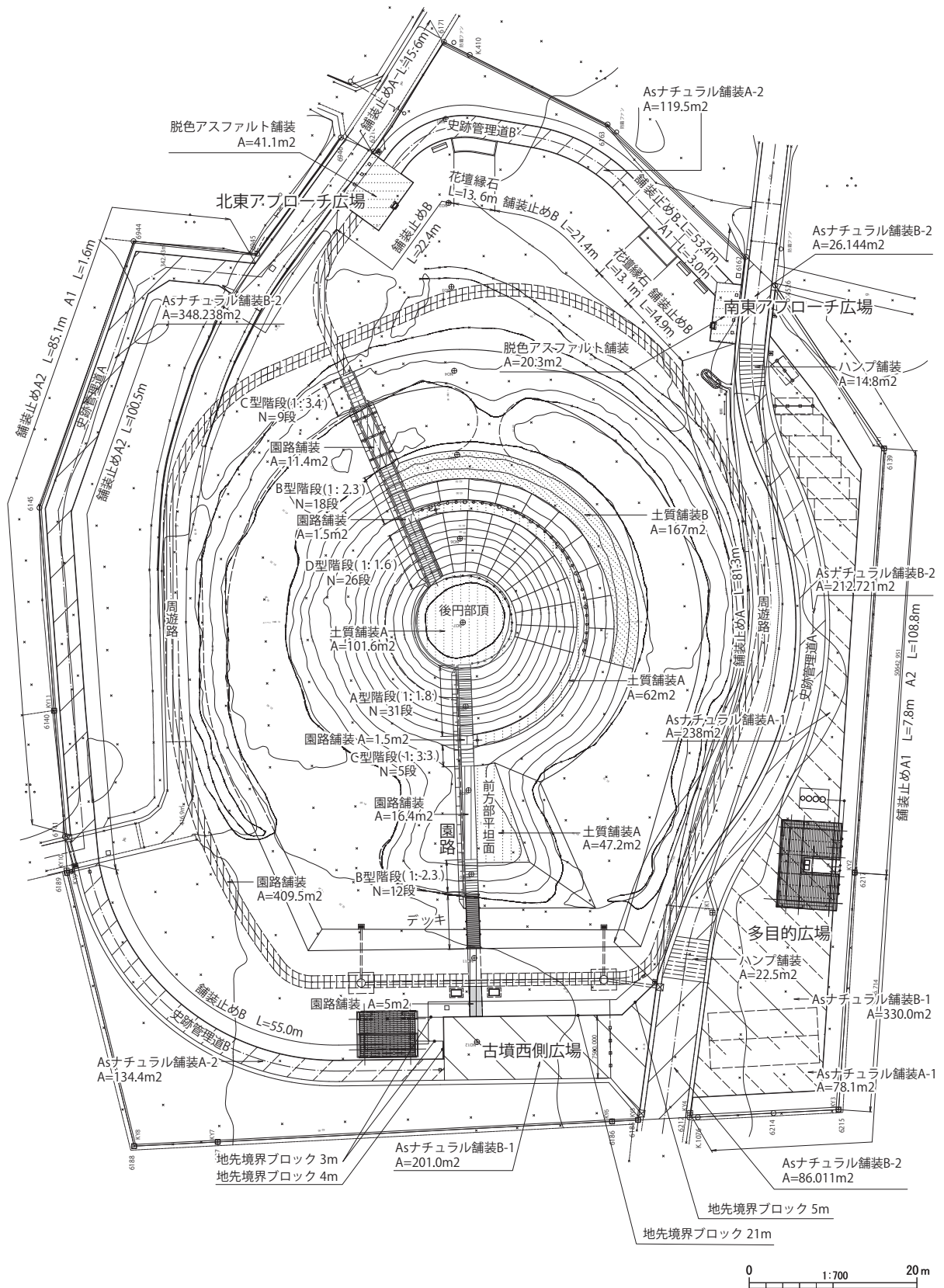
第41図 園路及び広場計画平面図
