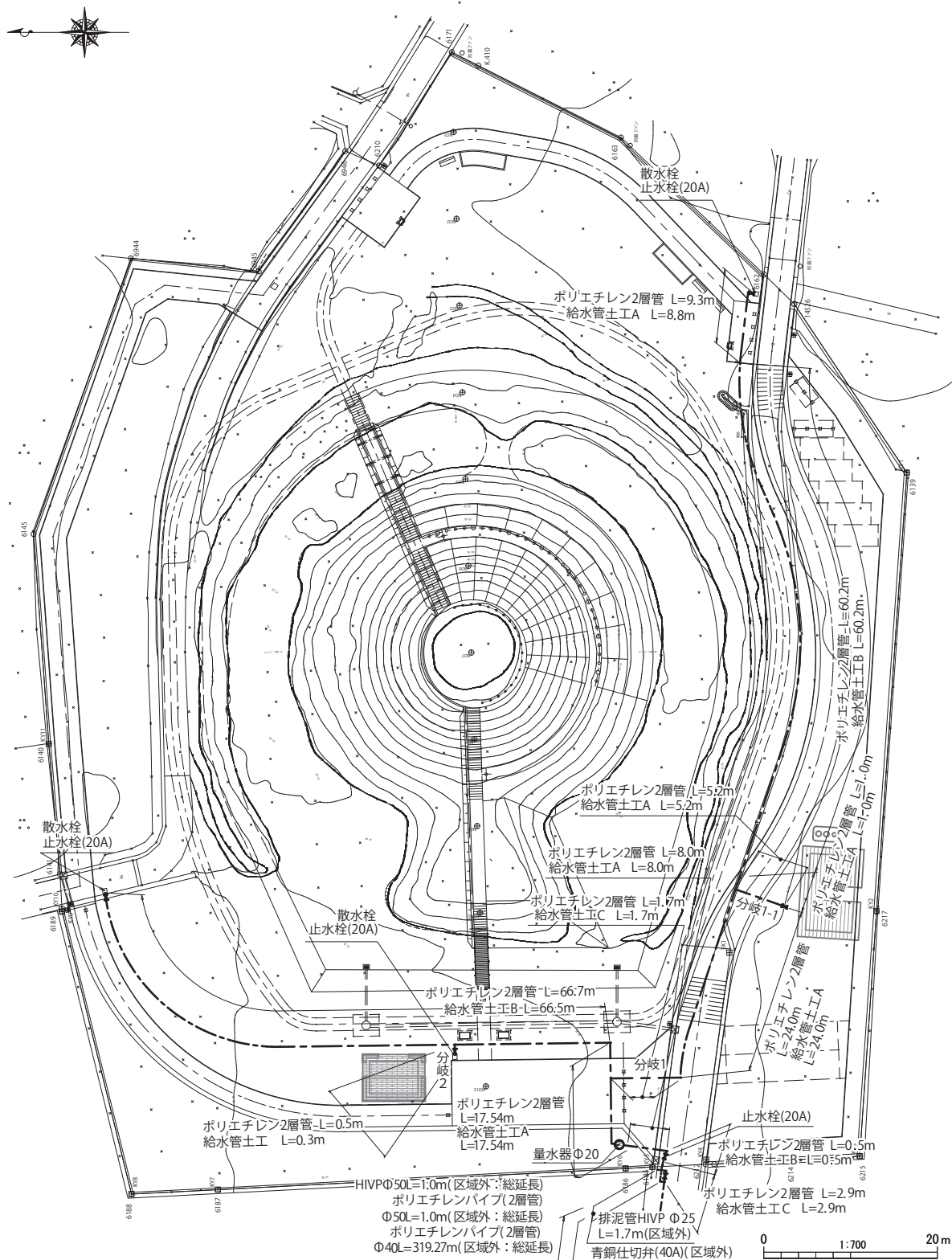
第39図 給水計画平面図 (場内)
