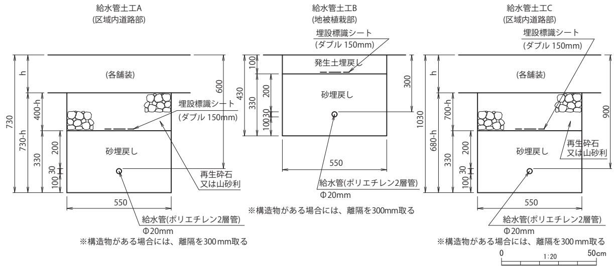
第55図 給水工（場内）の標準断面図
