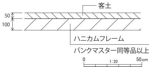
第 24 図 地盤補強材標準断面図
