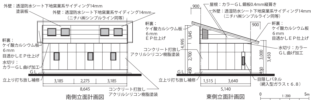
第81図 トイレ立面図
