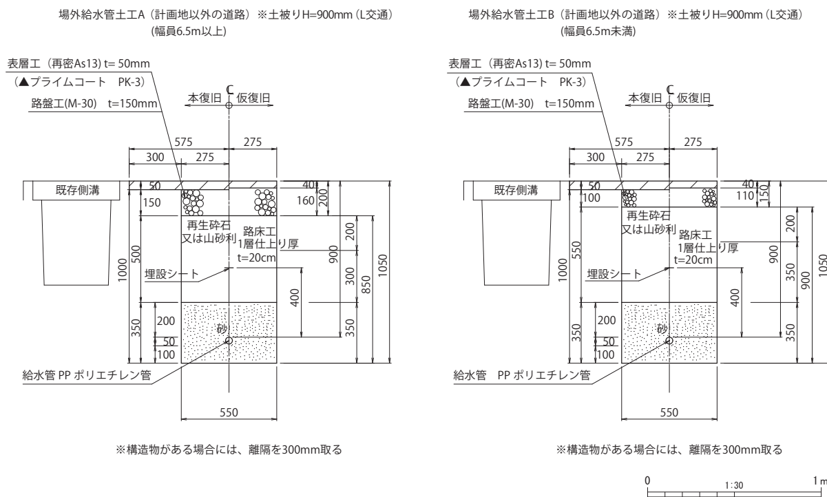
第 54 図 給水工（場外）の標準断面図
