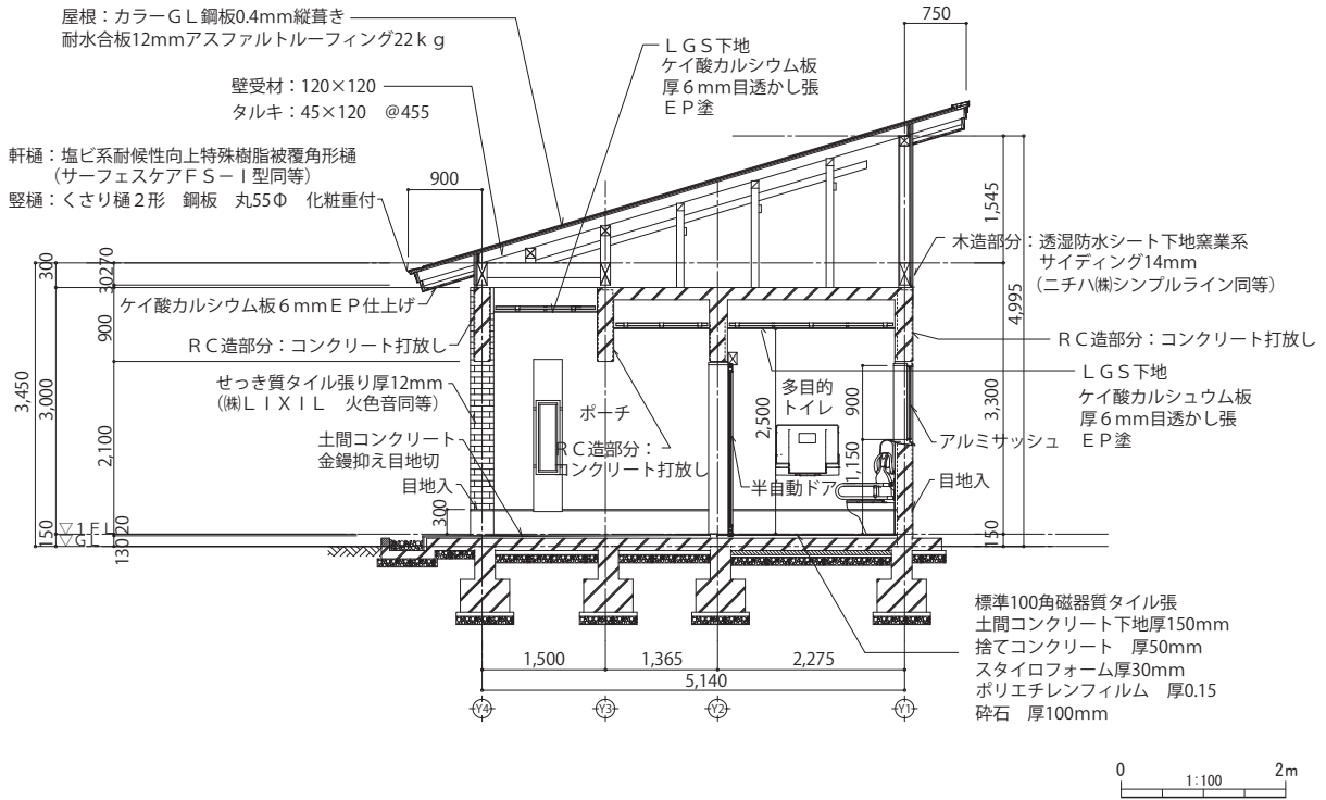
第 83 図 トイレ矩形図 (2)
