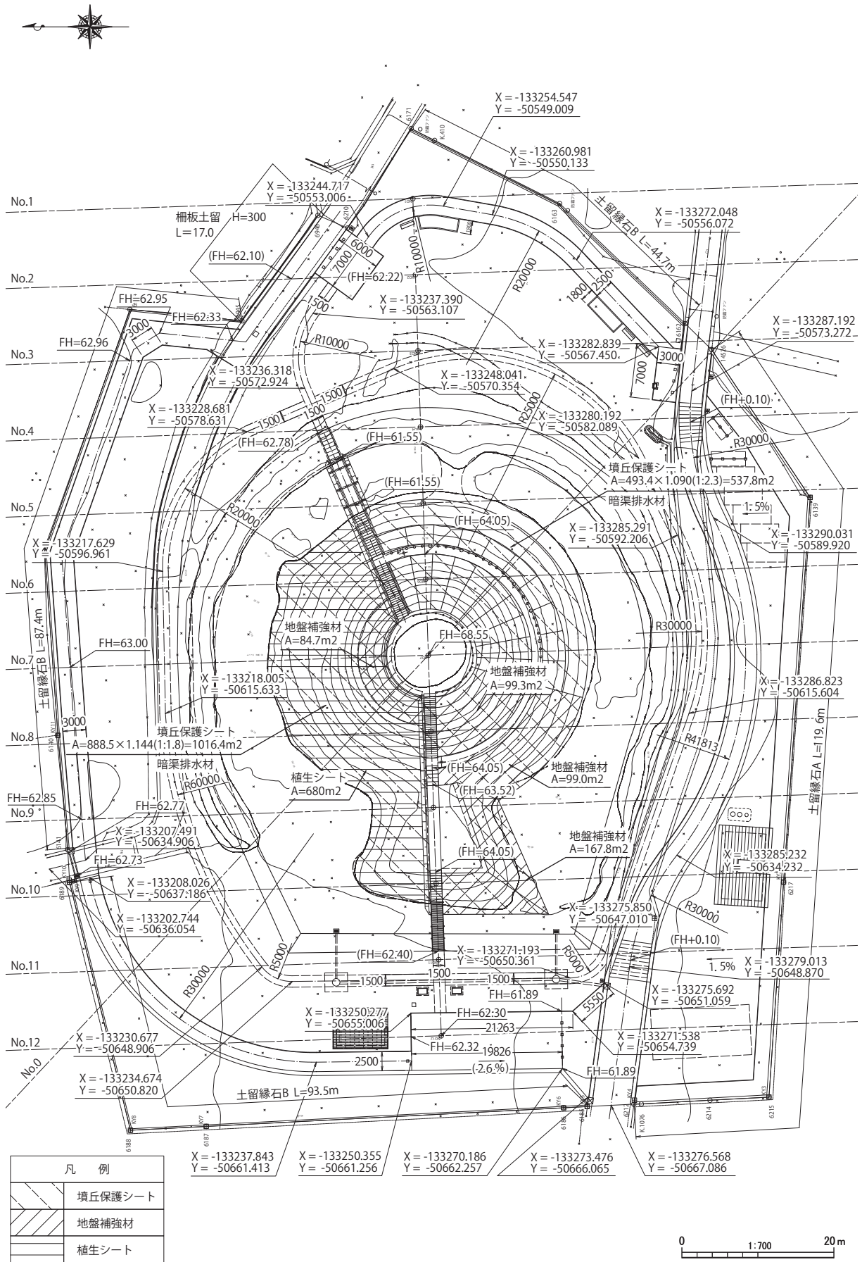
第 29 図 造成計画平面図
