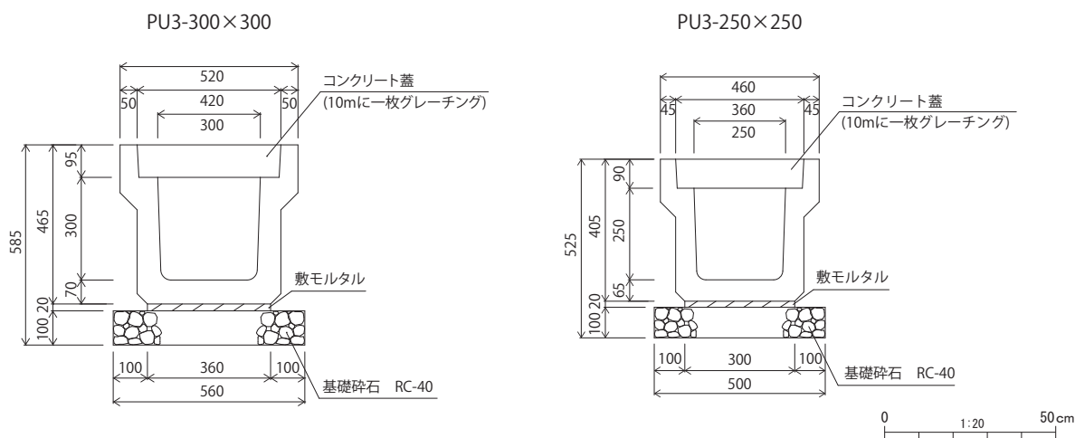
第 46 図 排水施設構造図 (1)
