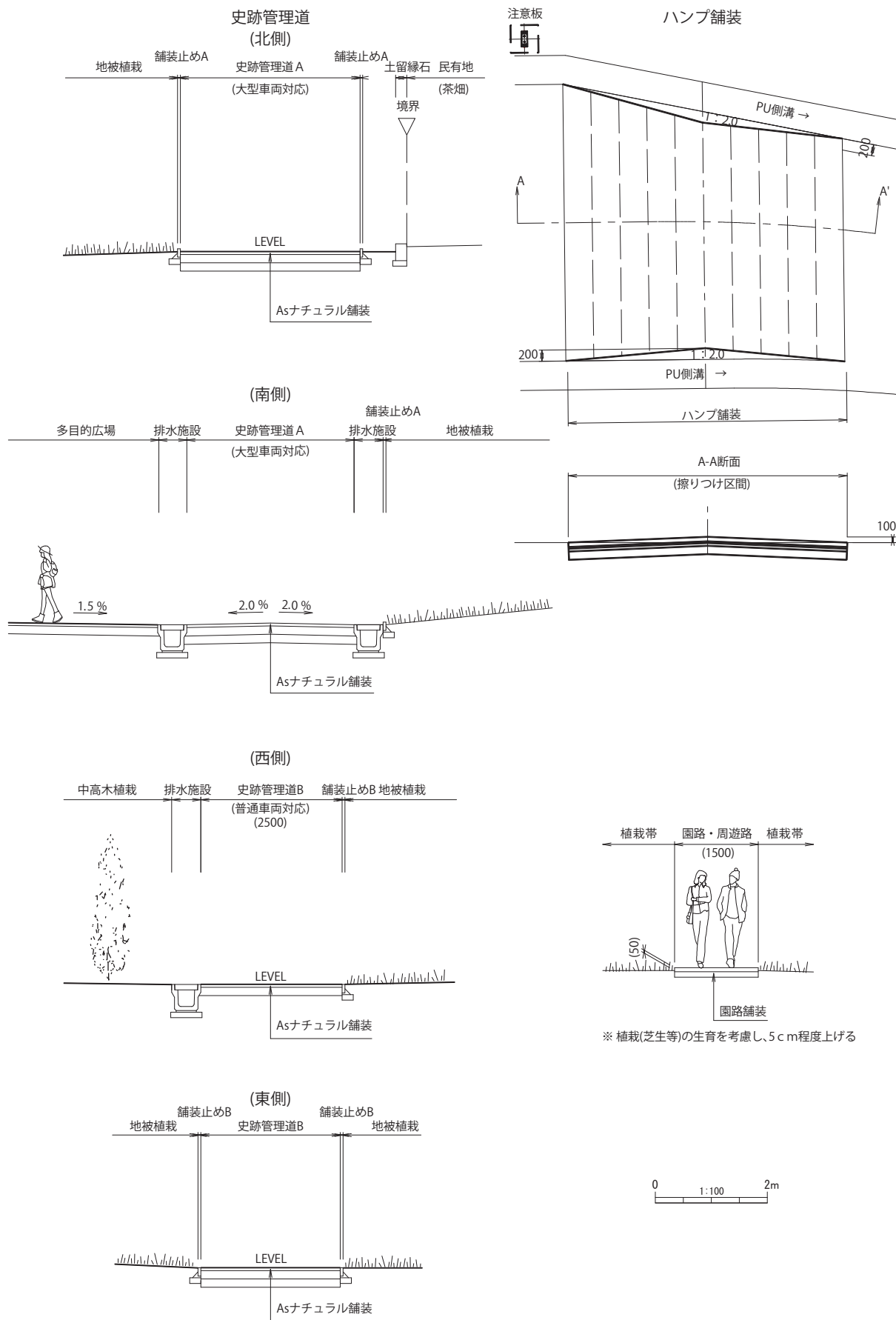
第 42 図 園路の整備イメージ断面図
