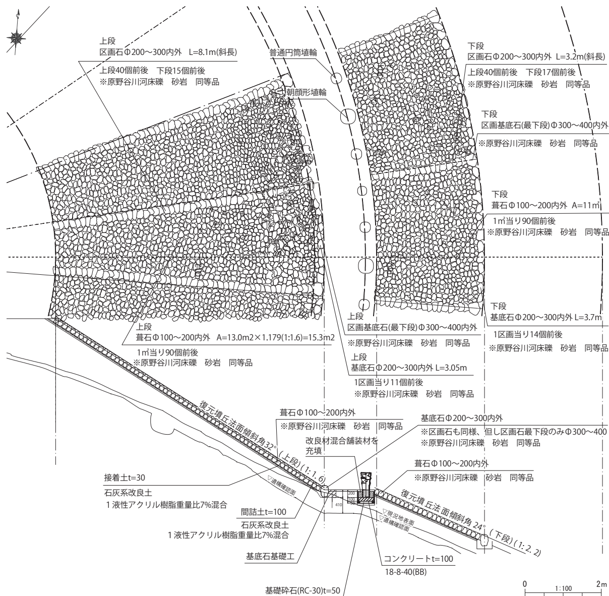
第49図 葺石工の標準断面図及び施行参考平面図
