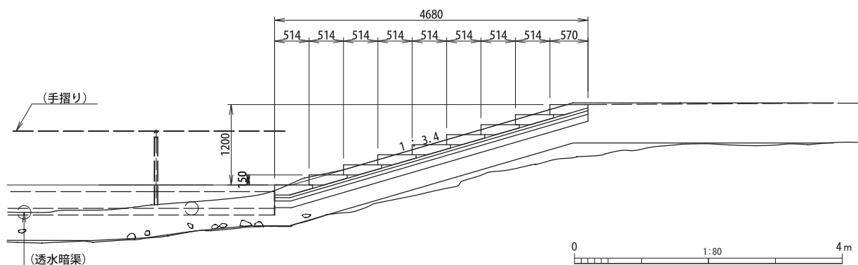
第 68 図 階段工詳細図 (2)
