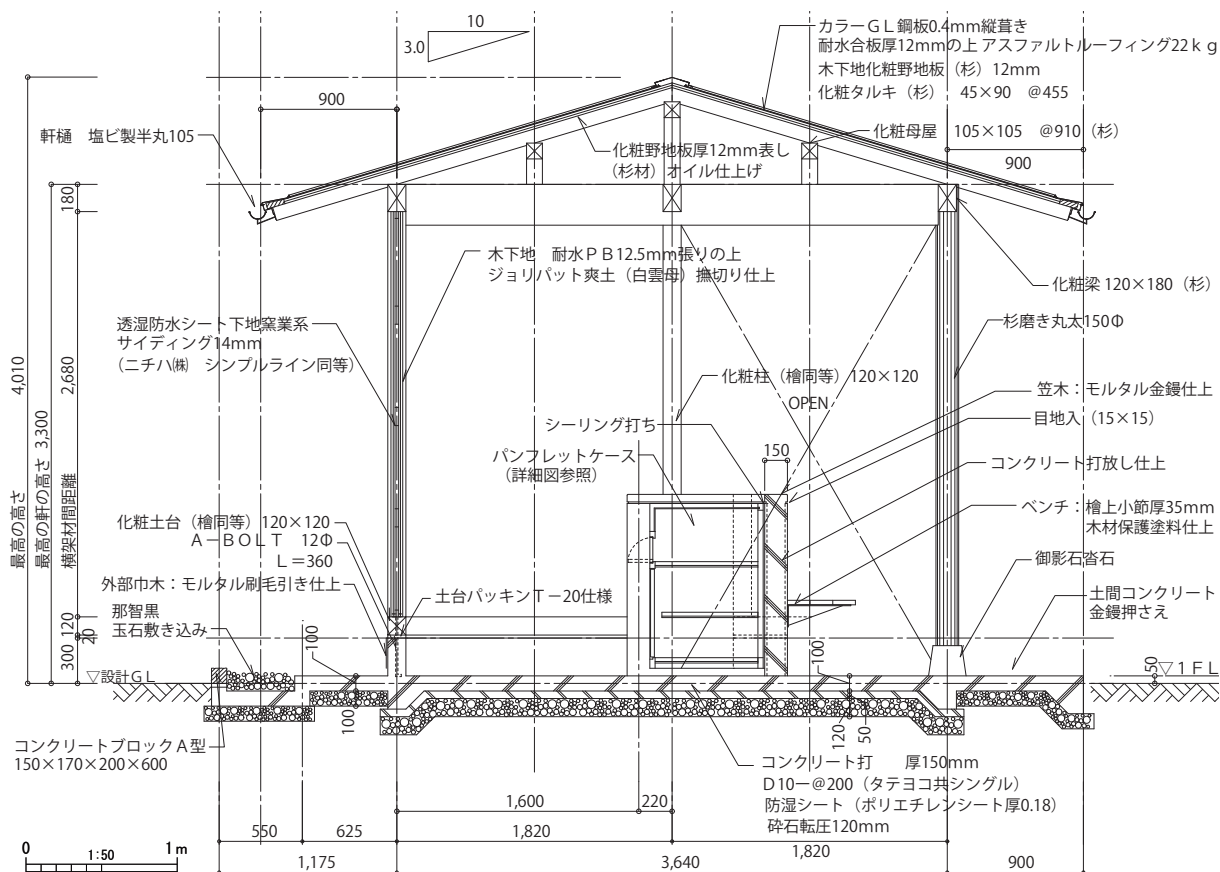
第 86 図 休憩施設矩形図
