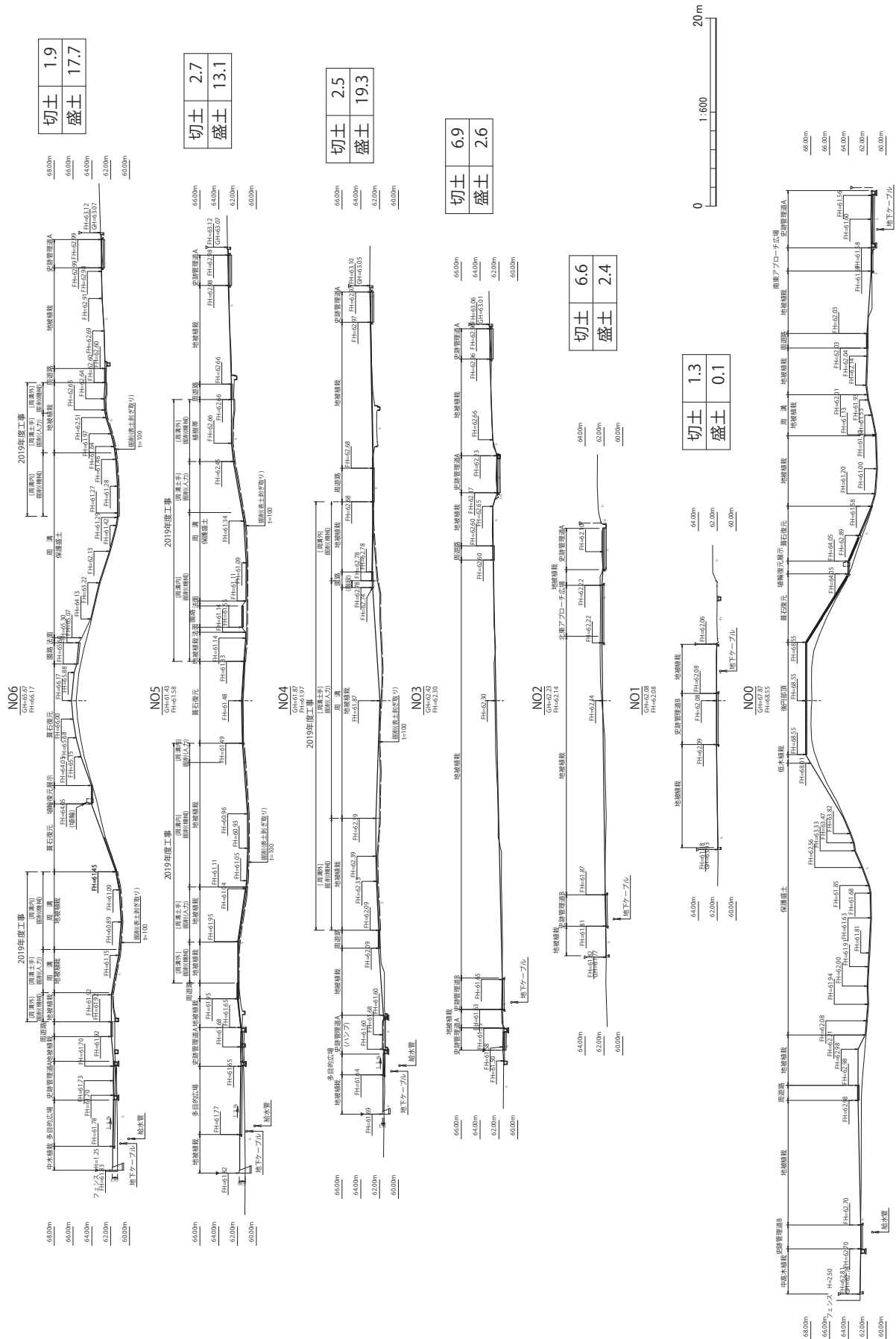
第31図 造成計画断面図(2)
