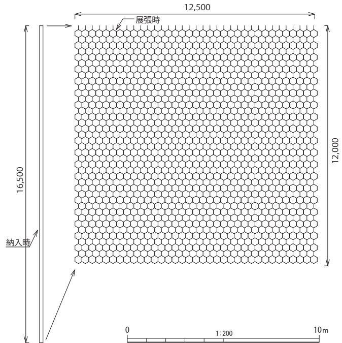
第 25 図 地盤補強材標準展開図
