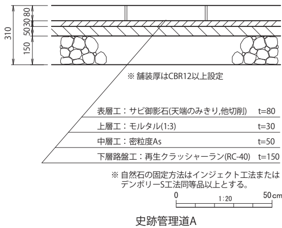
第61図 ハンプ舗装工標準断面
