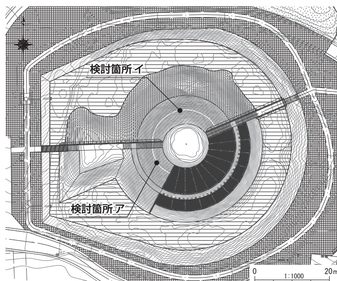
第27図 構造設計（滑動計算）検討箇所位置図
