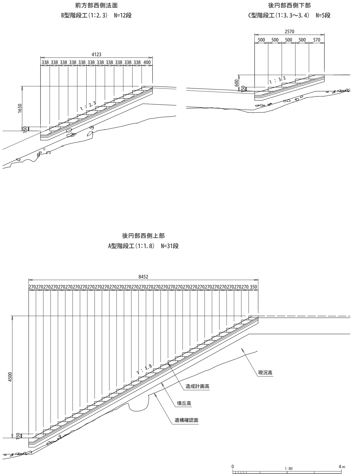
第 67 図 階段工詳細図 (1)
