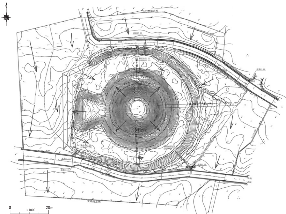
第 34 図 排水対策検討図
