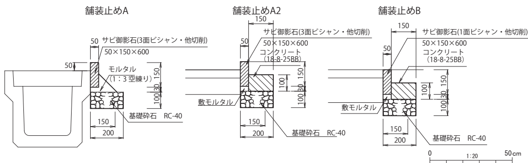
第 65 図 縁石詳細断面図
