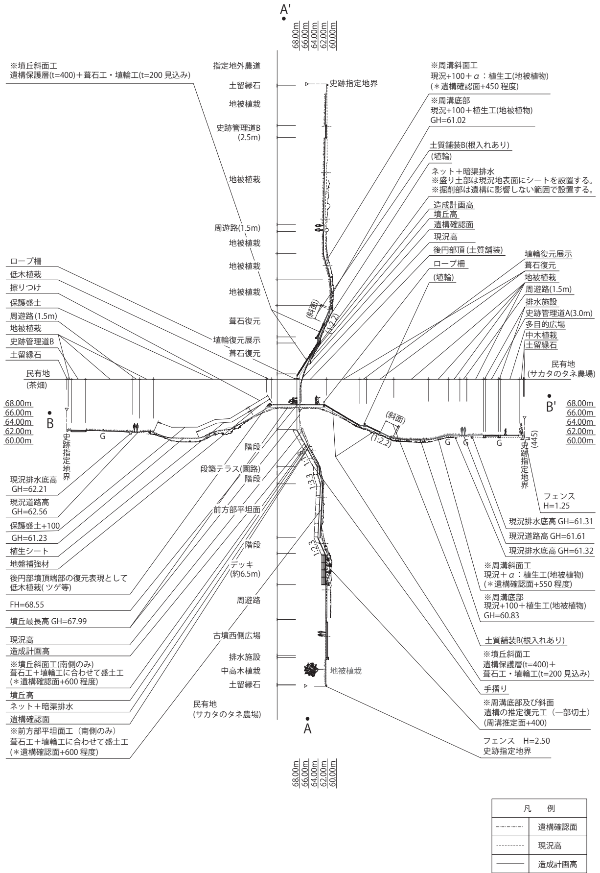
第22図 全体計画標準断面図
