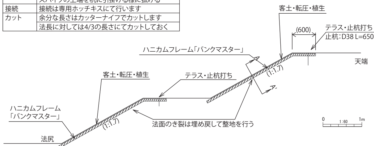
第28図 構造設計参考断面図
