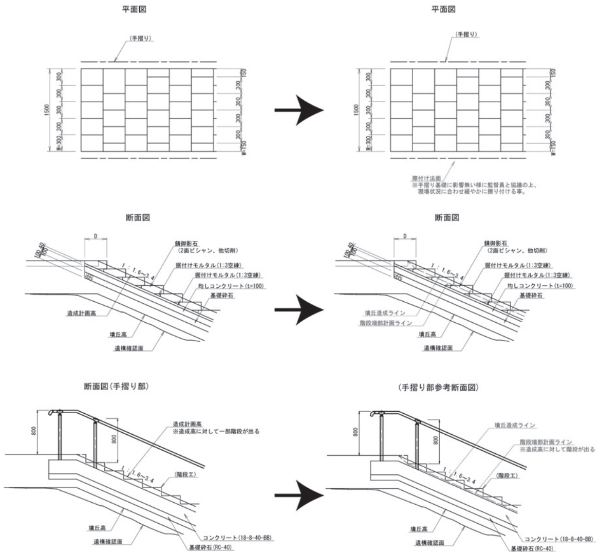
第45図 墳丘盛土と階段部との施行上取合い参考図
