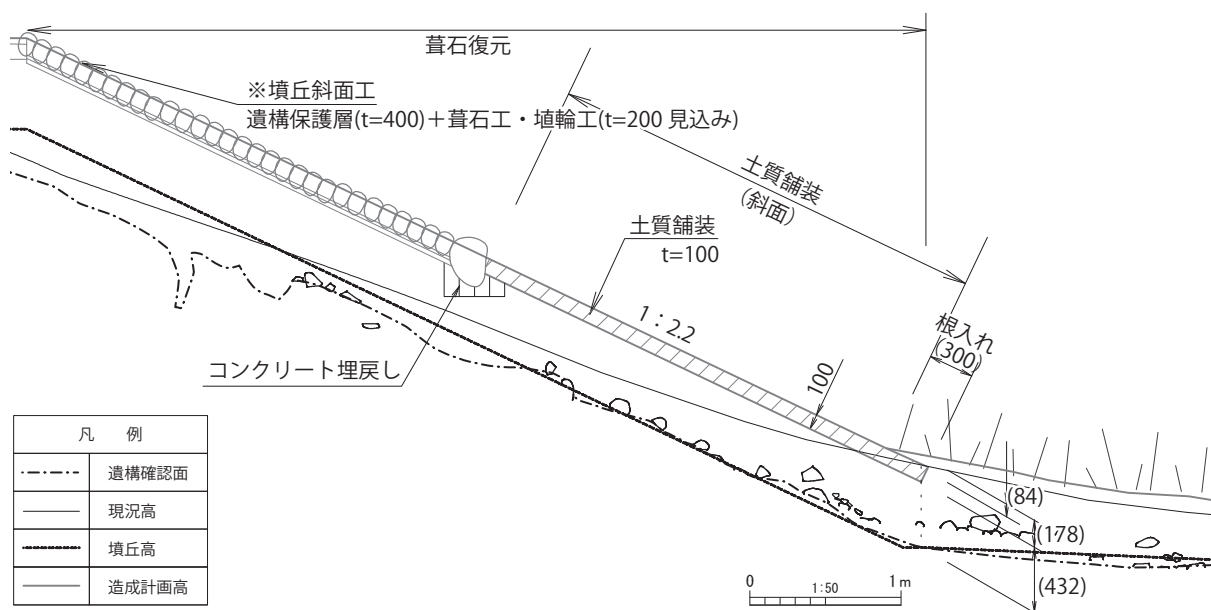
第 53 図 葺石復元部下段直下の標準断面
