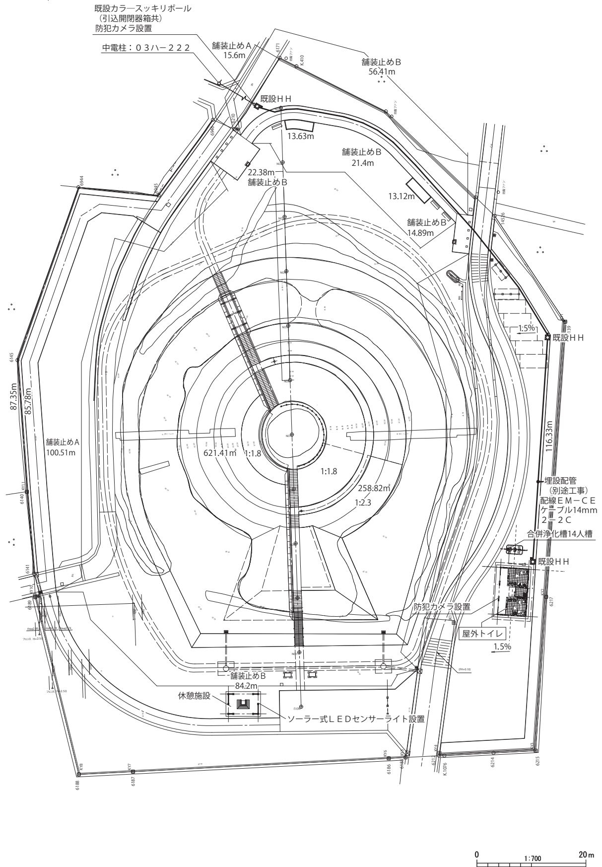
第 88 図 トイレ・休憩施設電気工事平面図
