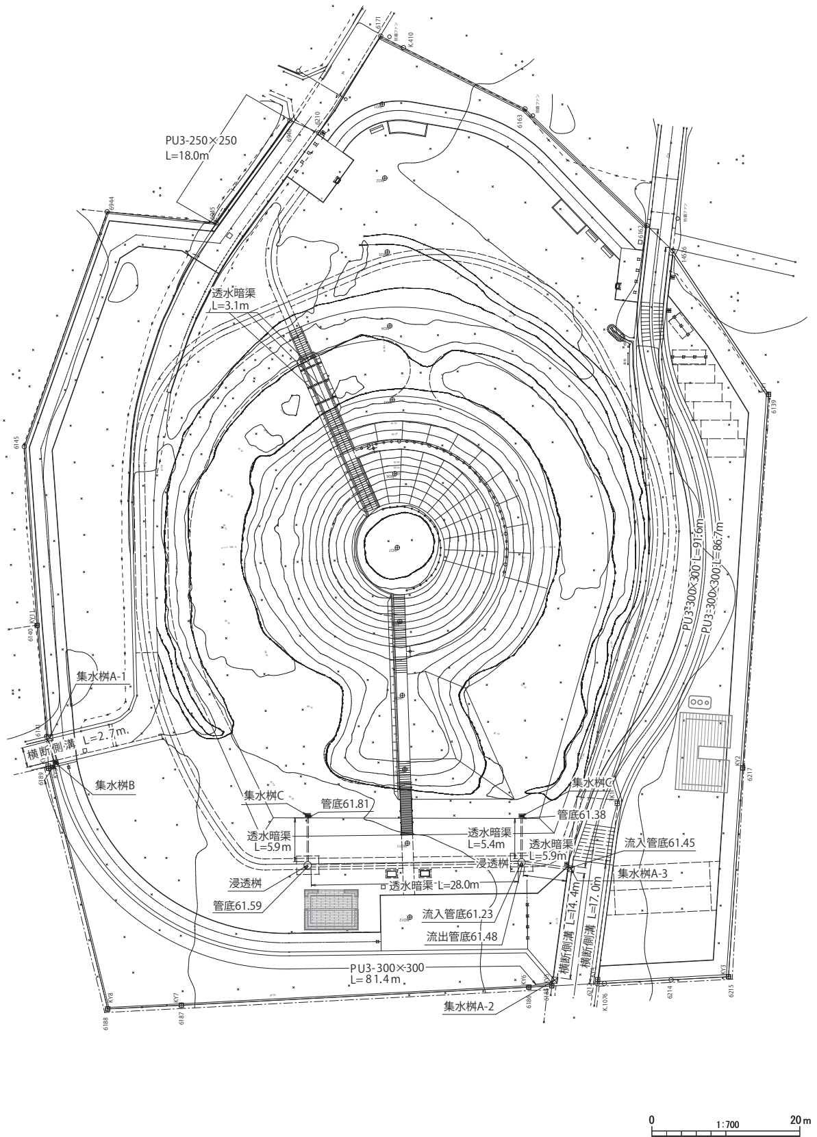
第 35 図 排水計画平面図
