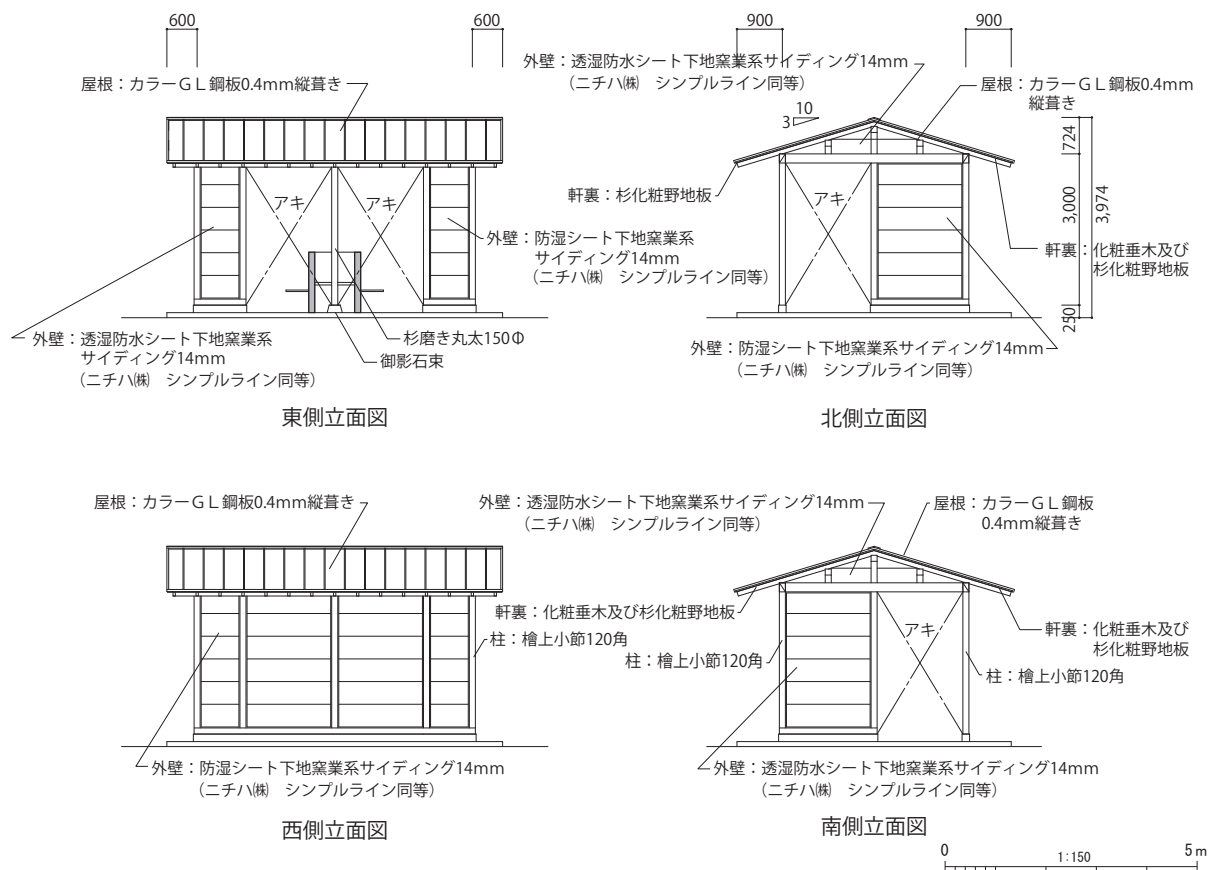
第 85 図 休憩施設立面図
