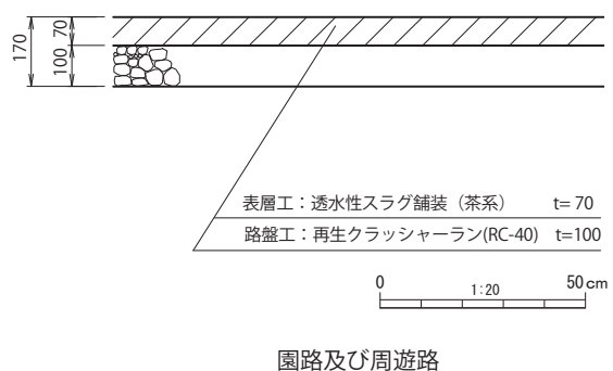
第64図 透水性スラグ舗装工標準断面図
