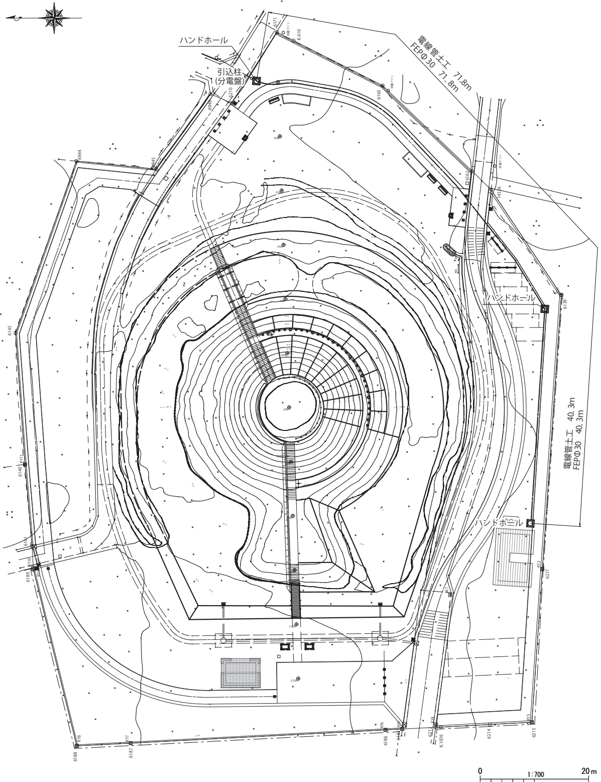
第40図 電気計画平面図
