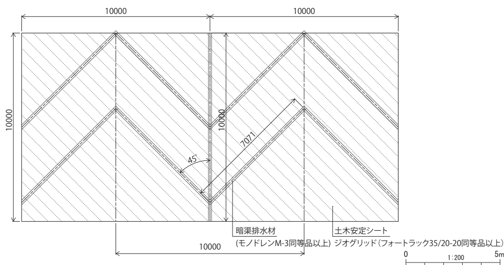
第23図 セパレート材及び排水材の平面施工図
