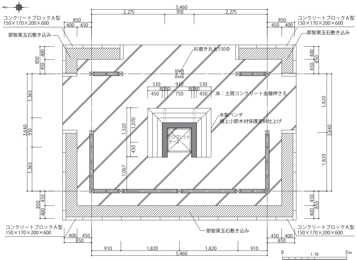
第 84 図 休憩施設全体平面図
