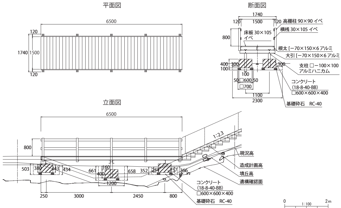
第 69 図 デッキ園路詳細図
