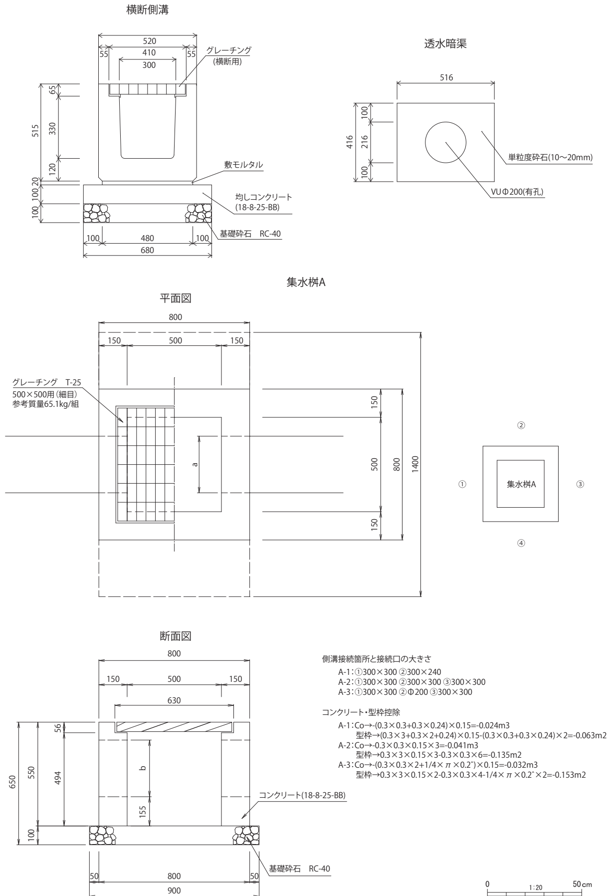
第47図 排水施設構造図(2)
