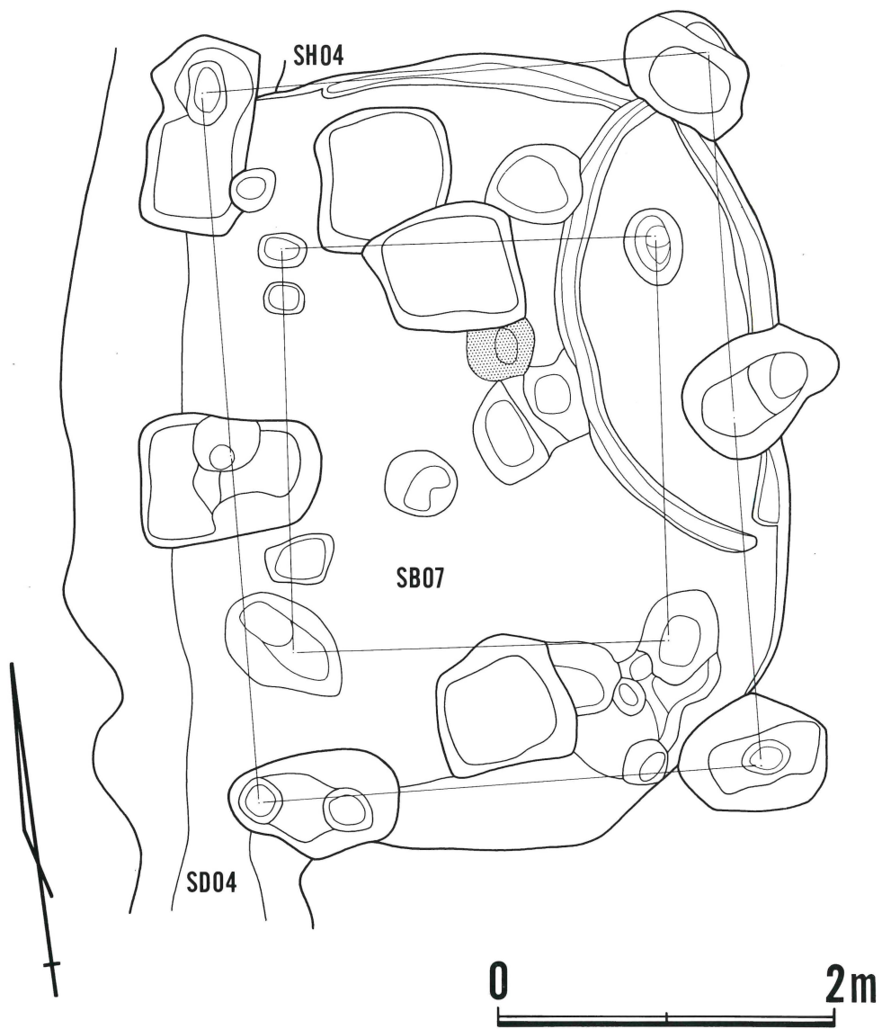
第 4 图 S B 07 平面实测图
