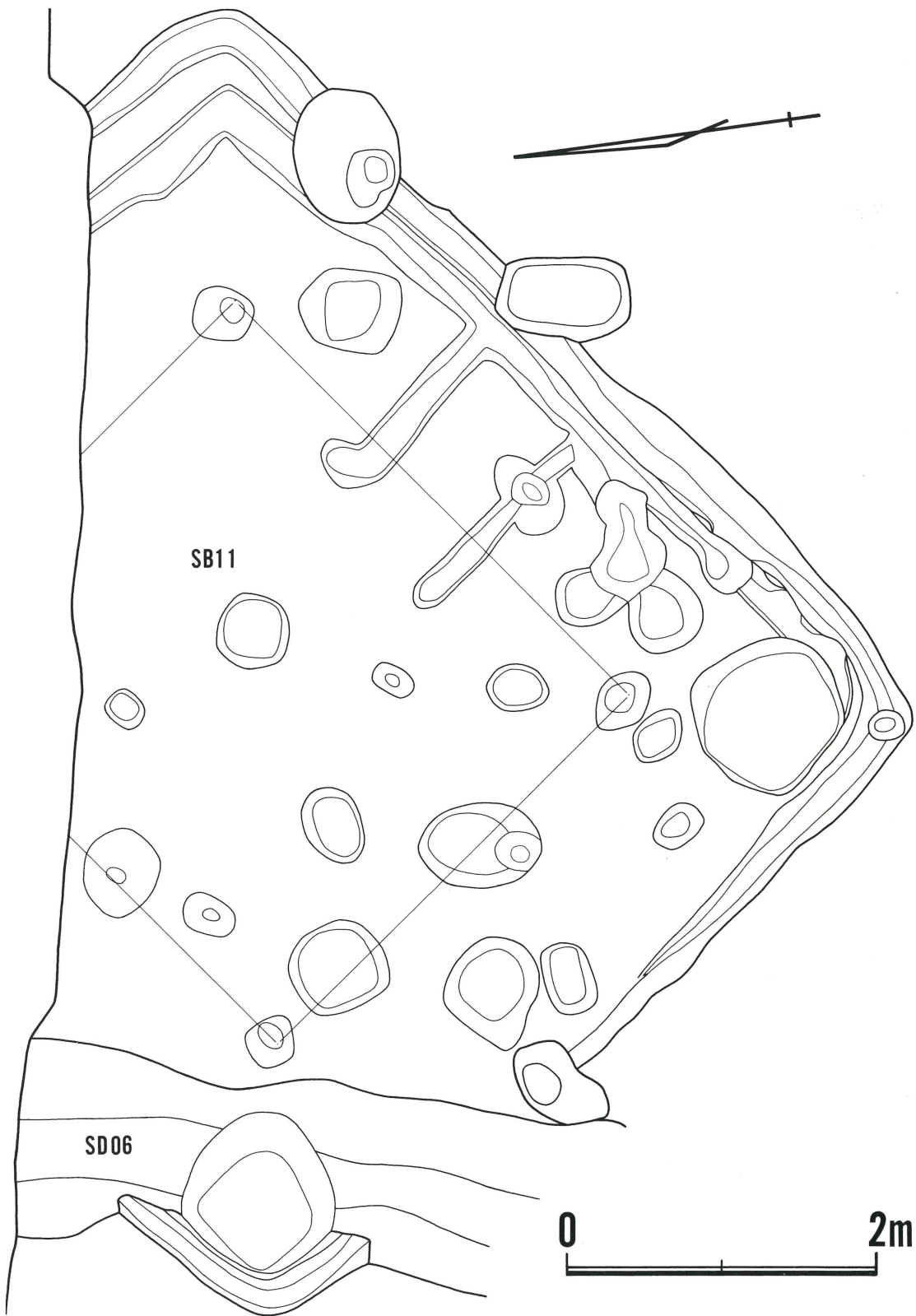
第5図 SB11 平面実測図
