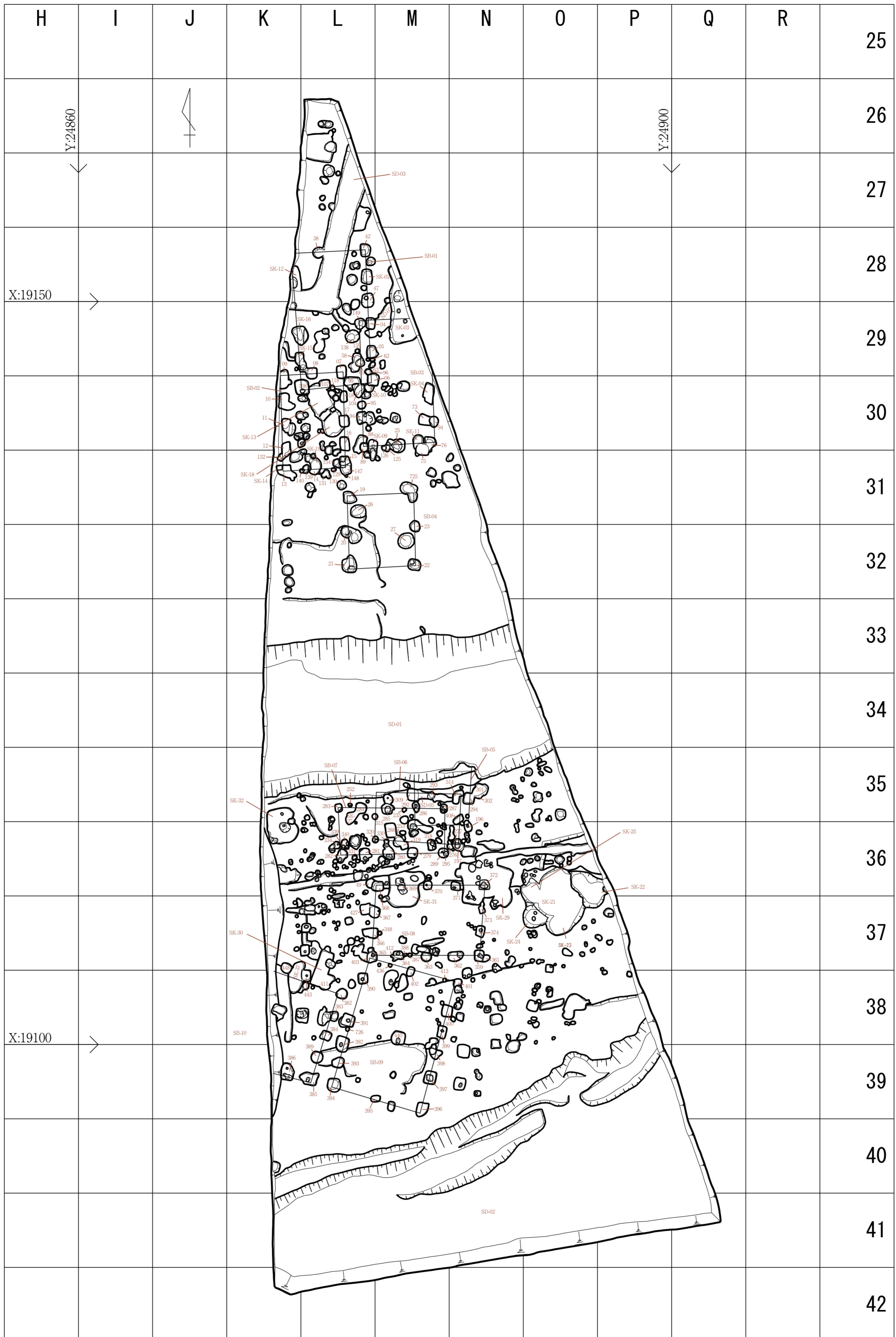
付図2 乗兼・坪江遺跡 2区遺構全体図
