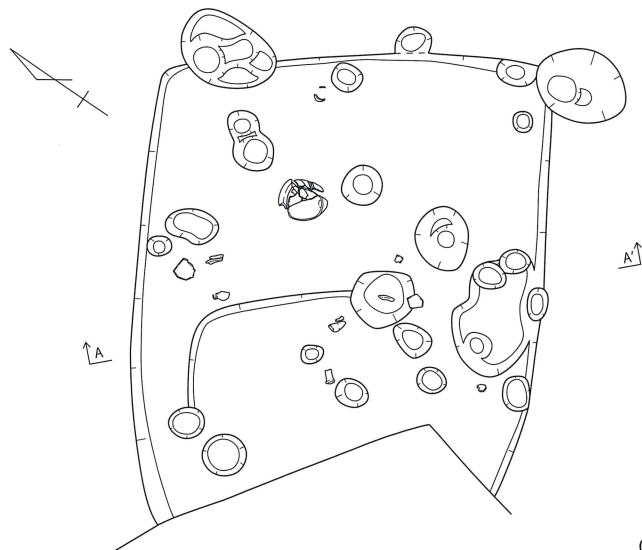
第 396 図 SH104 実測図
