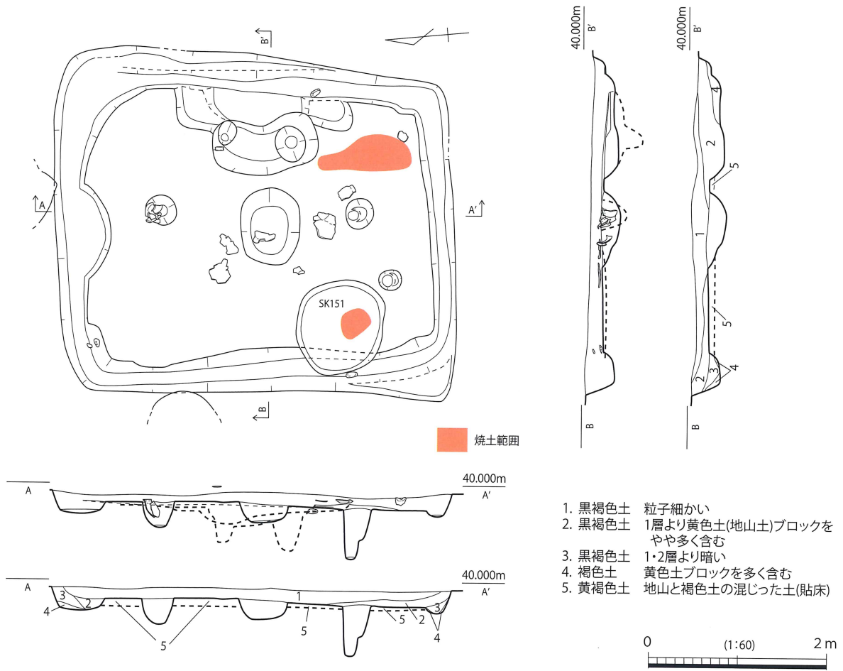
第 365 図 SH064 実測図
