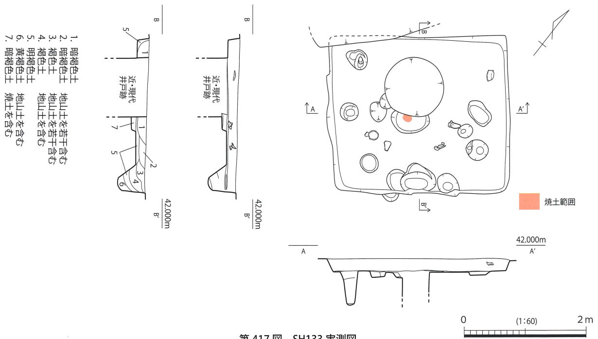
第417図 SH133 実測図
