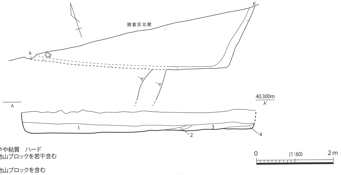
第352図 SH050 実測図
