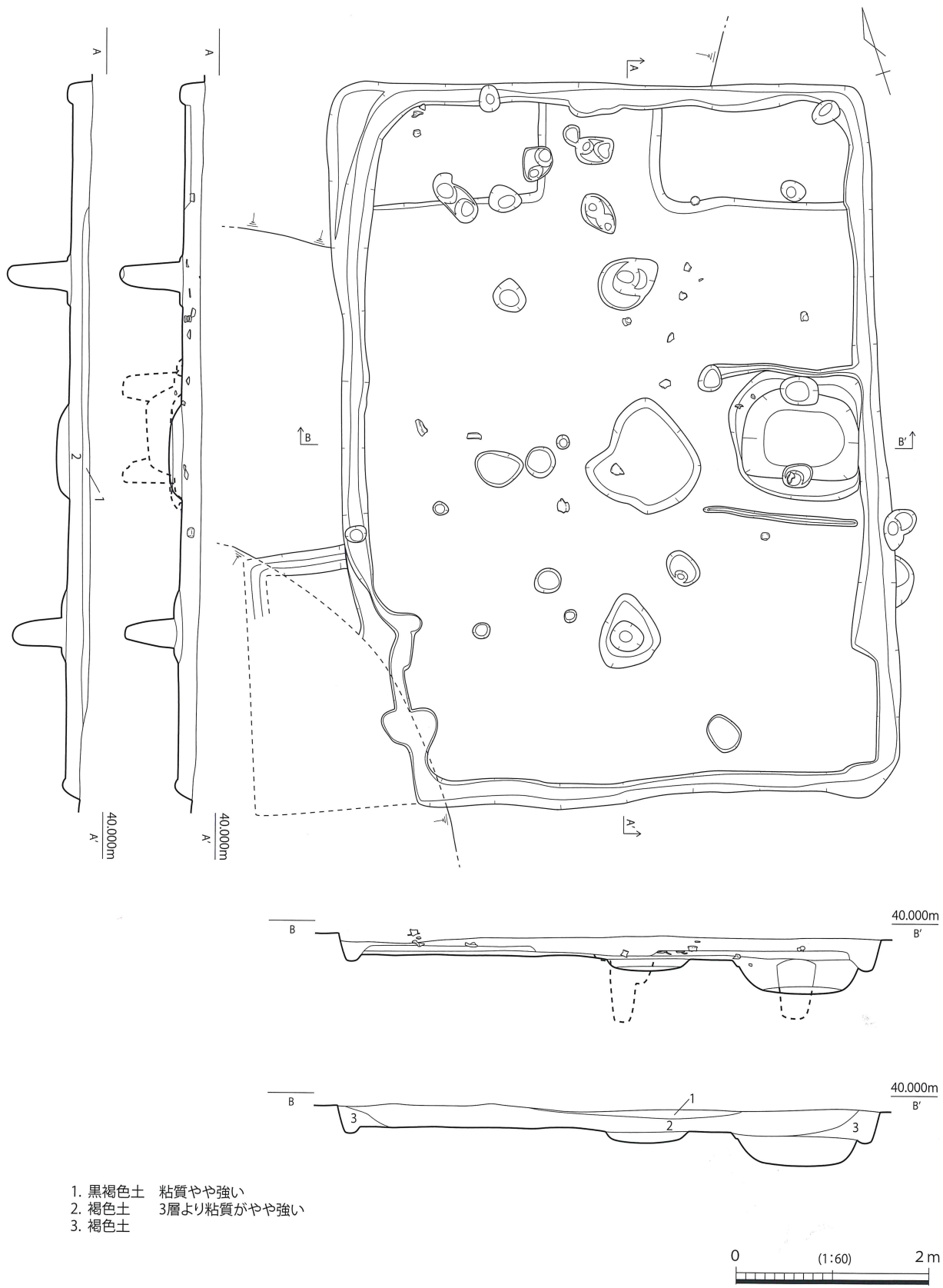
第360図 SH059 実測図
