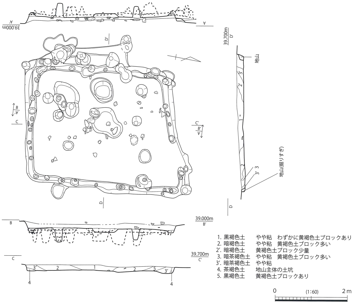
第 316 図 SH013 実測図
