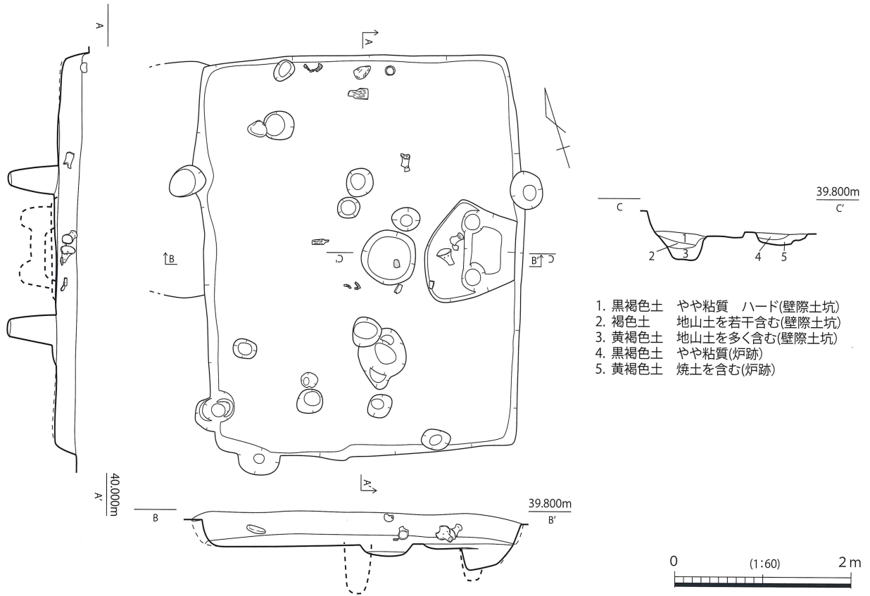
第350図 SH048 実測図
