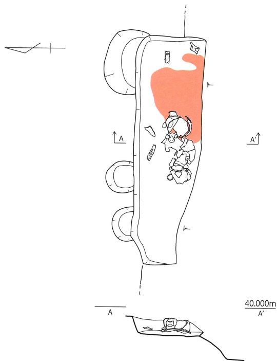
第 376 図 SH080 実測図
