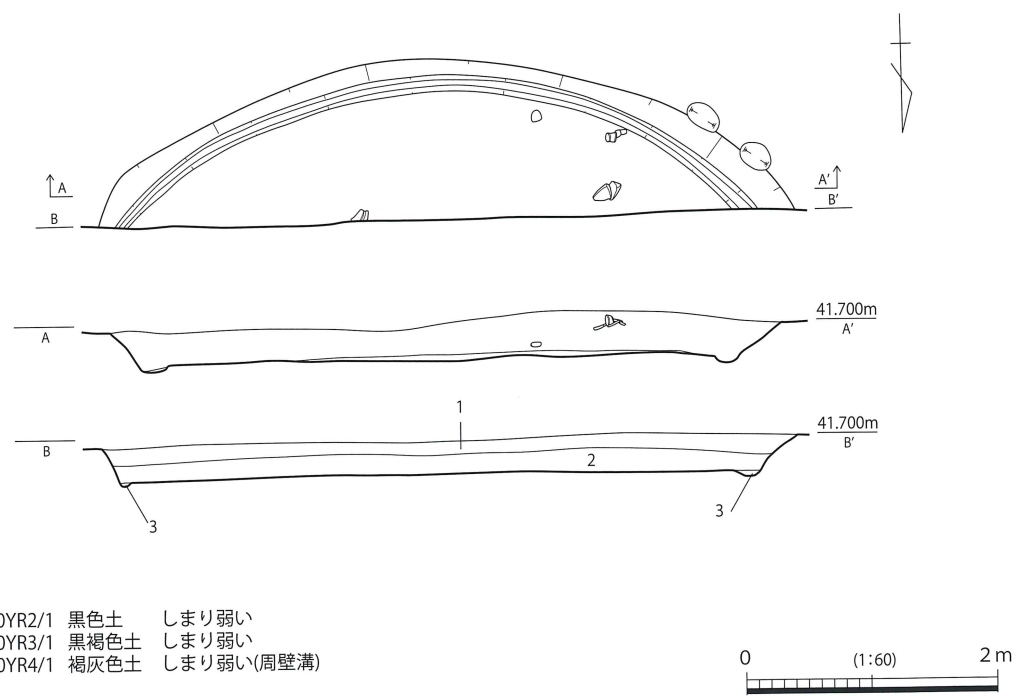
第 427 図 SH138 実測図
