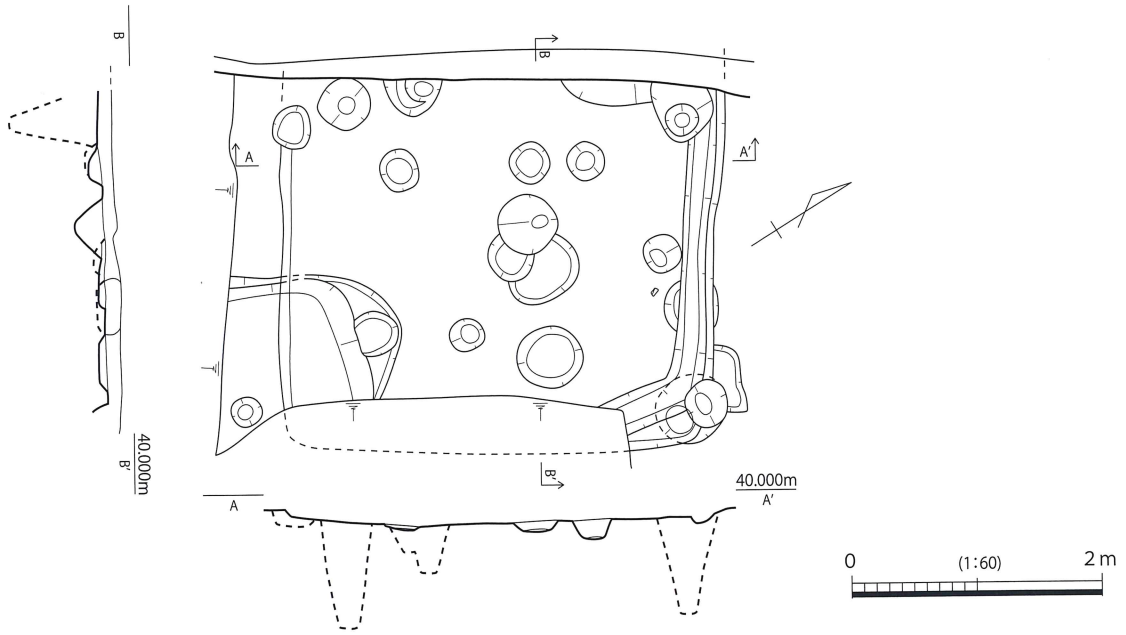
第 385 図 SH085 実測図
