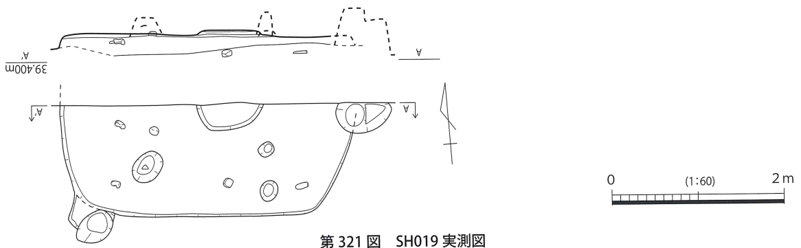
第 321 图 SH019 实测图
