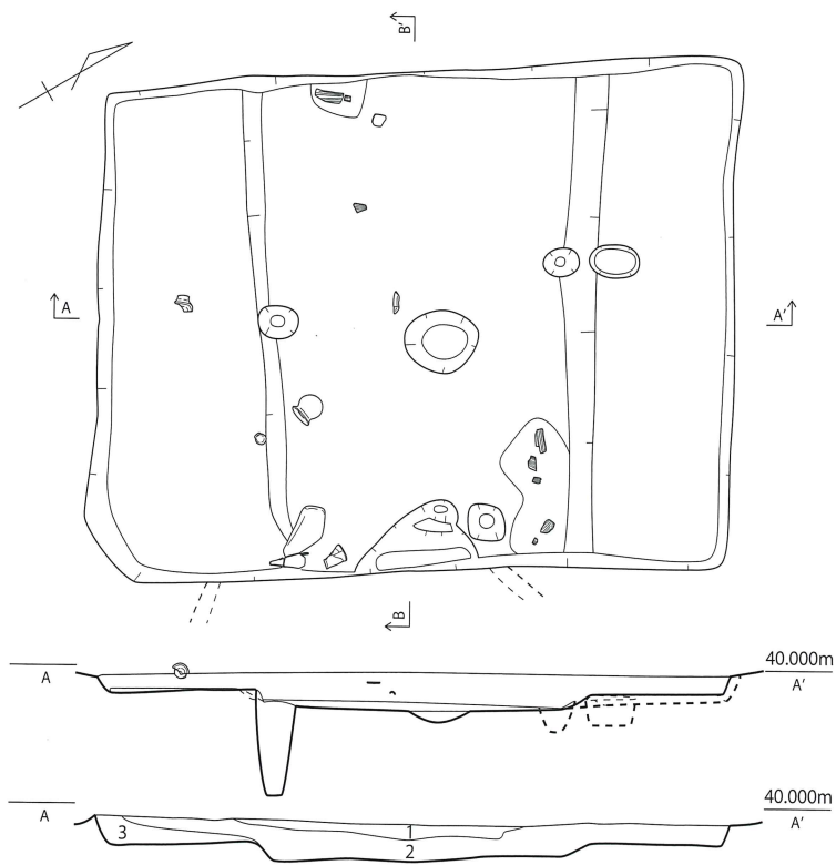
第392図 SH098 実測図
