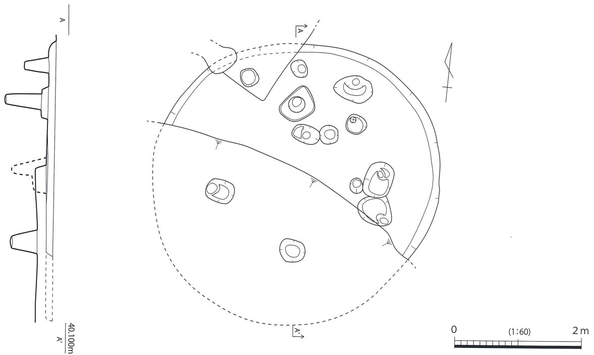
第 366 図 SH065 実測図
