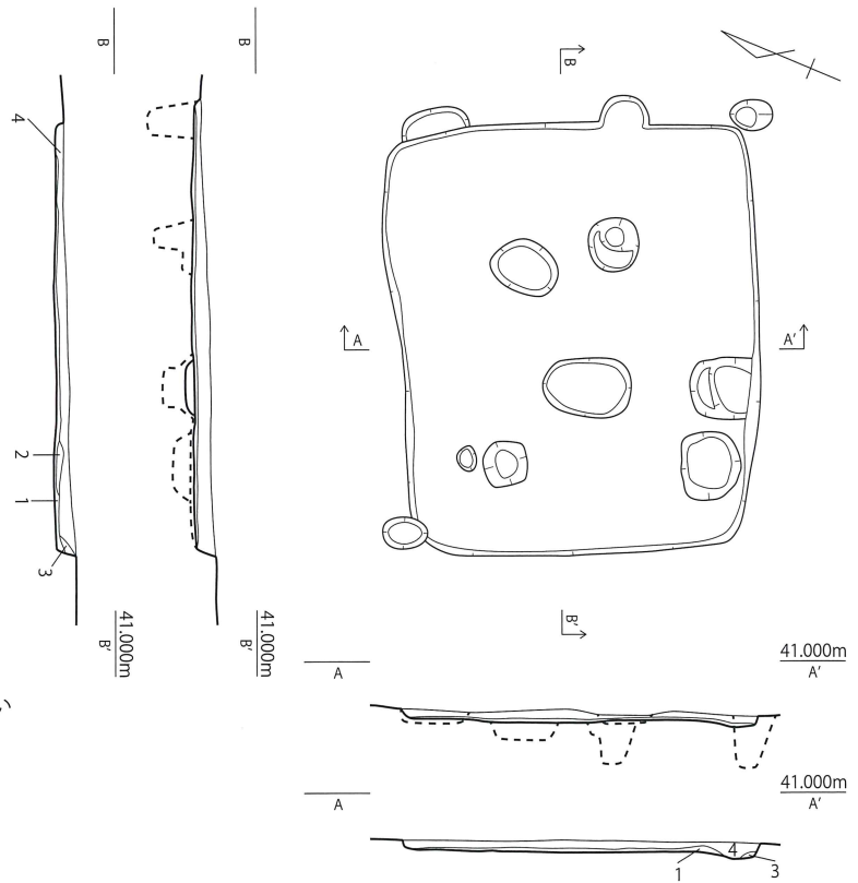
第 413 図 SH124 実測図
