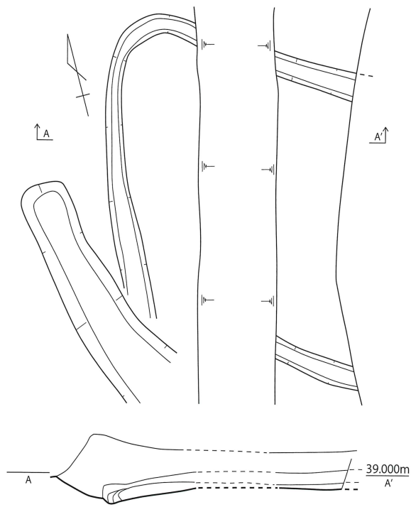
第 389 图 SH094 实测图
