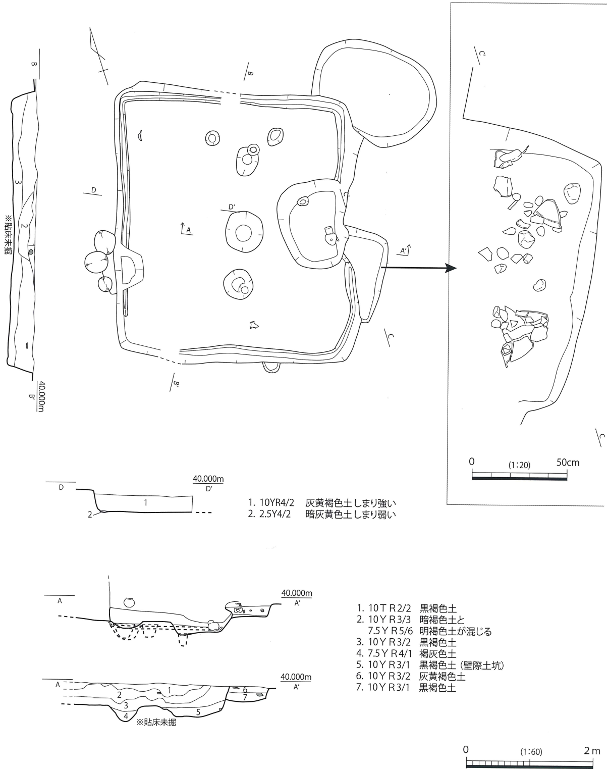
第 380 図 SH078 実測図
