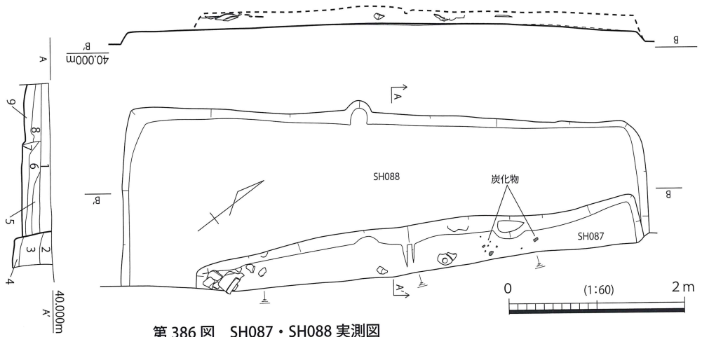
第 386 図 SH087・SH088 実測図
