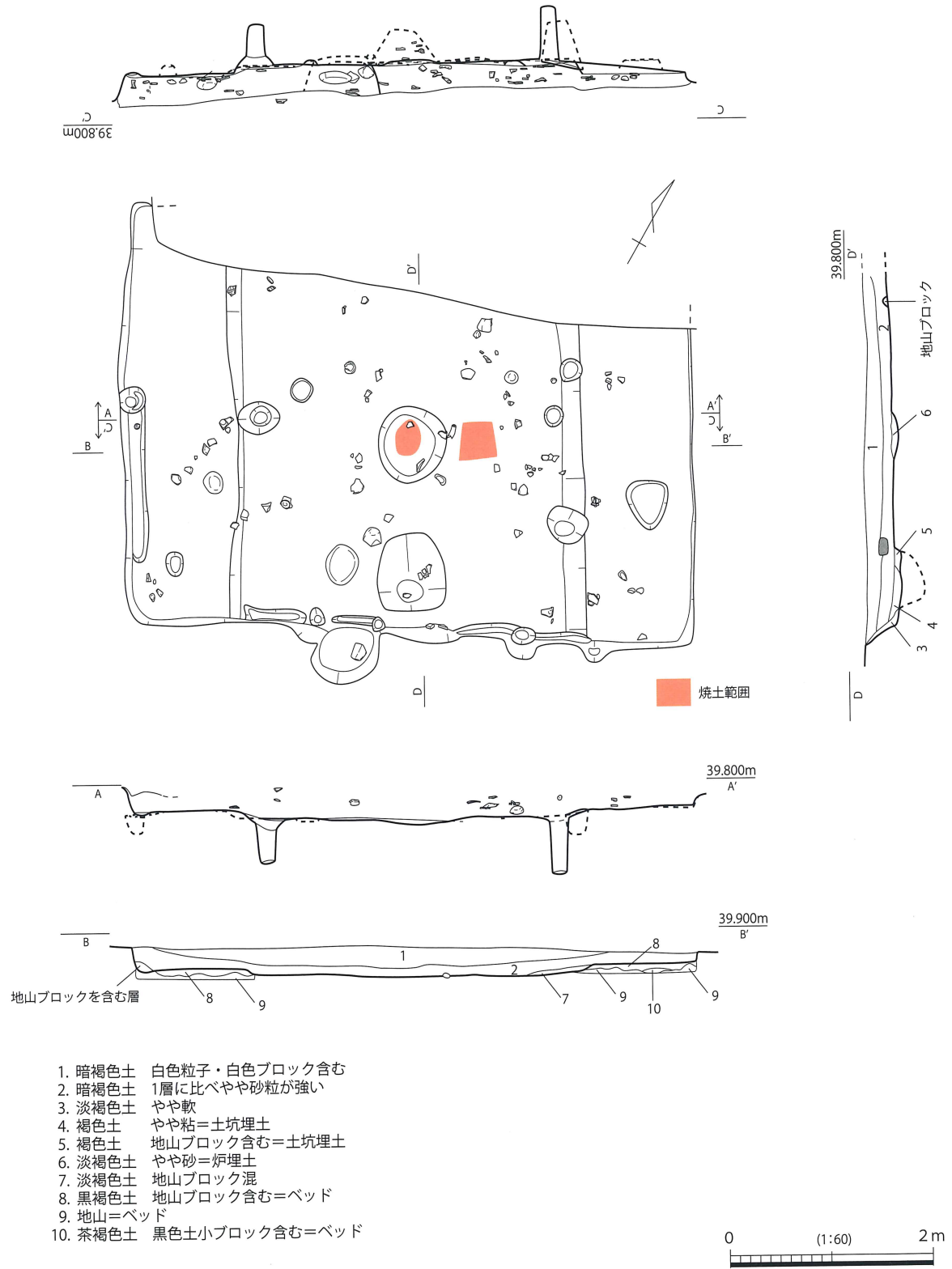
第 364 図 SH062 実測図
