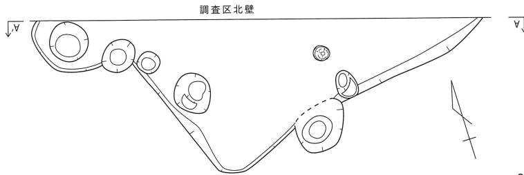
第 381 図 SH081 実測図
