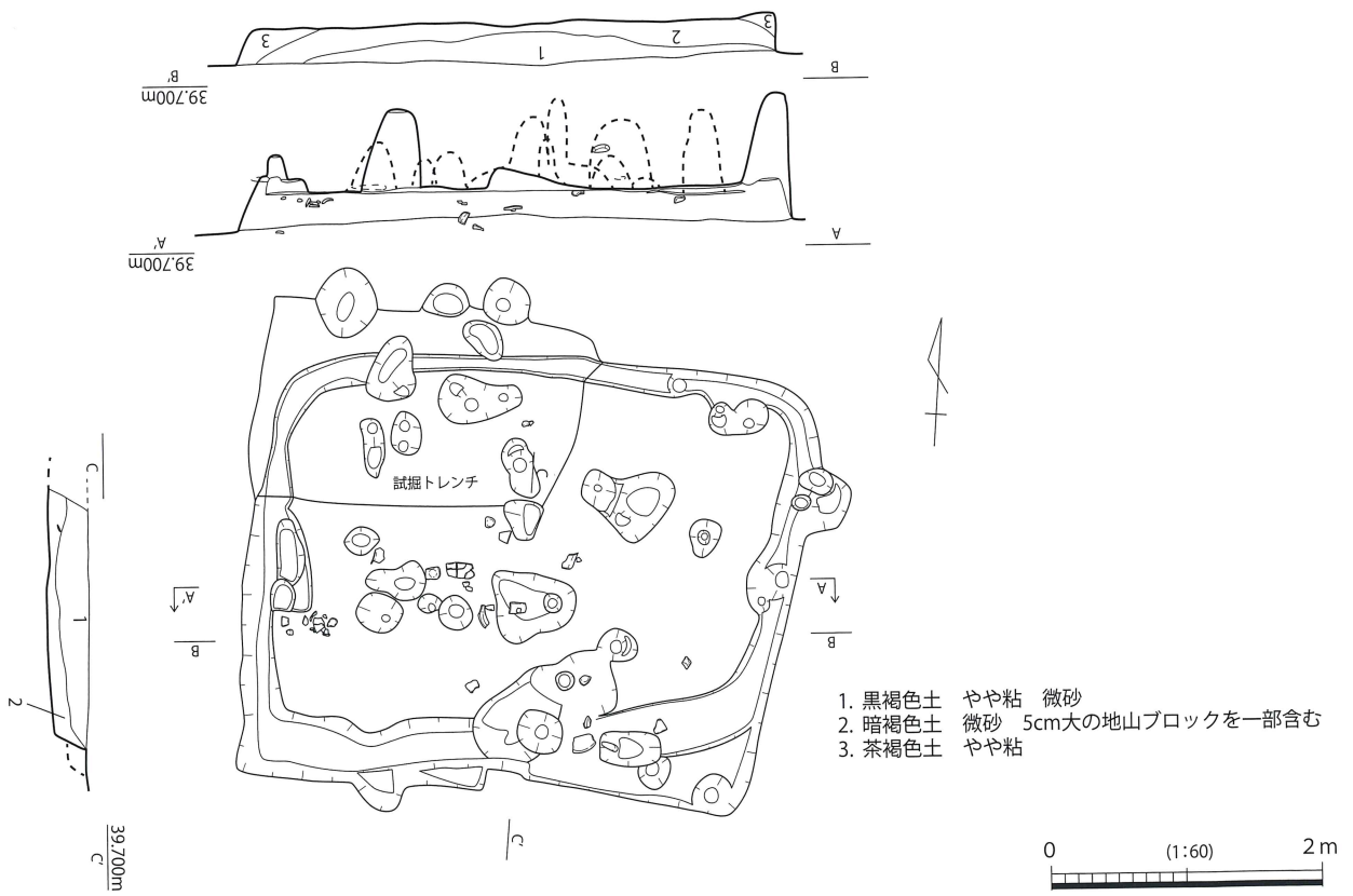
第 337 図 SH037 実測図
