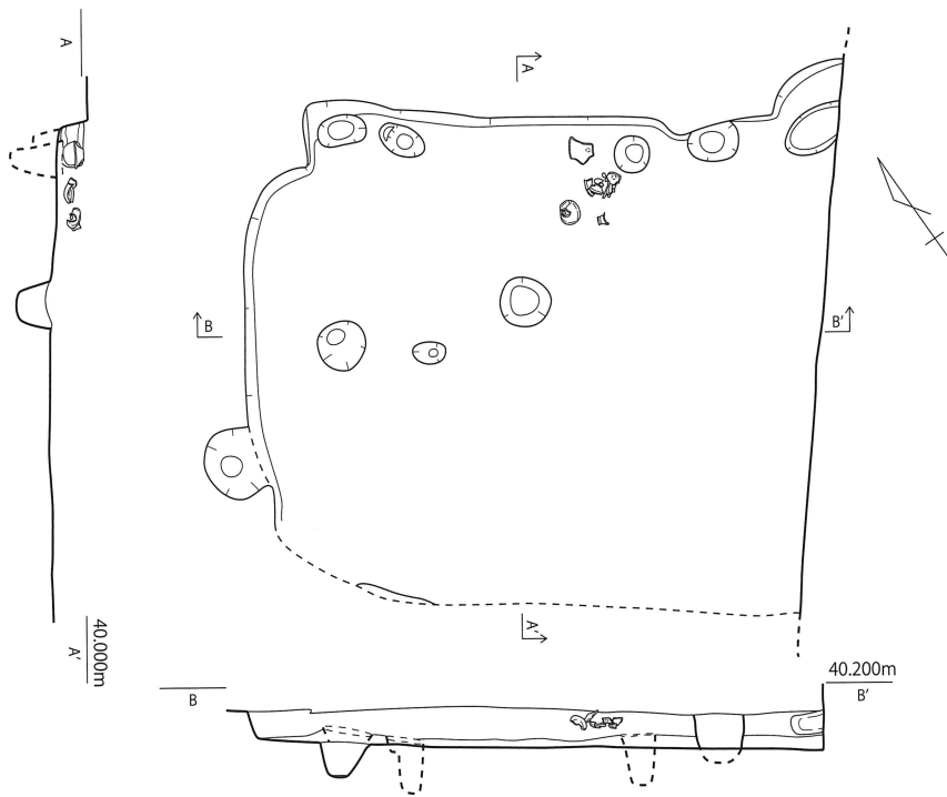
第 381 図 SH081 実測図
