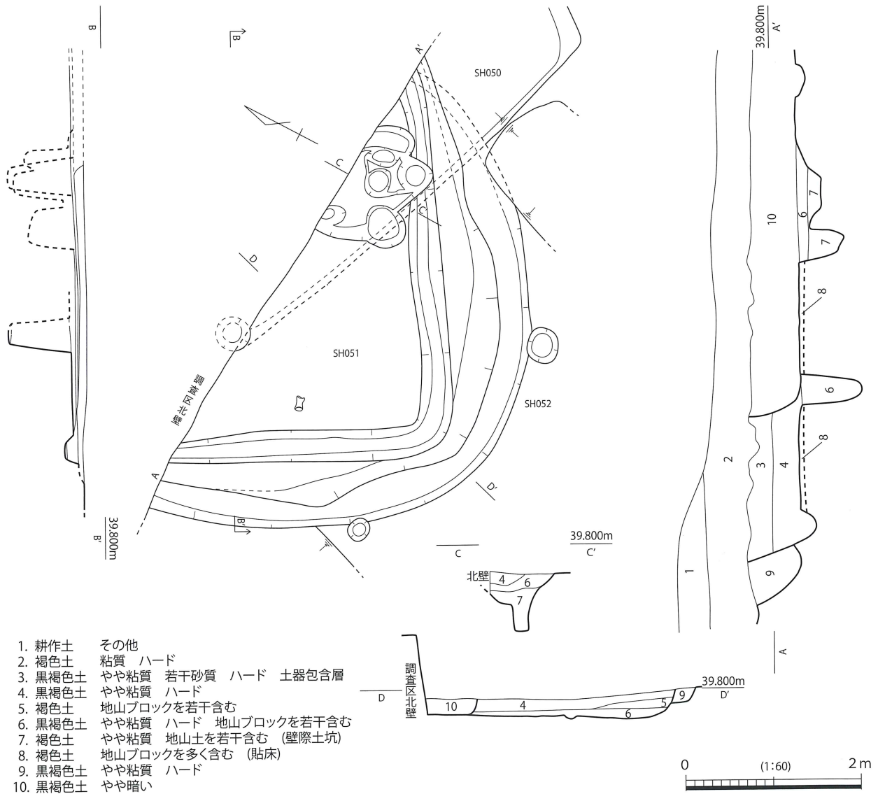
第353図 SH051・SH052 実測図
