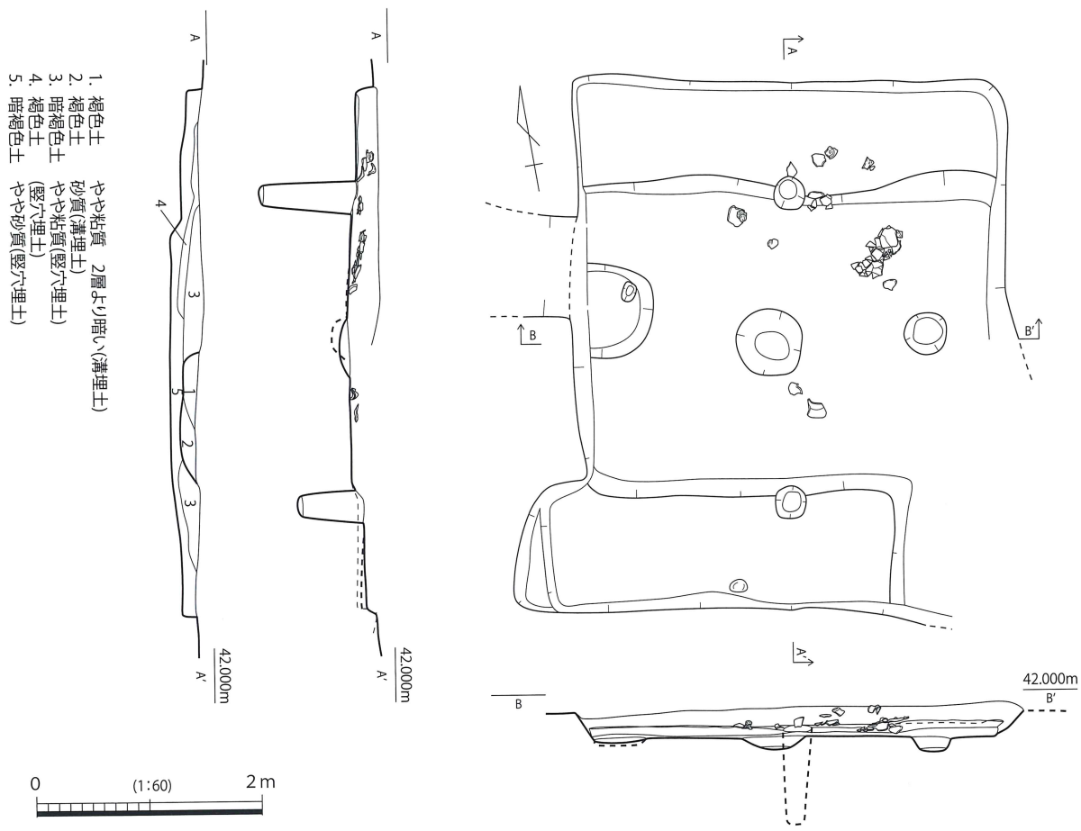
第 426 図 SH137 実測図
