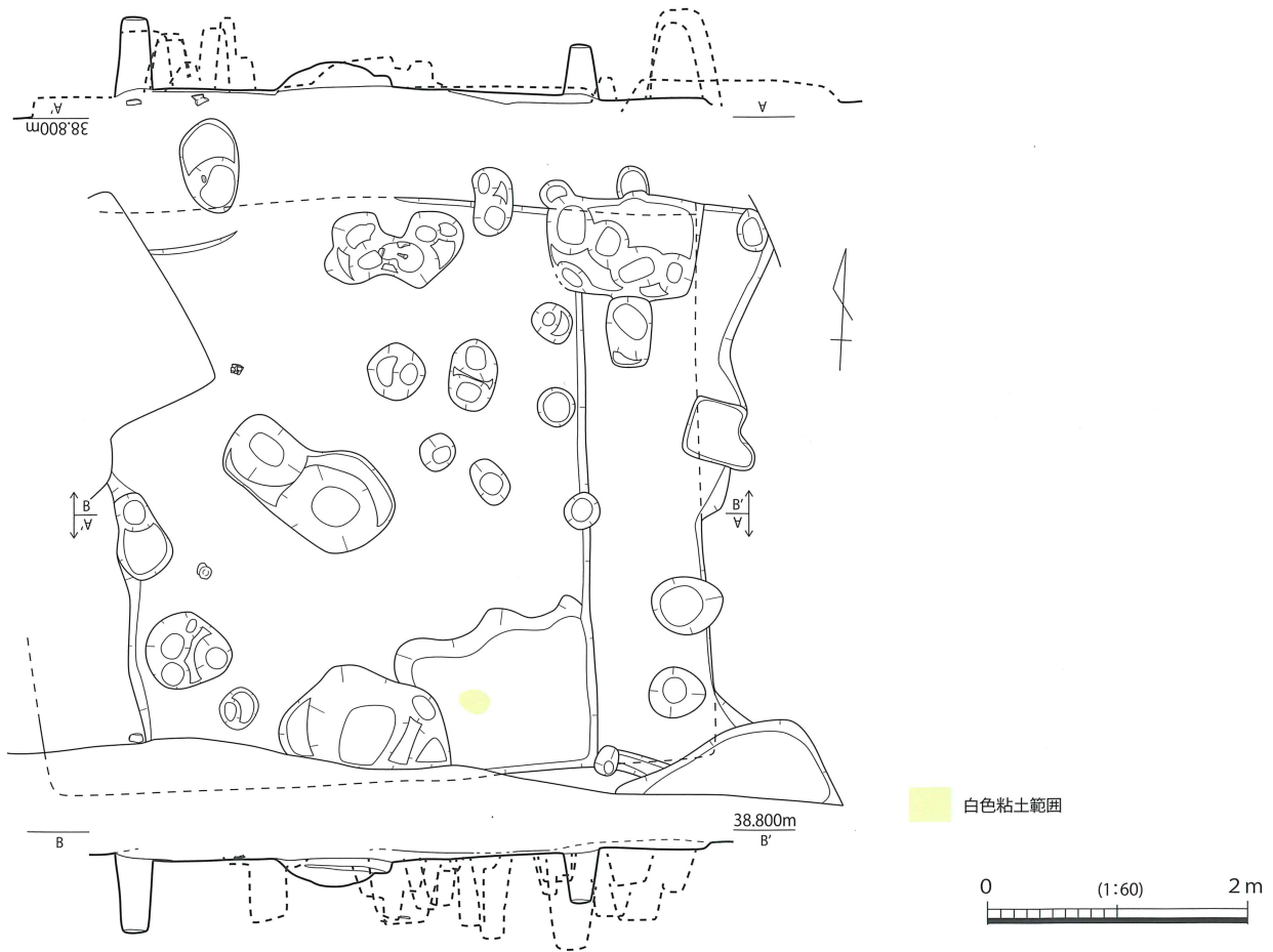
第 305 図 SH002 実測図
