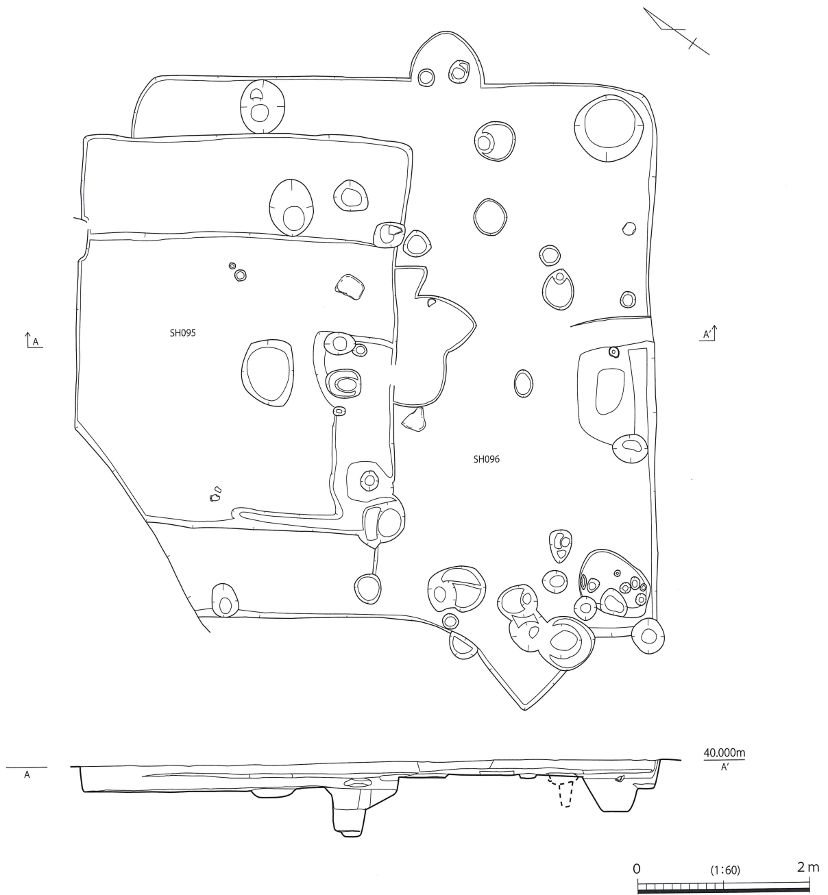
第 390 図 SH095・SH096 実測図
