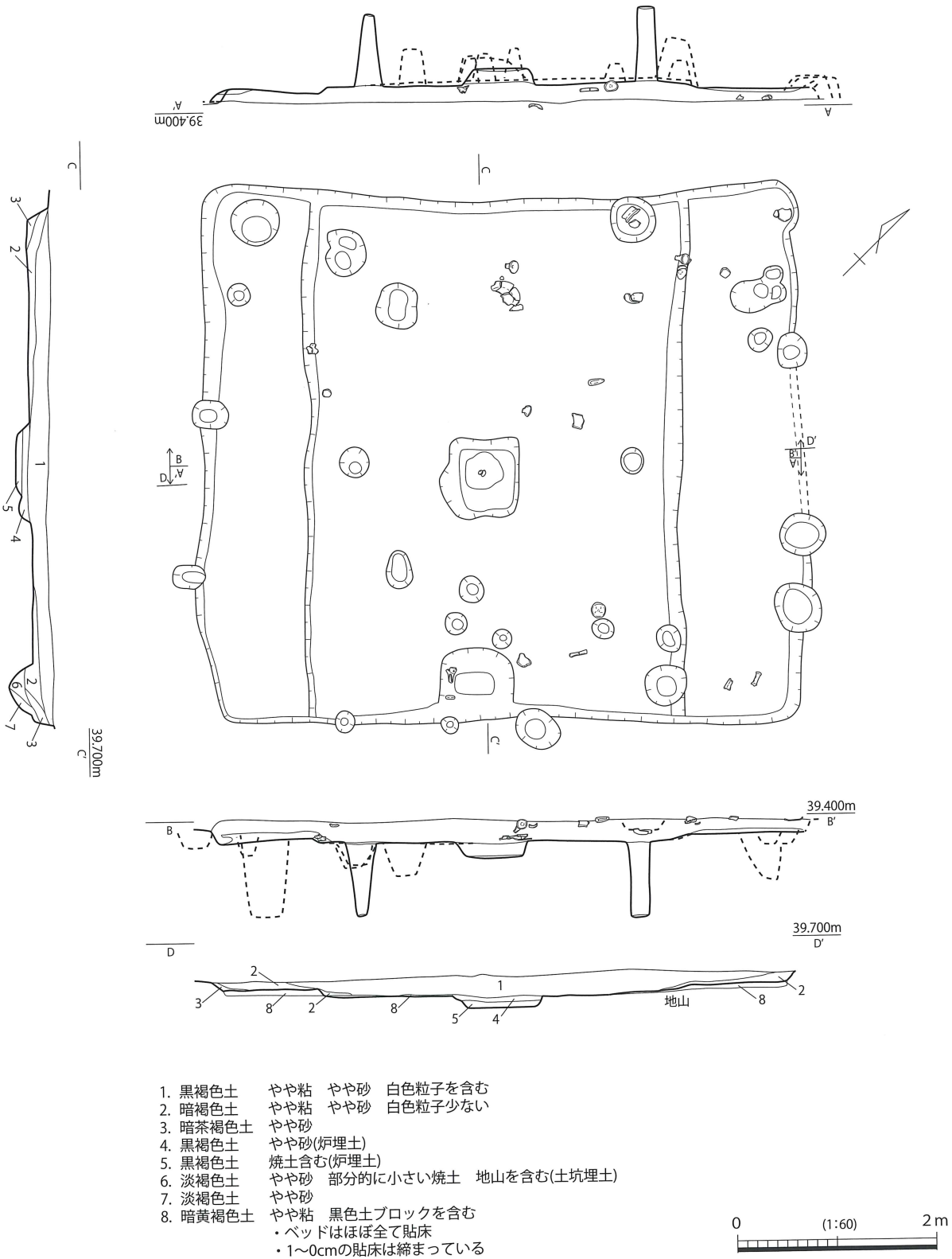
第 327 図 SH025 実測図
