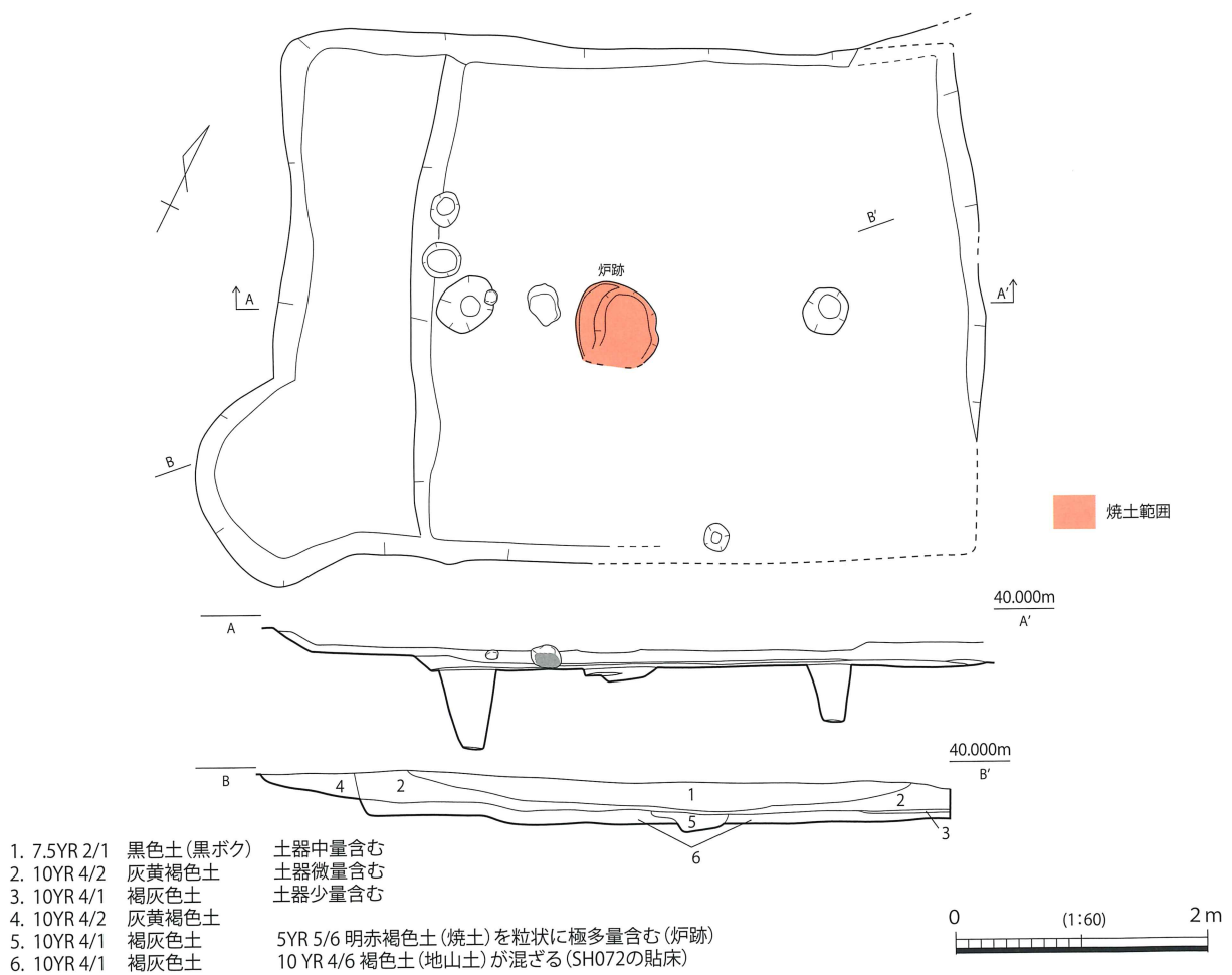
第 374 図 SH073 実測図
