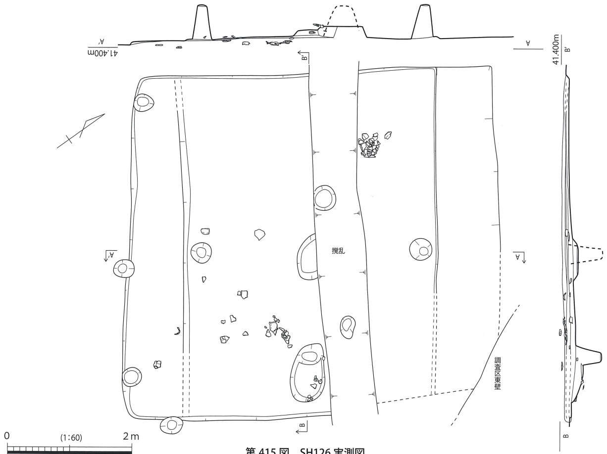
第415図 SH126 実測図
