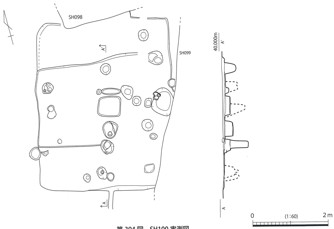
第 394 図 SH100 実測図
