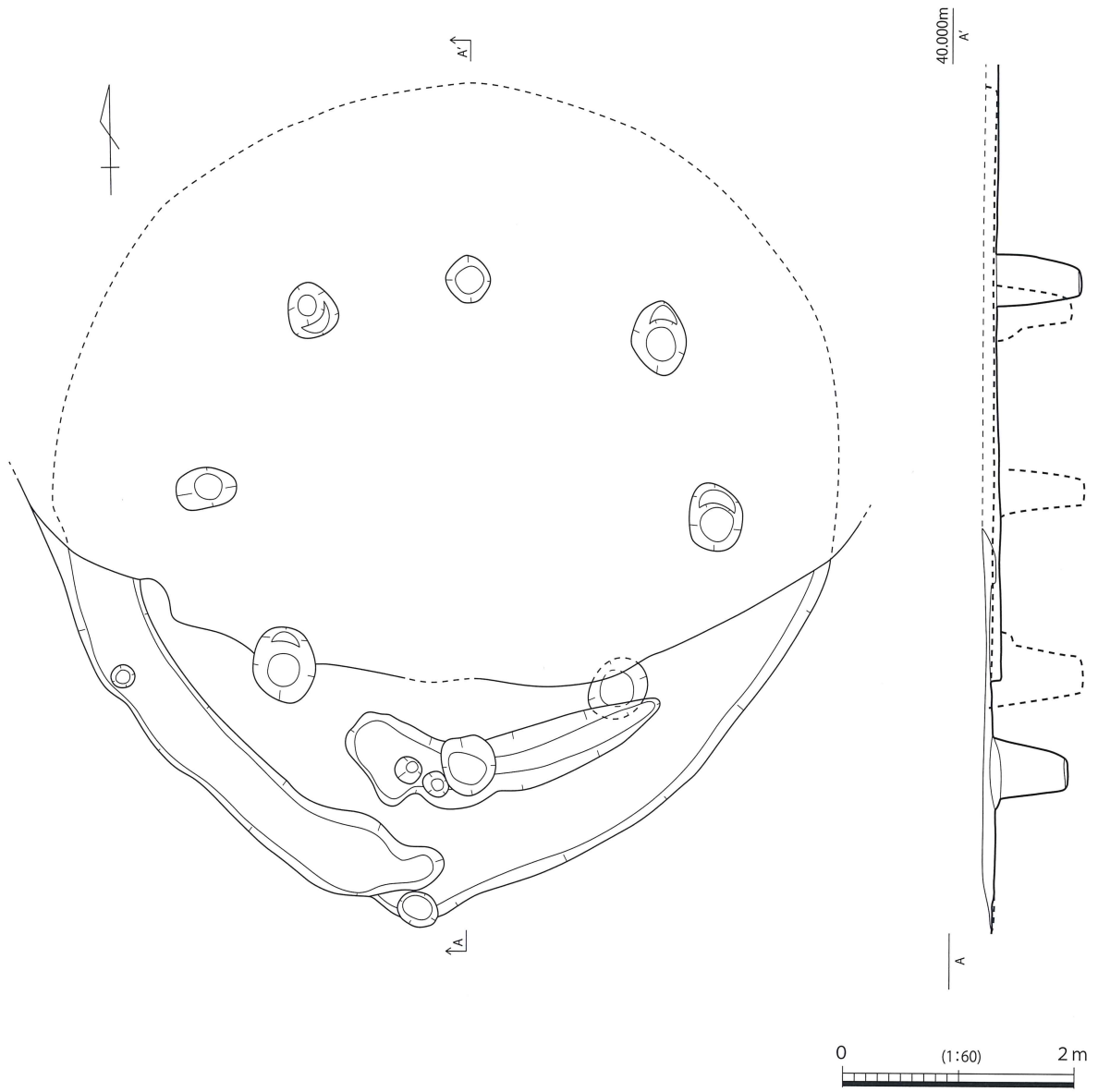
第 368 图 SH067 实测图
