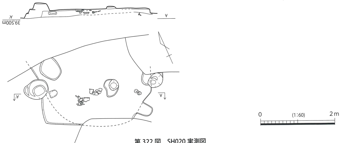
第 322 图 SH020 实测图
