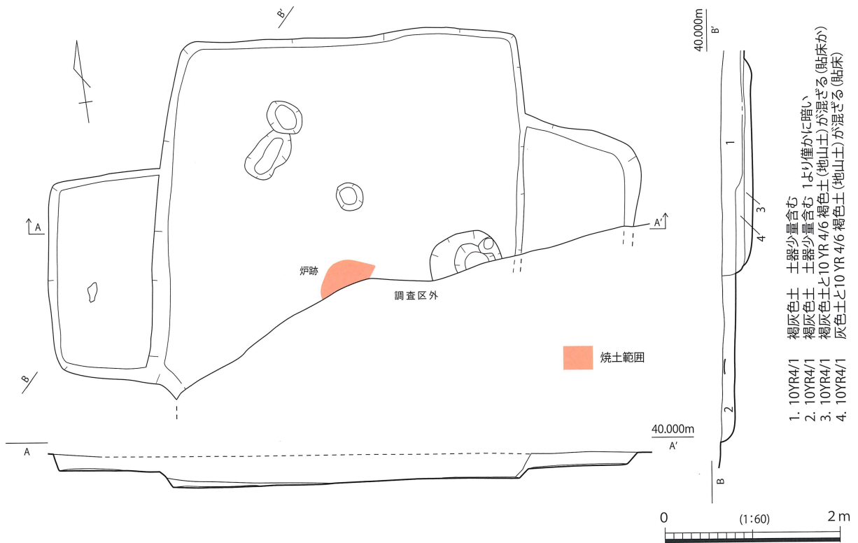
第 373 図 SH072 実測図
