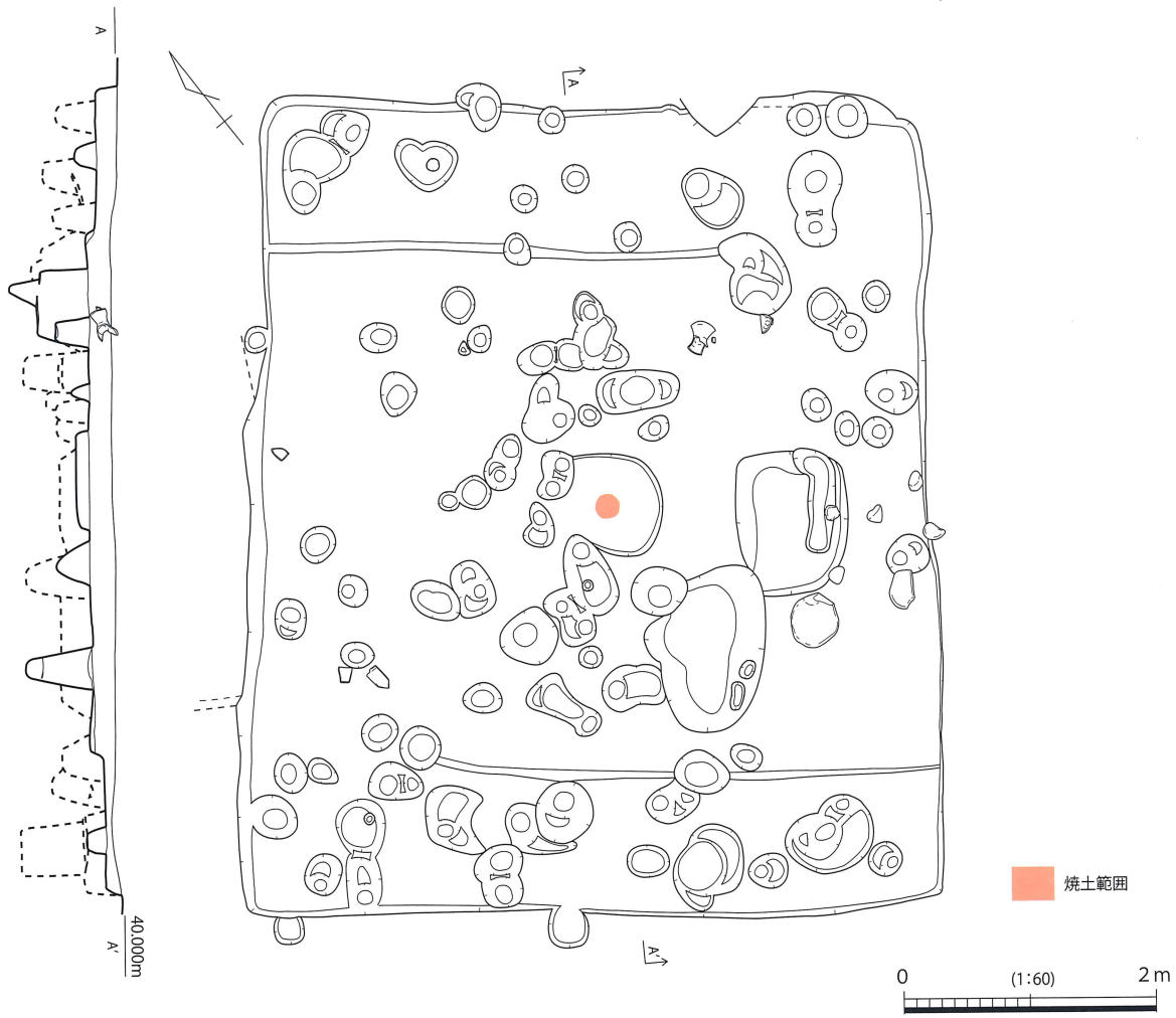
第 393 図 SH099 実測図
