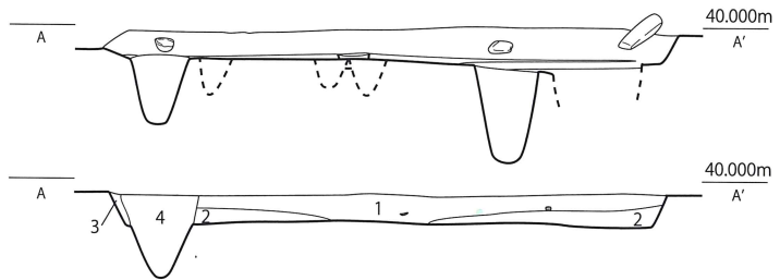
第 395 図 SH101 実測図
