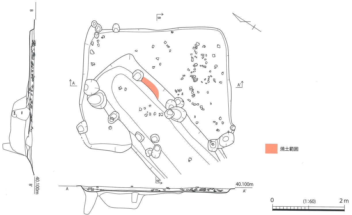
第408図 SH116実測図
