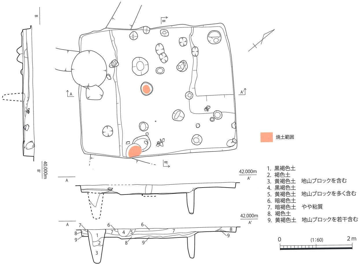
第 423 図 SH134 実測図
