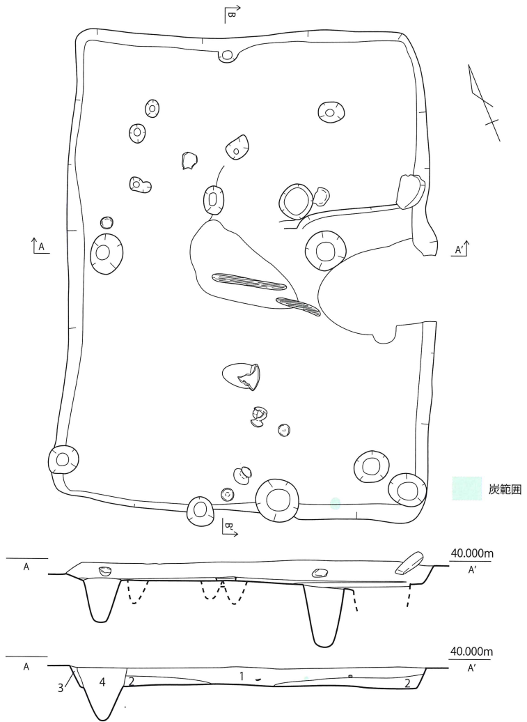
第 395 図 SH101 実測図
