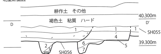
北壁断面図
