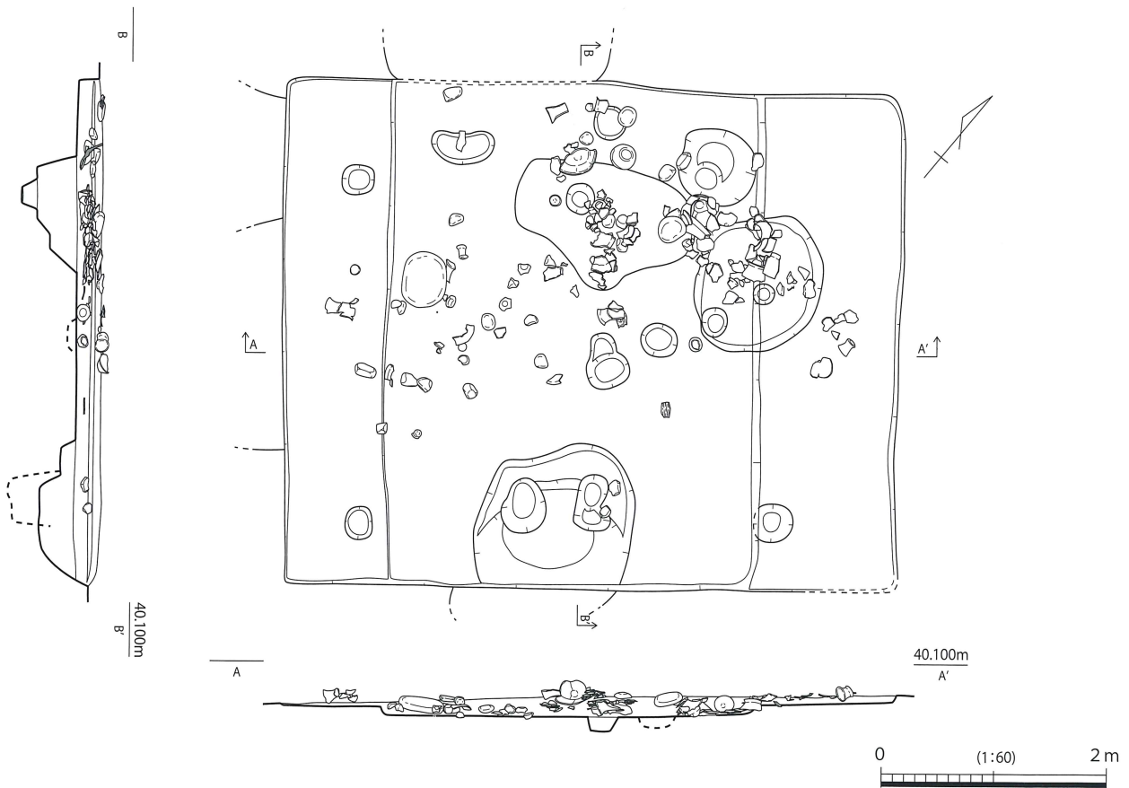
第351図 SH049 実測図
