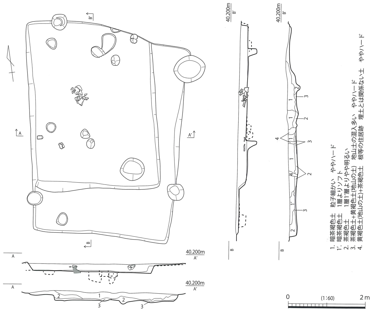
第409図 SH117実測図
