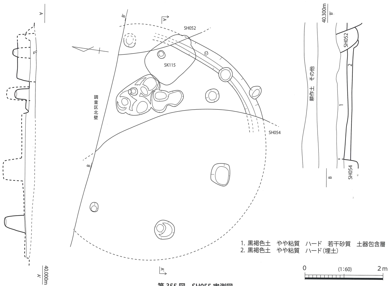
第 355 図 SH055 実測図
