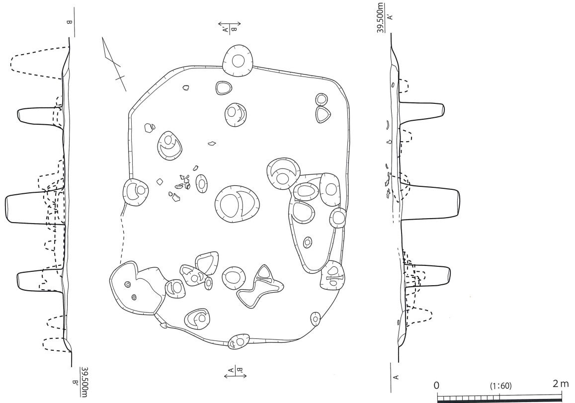
第 336 図 SH034 実測図
