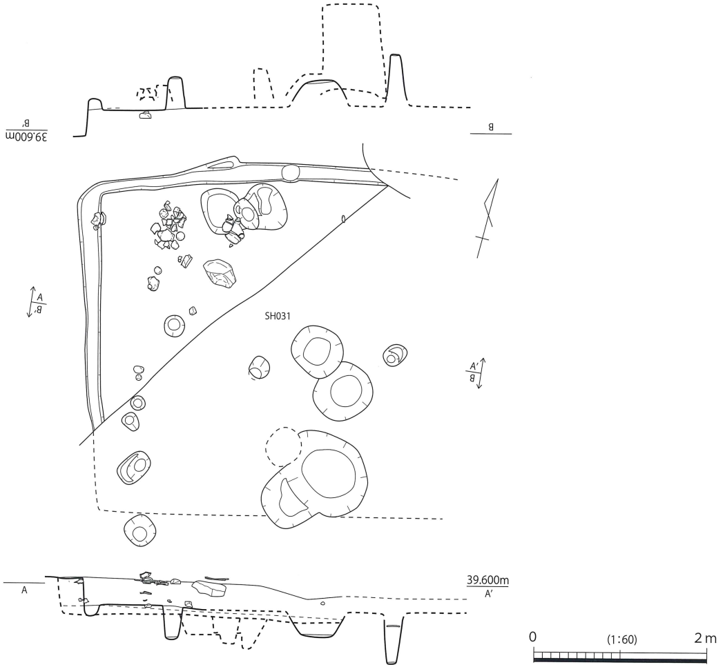
第 334 图 SH032 实测图
