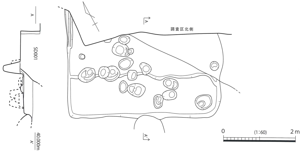
第401図 SH109実測図
