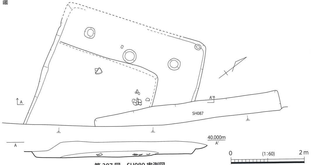
第 387 図 SH089 実測図
