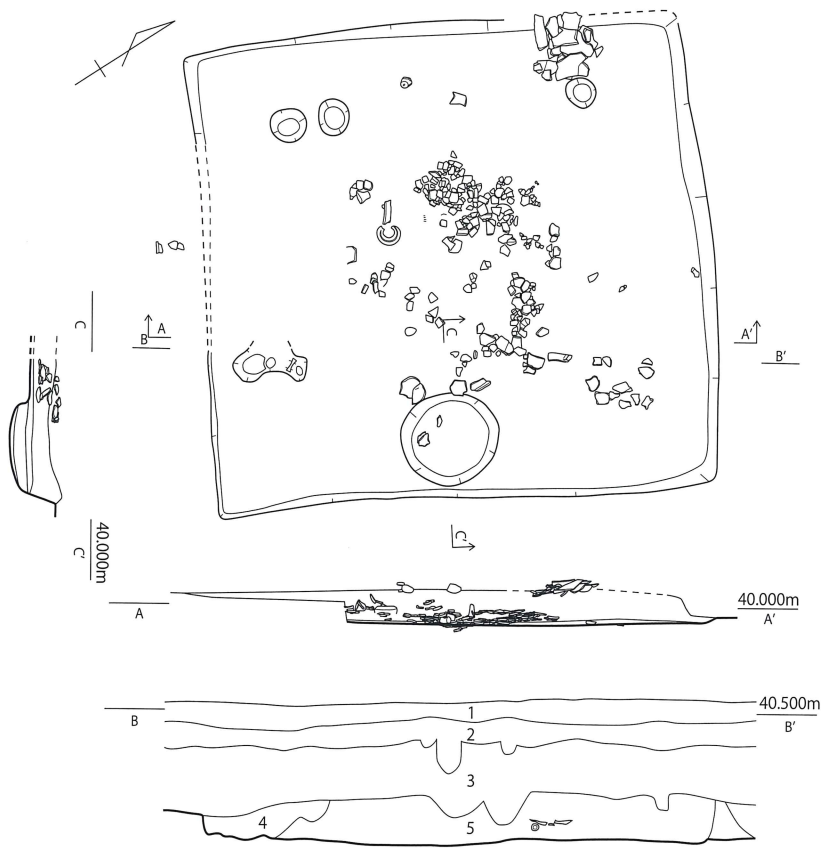
第 388 图 SH090 实测图
