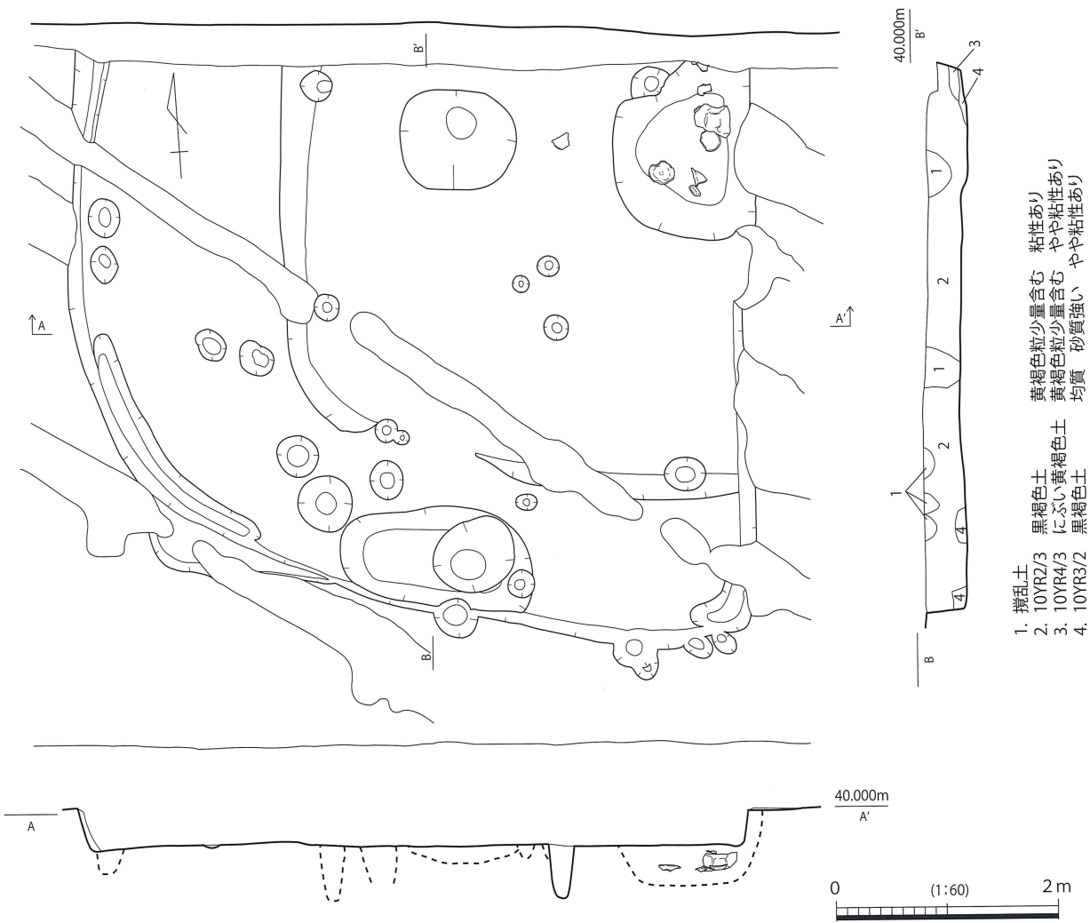
第406図 SH114 実測図
