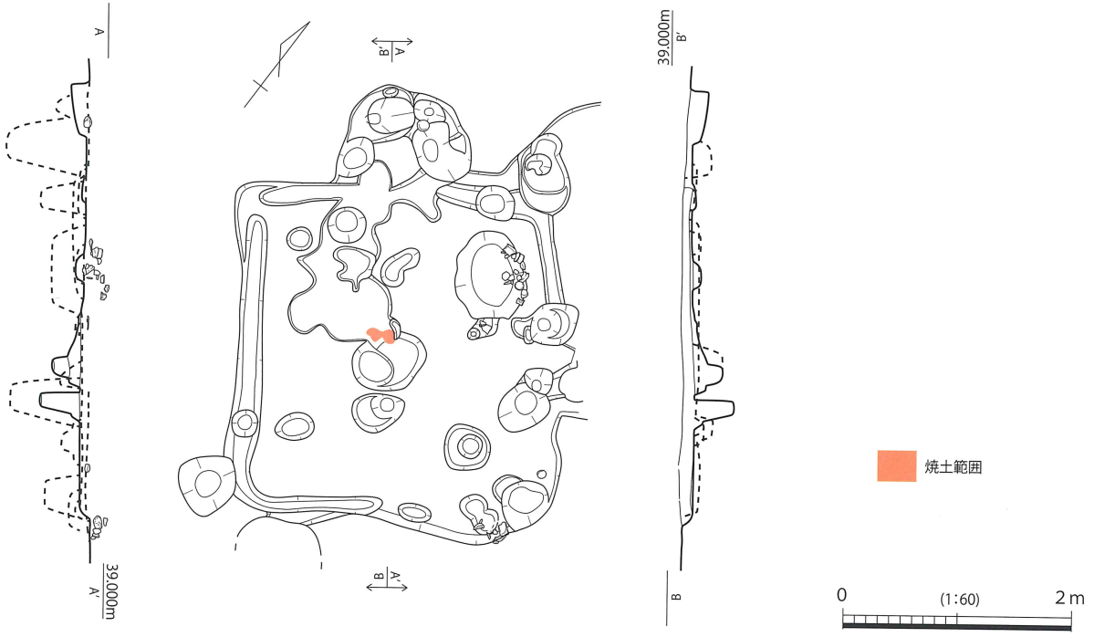
第313図 SH006 実測図
