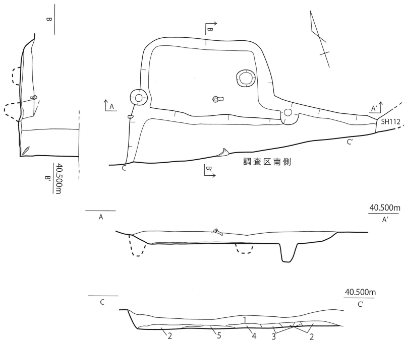
第 405 図 SH113 実測図
