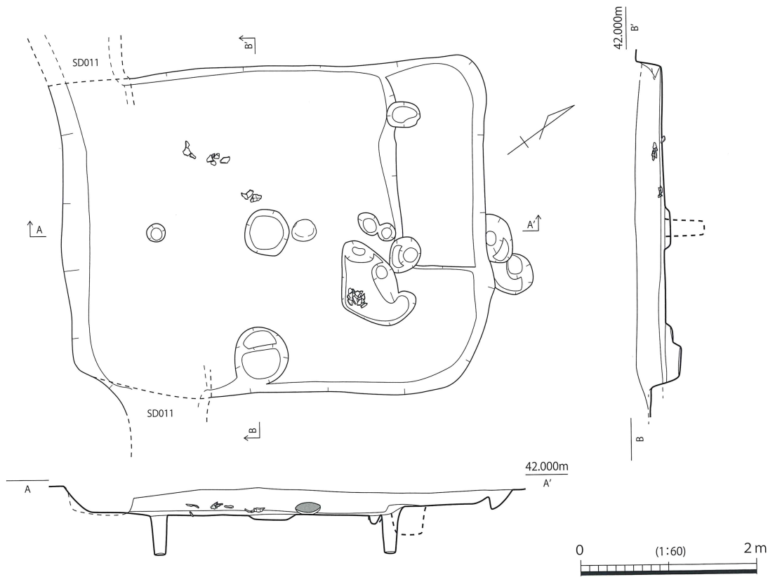
第 424 図 SH136 実測図
