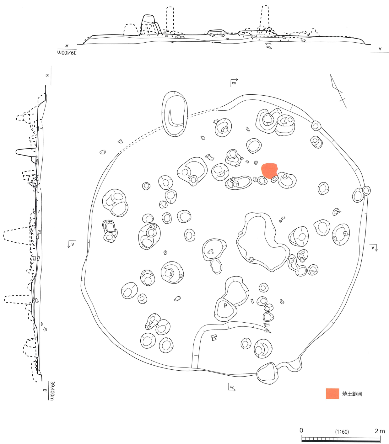
第 319 図 SH017 実測図
