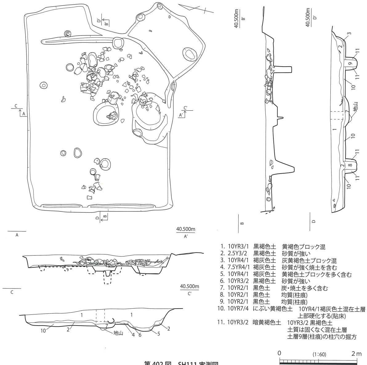
第402図 SH111実測図
