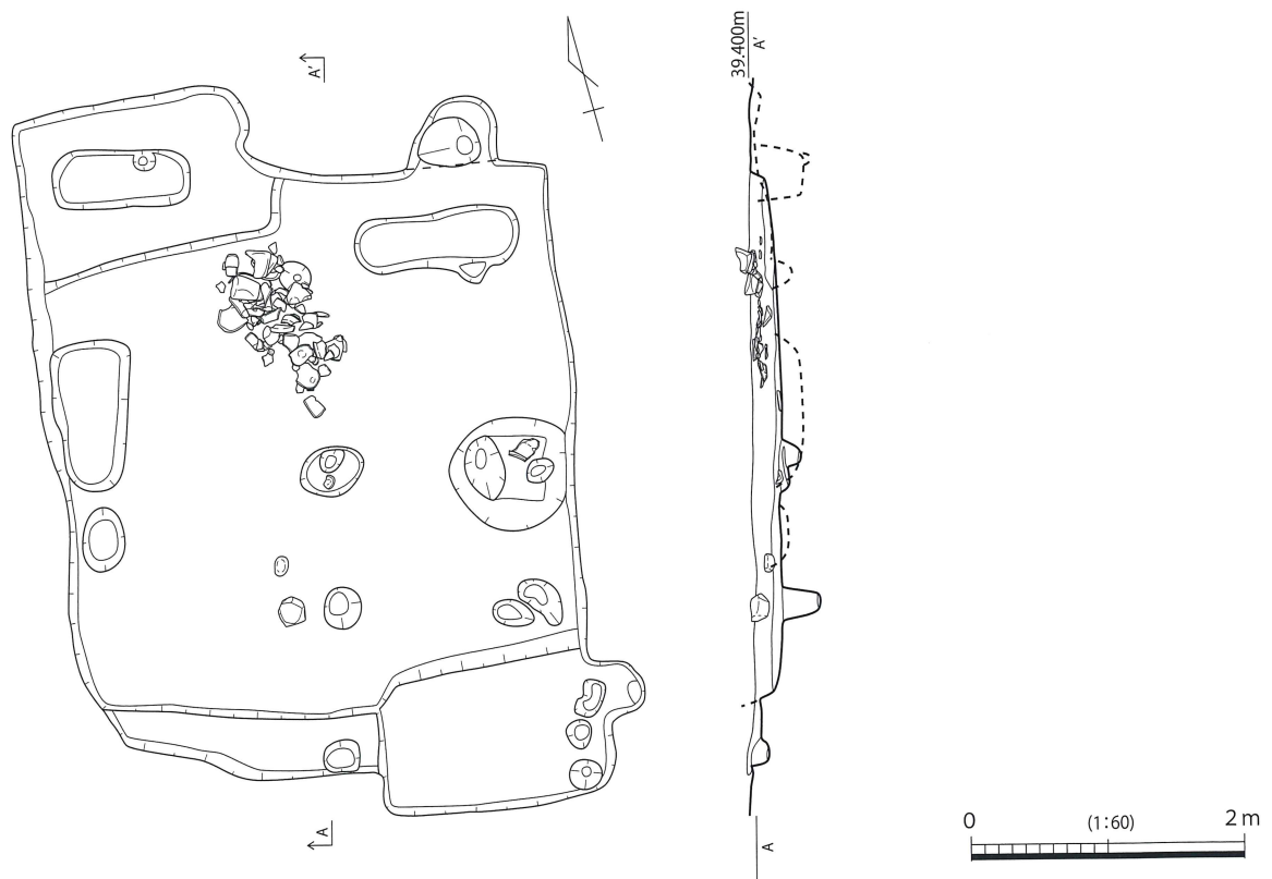
第 342 図 SH039 (下層) 実測図
