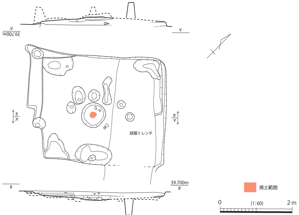
第346図 SH046 実測図
