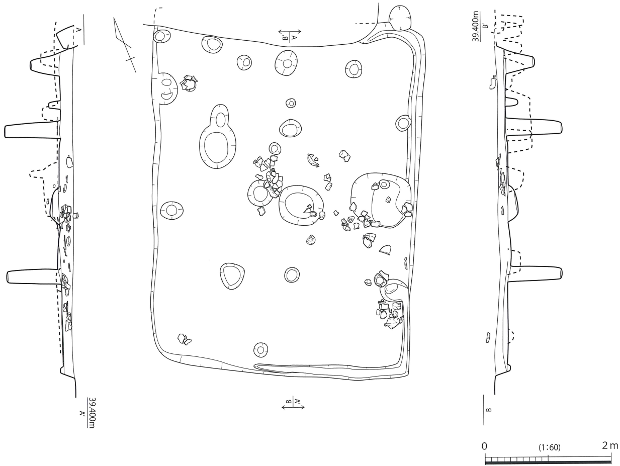
第 329 图 SH027 实测图
