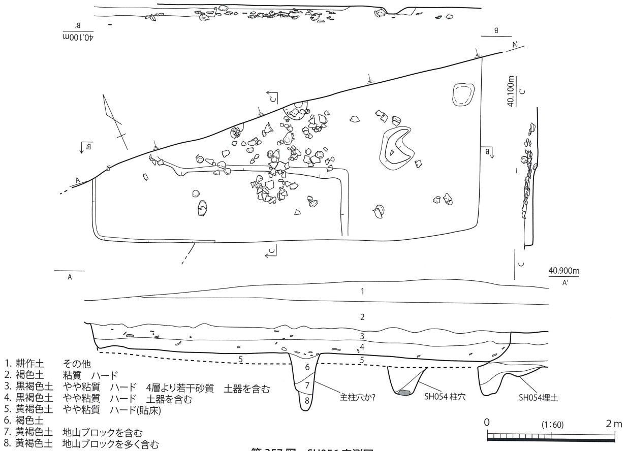
第 357 図 SH056 実測図
