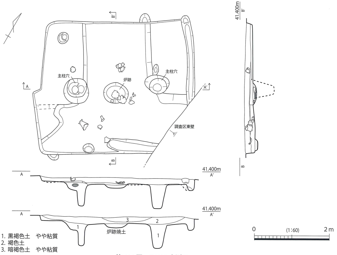
第414図 SH125 実測図
