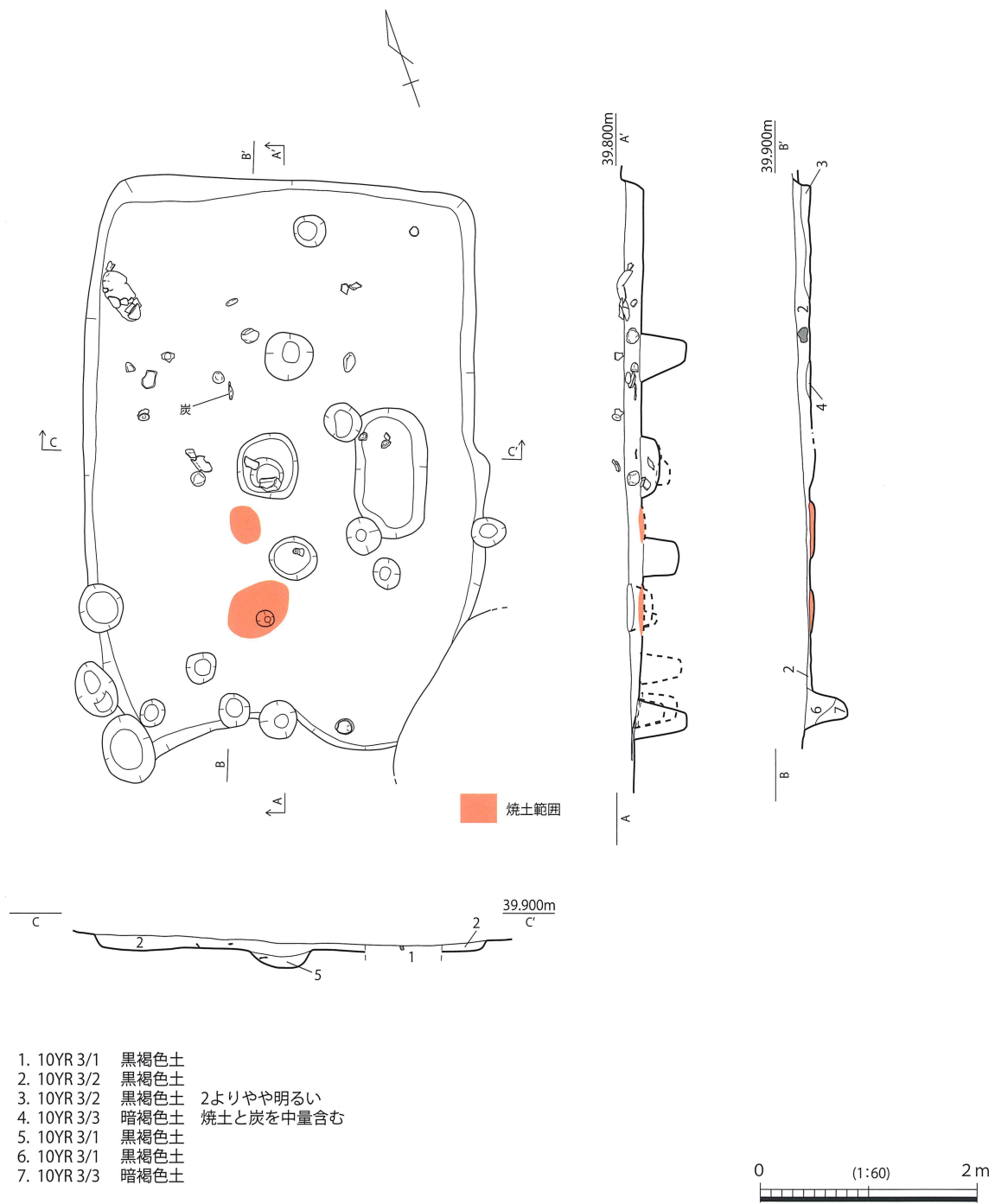
第 370 図 SH069 実測図
