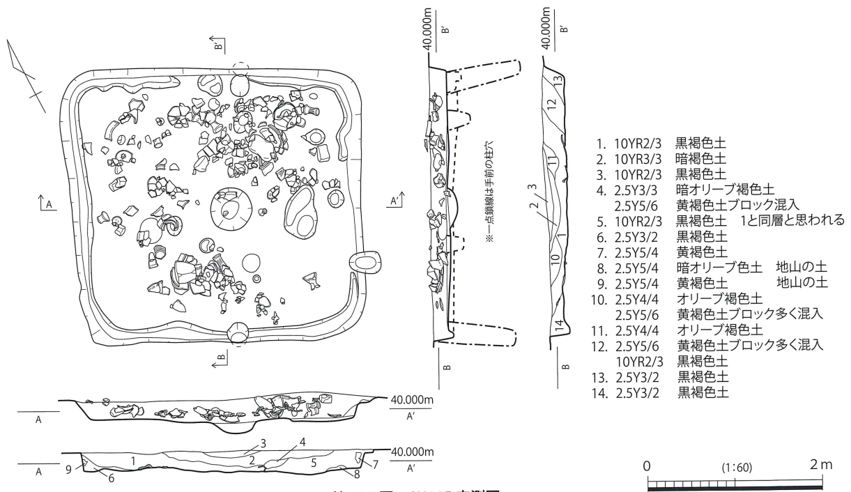
第407図 SH115 実測図
