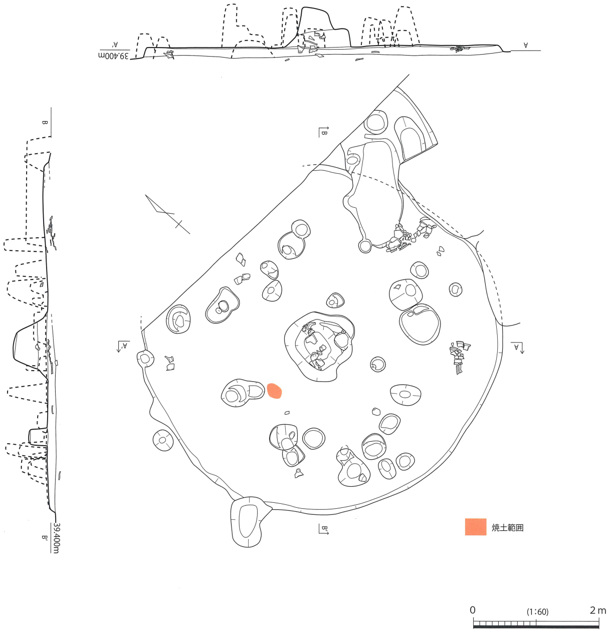
第 326 図 SH024 実測図
