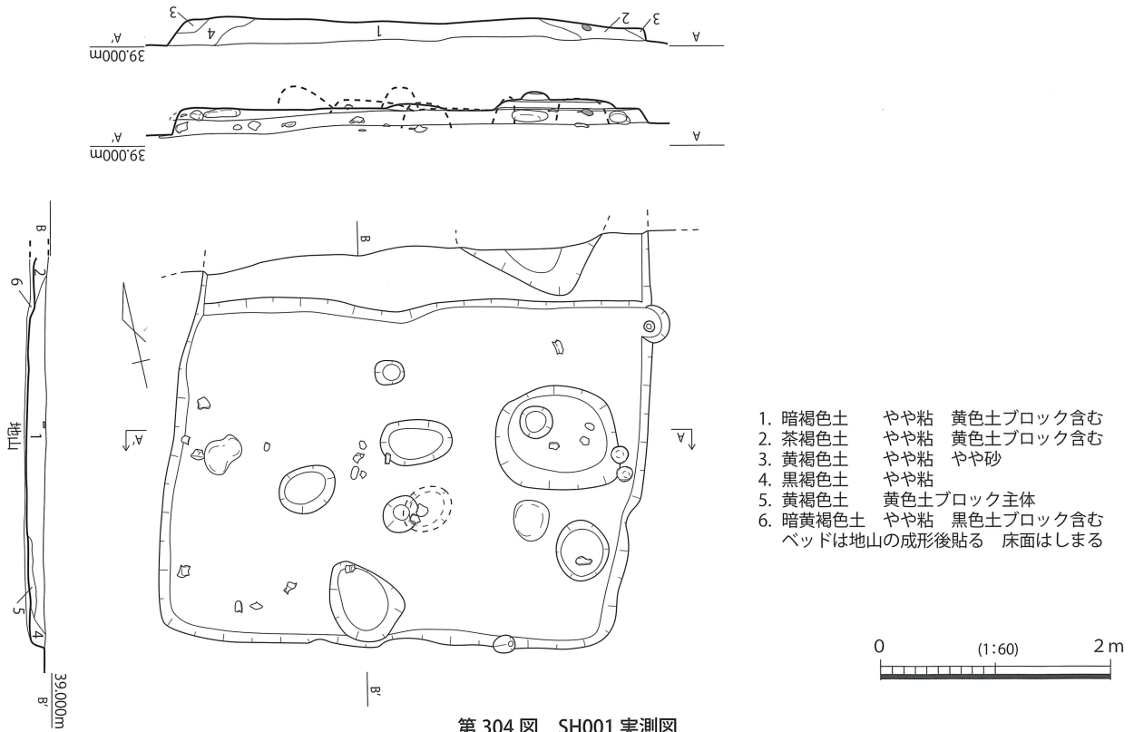
第 304 図 SH001 実測図
