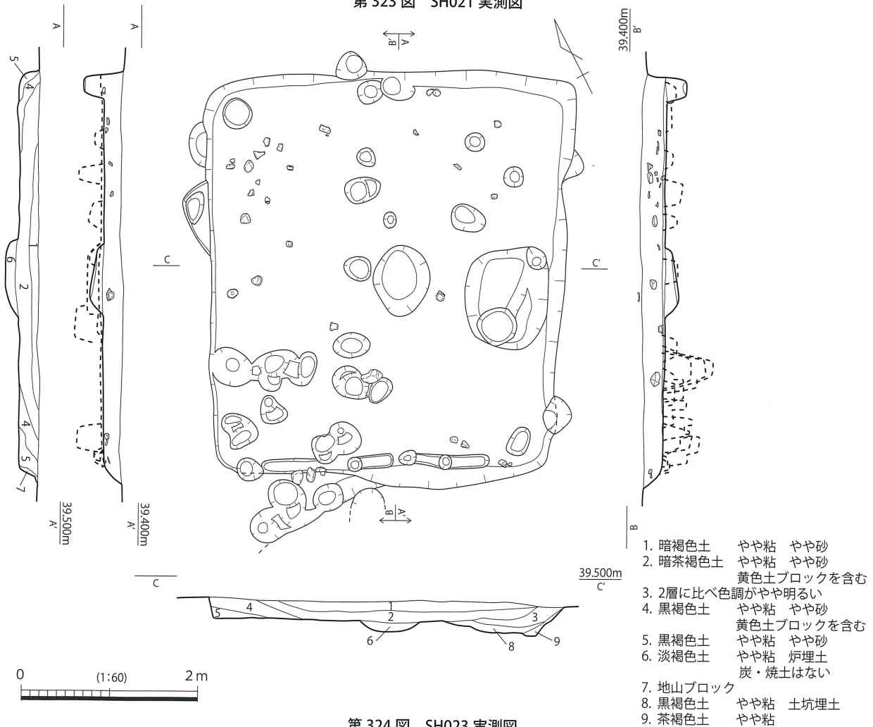
第324図 SH023 実測図
