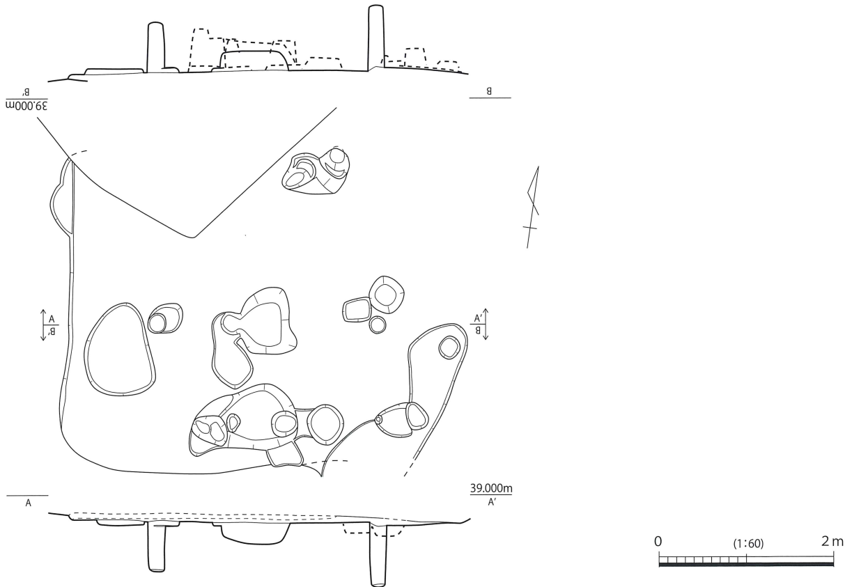
第 307 図 SH005 実測図
