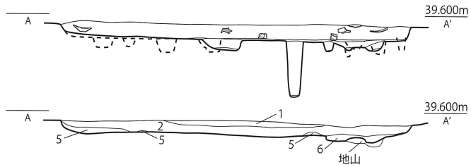
第331図 SH029 実測図
