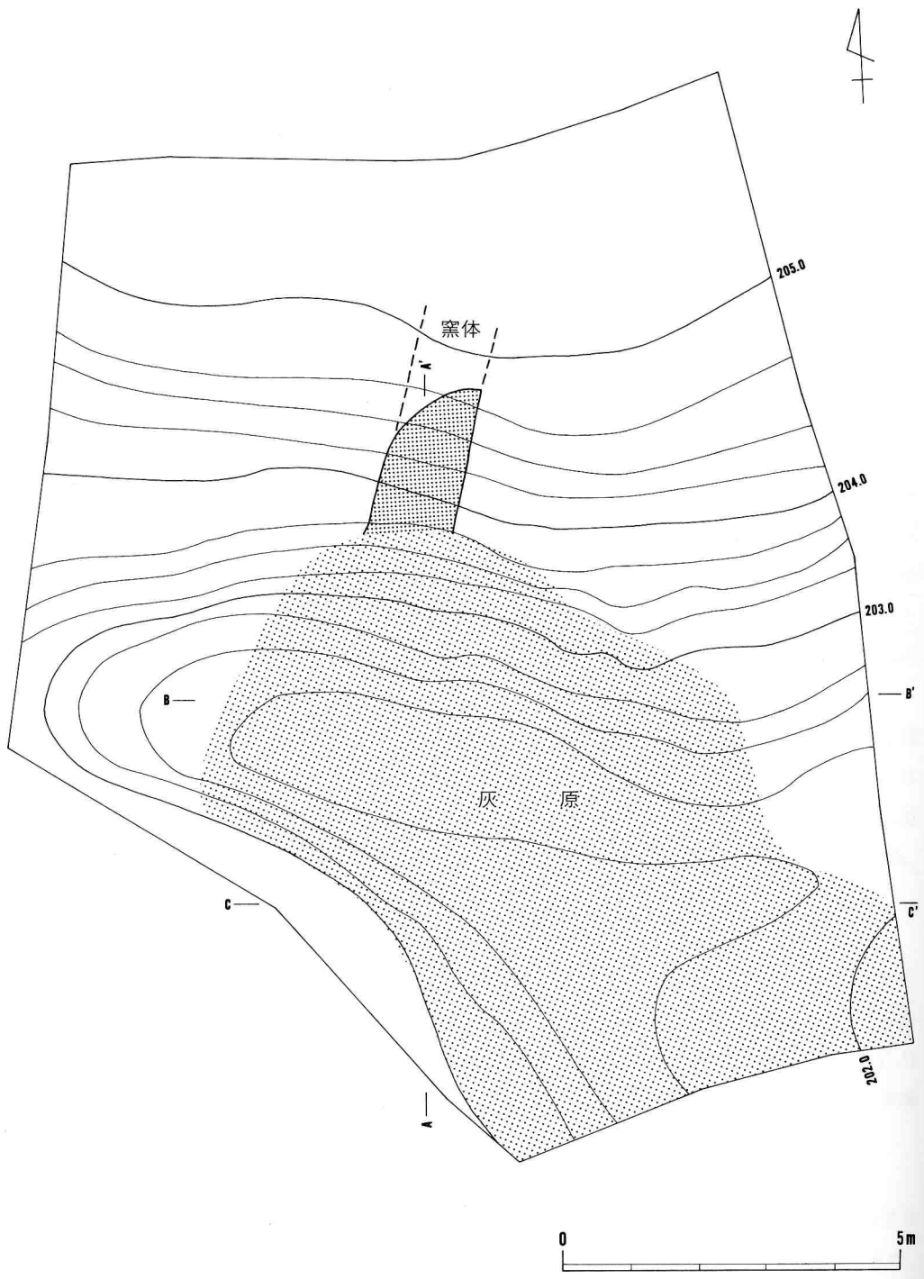
挿図100 古城5号窯跡 窯体と灰原遺構図
