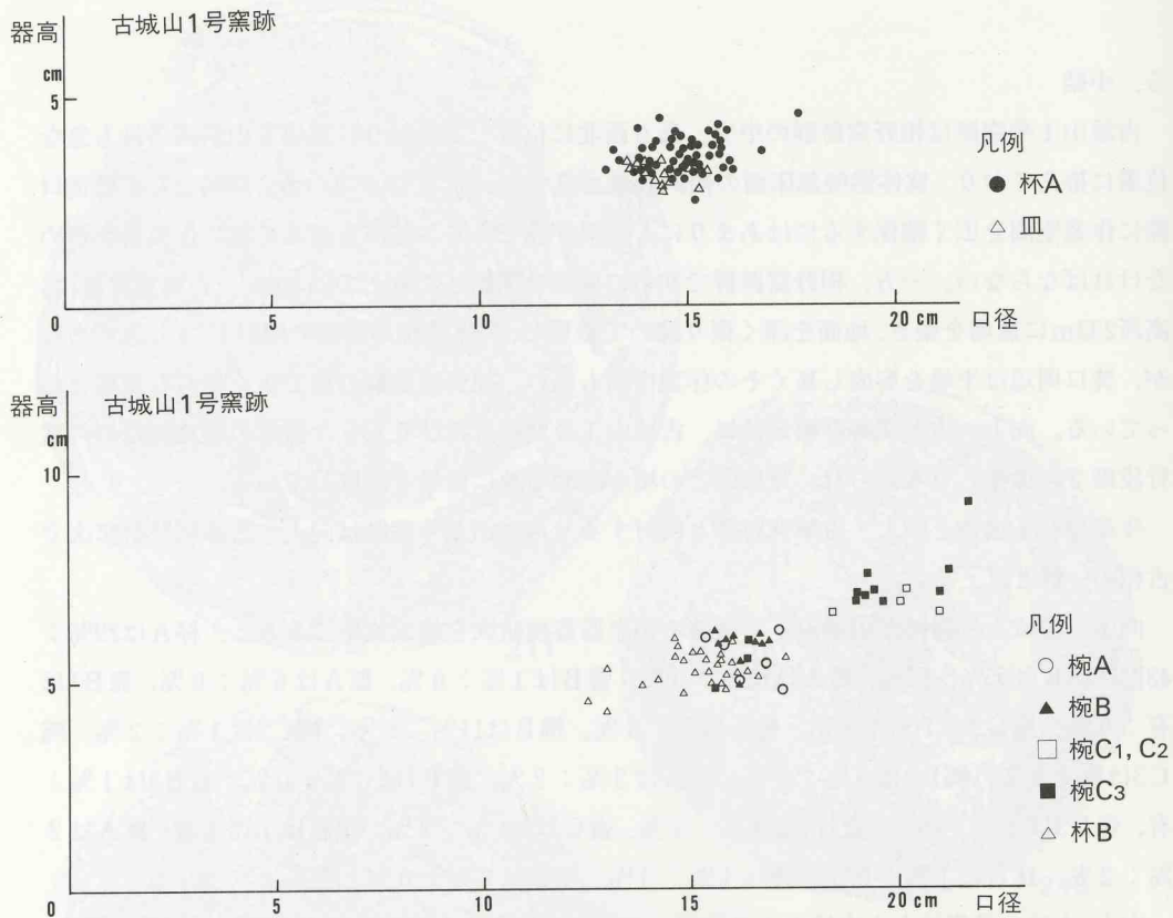
挿図61 古城山1号窯跡須恵器法量グラフ
