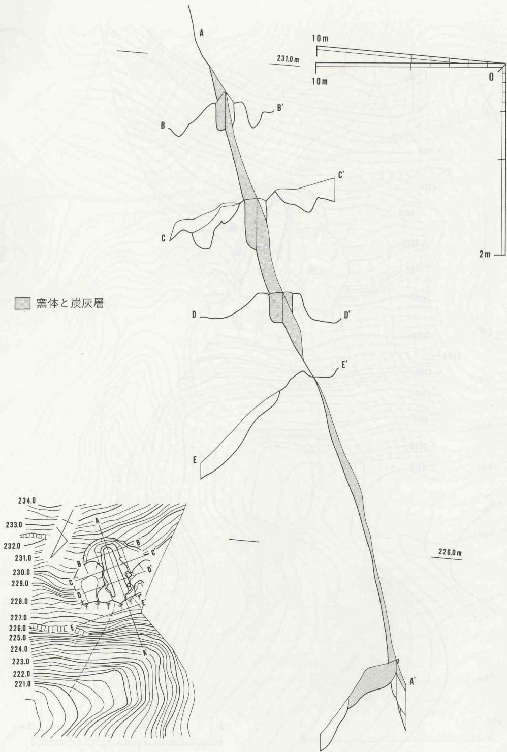
插图32 古城山1号窯跡 窯体・周溝・灰原土層堆積状況図
