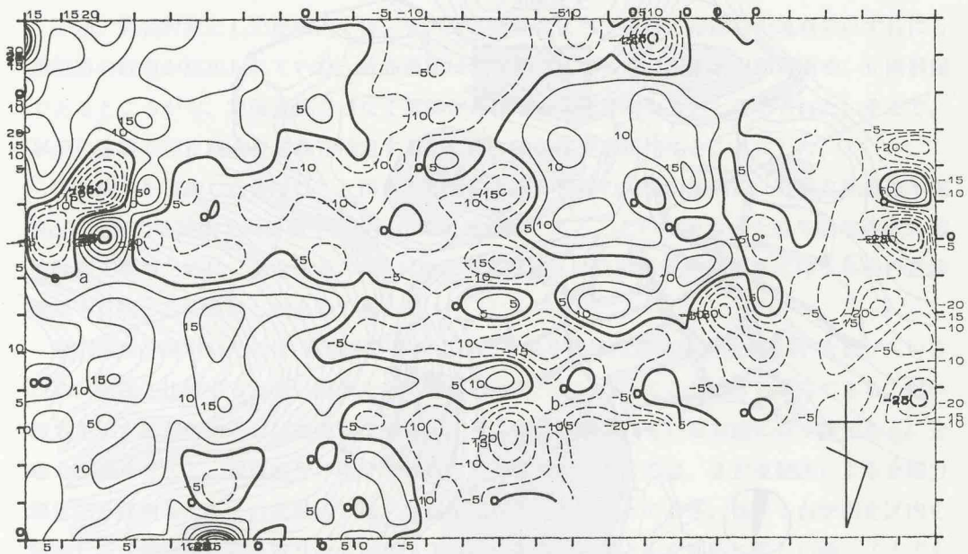
挿図14 大池地区地磁気探査データ
