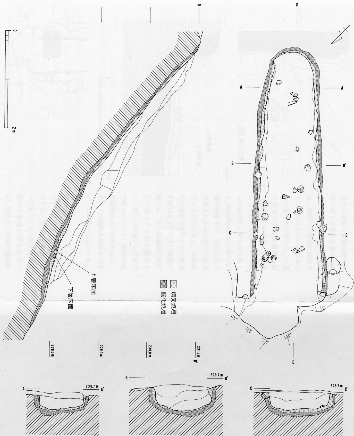
插图34 古城山1号寨迹 寨体图
