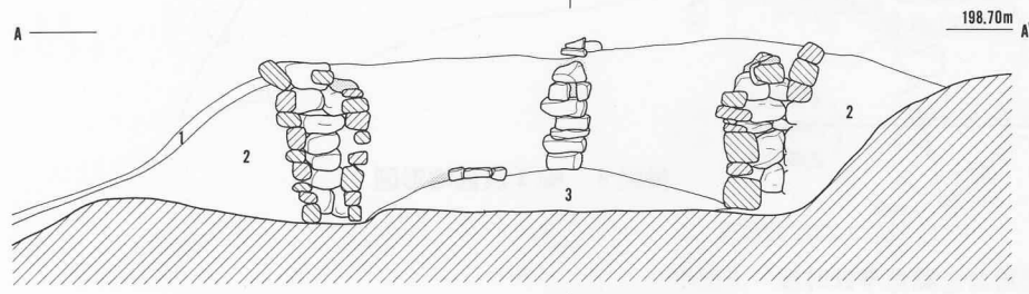
挿図10 No. 3 炭窯実測図
