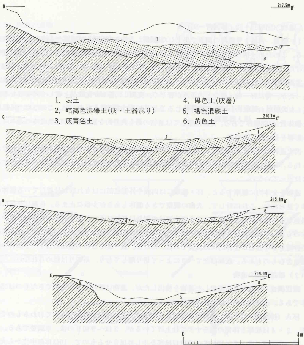
挿図66 古城1号窯跡 灰原土層堆積断面図
