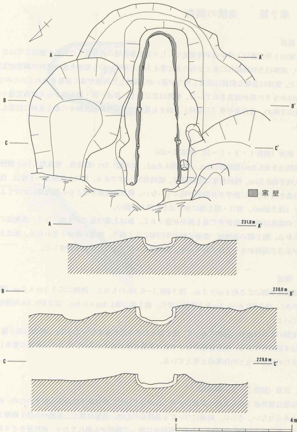
插图33 古城山1号窠迹 窠体·周溝遺構図
