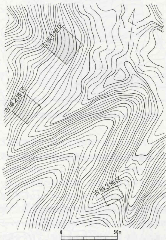
挿図19 古城1・2・3地区地磁気探査位置図
