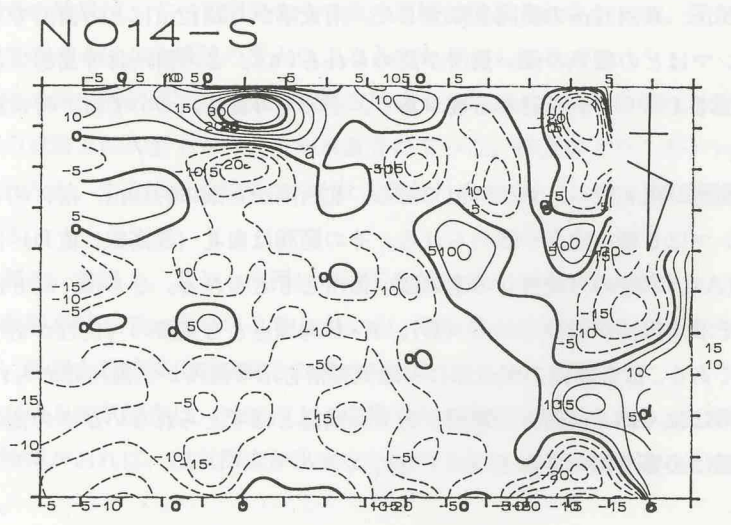
插图17 No.14地点S地区地磁気探查データ
