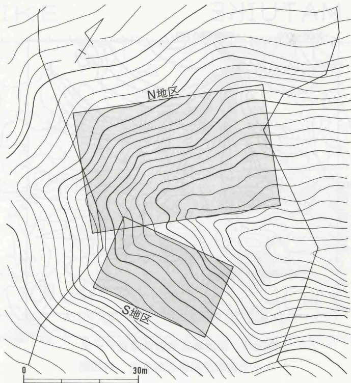
插图16 No.14地点地区地磁気探查位置図
