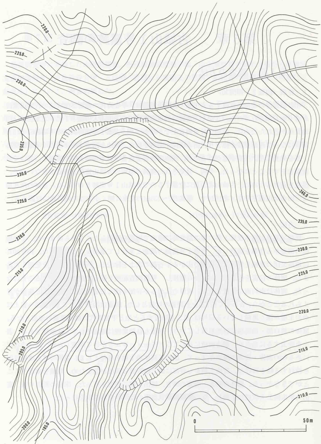
插图30 古城山1号寨迹位置图
