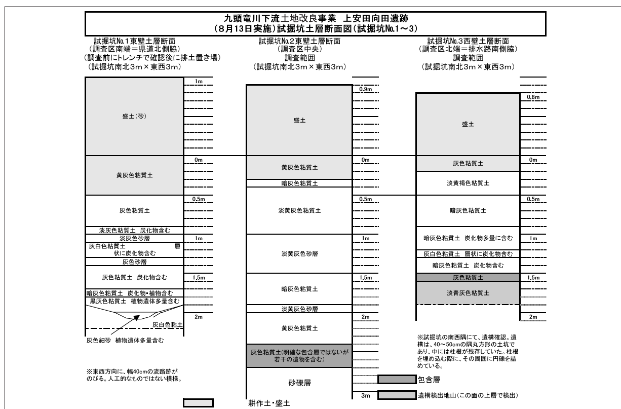
第3図 上安田向田遺跡試掘調査での土層柱状模式図
