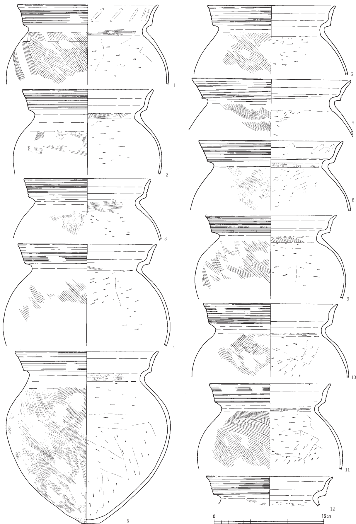
第13図 弥生土器（甕）実測図（縮尺1/3）
