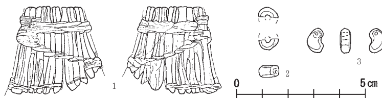
第23図 装飾品実測図（縮尺2/3）
