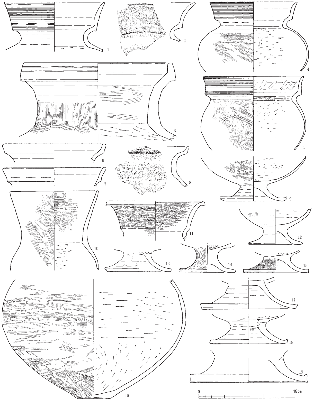
第17図 弥生土器（壺）実測図（縮尺1/3）
