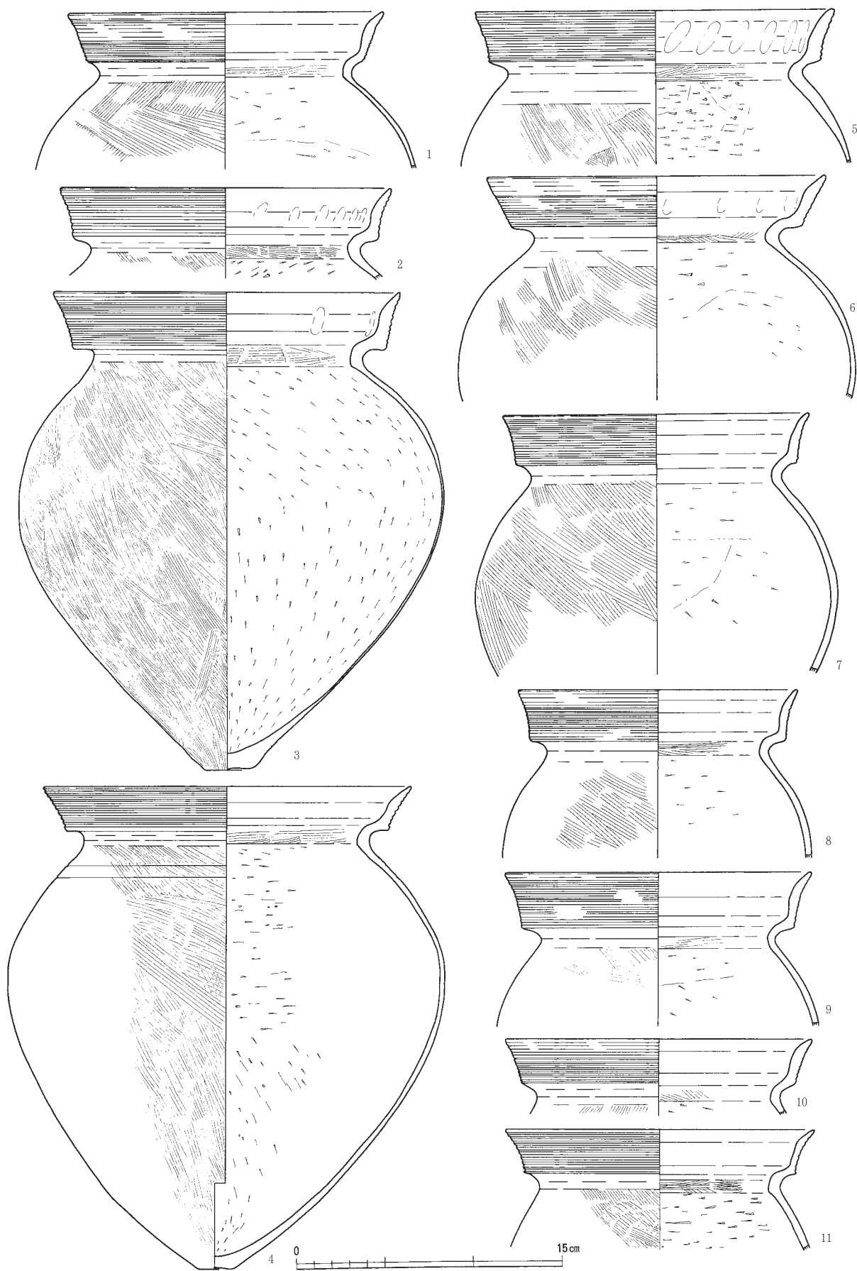
第12図 弥生土器（甕）実測図（縮尺1/3）
