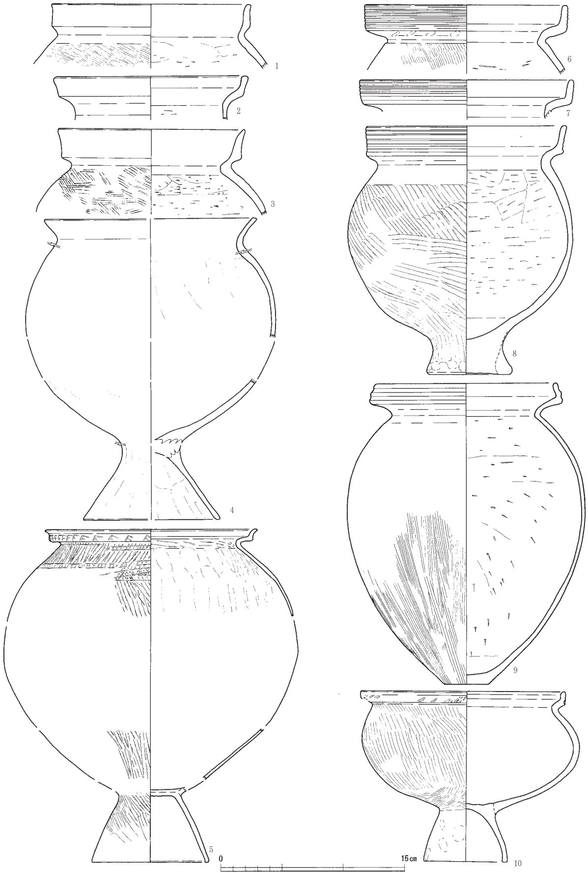
第15图 弥生土器（甕）实测图（缩尺1/3）
