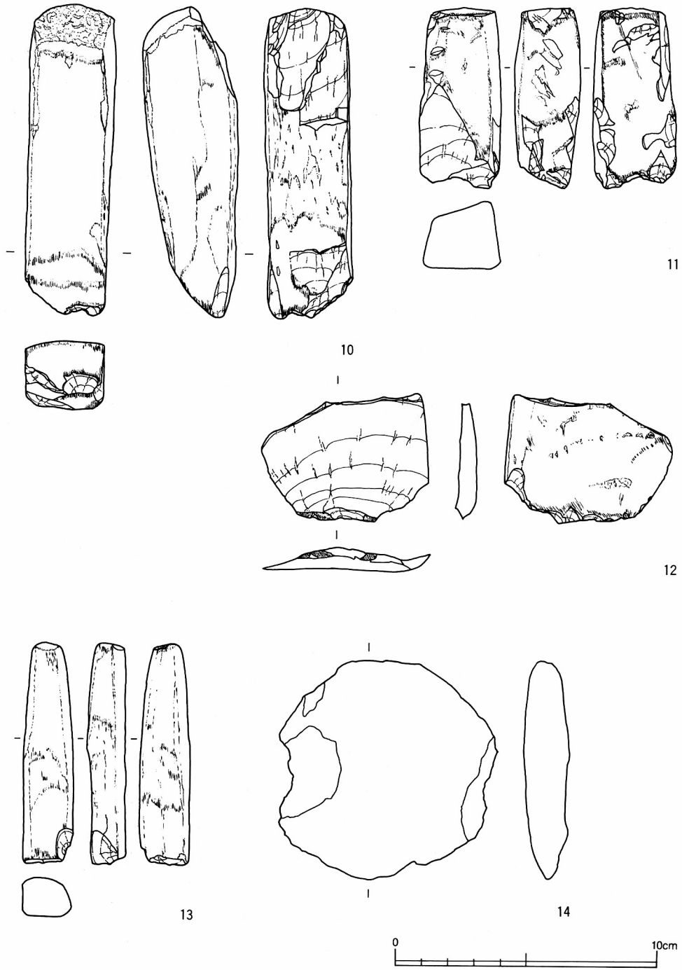
第51図 石器実測図(3)
