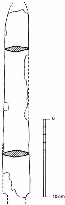
第56図 溝状遺構出土 鉄剣実測図
