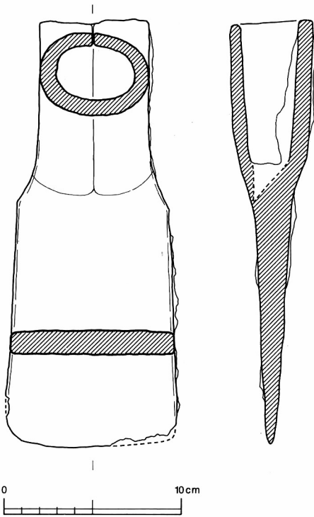
第55図 溝状遺構出土 鉄斧実測図
