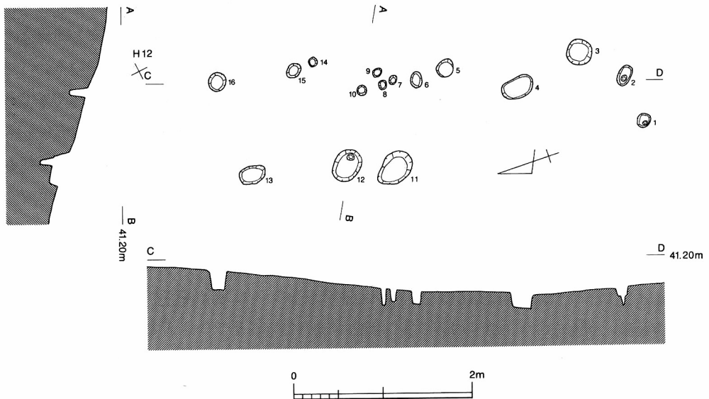
第37図 柵状遺構2実測図
