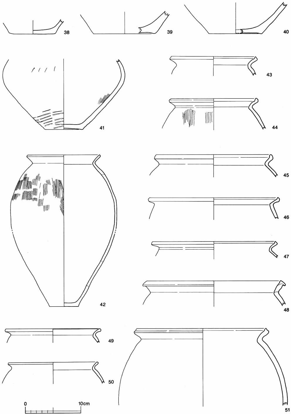
第43图 弥生土器实测图(4)
