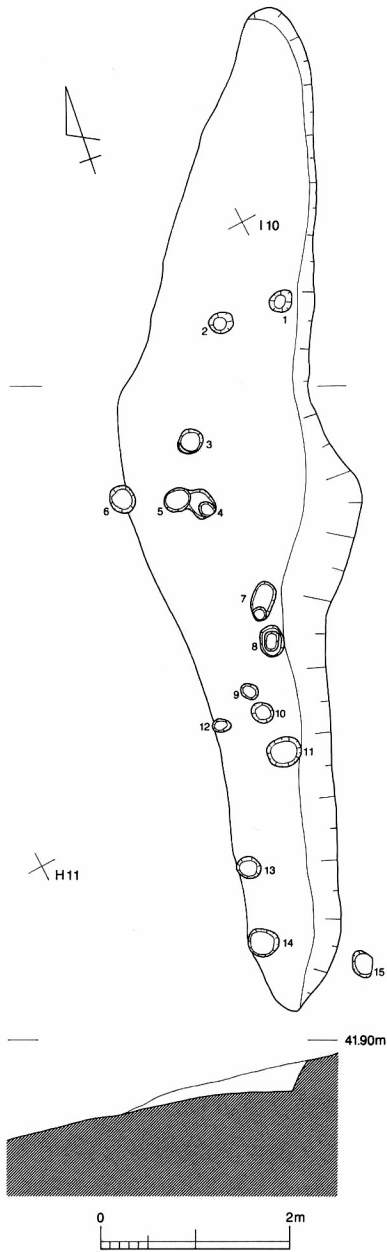
第36図 柵状遺構1実測図
