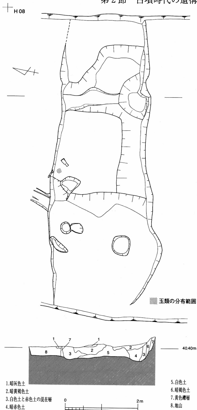
第53図 溝状遺構実測図
