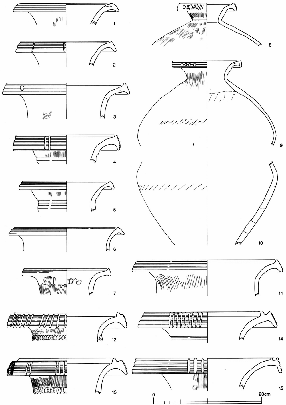
第39图 弥生土器实测图(1)
