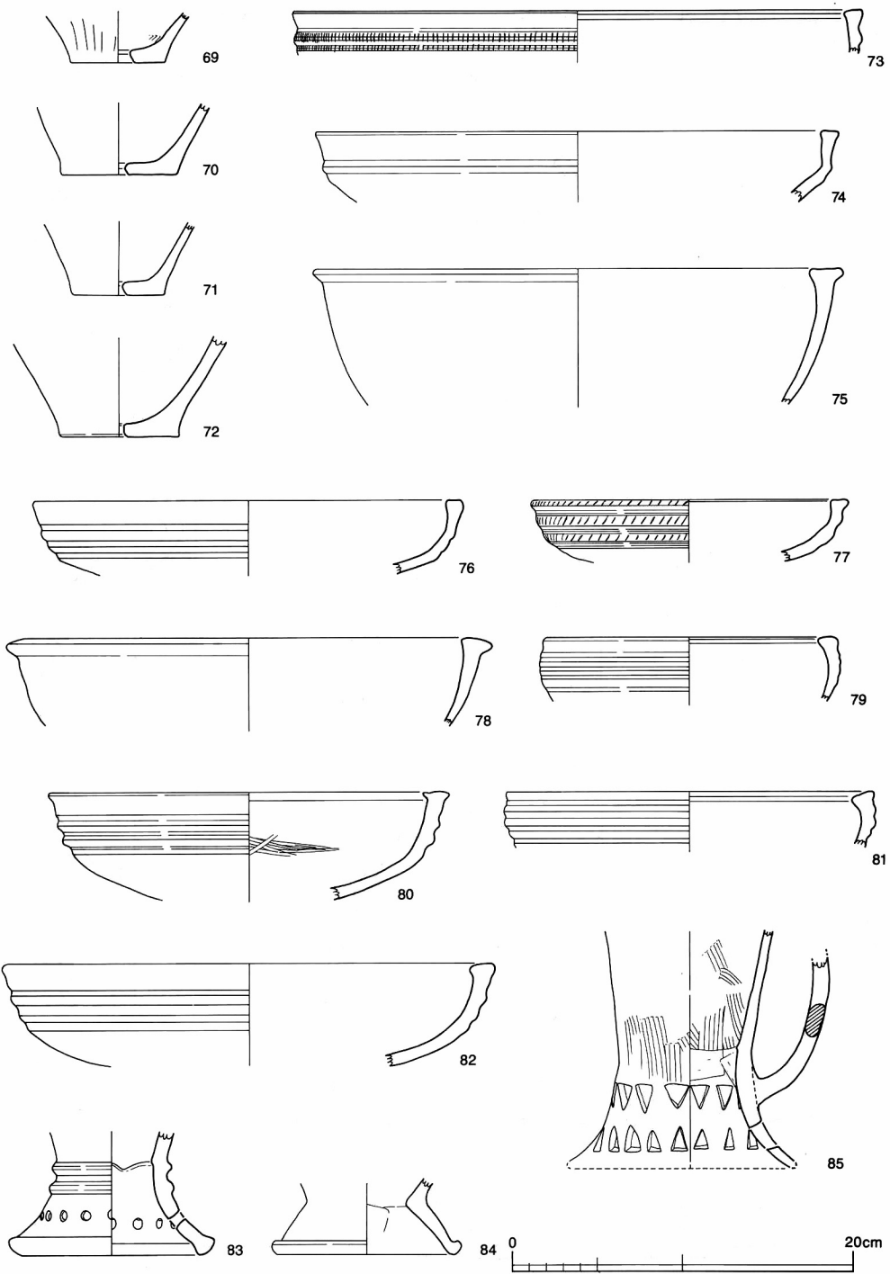
第45图 弥生土器实测图(6)
