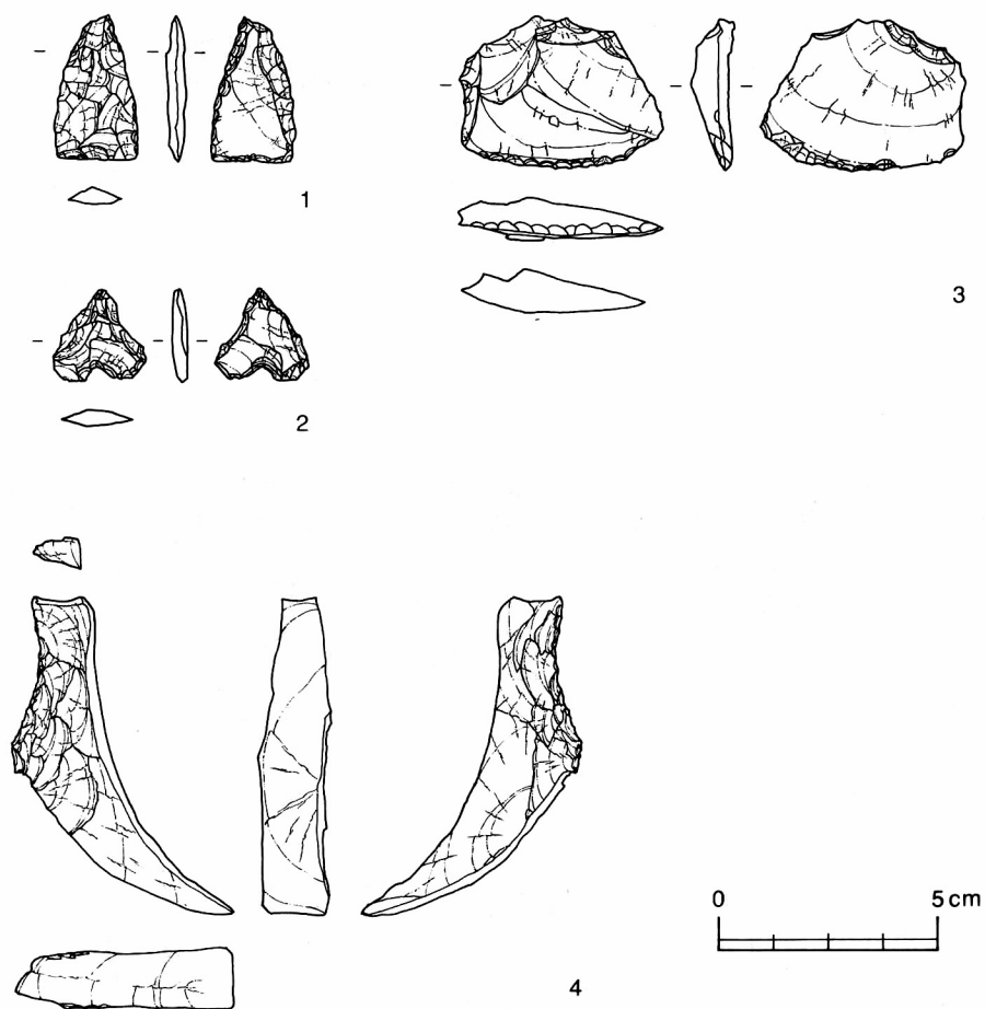
第49図 石器実測図(1)
