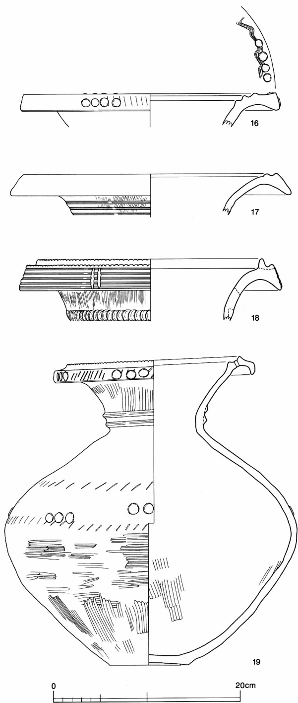
第40図 弥生土器実測図(2)
