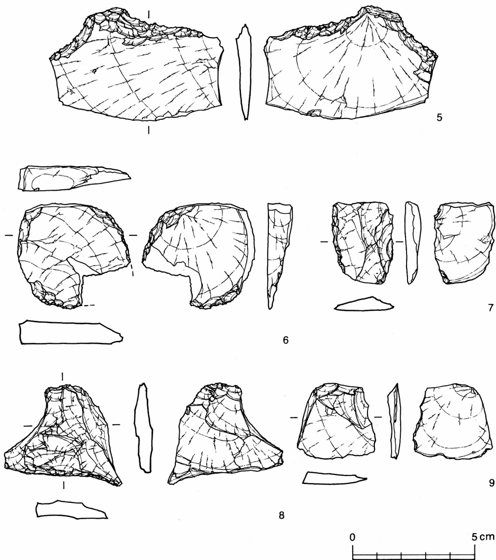
第50図 石器実測図(2)
