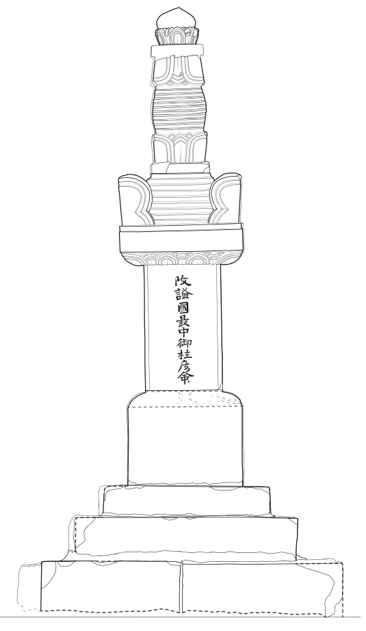
背面図
