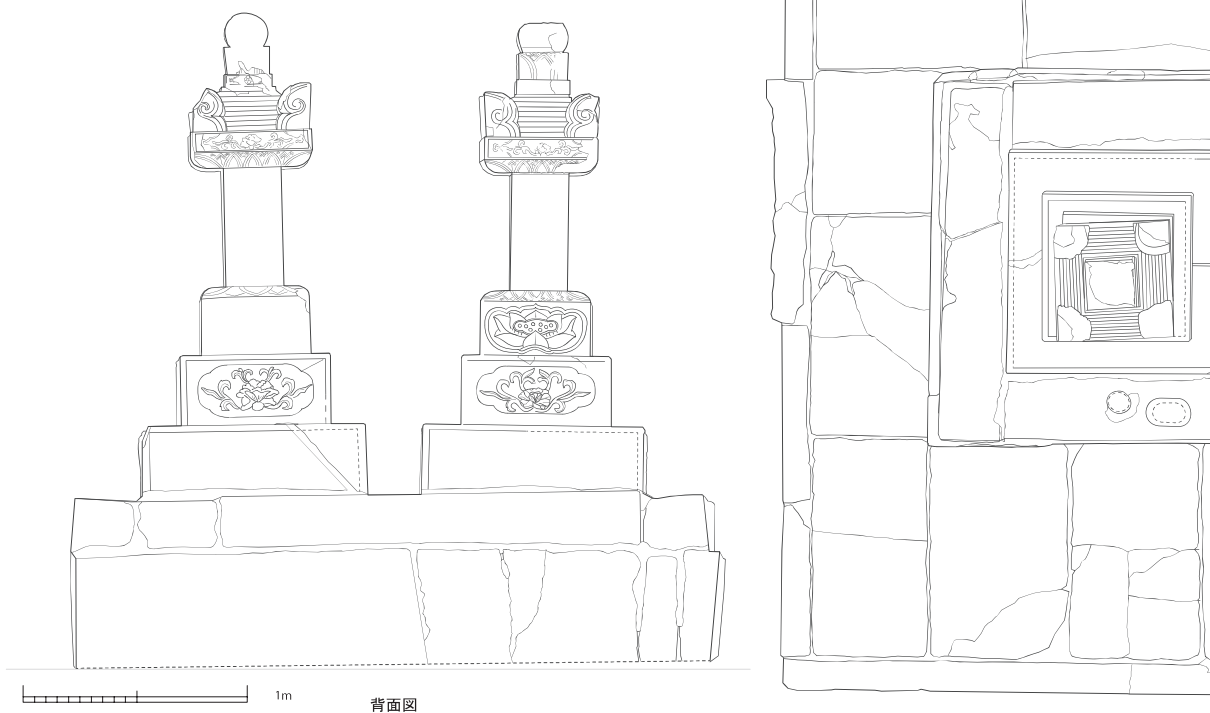
背面圖
