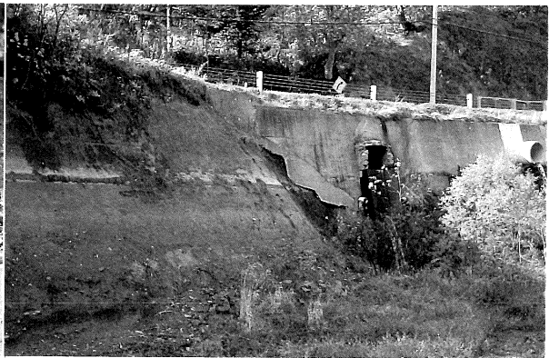
図86 宮島付近の瀨棚層
