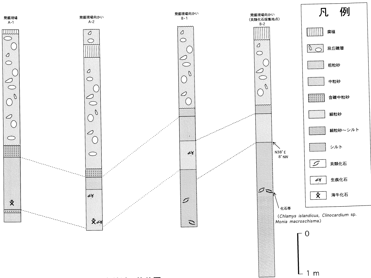
図87 カイギユウ化石産出地点付近の柱状図
