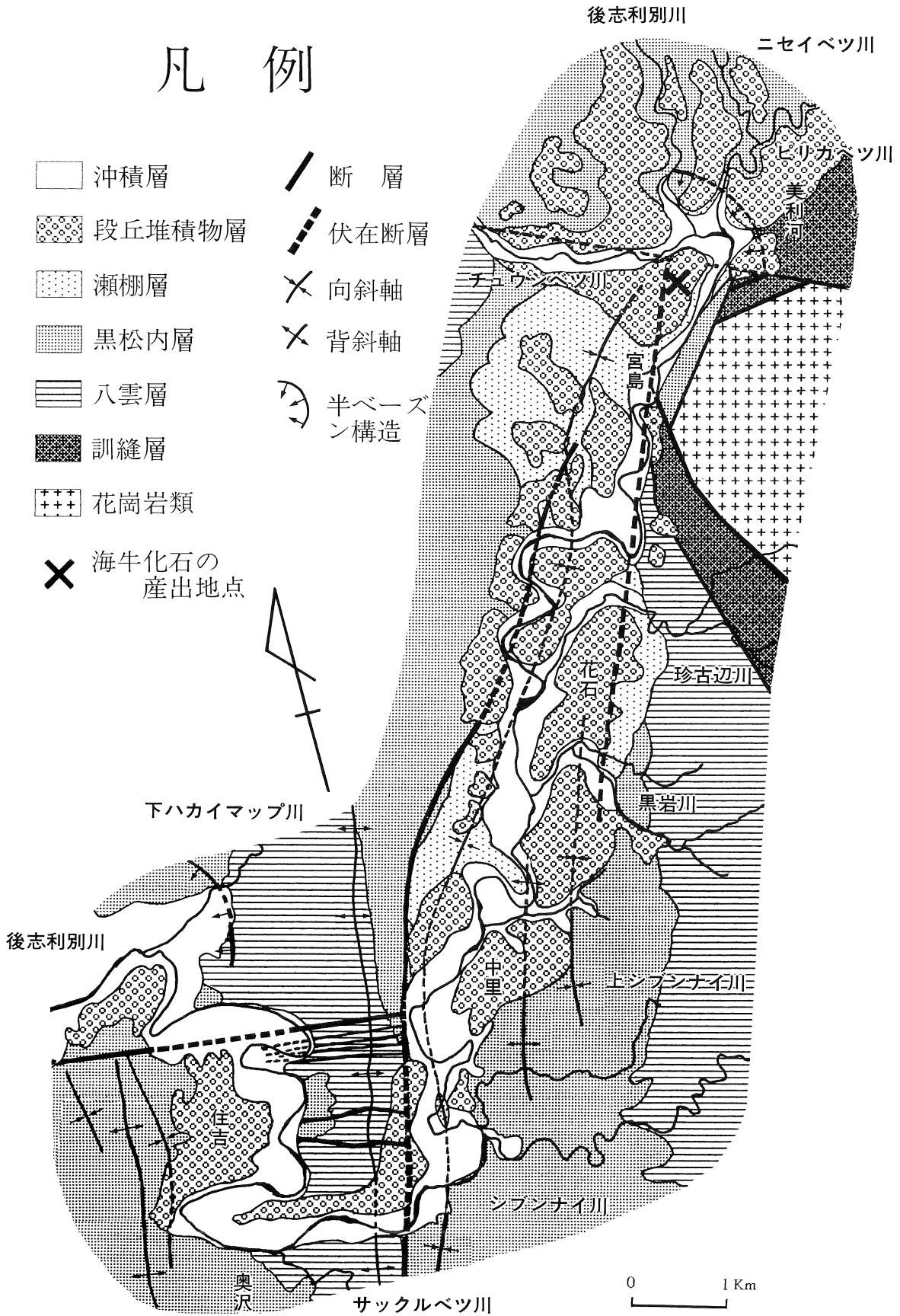
図67 美利河地域の地質図
