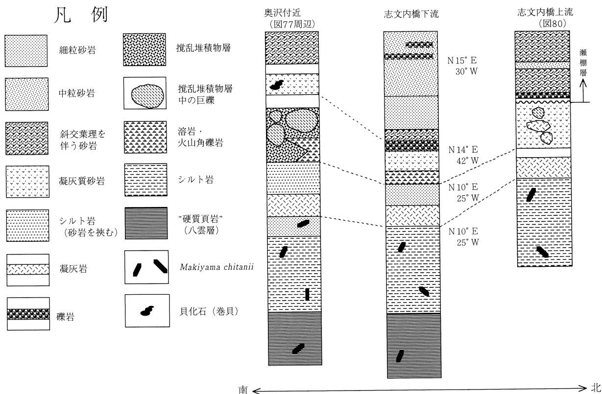
図81 奥沢～志文内間の柱状図
