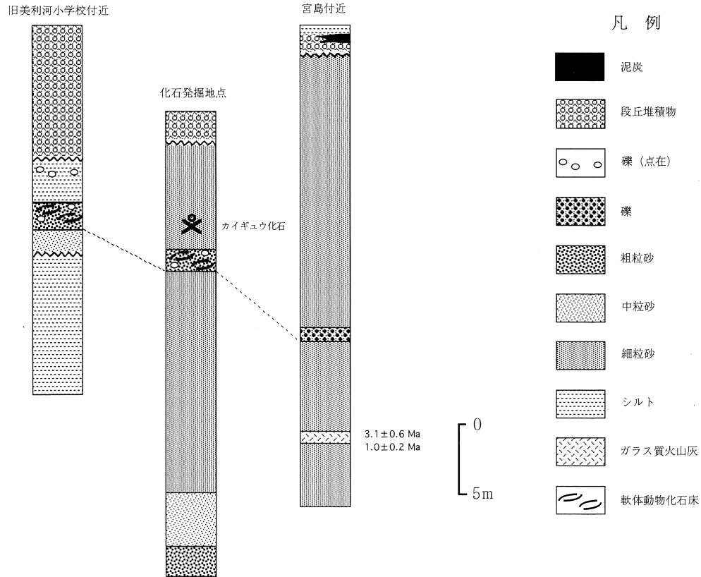
図89 美利河付近の柱状図
