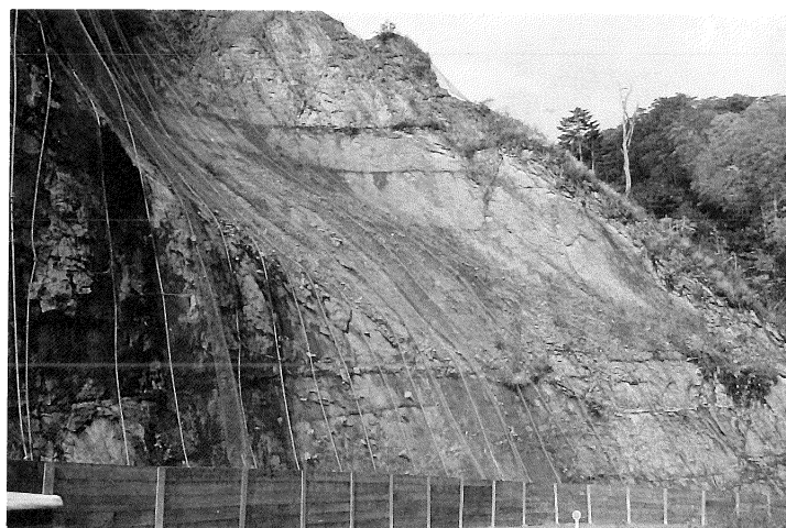
図70 訓縫層下部の砂岩・泥岩層 (熊すべりの盤)
