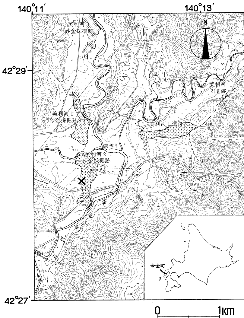
図66 化石産出地点（×印）
