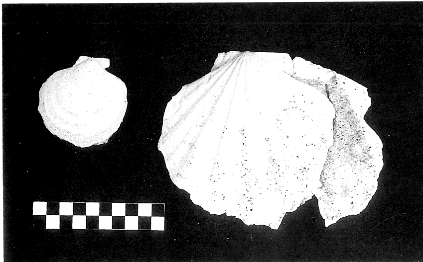
図74 八雲層産出の化石 左; Placopecten setanaensis (セタナツキヒ) 右; Kotorapecten kagamianus (カガミホタテ)
