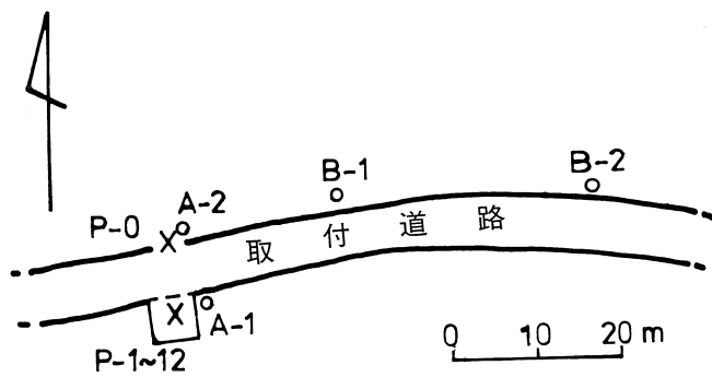
図88 化石産出地点付近の柱状位置図 A-1~2, B-1~2 : 図87の柱状図番号 P-0, P-1~12 : 発掘ブロックの番号
