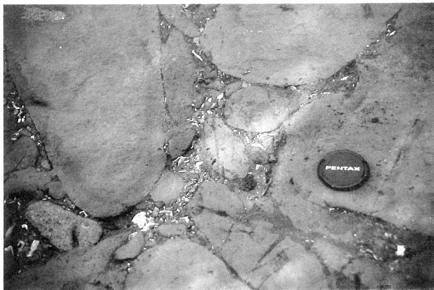
図84 美利河の不整合に見られる巨大ブロック状の基底礫 （ピリカベツ川-後志利別川合流点, 既に水没）
