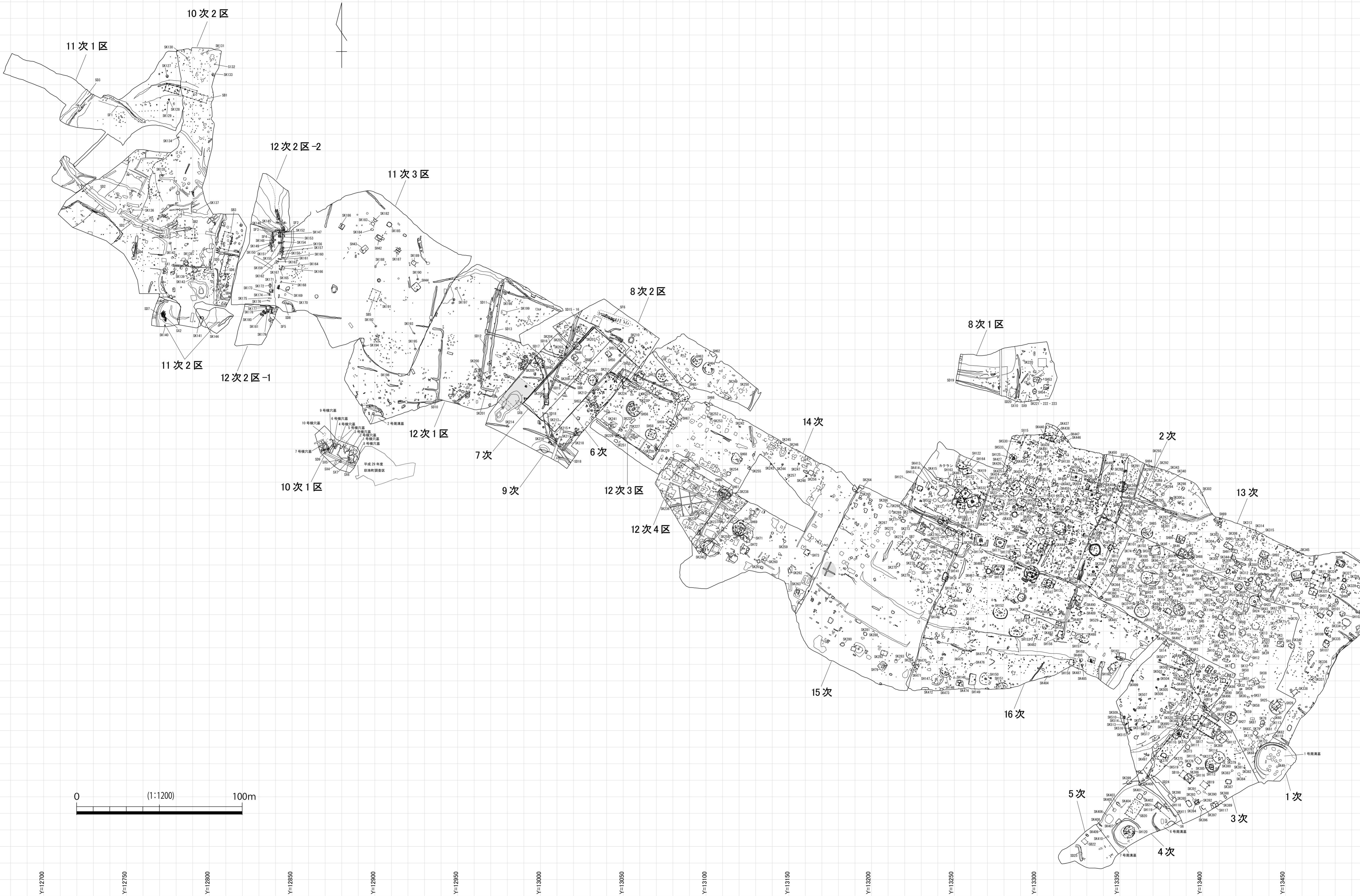
付図 四日市遺跡遺構配置図 (1/1200)
