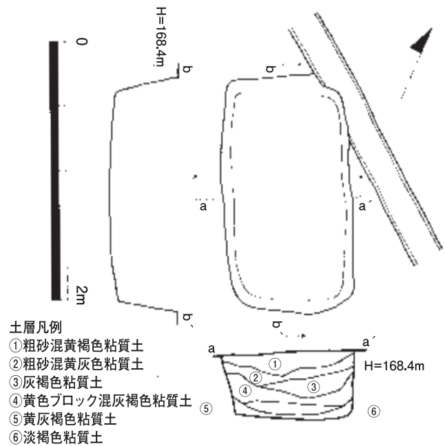
図17 土壇墓 SK0226 1:40
