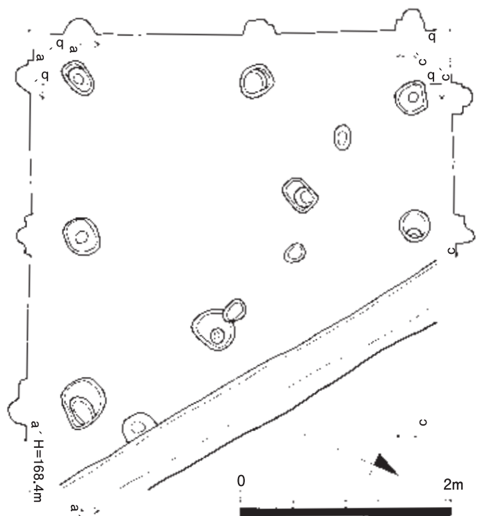
図18 掘立柱建物 SB0232 1:50
