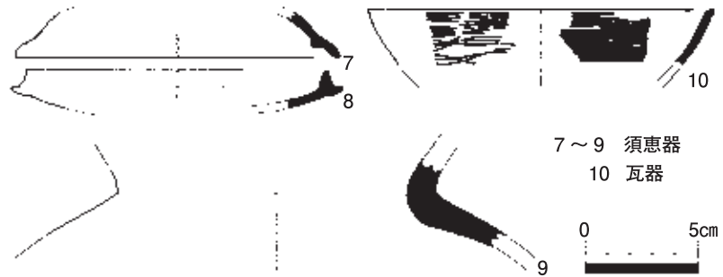
図 21 土墳墓 SK0226 出土土器 1 : 3
