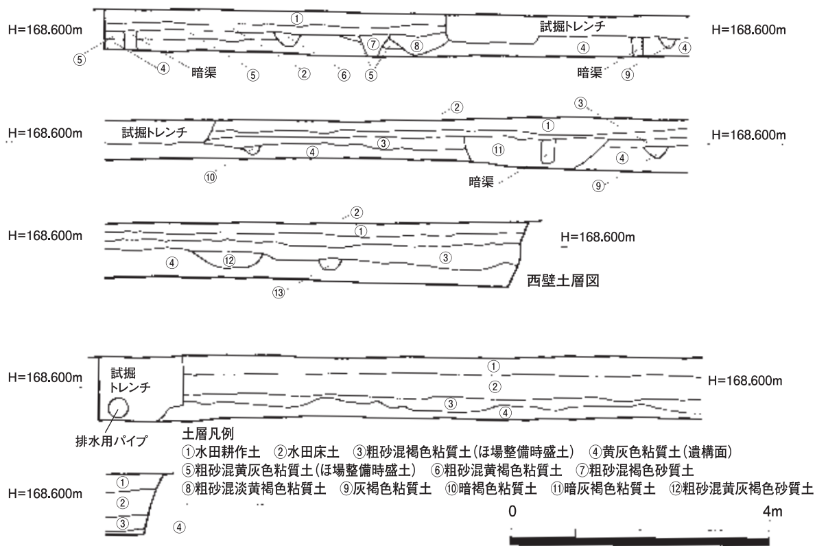
図 13 第2トレンチ土層断面図 1：80
