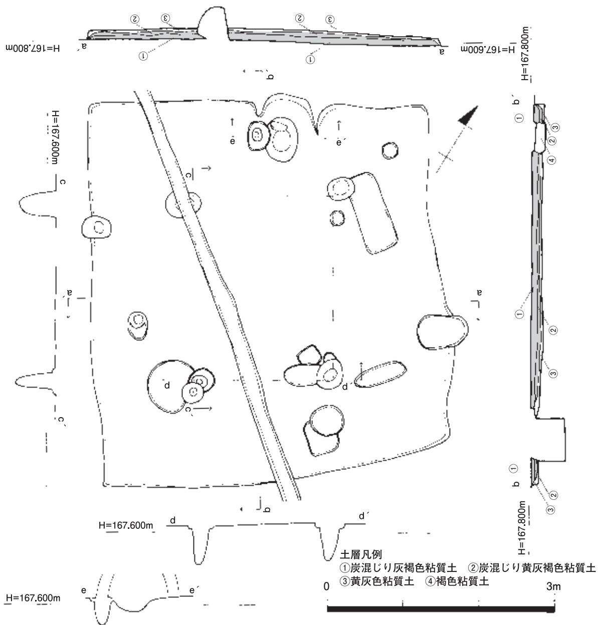
図 15 竪穴住居 SB0102 1 : 50
