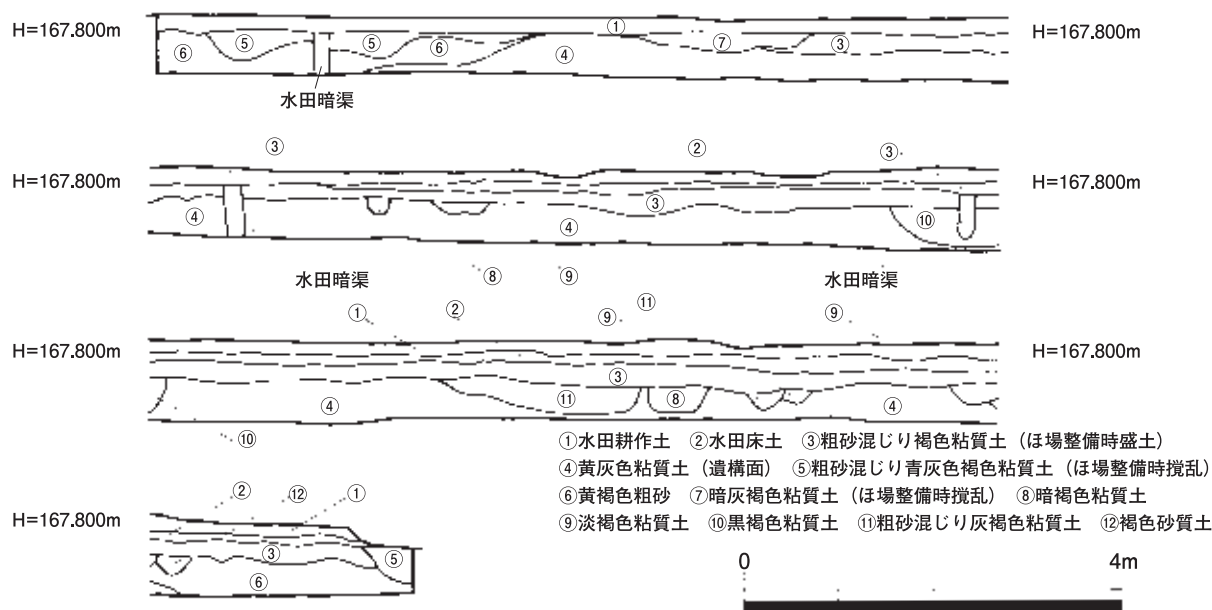
図12 第1トレンチ土層断面図 1:80
