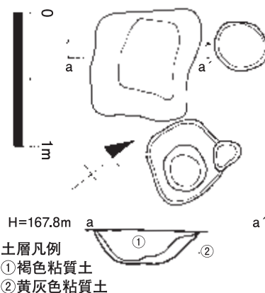
図16 土坑 SK0116 1:40
