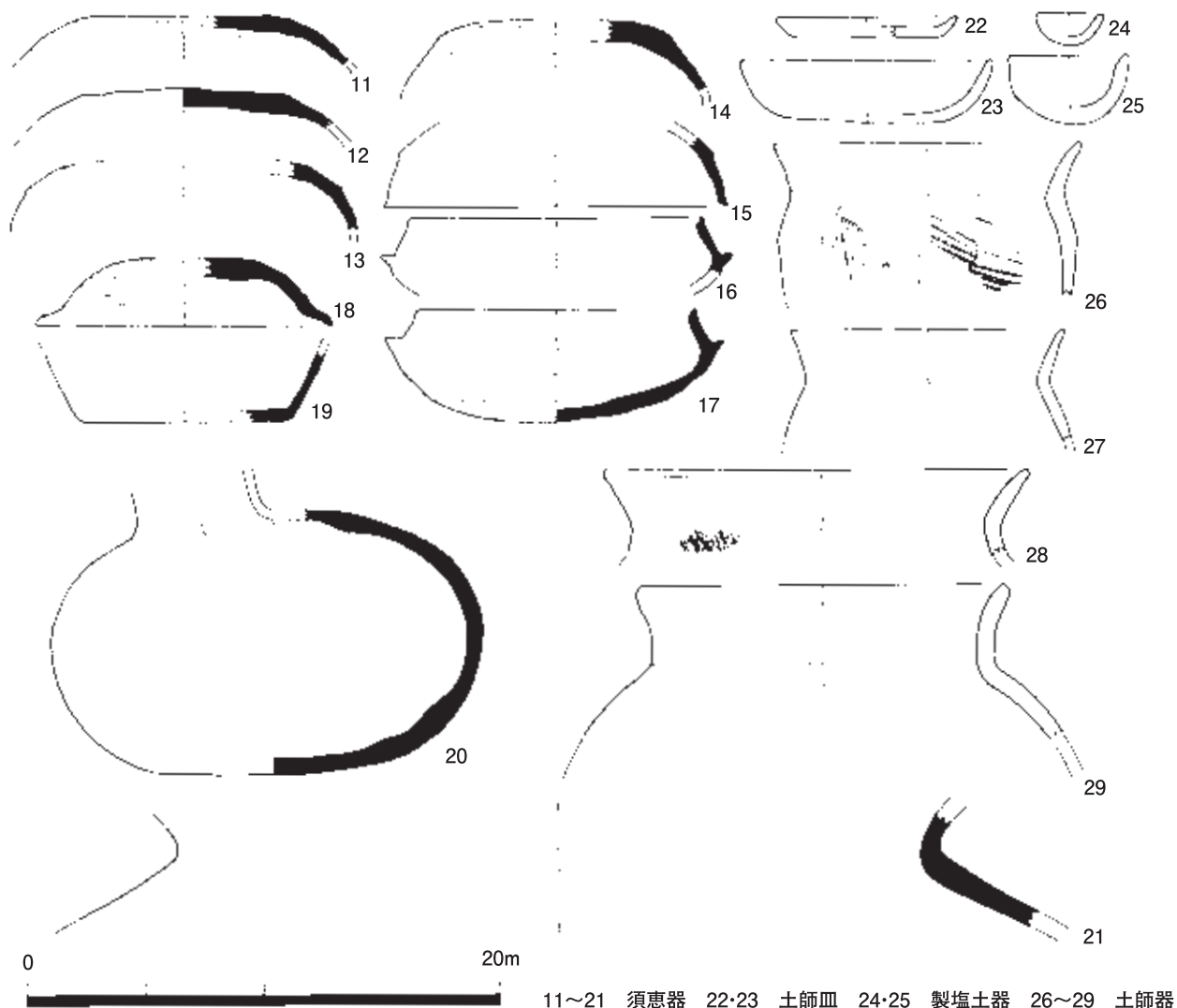
図 22 その他の出土土器 1 : 3
