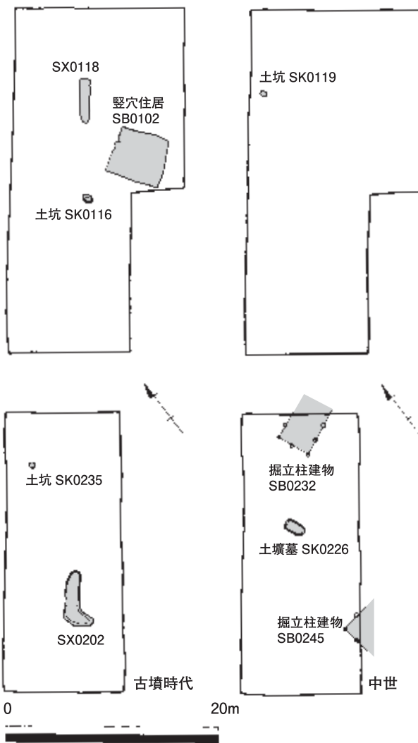
図23 時期区分による遺構配置 1:500
