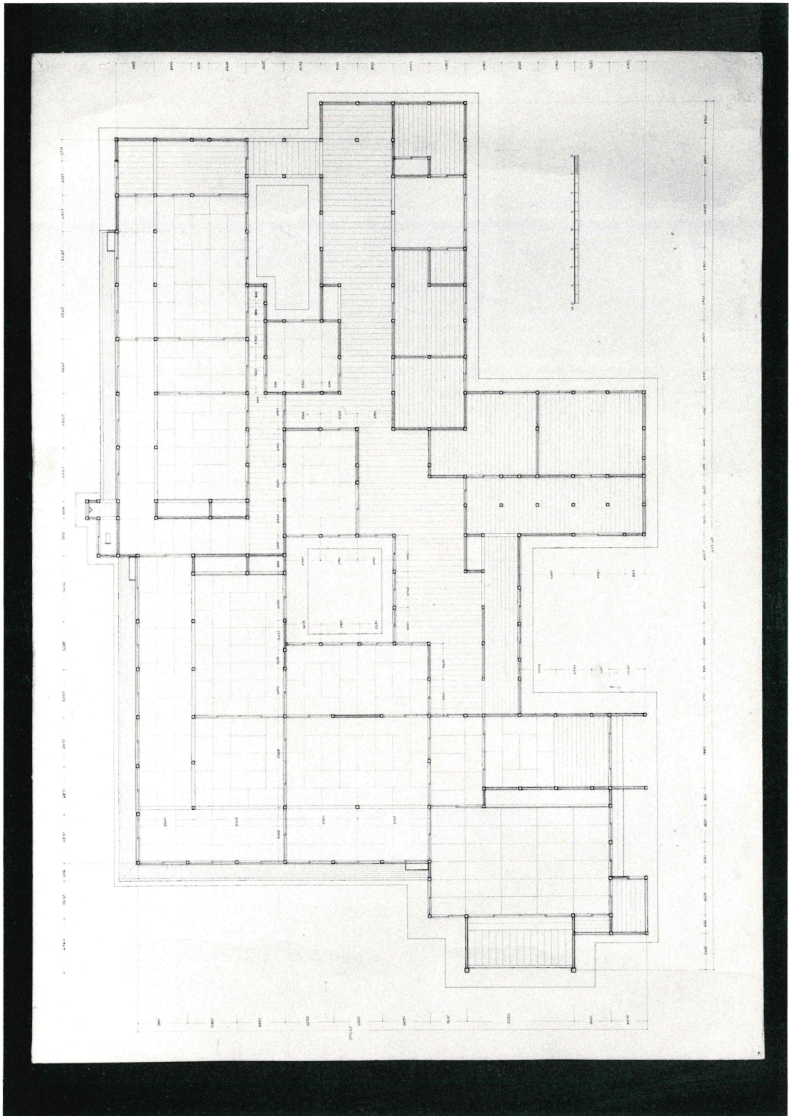
掛川城御殿竣工平面図
