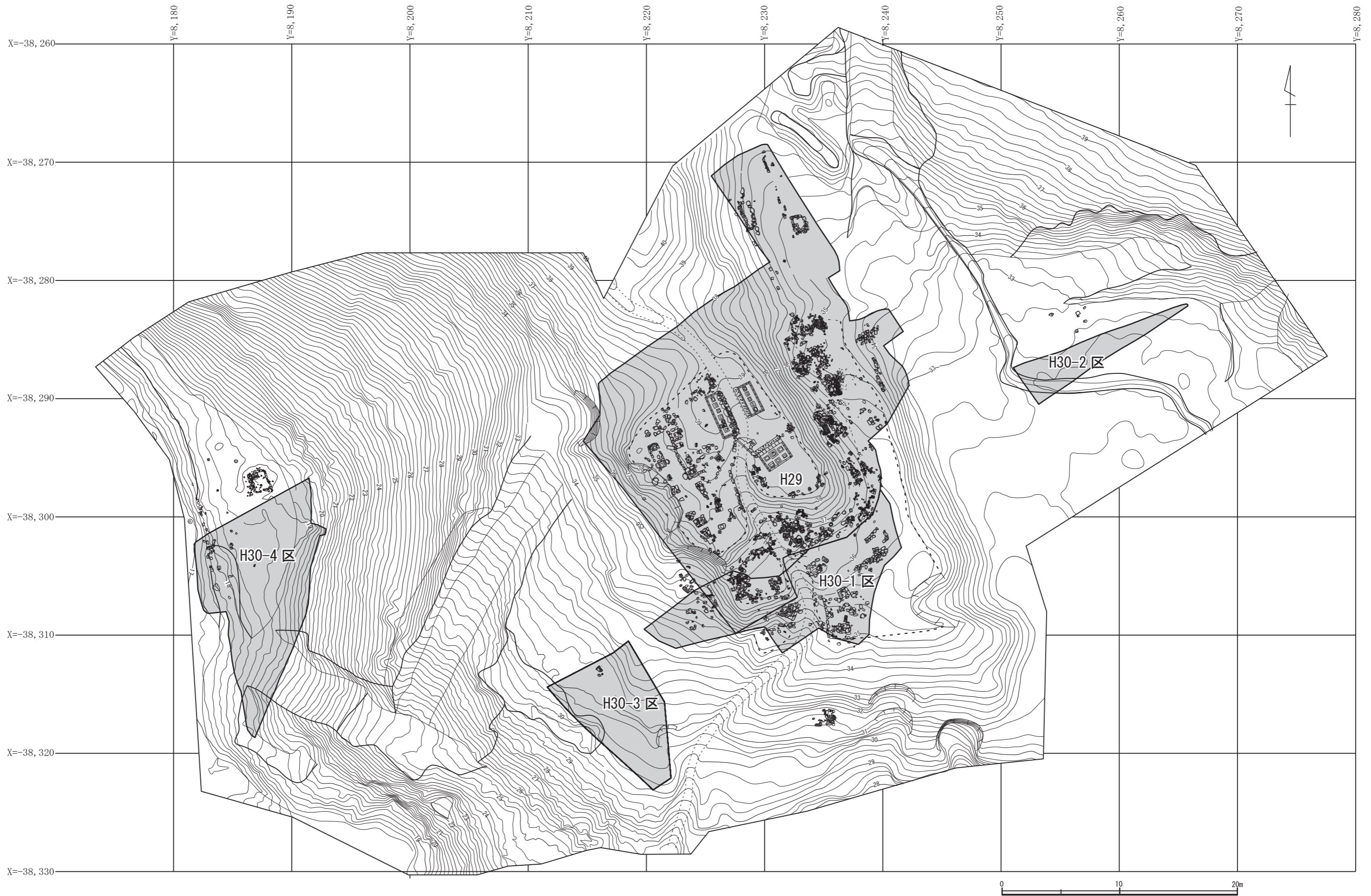
第2図 現況測量図 (縮尺 1 / 300)
