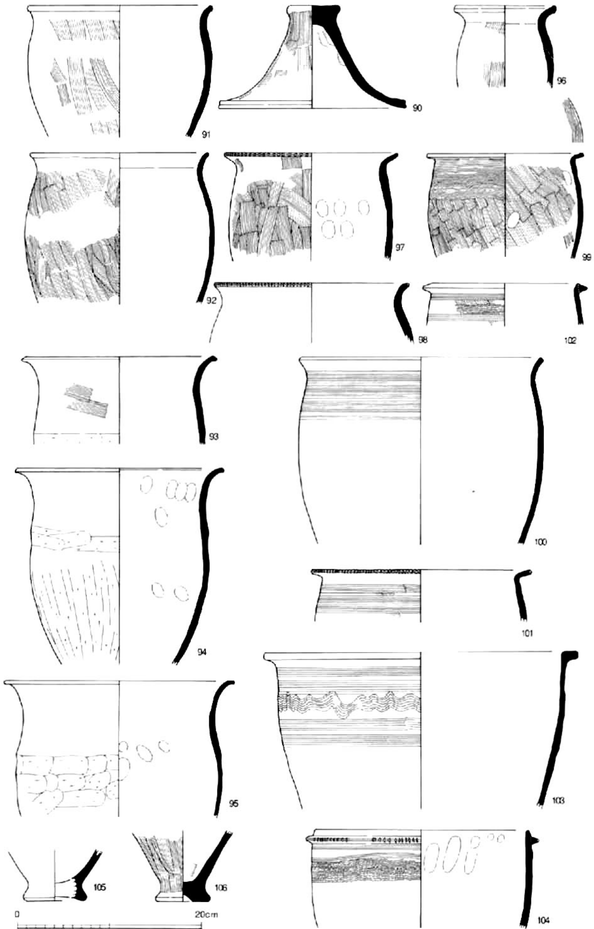
土器3 (溝/90~106)
