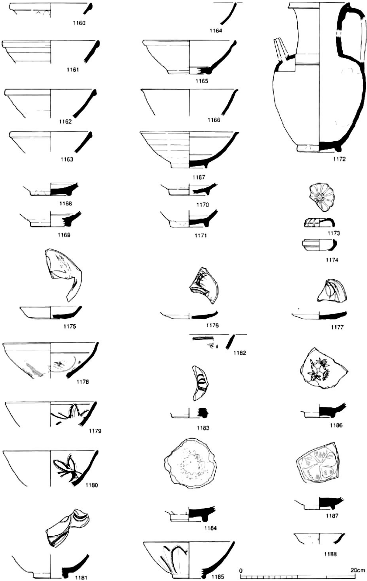
輸入磁器 (1160~1188)
