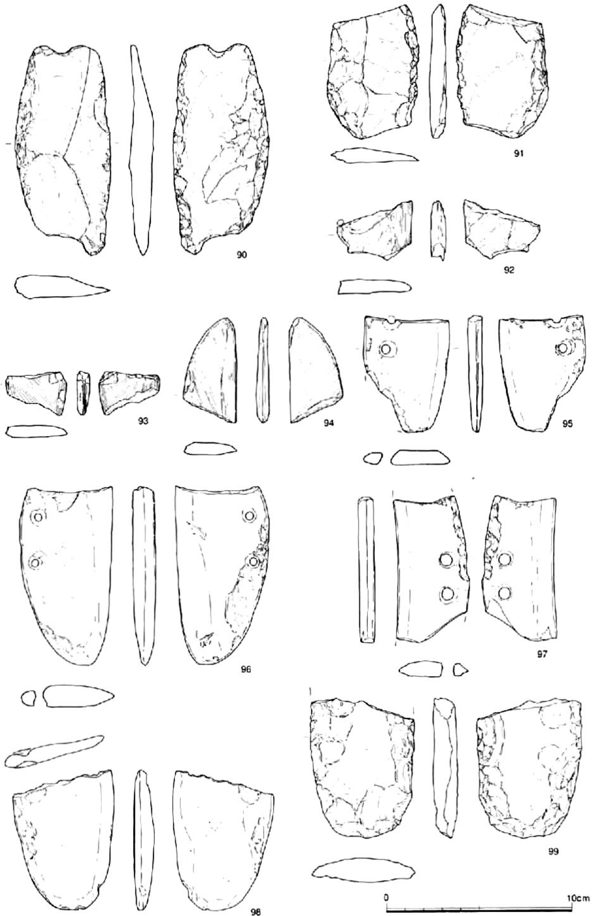
石器7 (90~99) [下層:92]
