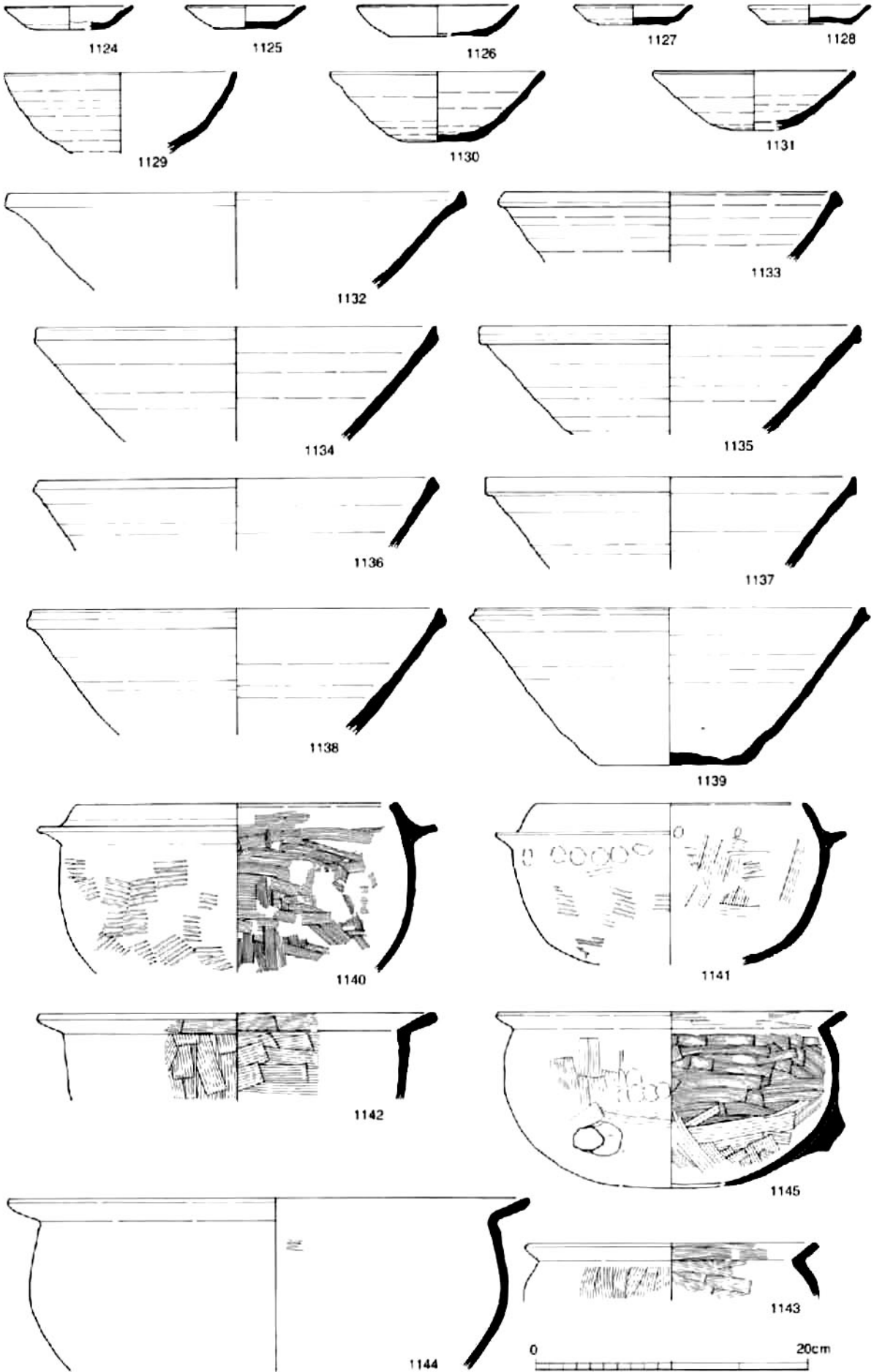
土器13 (土器群/1124~1145)
