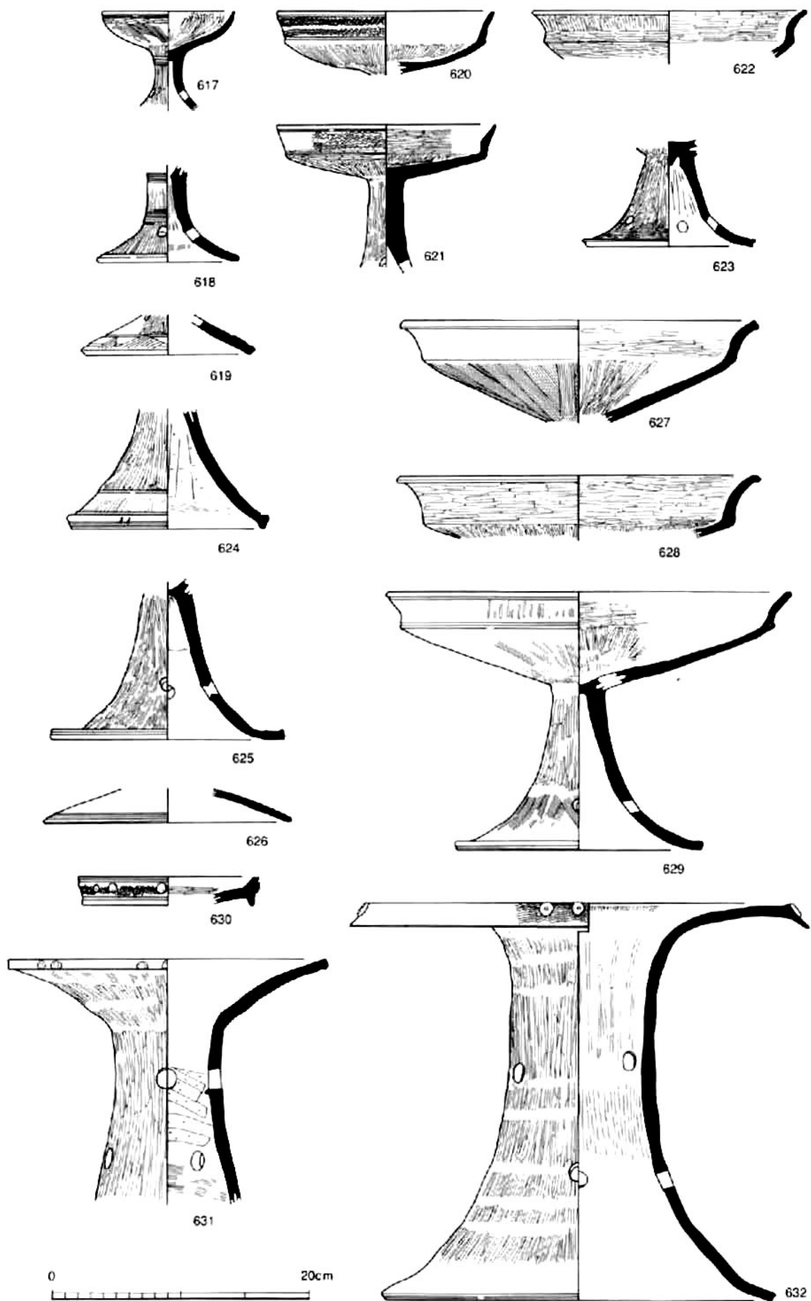
土器4 (河道/617~632)
