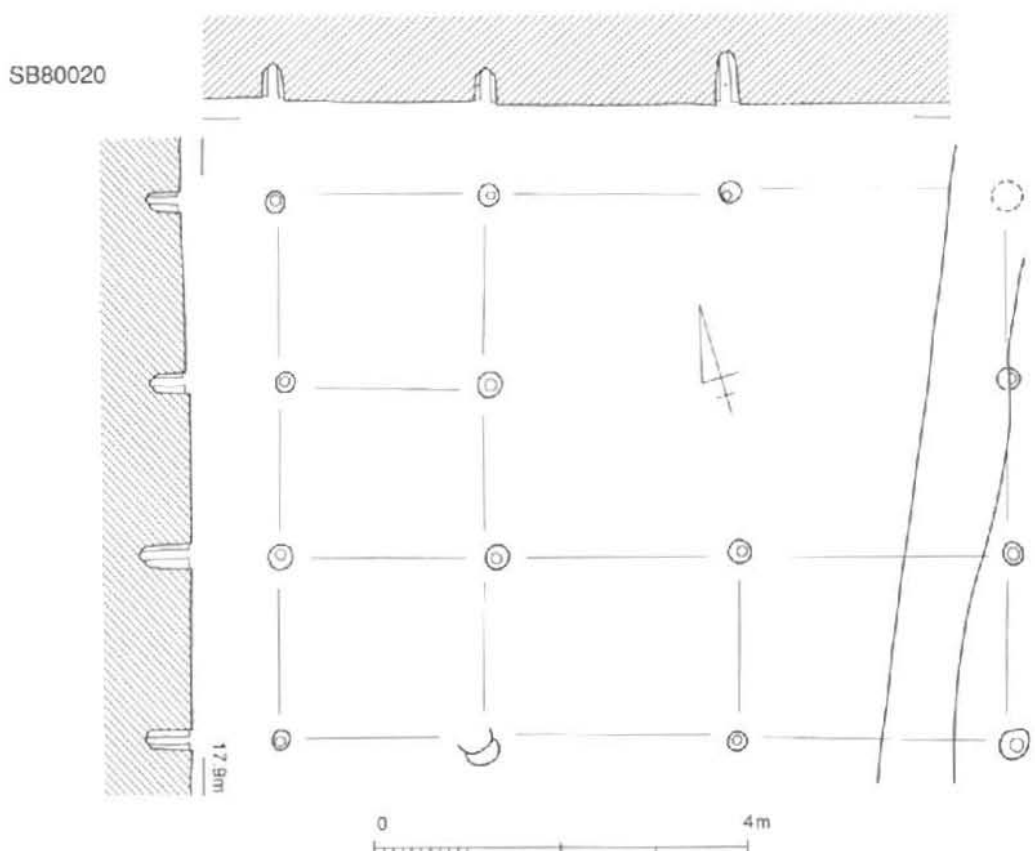
掘立柱建物10 (SB80019・80020)
