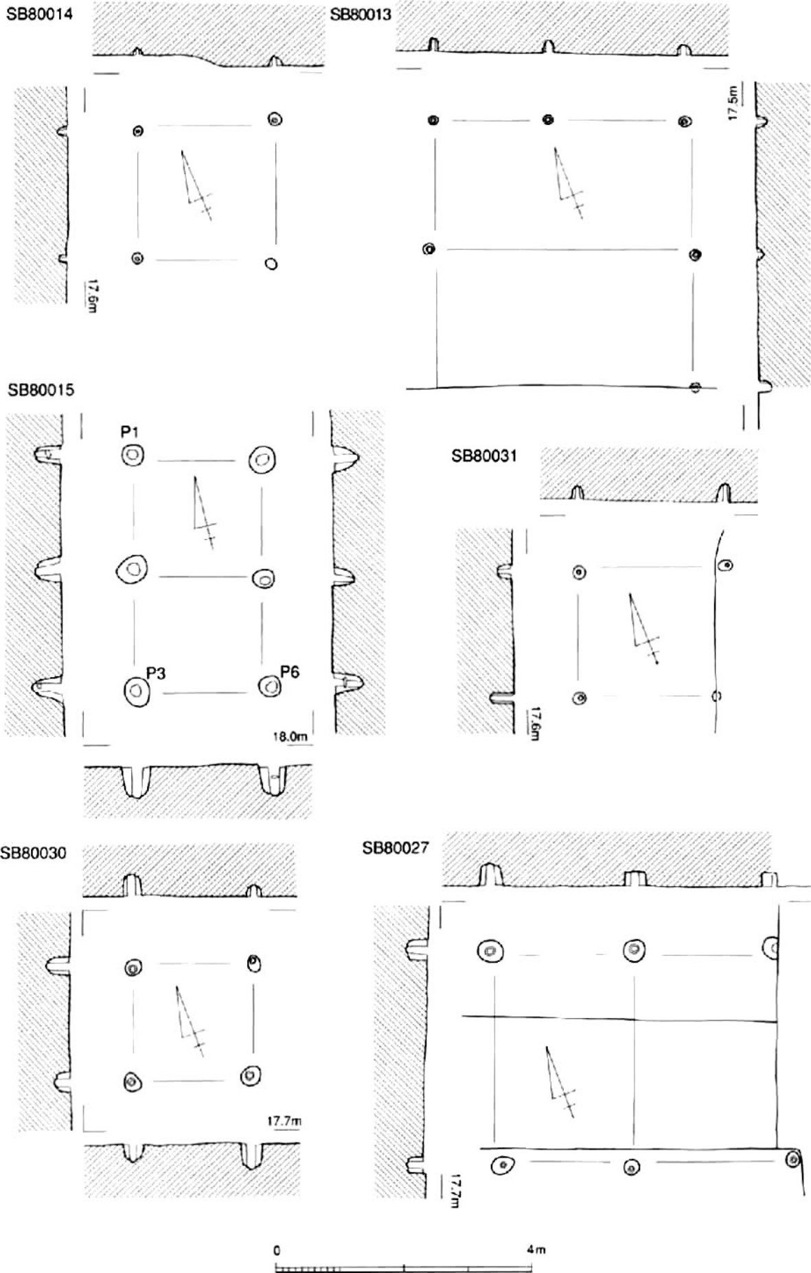
掘立柱建物7 (SB80013~80015・80027・80030・80031)
