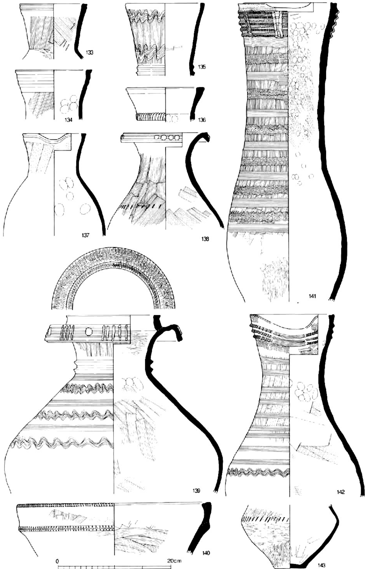
土器2 (河道/133~143)
