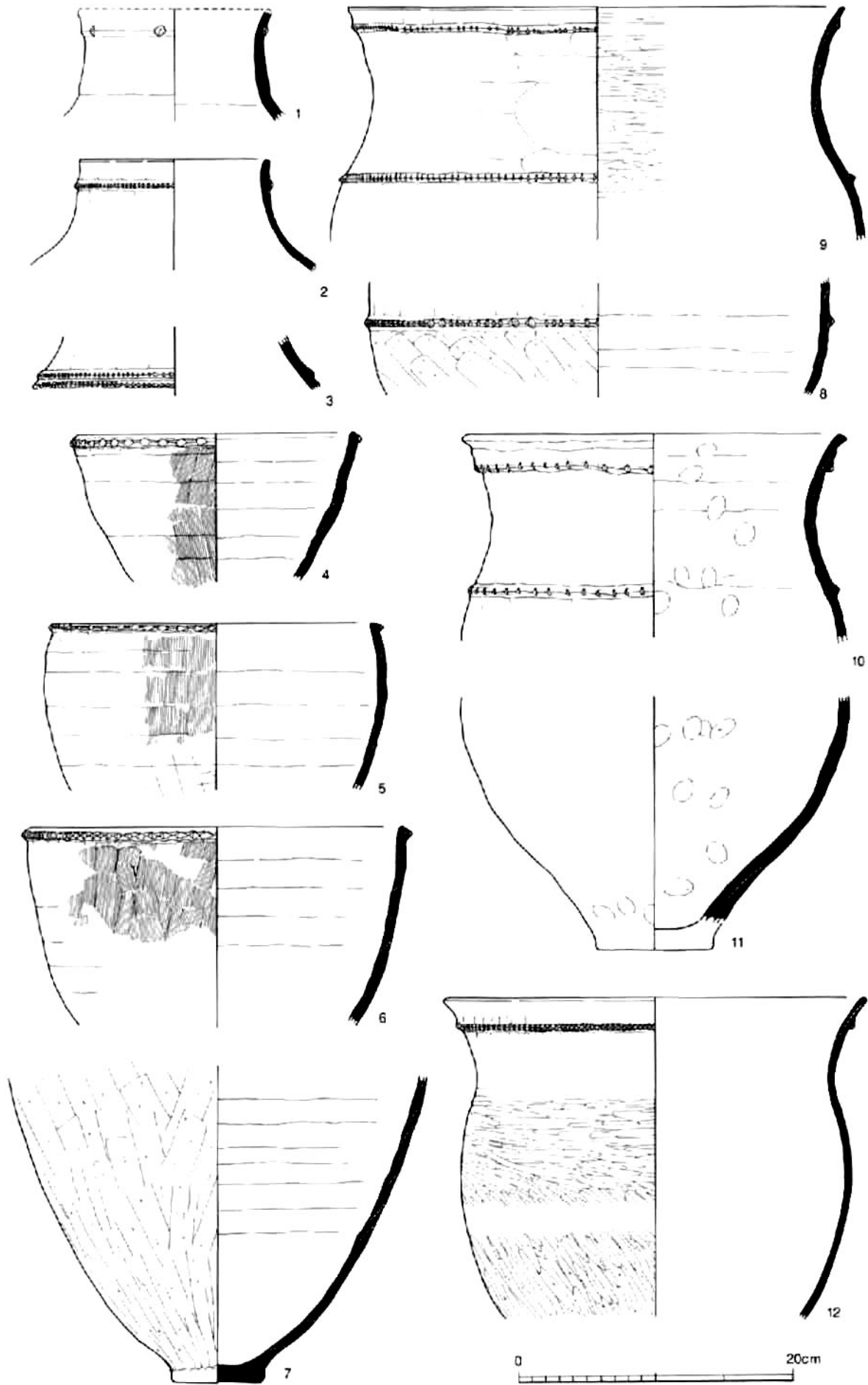
土器1 (河道/1~12)
