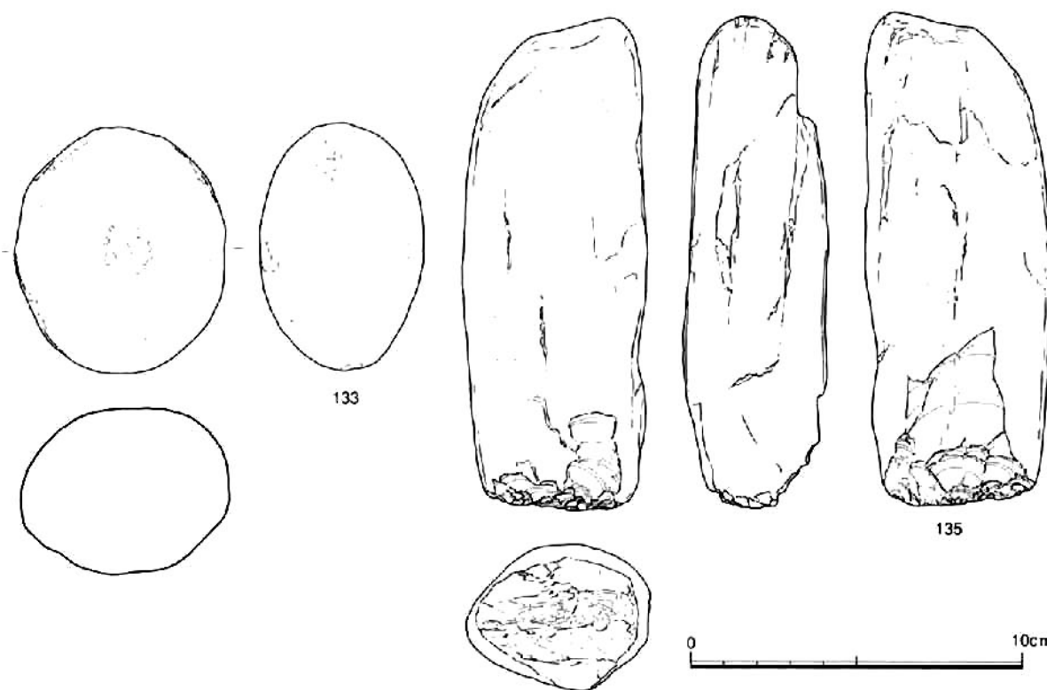
石器12 (130~135) [下層:132]
