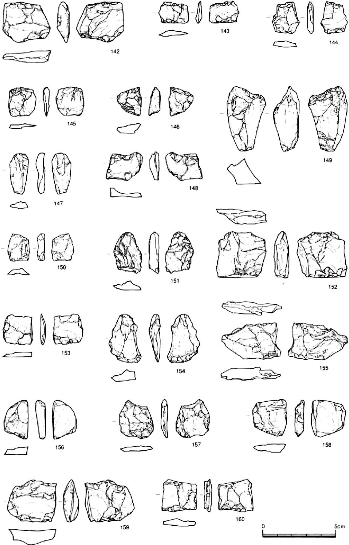
石器14 (142~160)
