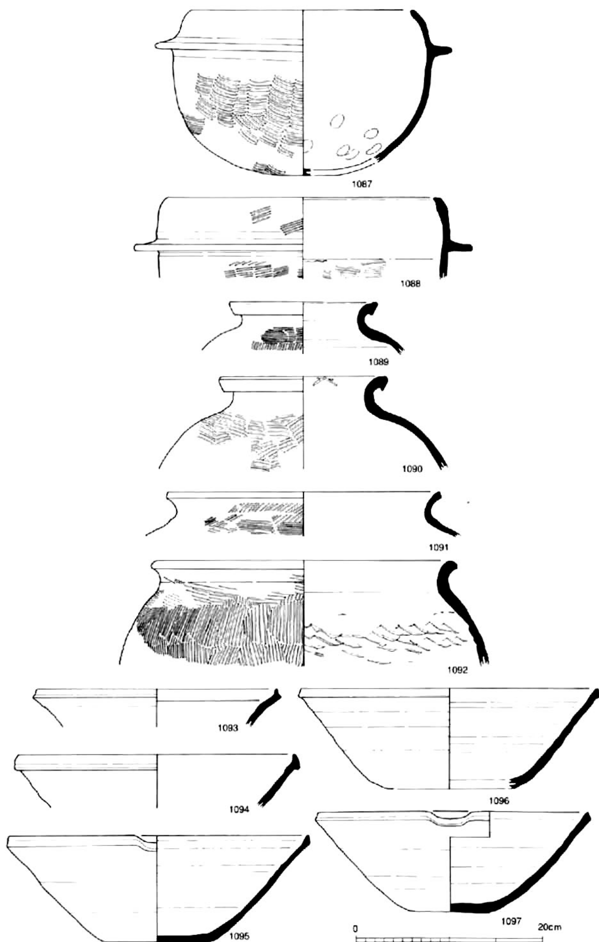
土器11 (土坑/1087~1097)
