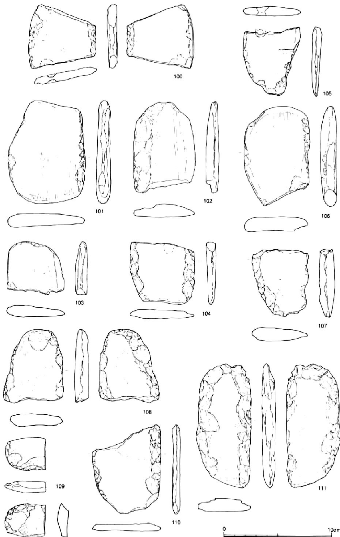
石器8 (100~111) [下層: 100・102]
