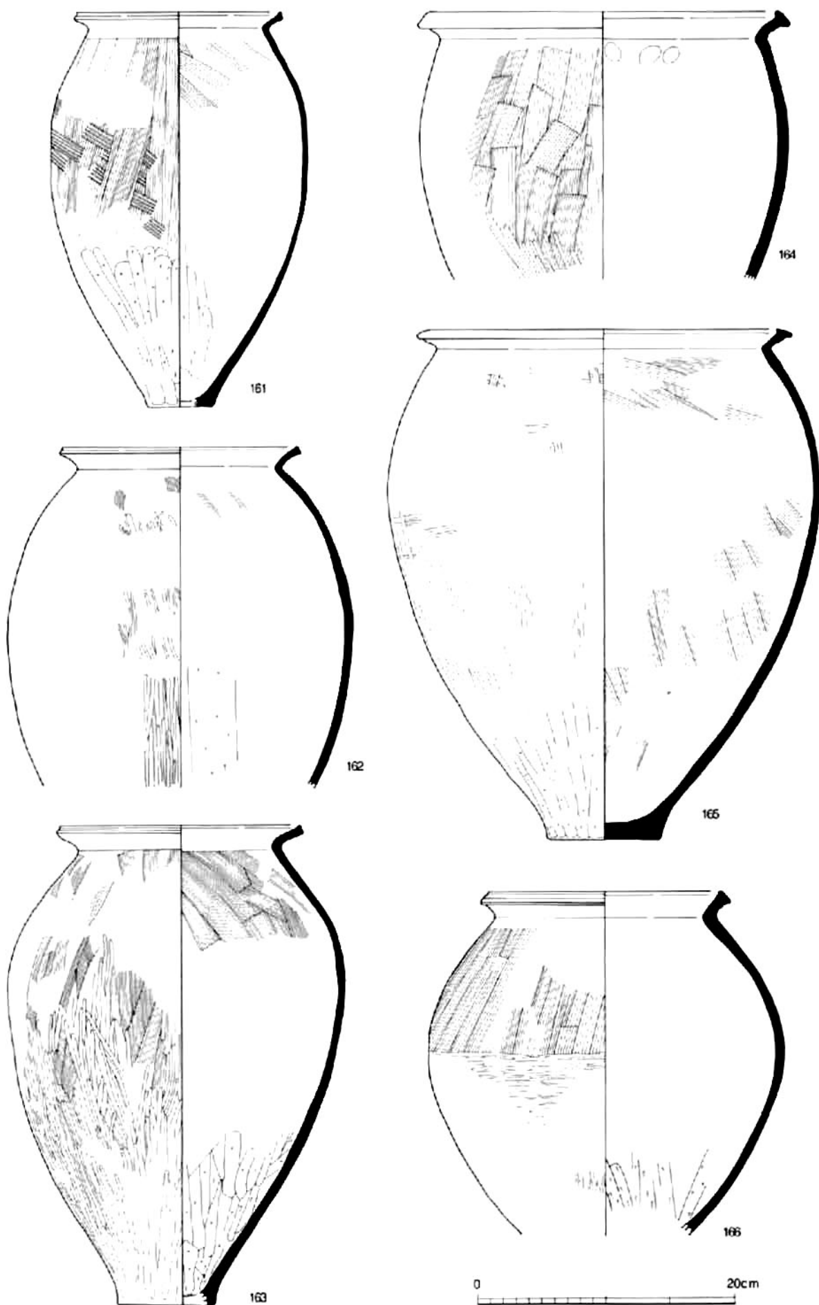
土器4 (河道/161~166)
