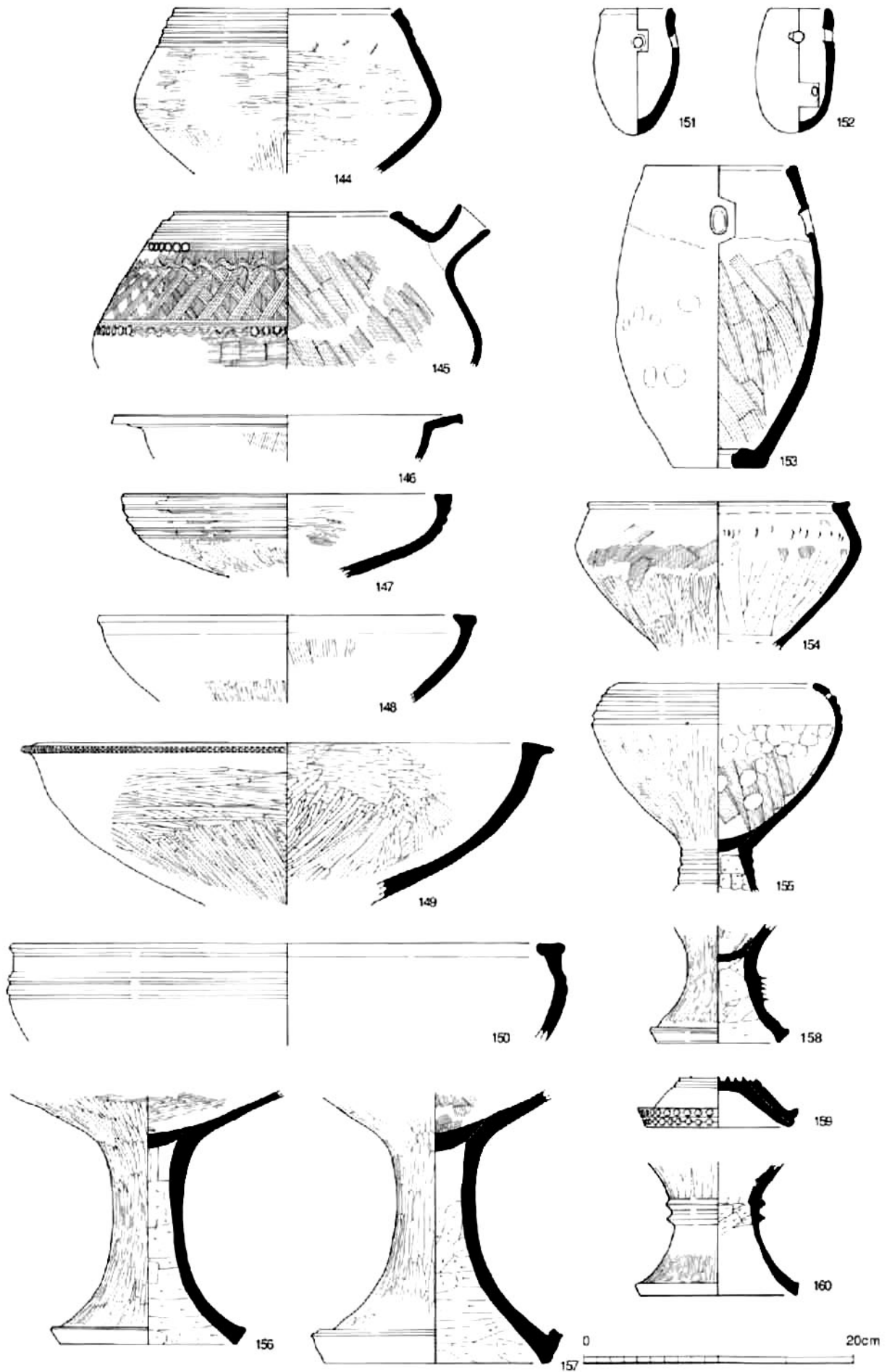
土器3 (河道/144~160)
