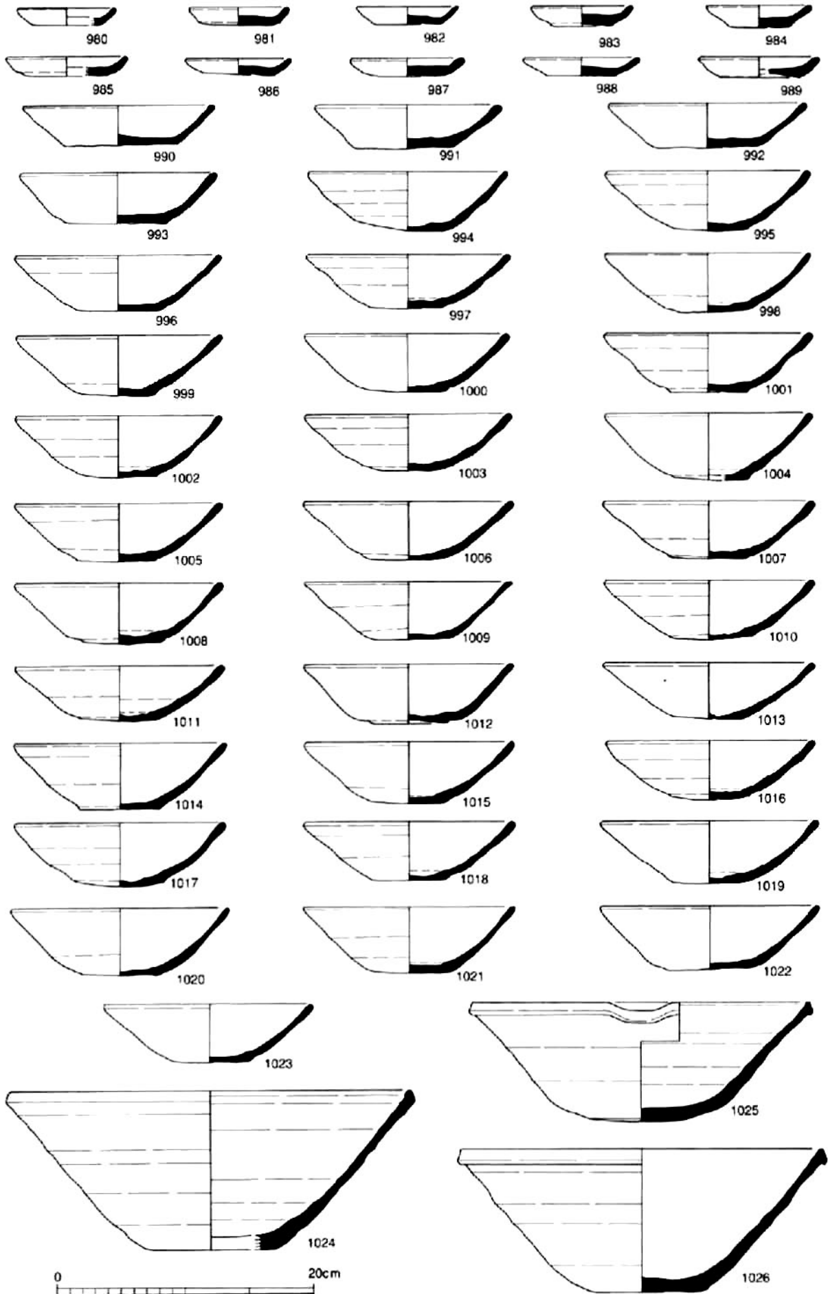
土器6 (土坑/980~1026)
