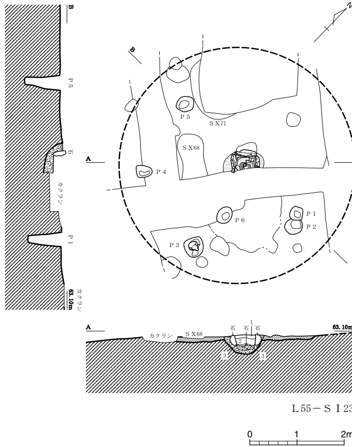
1. L 55 - S I 23 実測図 (1/80)
