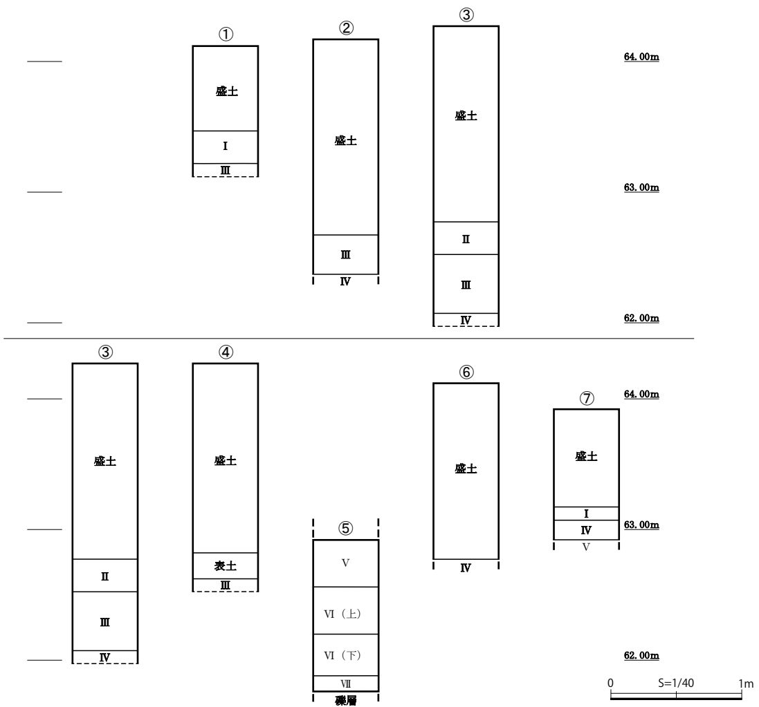
第6図 基本土層観察位置図 (1/400), 柱状図 (1/40)
