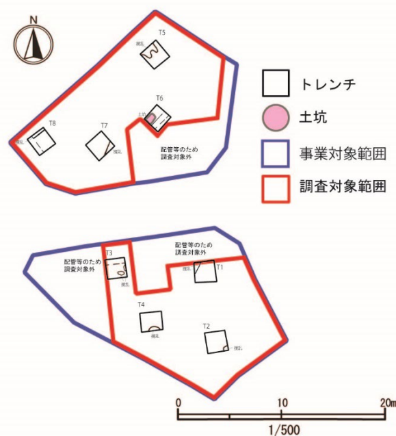
第 19 図：遺構配置図
