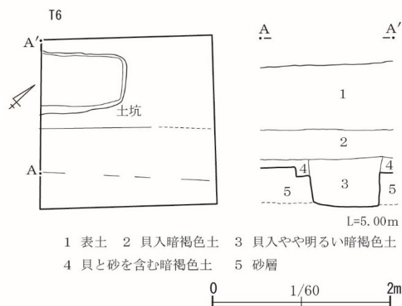
第 20 図：遺構セクション図
