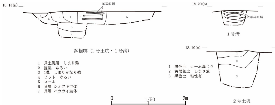
第5図：遺構セクション図
