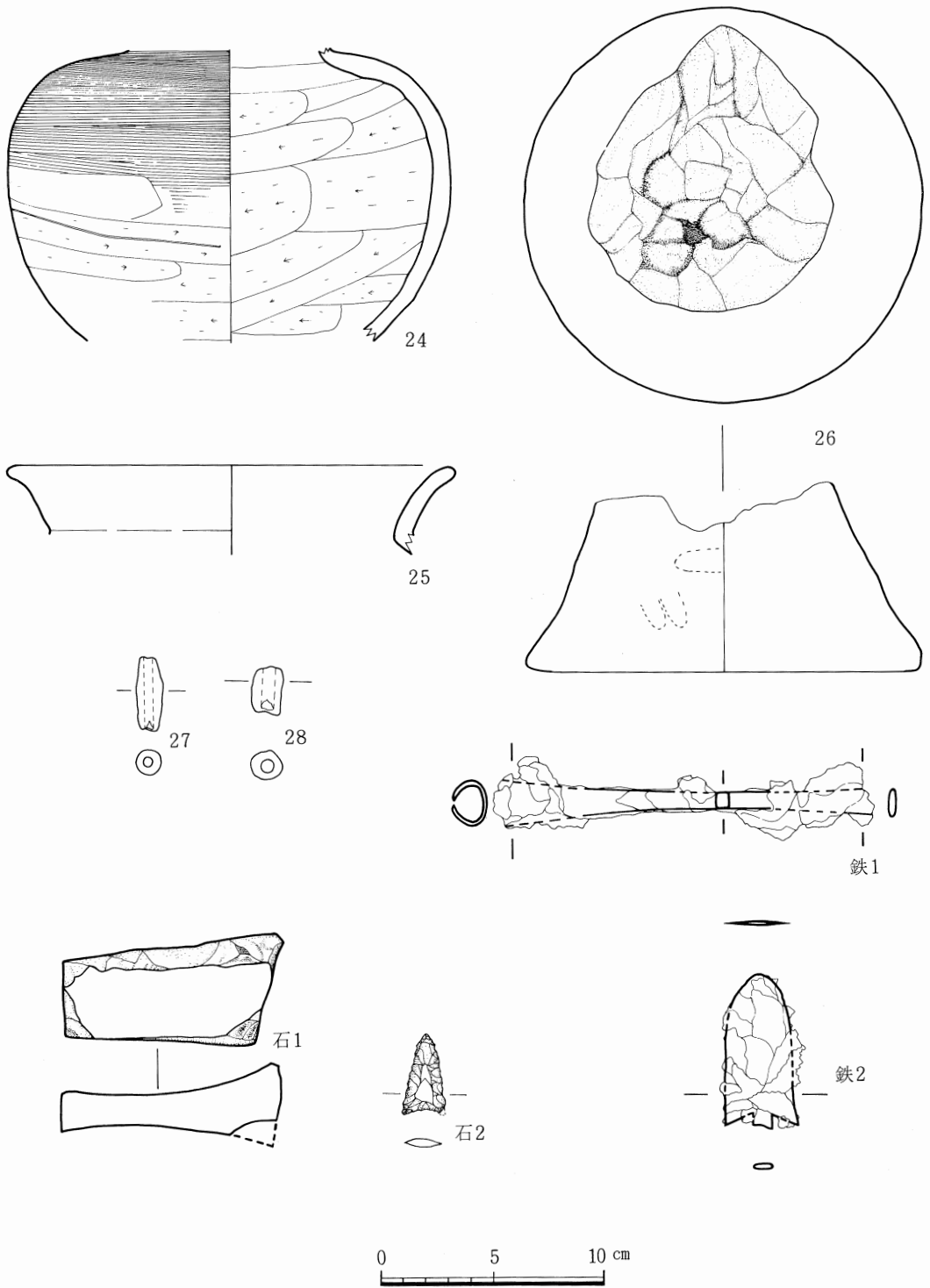
第 8 図 土師器、石器、鉄器実測図
