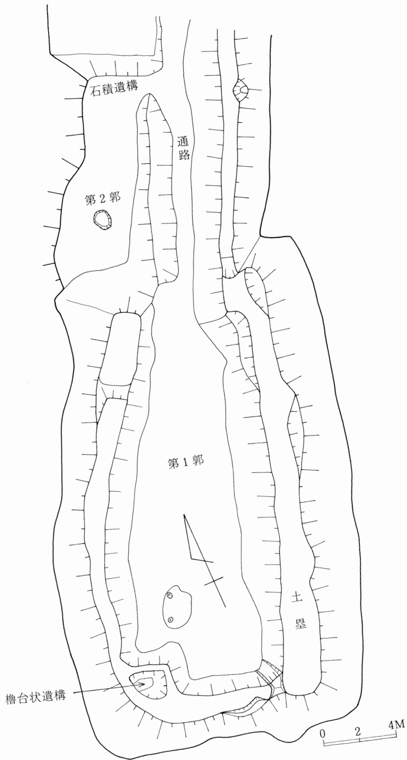
第4図 平面実測図 (調査後)
