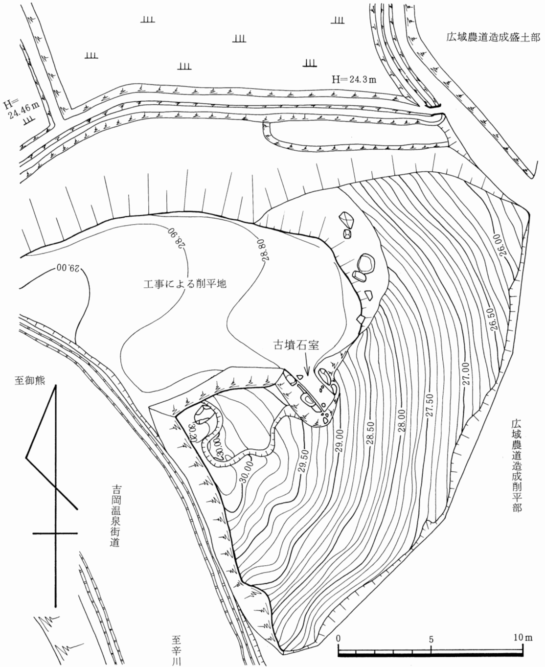
第3図 地形実測図（調査前）
