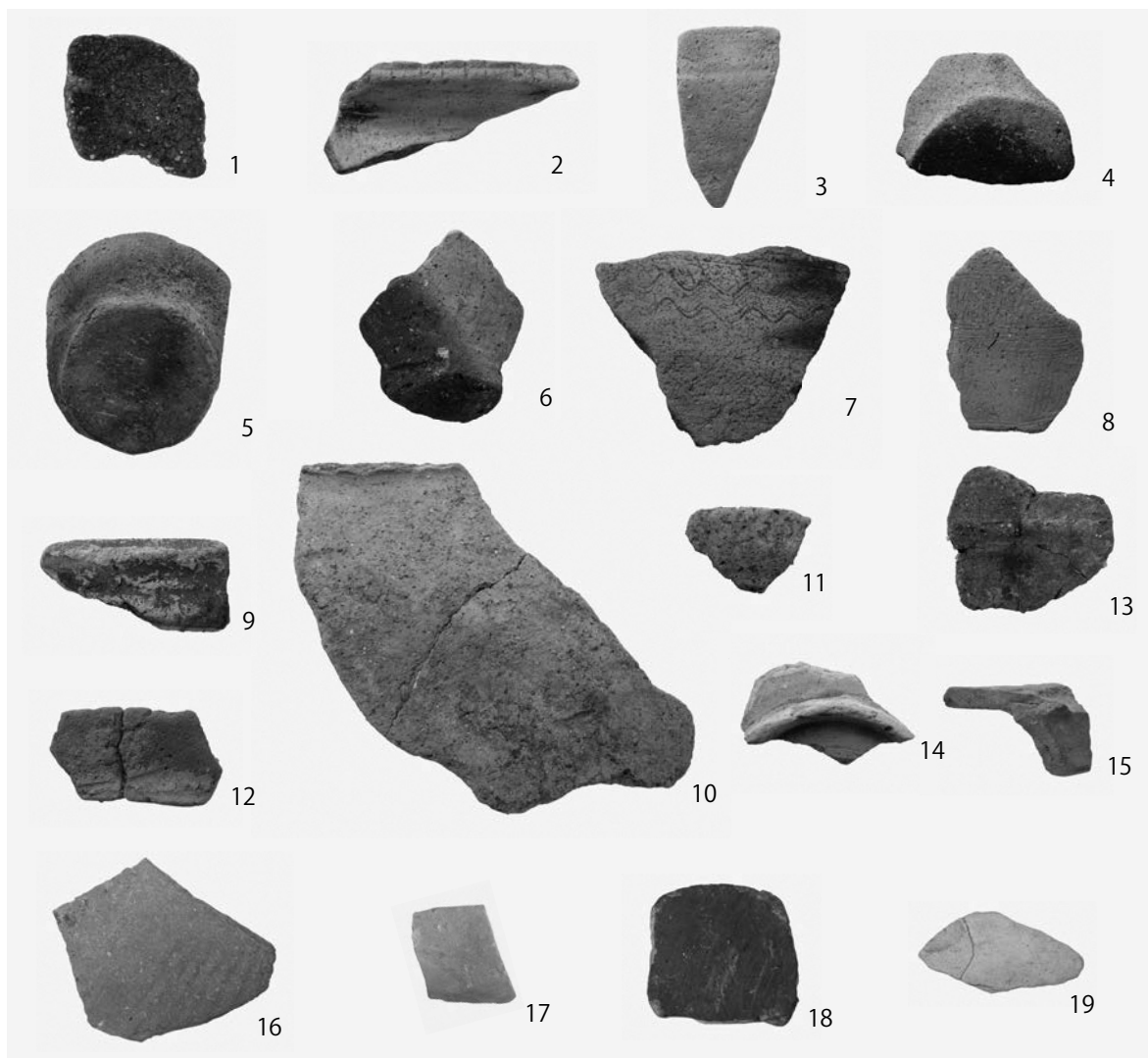
1. 出土遺物
