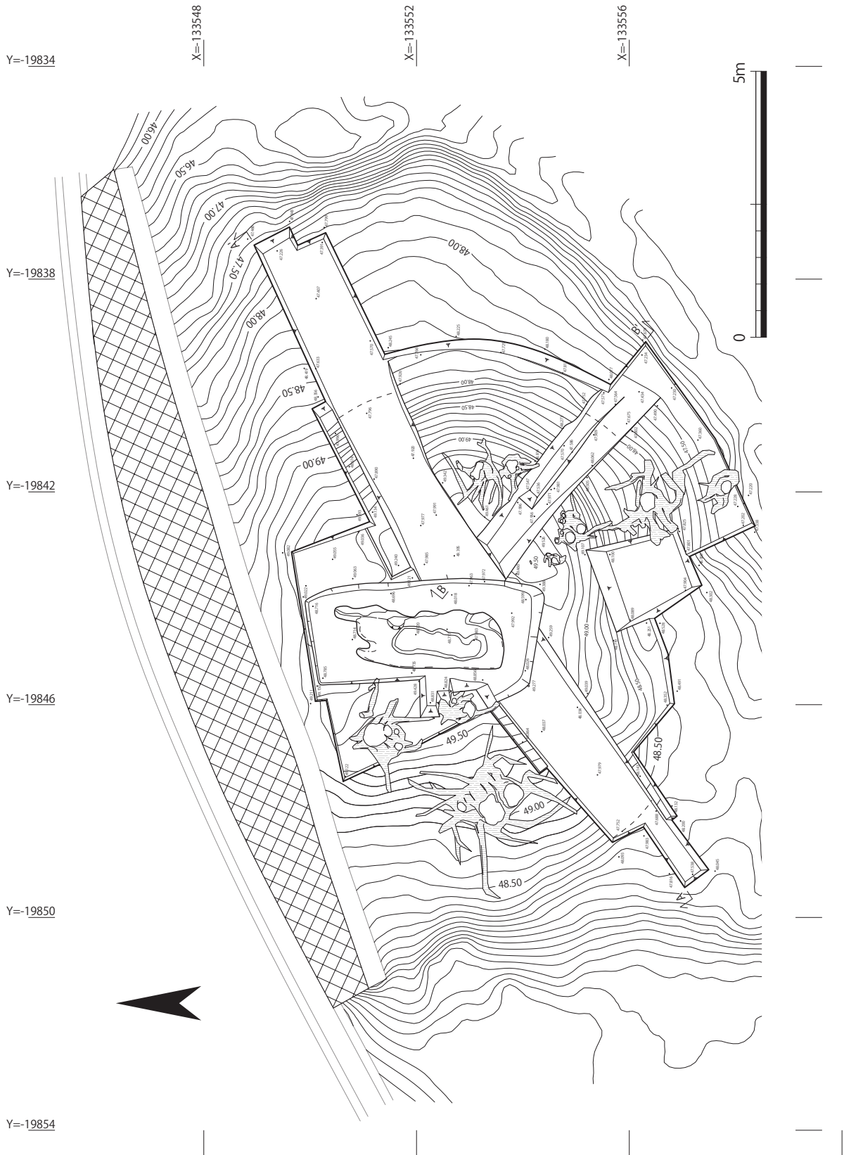
第7図 平面図 (1 / 100)
