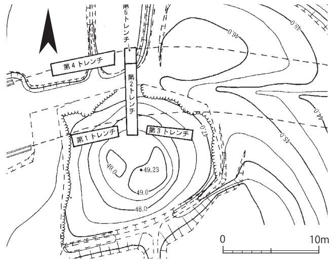
第4図 昭和46年測量図(田辺町1981)(1/400)
