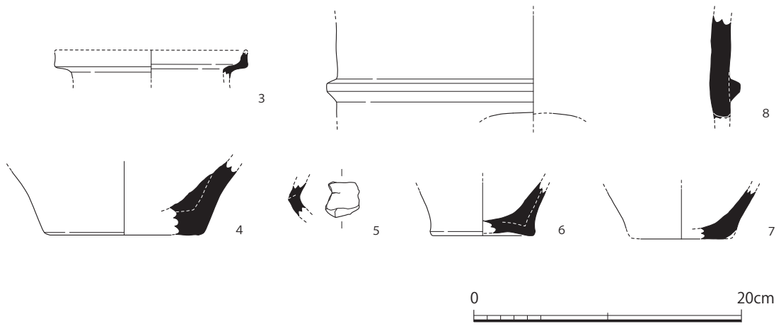
第13図 盛土内遺物1 (1/4)
