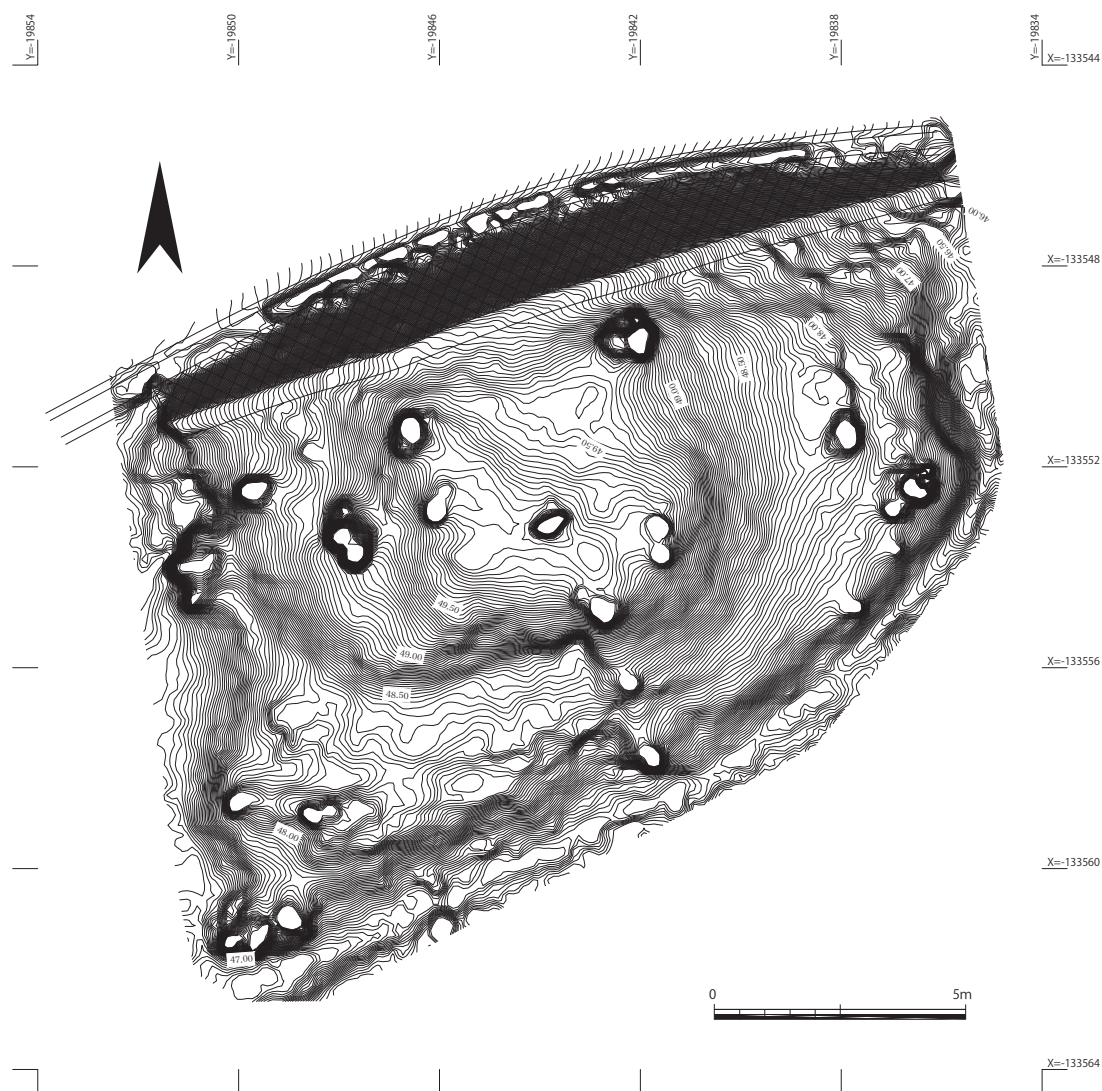
第3図 調査前測量図(1/120)
