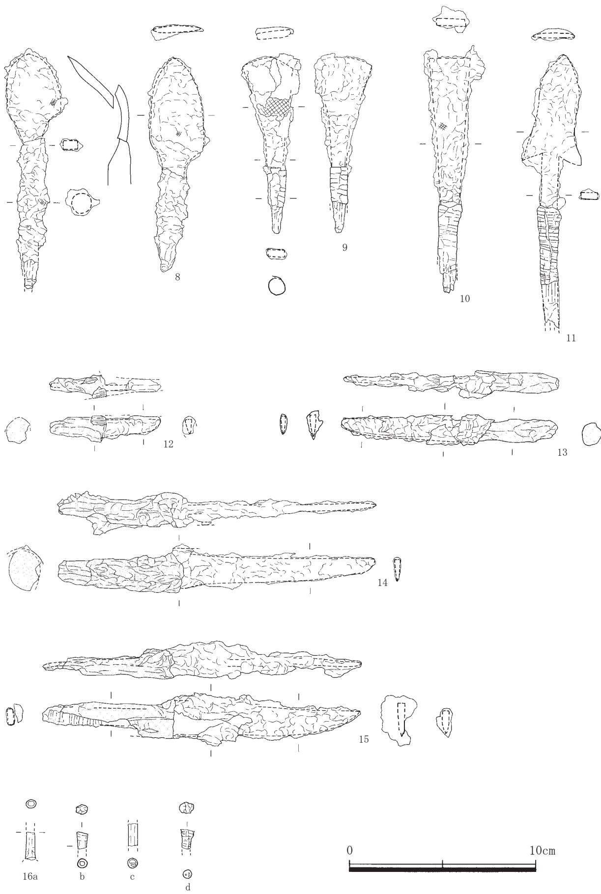
第13图 ST-178 出土遺物実測図(1)
