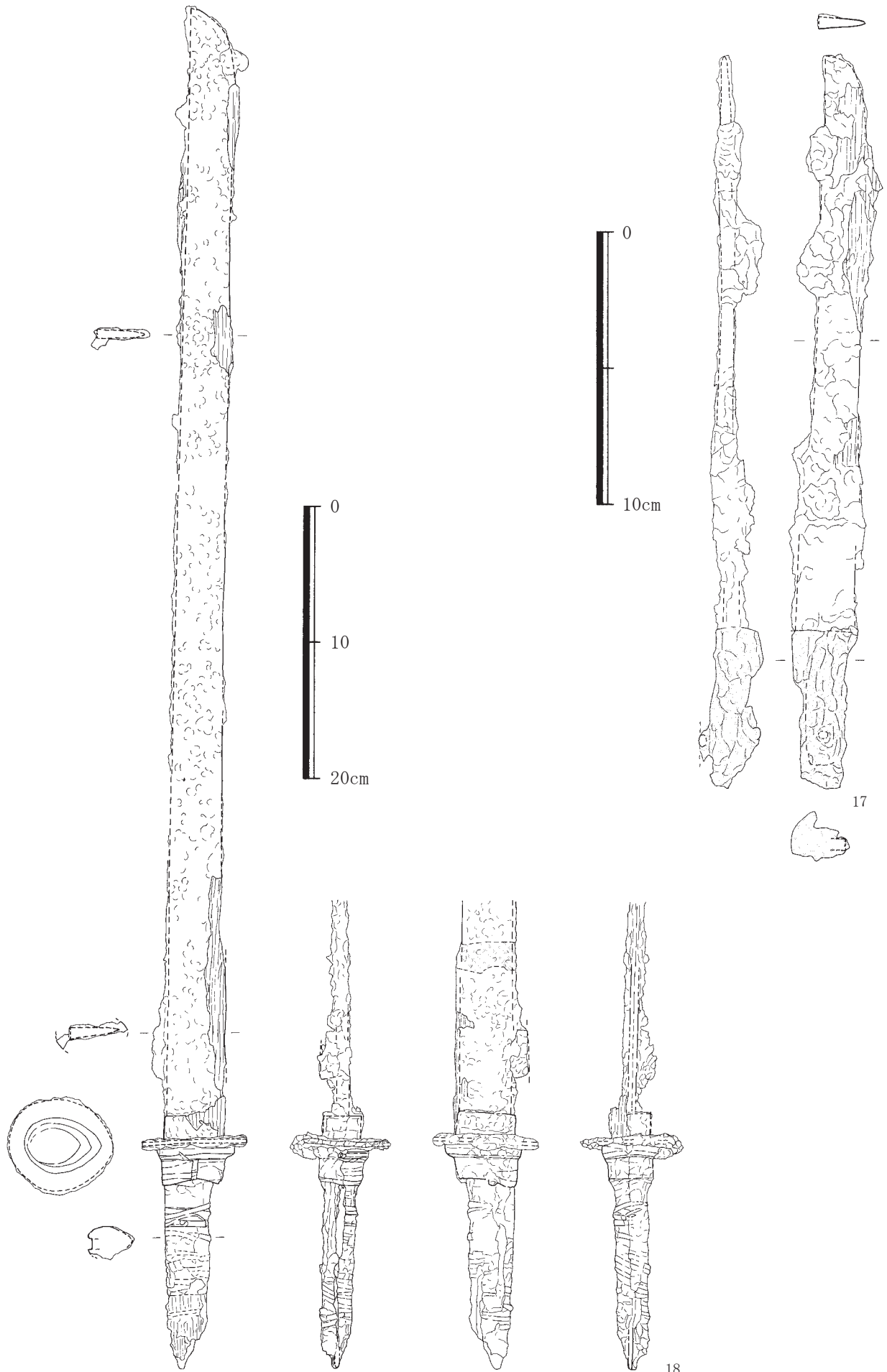
第14图 ST-178 出土遺物実測図(2)
