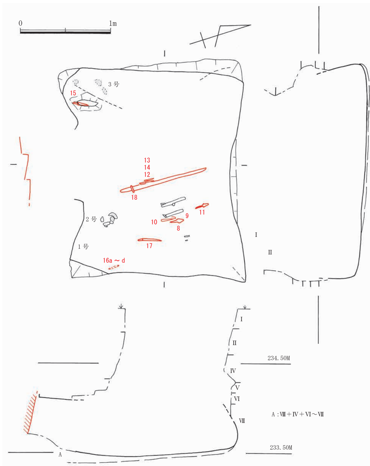
第 11 図 ST-178 遺構実測図
