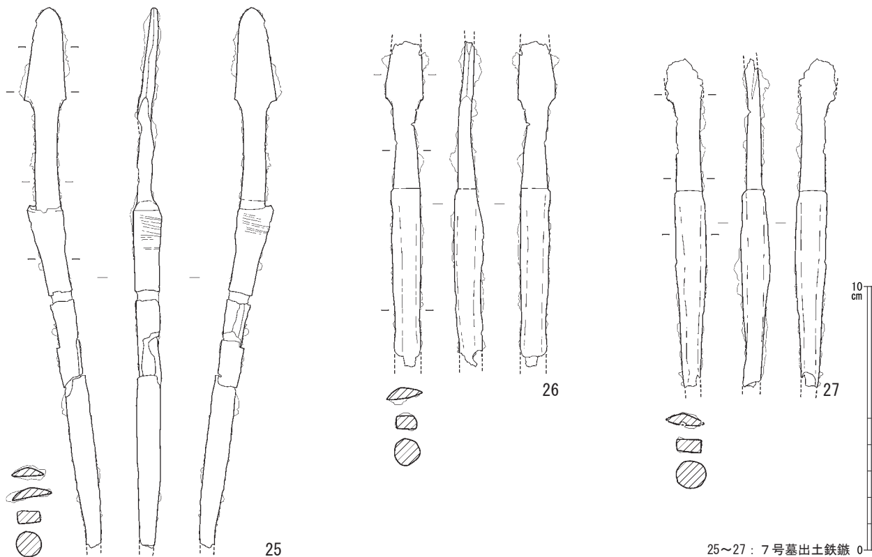
第4図 島内4・7号墓出土鉄鏃(2)
