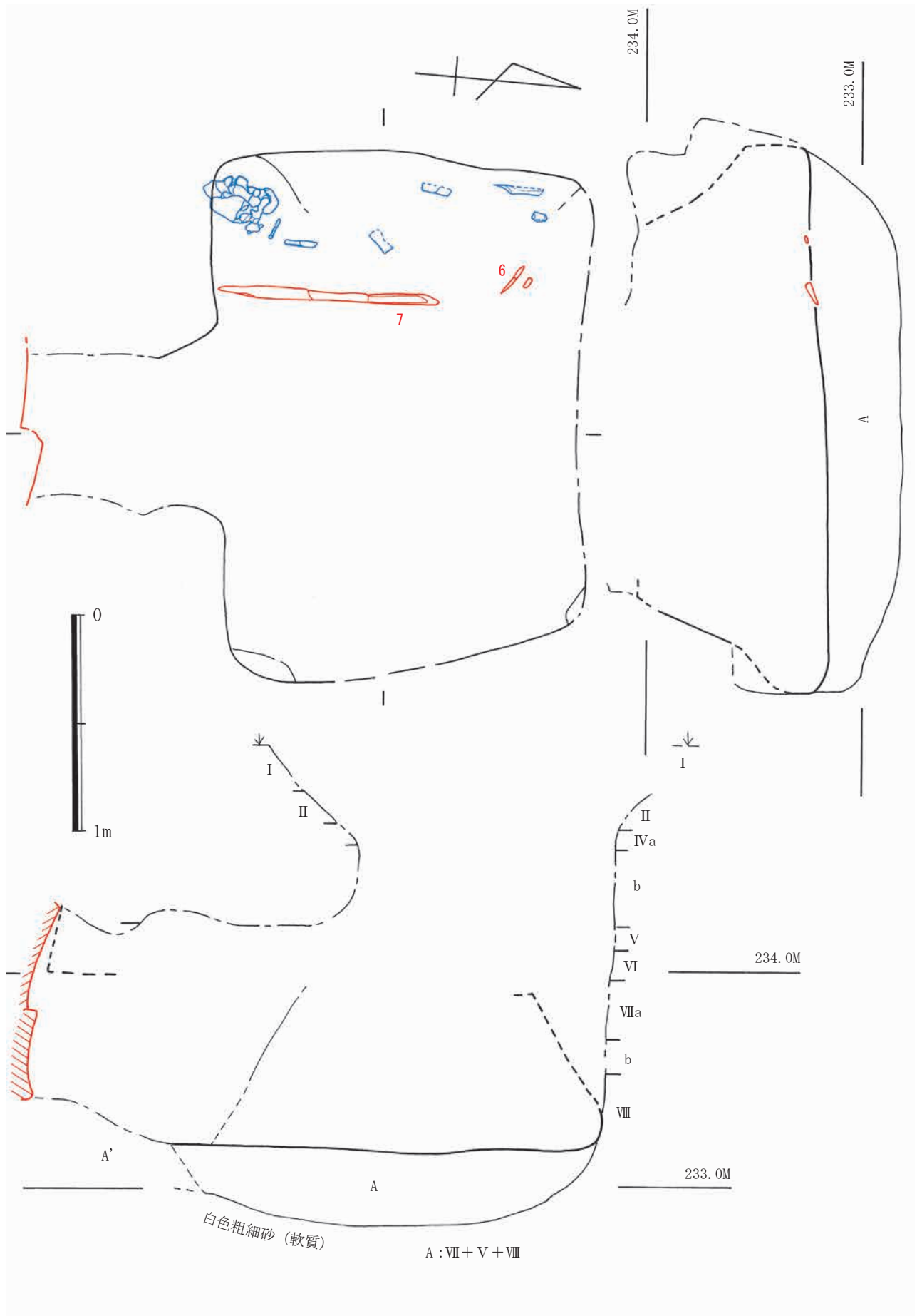
第9図 ST-177 遺構実測図
