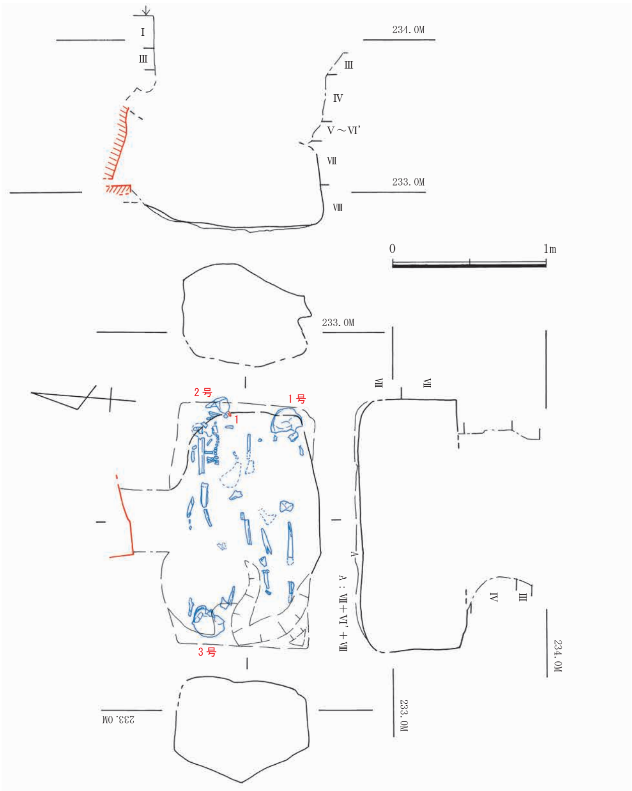
第4図 ST-175 遺構実測図
