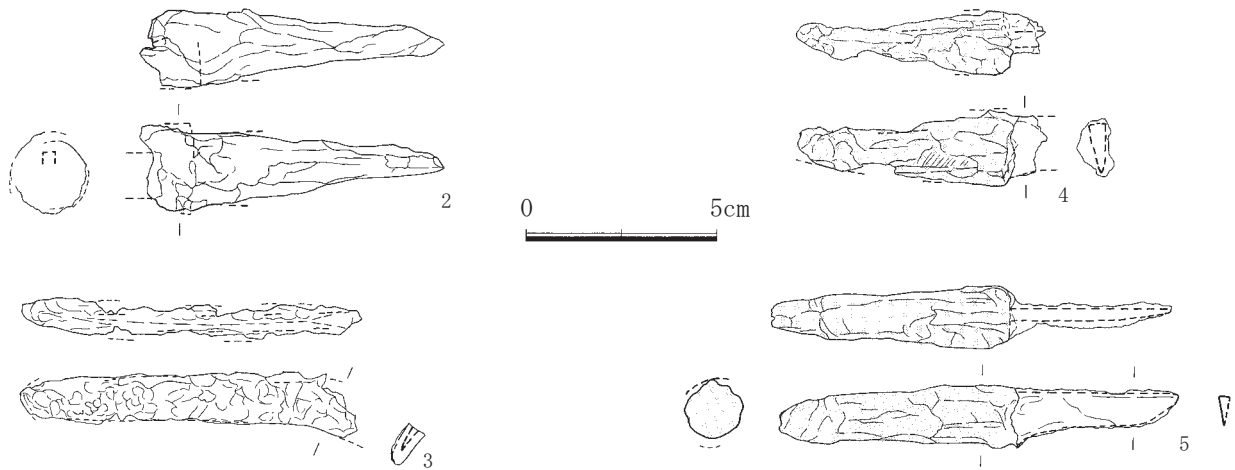
第8図 ST-176 出土遺物実測図
