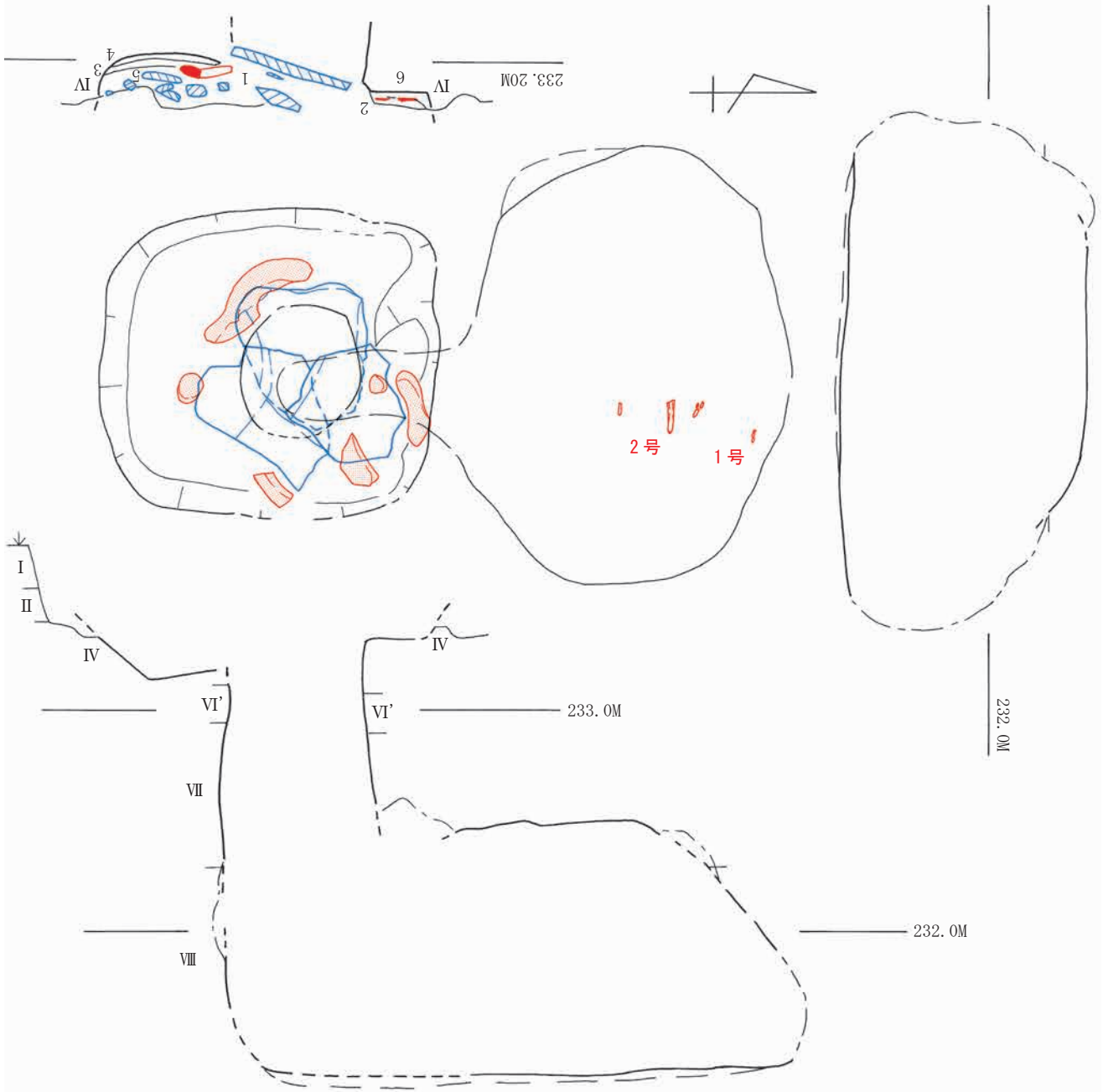
第 15 図 ST-179 遺構実測図
