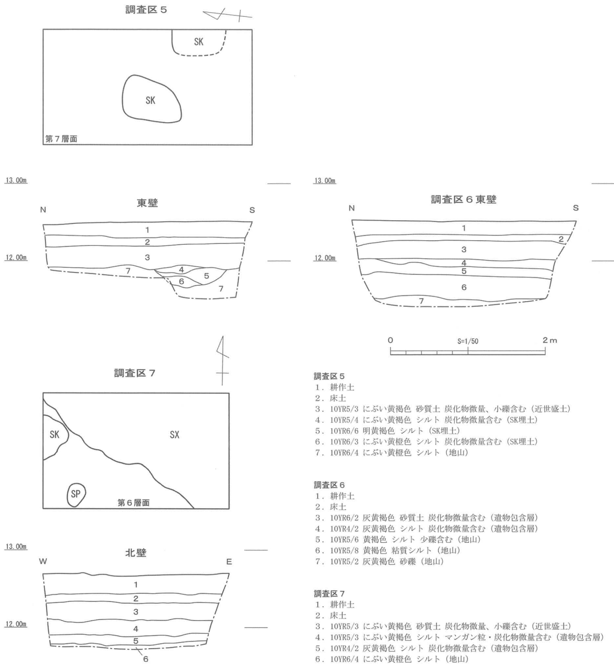
図9 調査区5～7平面図、土層断面図
