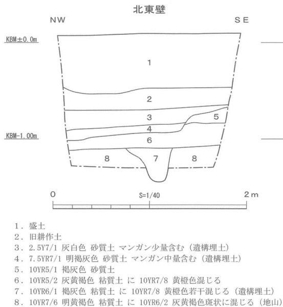
図 17 調査区 1 土層断面図
