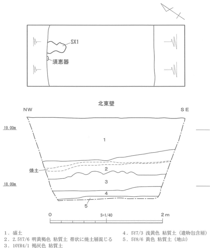
図4 調査区1平面図、土層断面図
