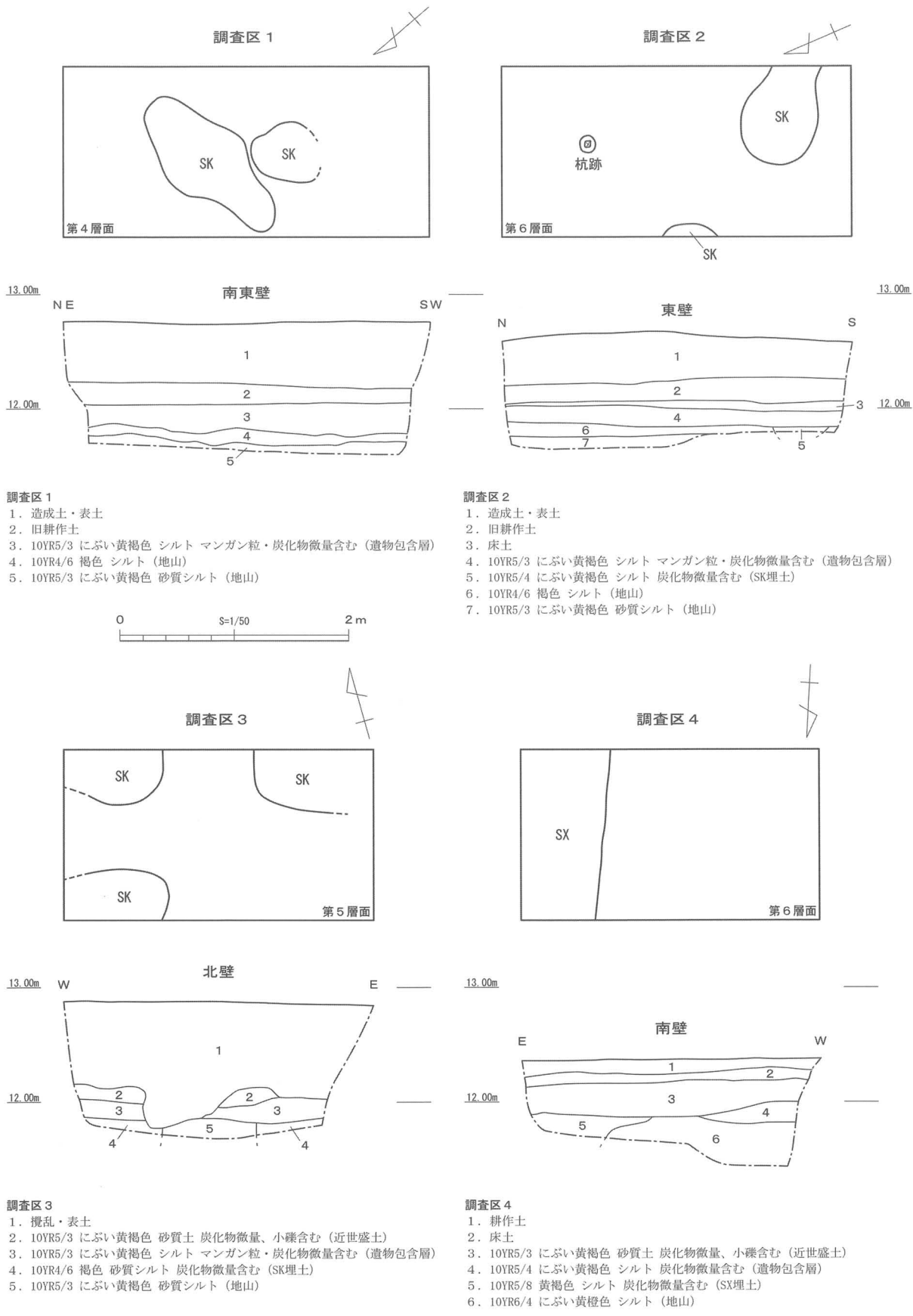
図8 調査区1～4平面図、土層断面図
