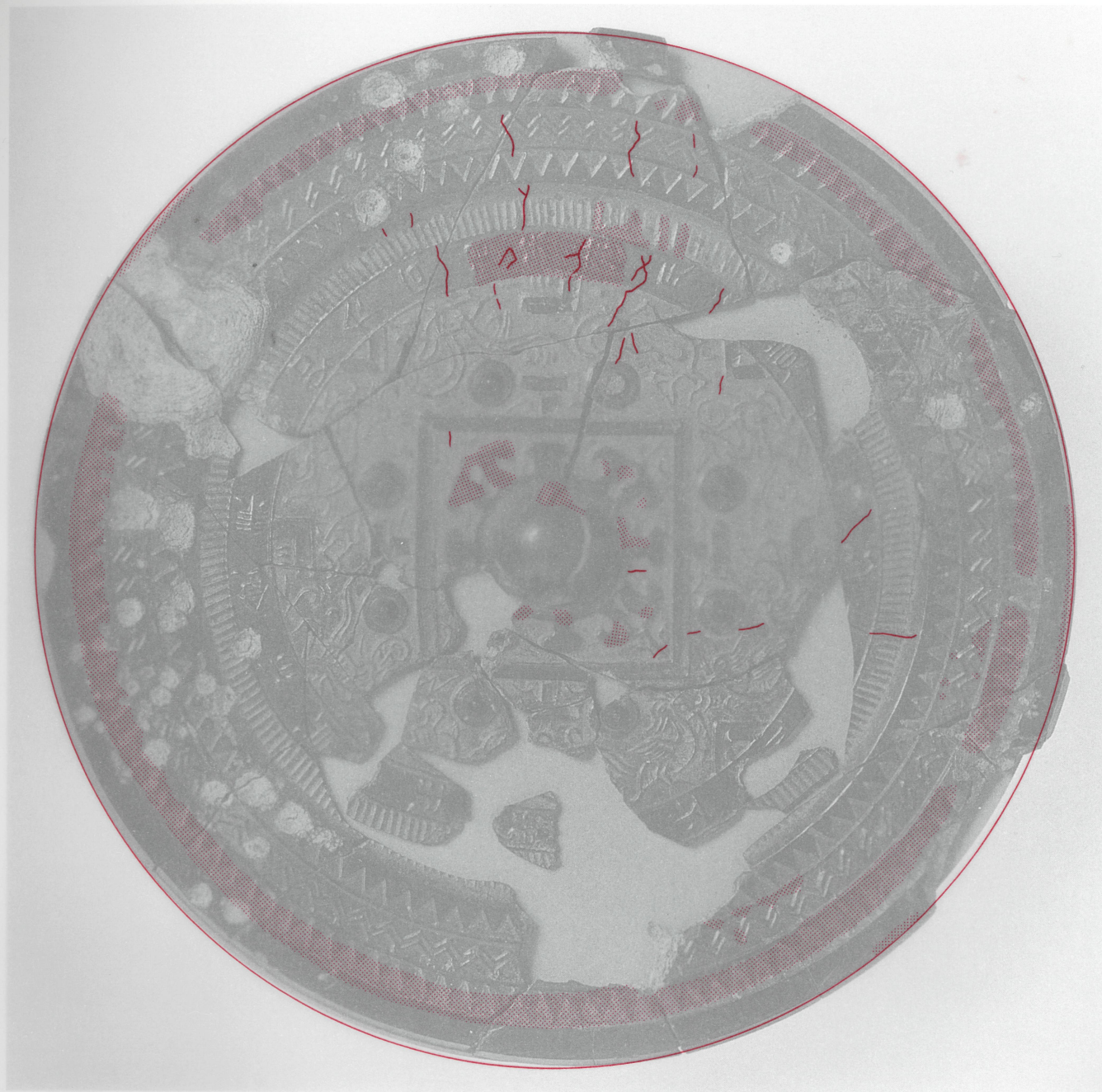
第 56 図 34号鏡鑄造関係観察図
