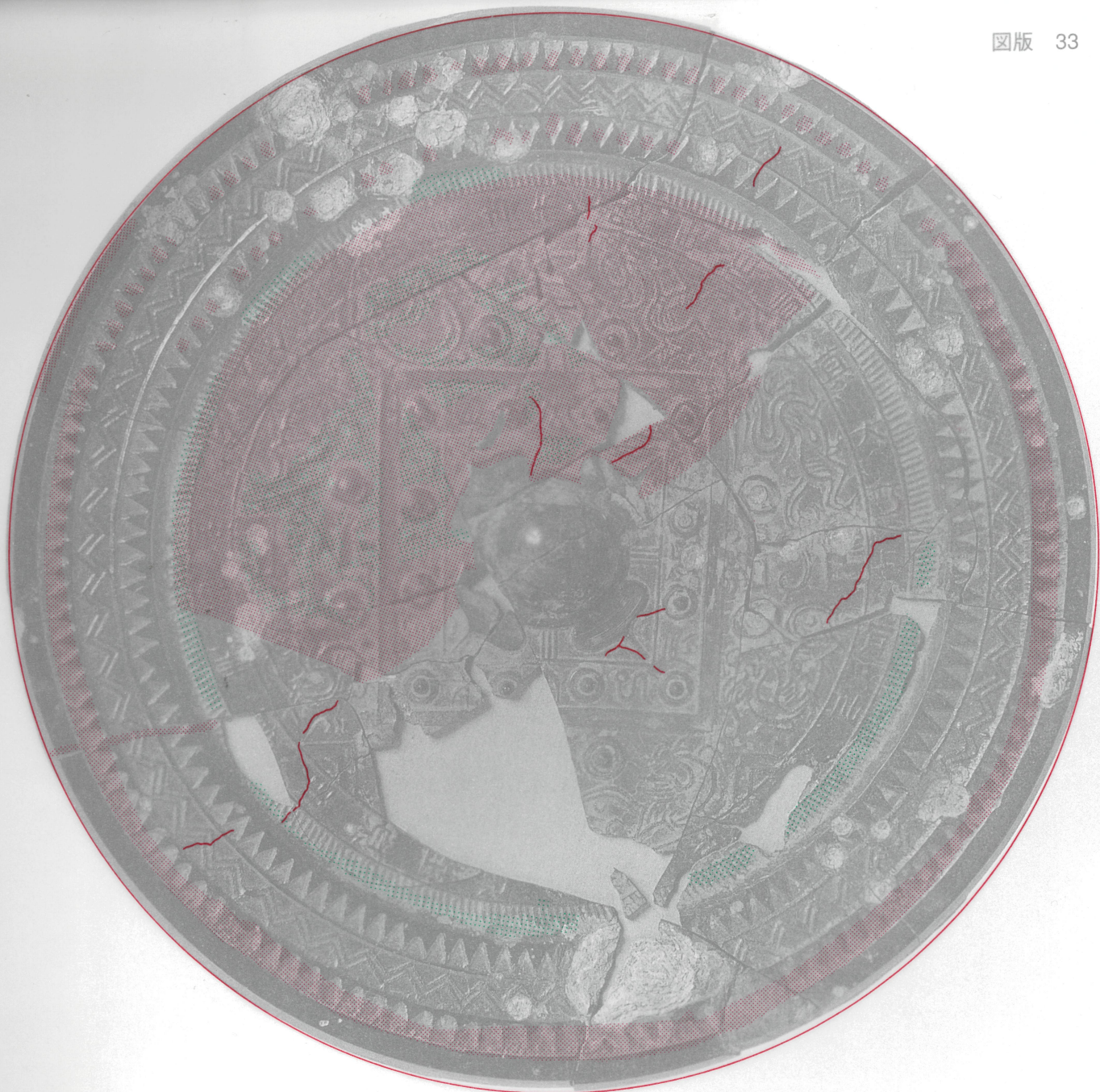
第 55 図 33号鏡鑄造関係観察図
