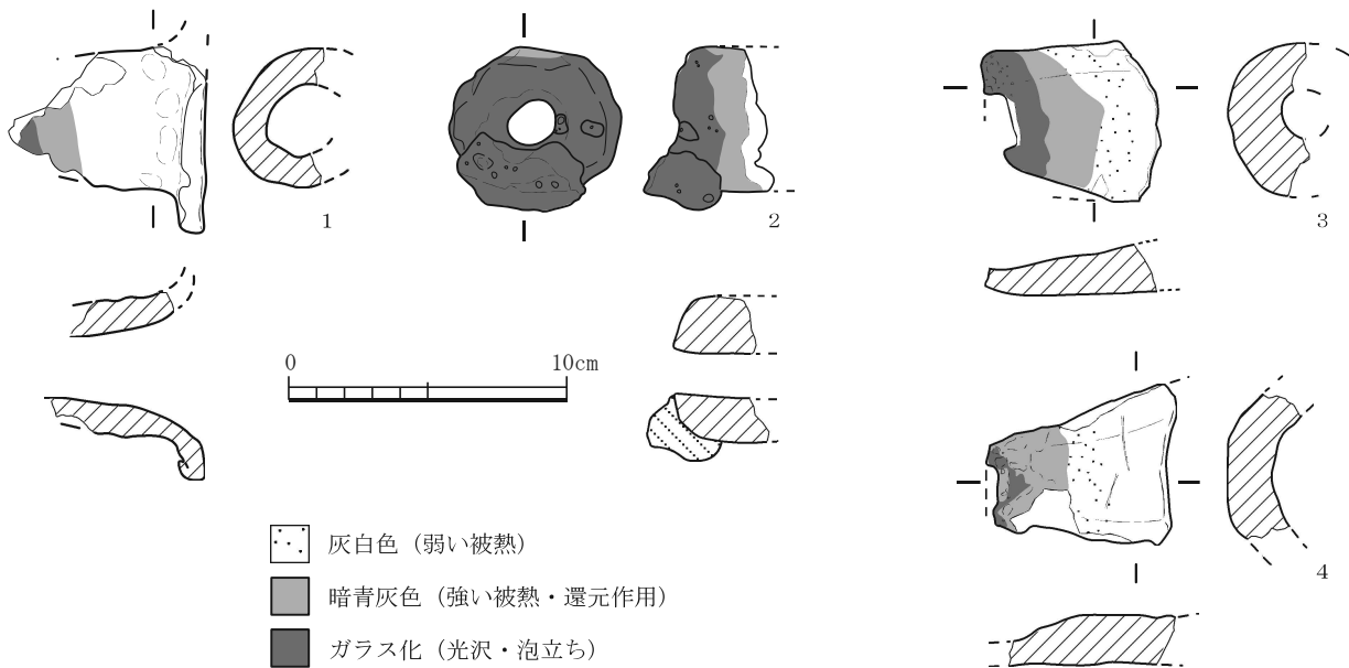
第4図 六A遺跡出土の鍛冶関連遺物 (S=1/3)
