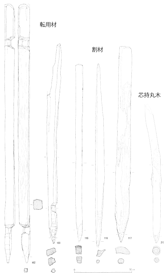
第 6 図 堰構築材の構成 (1:20)
