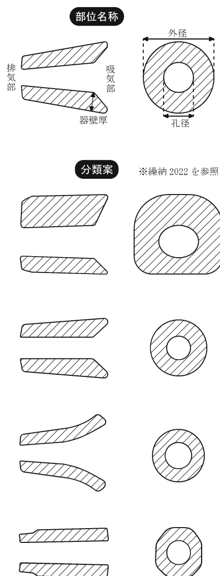
第 1 図 鞆羽口の部位名称と分類
