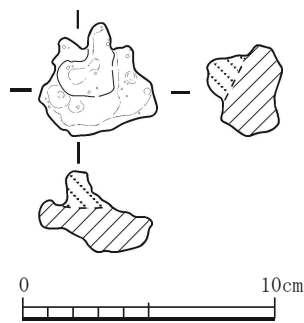
第6図 山室遺跡出土の鉄滓（S = 1 / 3）
