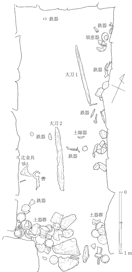
図8 石室内遺物出土状況図 1 : 30
