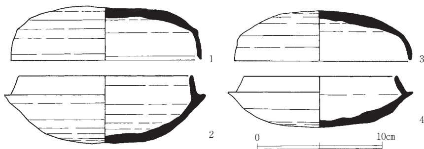
図10 舟塚古墳出土須恵器 1 : 3
