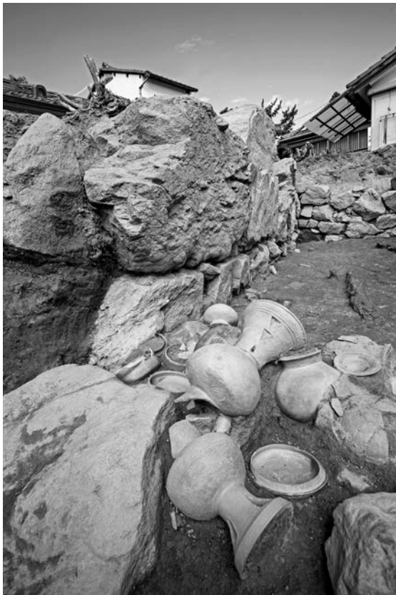
2 袖石付近土器出土状況（南東から）
