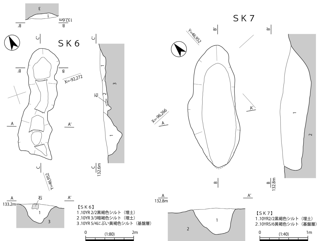
第11図 SK 6・7 平面図・土層断面図 (1:80・1:40)
