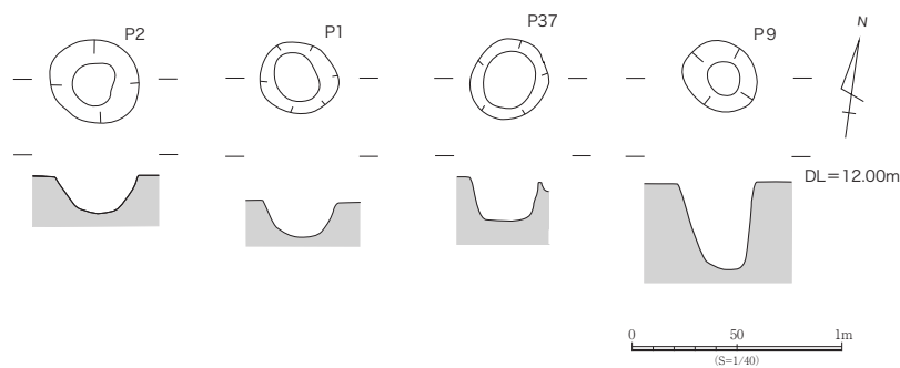
第12図 ピット列1 (SA1) 平面・エレベーション図(S=1/40)
