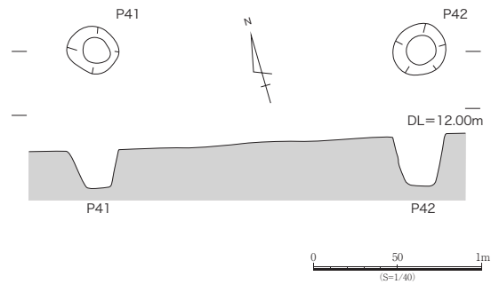
第16図 ピット列5 平面・エレベーション図(S=1/40)
