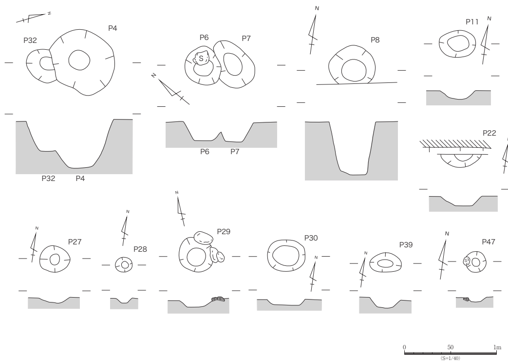
第17図 その他のピット 平面・エレベーション図(S=1/40)
