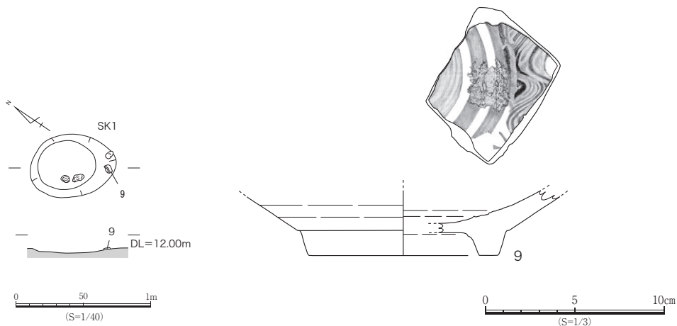
第21図 SK1 平面・エレベーション図(S=1/40) 出土遺物実測図(S=1/3)
