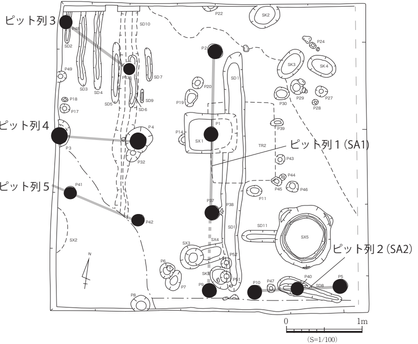
第11図 ピット列1～5 平面図(S=1/100)
