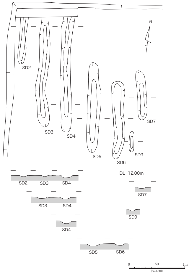
第24図 SD2~7・9 平面・エレベーション図 (S=1/40)
