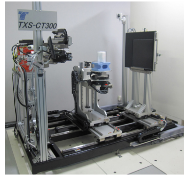
X線CT撮影装置
