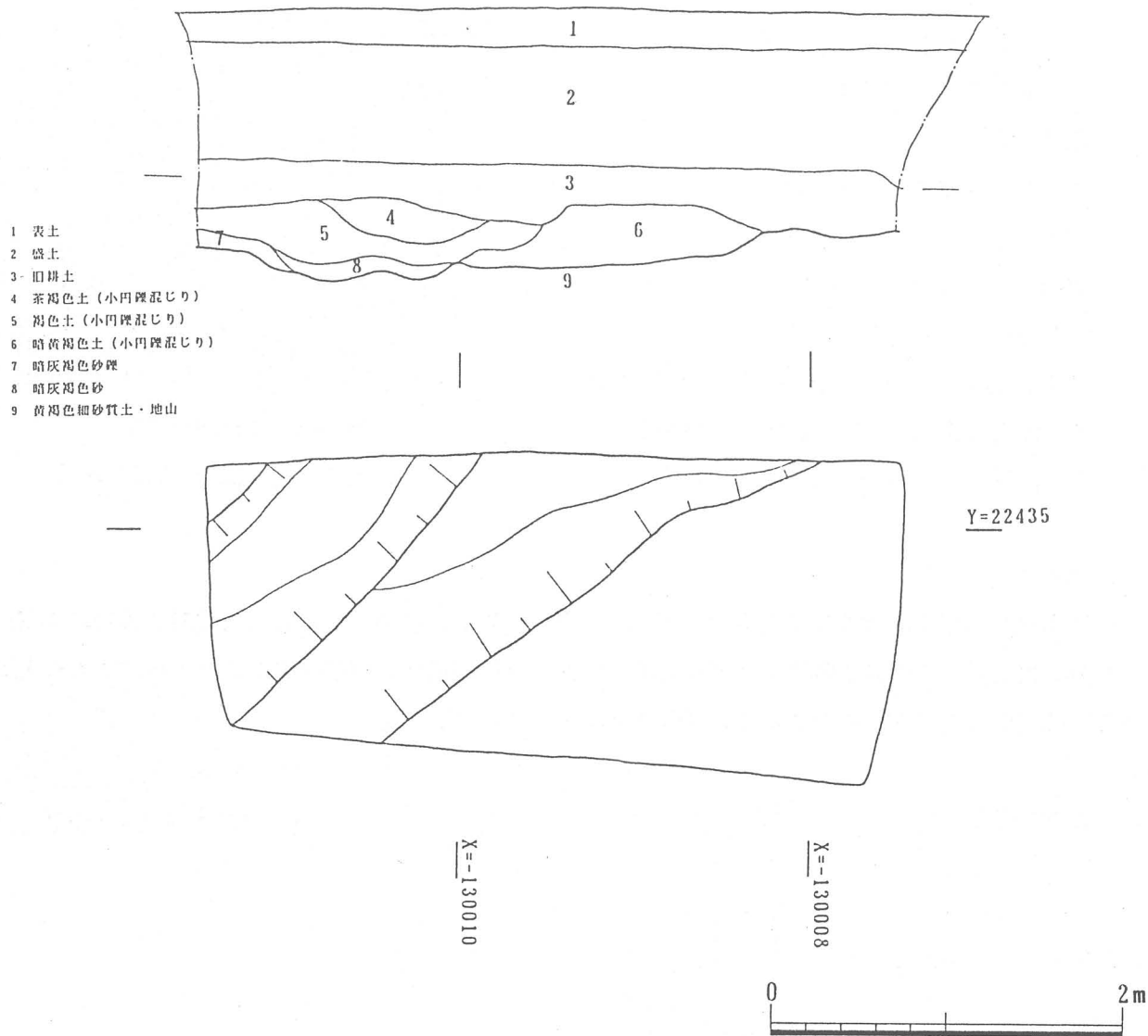
第3図 No. 3 トレンチ実測図
