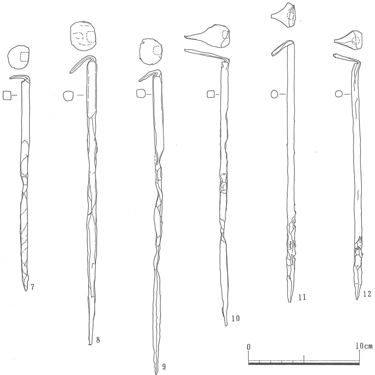
瓦釘実測図 (2)
