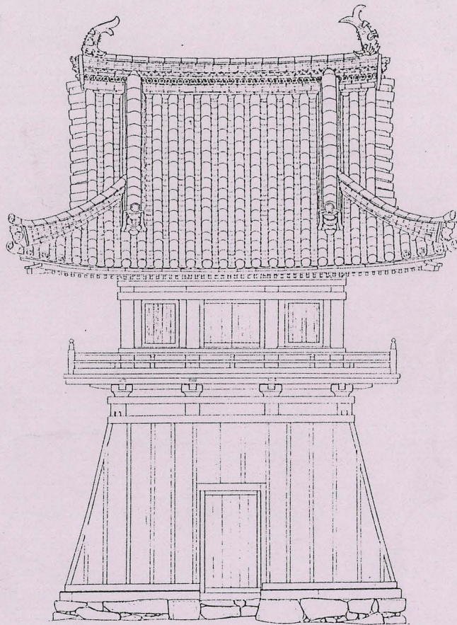
斑鳩寺鐘楼 (西立面図)
