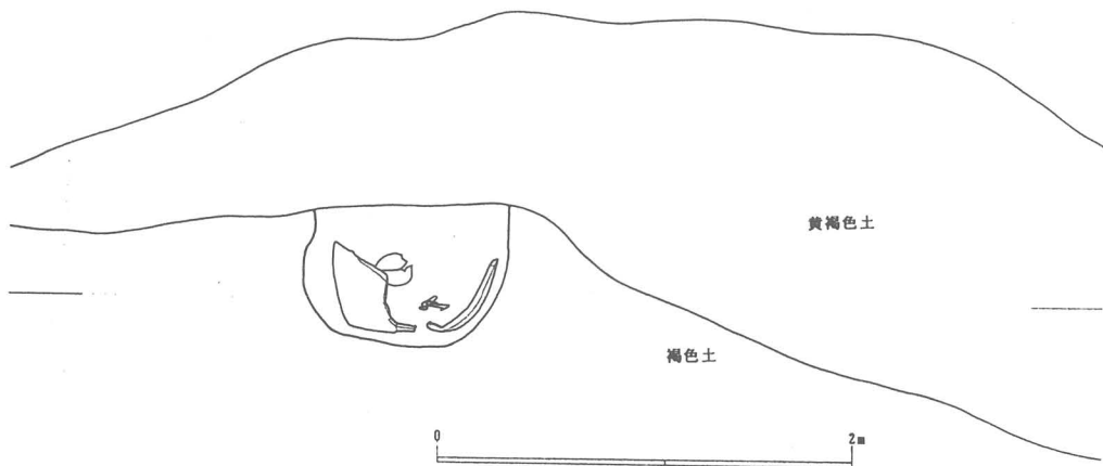
第2図 甕棺遺構断面実測図 (1:40)
