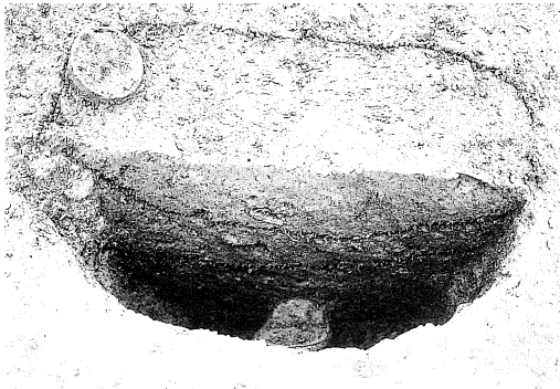
第27号住居跡貯蔵穴
