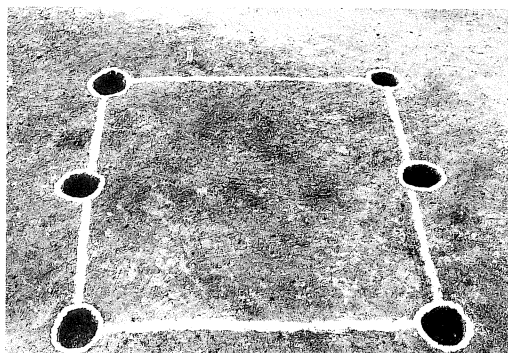
第8号掘立柱建物跡
