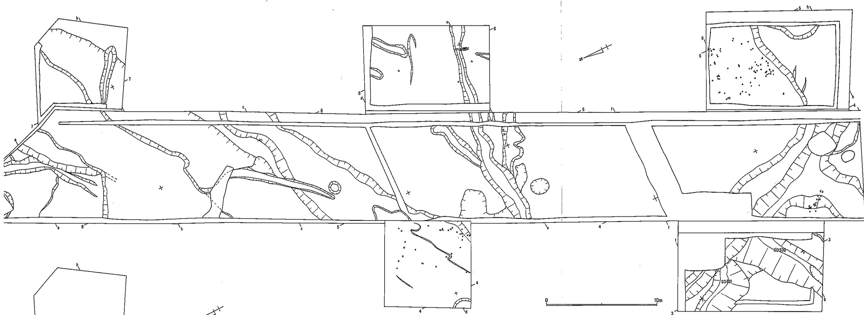
fig. 68 H区第5遺構面b 平面図
