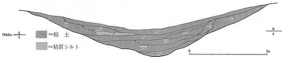
fig.37 H 5 グリッド第6 遺構面 a 下 周溝 S D530土層断面 及び下層土器出土状況図 (Sec. B)
