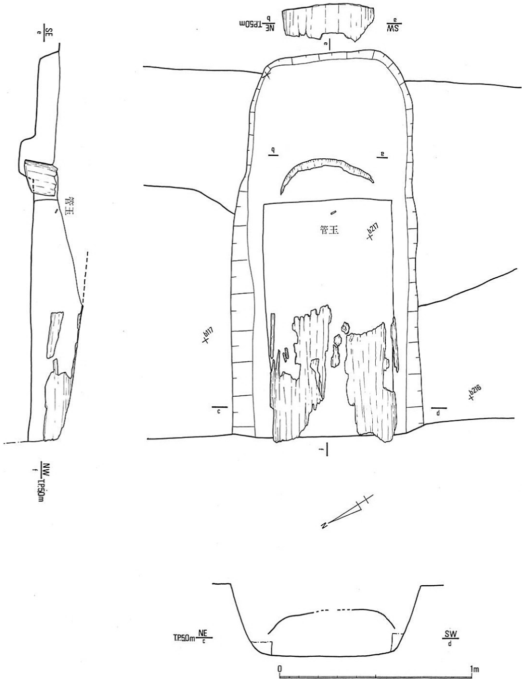
fig. 65 F 2 グリッド第 5 遺構面 b 土墳墓 S K202 平面、土層断面図
