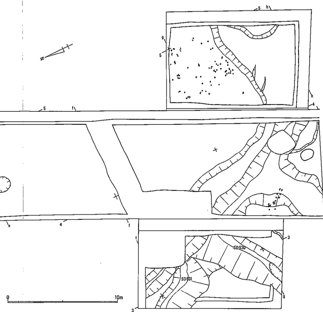
fig. 68 H区第5遺構面b 平面図
