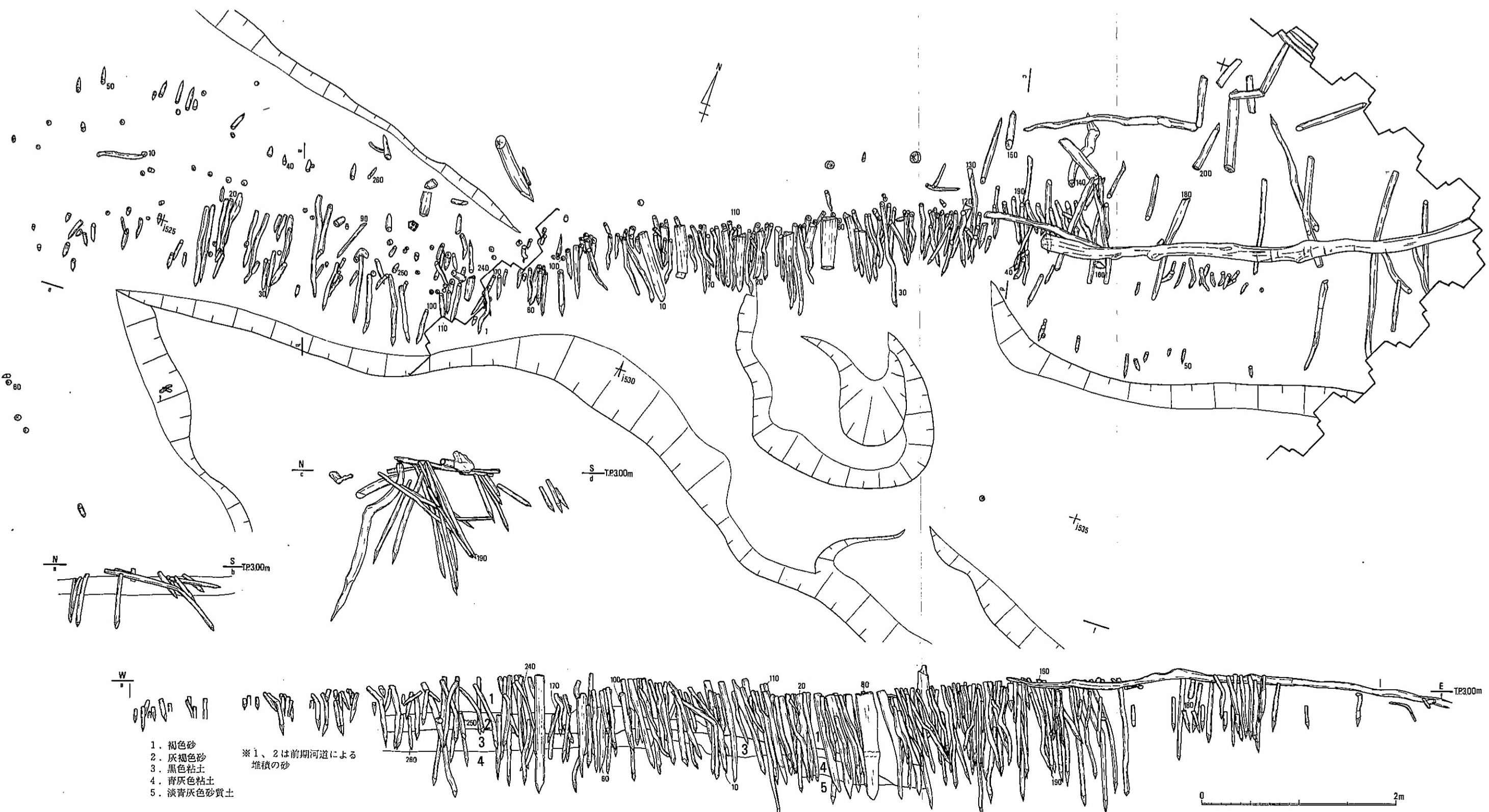
fig. 45 I区第6遺構面d シガラミ205平面、立面図
