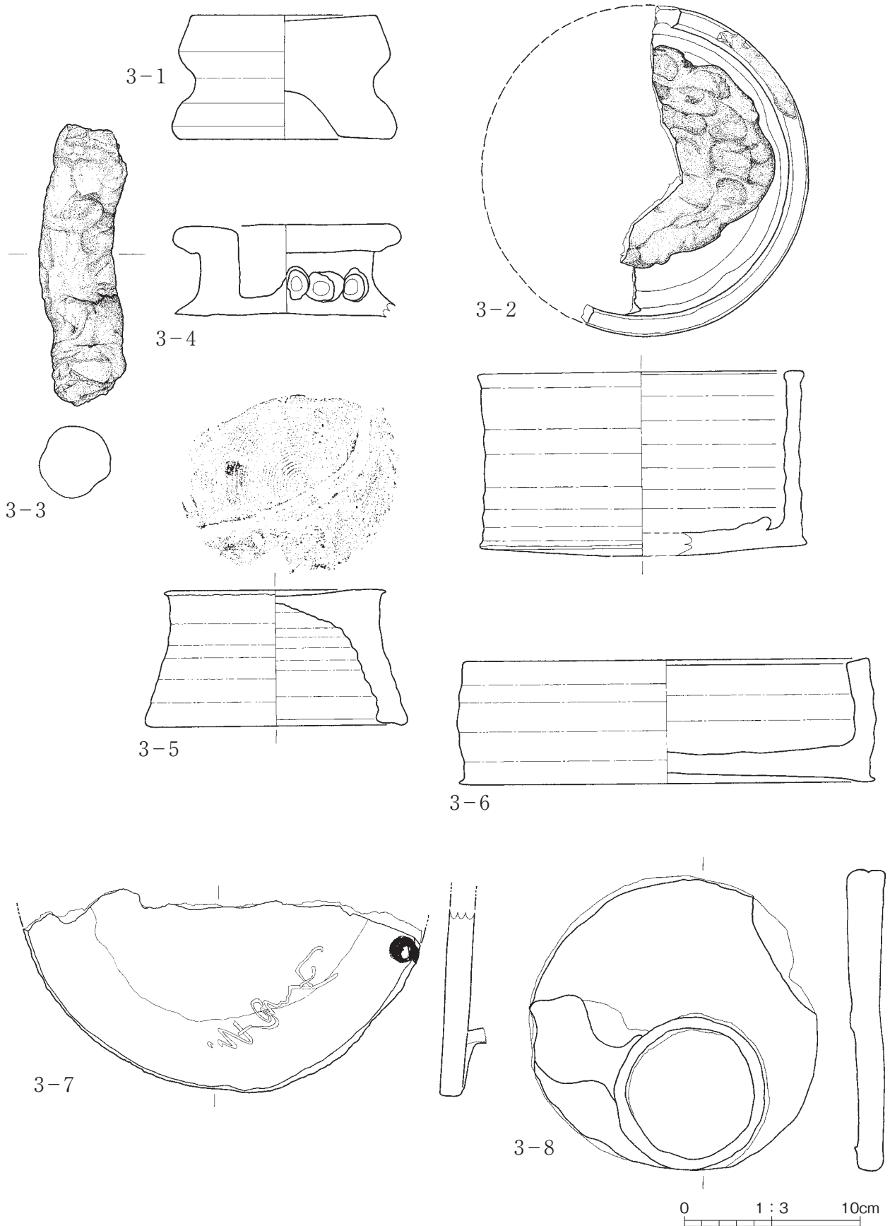
第9図 窯道具類 実測図
