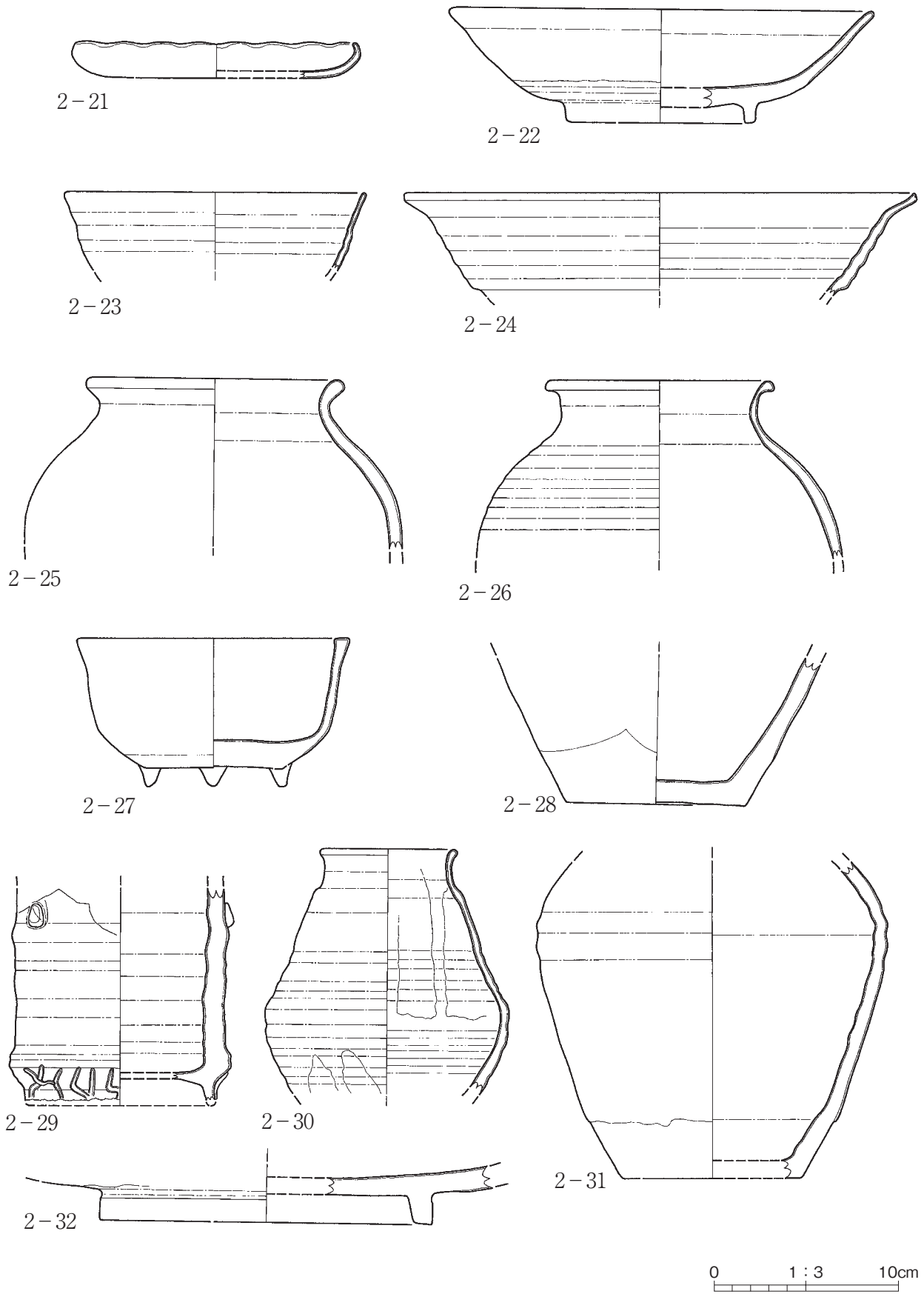
第7図 陶器 実測図
