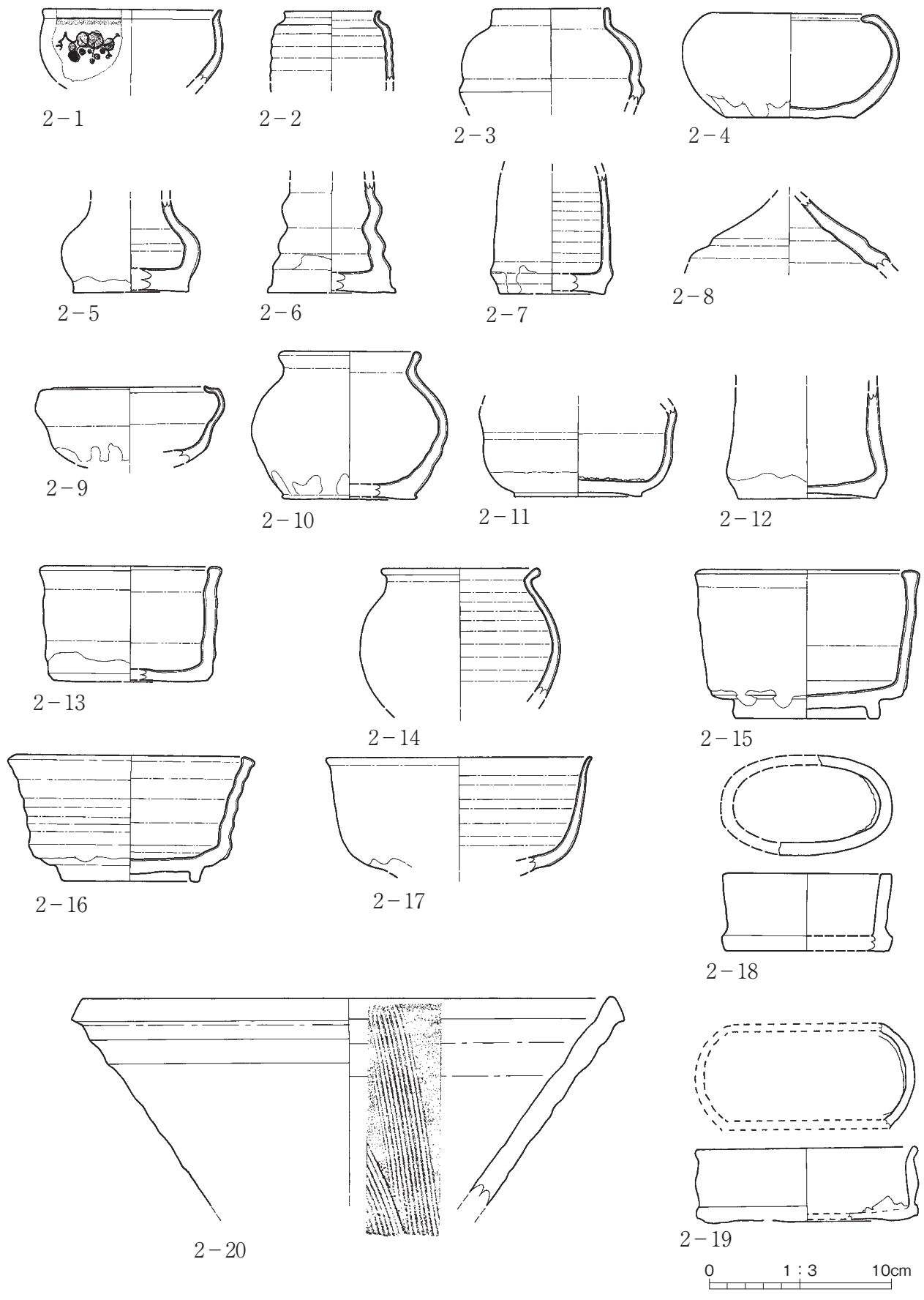
第6図 陶器 実測図
