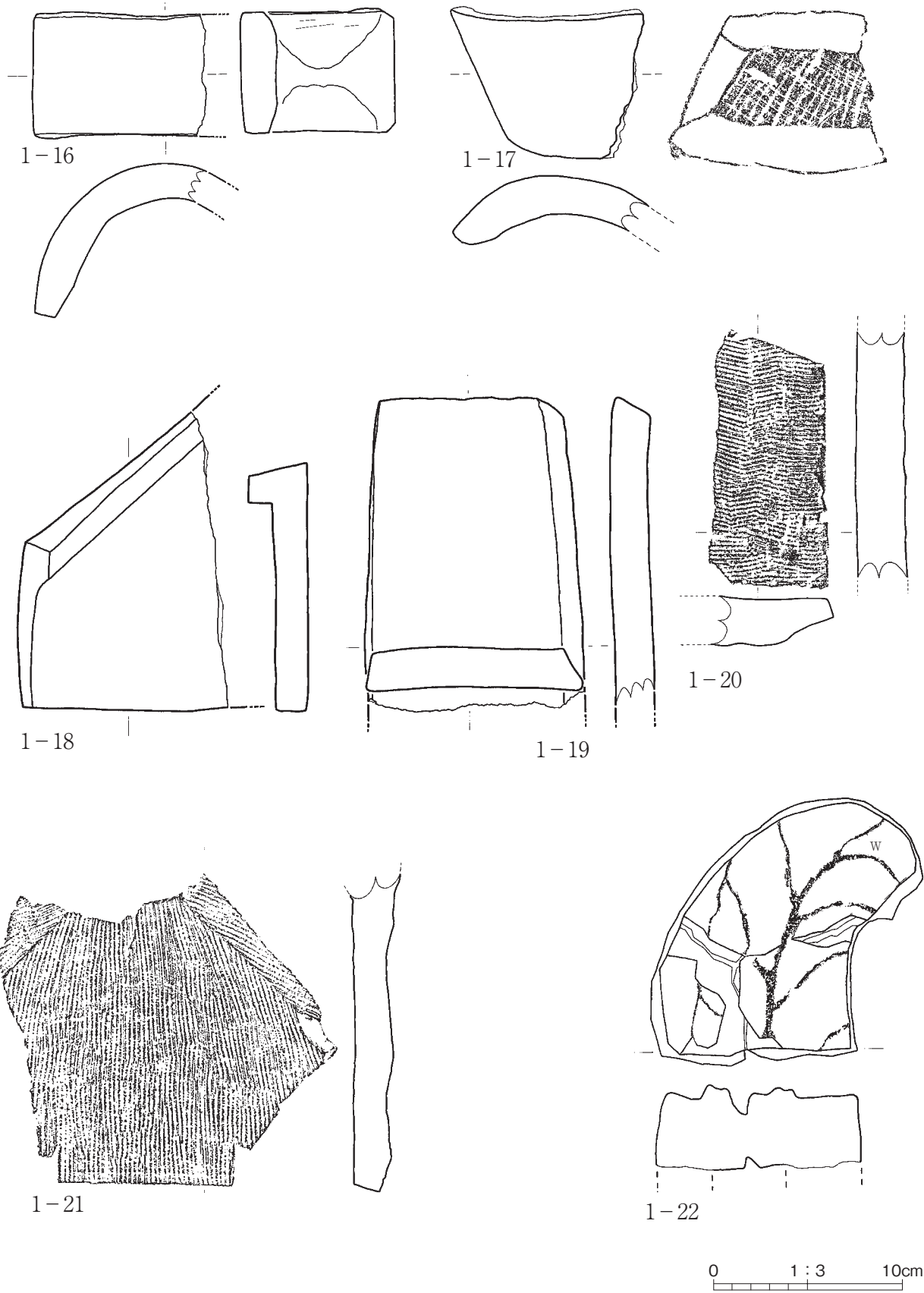
第5図 瓦 実測図
