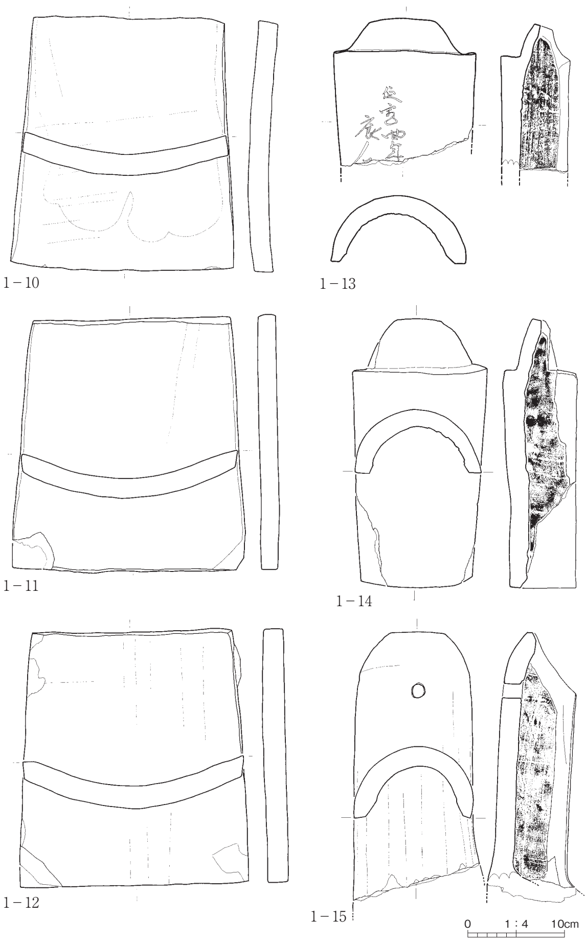
第4図 瓦 実測図
