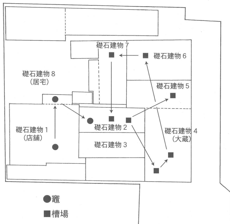
第187図 酒蔵遺構の変換（昭和2年酒蔵図面）
