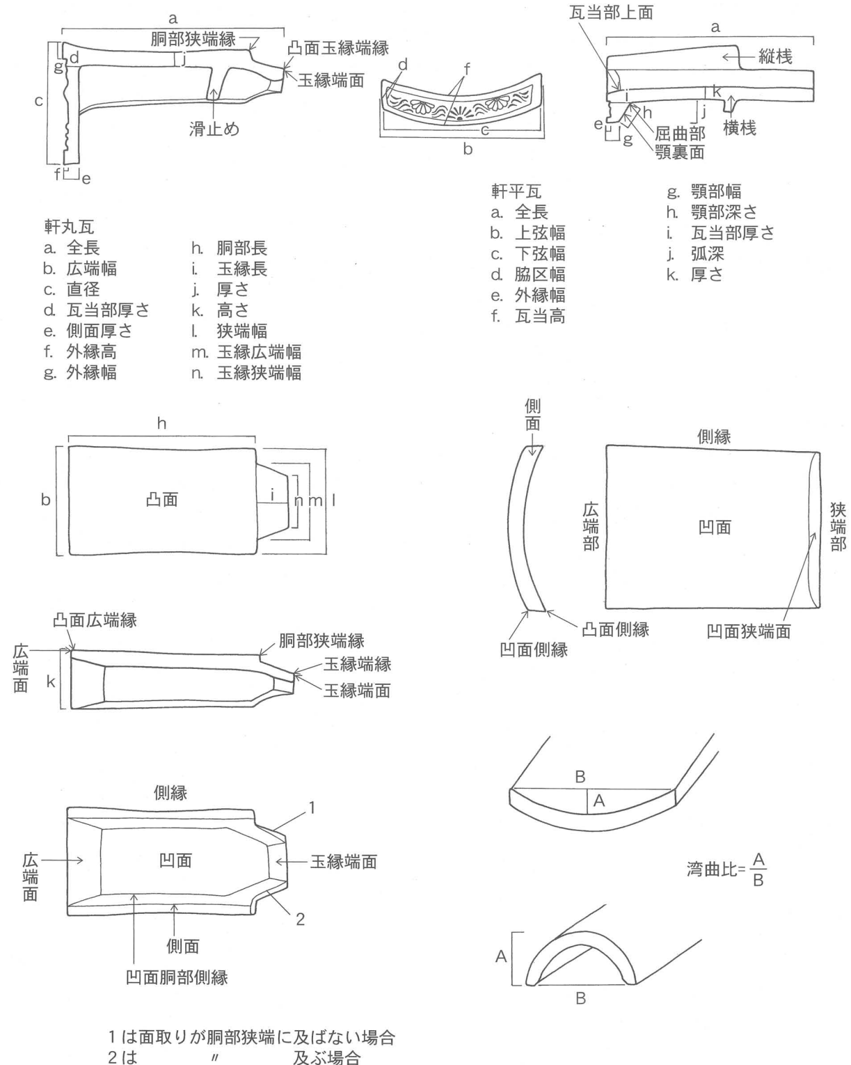
第164図 瓦の部位名称
