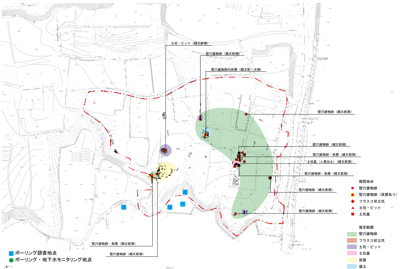
図 95 地下水観測地点配置図 (S=1/4000)
