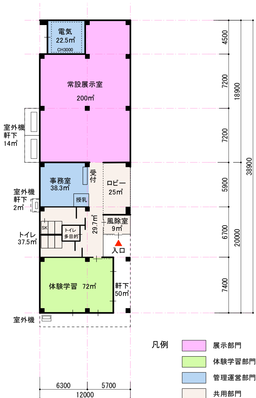
図 91 ガイダンス施設平面図 S=1/300
