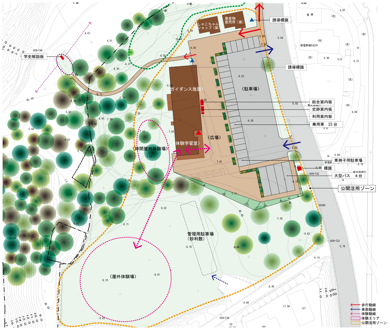
図 90 公開活用ゾーン配置図 S=1/1000
