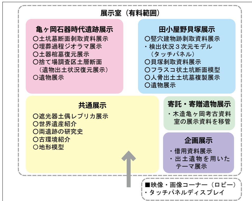
図 93 展示概念図
