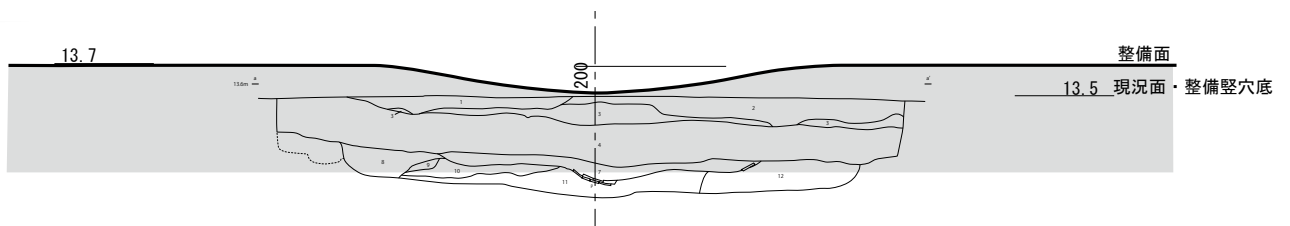
図 78 36号（竪穴建物跡）廃絶状況表示模式図 S=1/60
