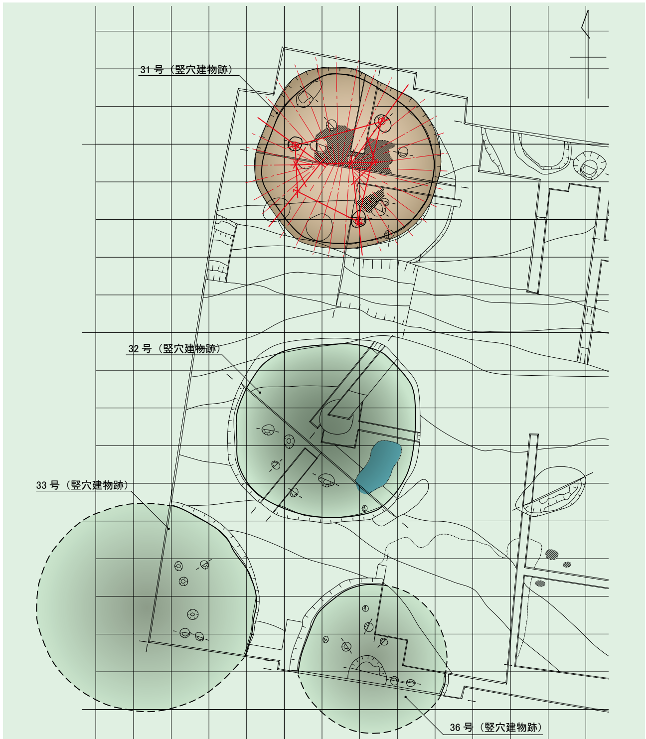
図 75 遺構配置・計画配置図 S=1/100
