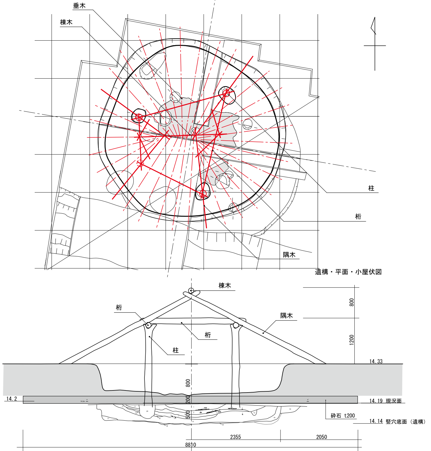
東西セクション結合・断面図 ※周堤の有無・出入口については今後検討する
