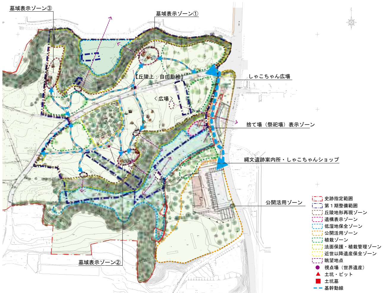
図 56 動線計画図(S=1/3000)
