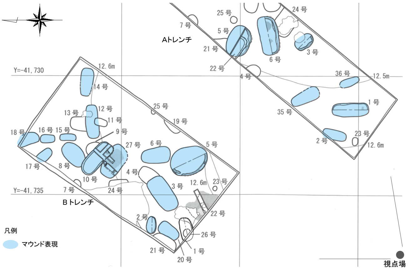
図 60 墓域表示ゾーン①現地整備 遺構配置図 S=1/100
