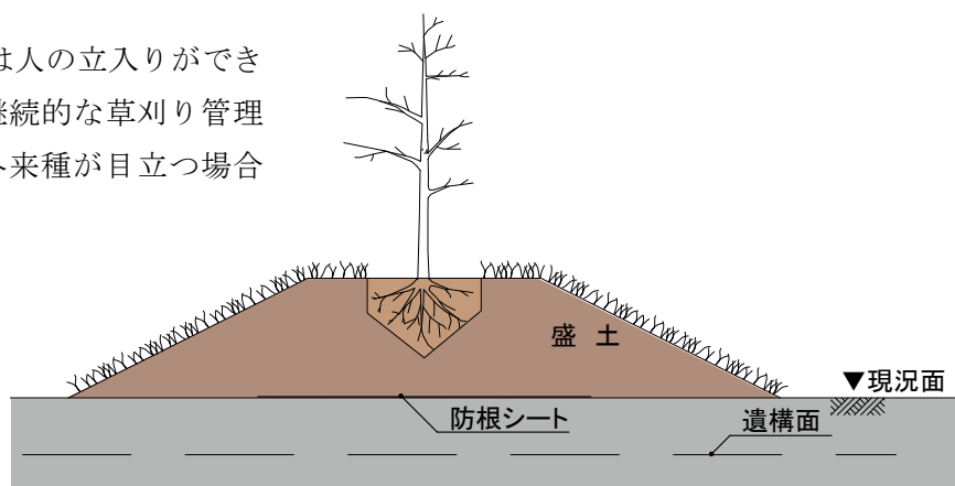
図 69 植栽整備模式図 S=1/30 (上：遺構の存在が想定されない場合・下：遺構の存在が想定される場合)
