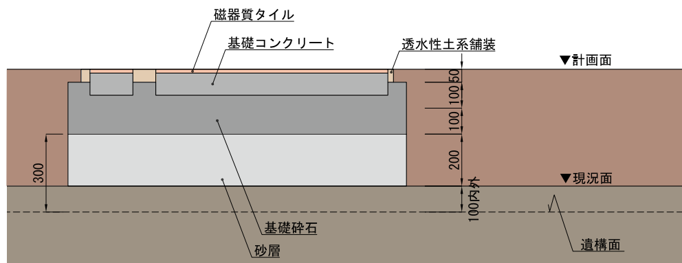
断面図
