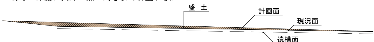
図 57 敷地造成模式図(S=1/200)
