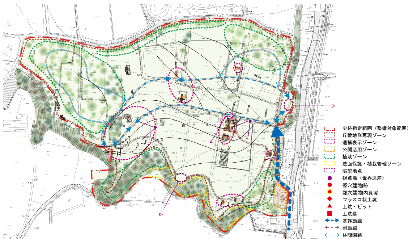
図 72 動線計画図 (S=1/3000)
