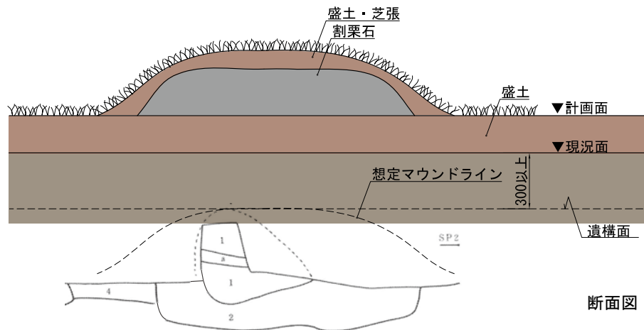
図 62 遺構表示模式図（土坑墓マウンド表現） S=1/30
