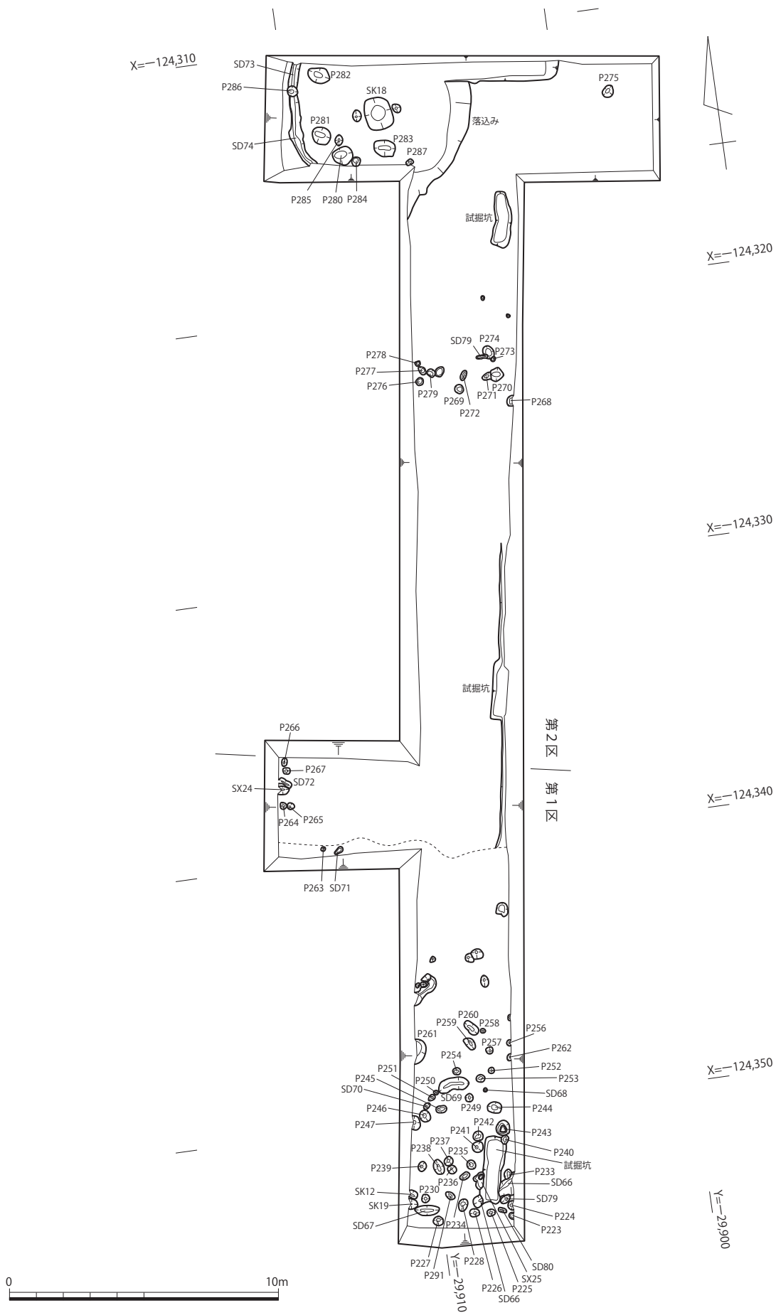
第7図 第3遺構面平面図 (1/200)
