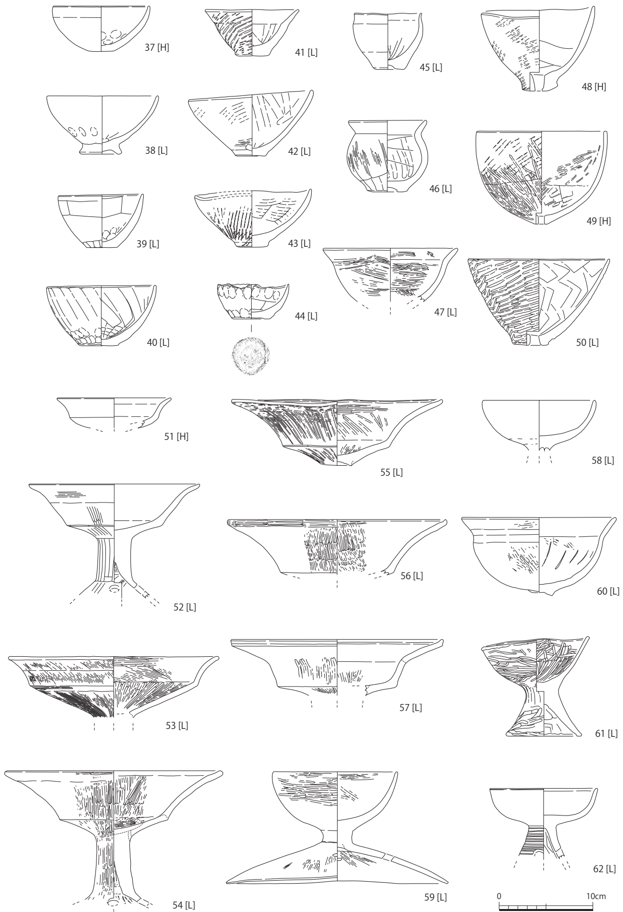
图21 S005地凹出土土器 (3) (1:4)
