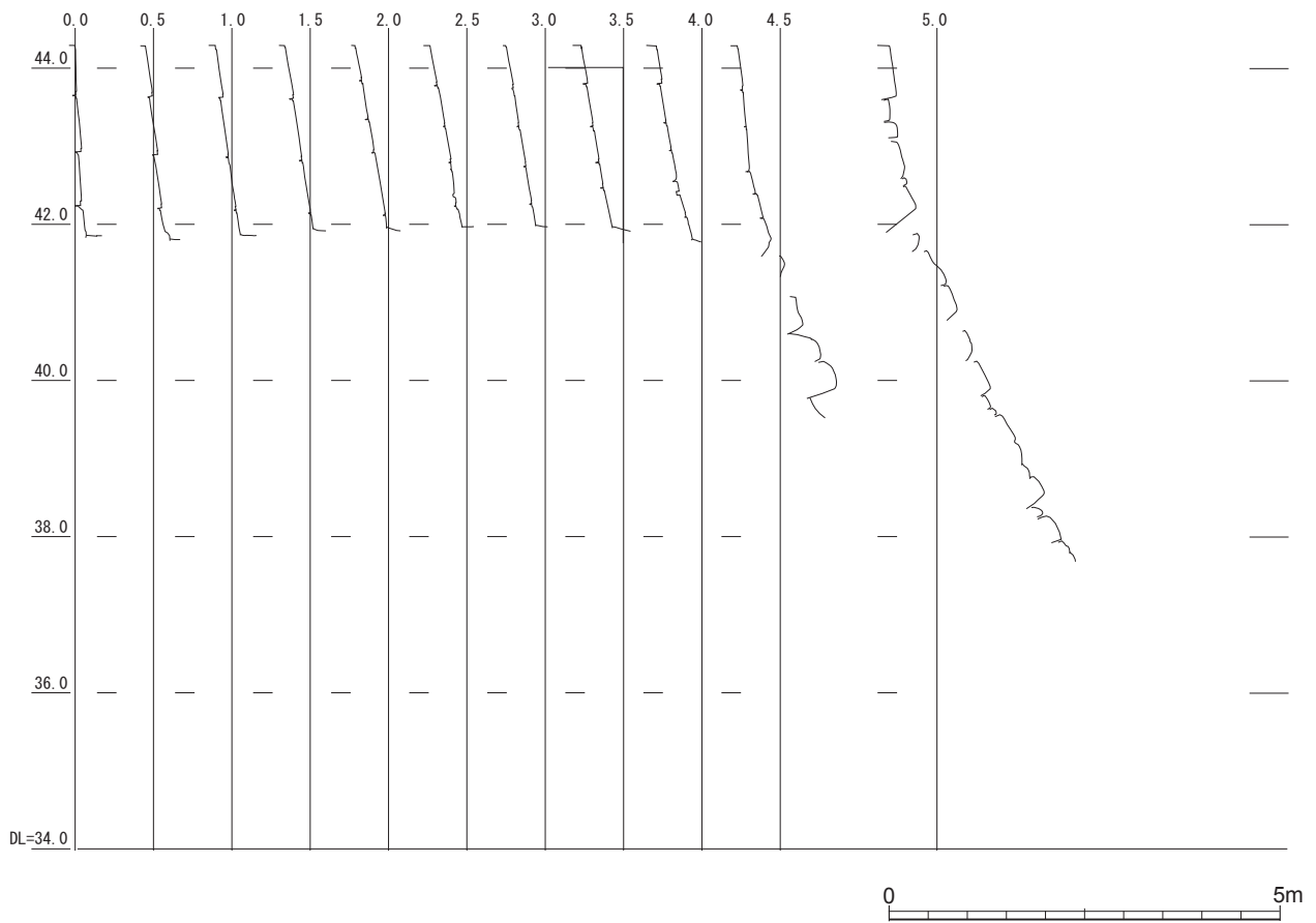
第 56 図 遺構図版 ニラミ櫓台北面 (ID3500N) 垂直断面図 1 (S=1/100)
