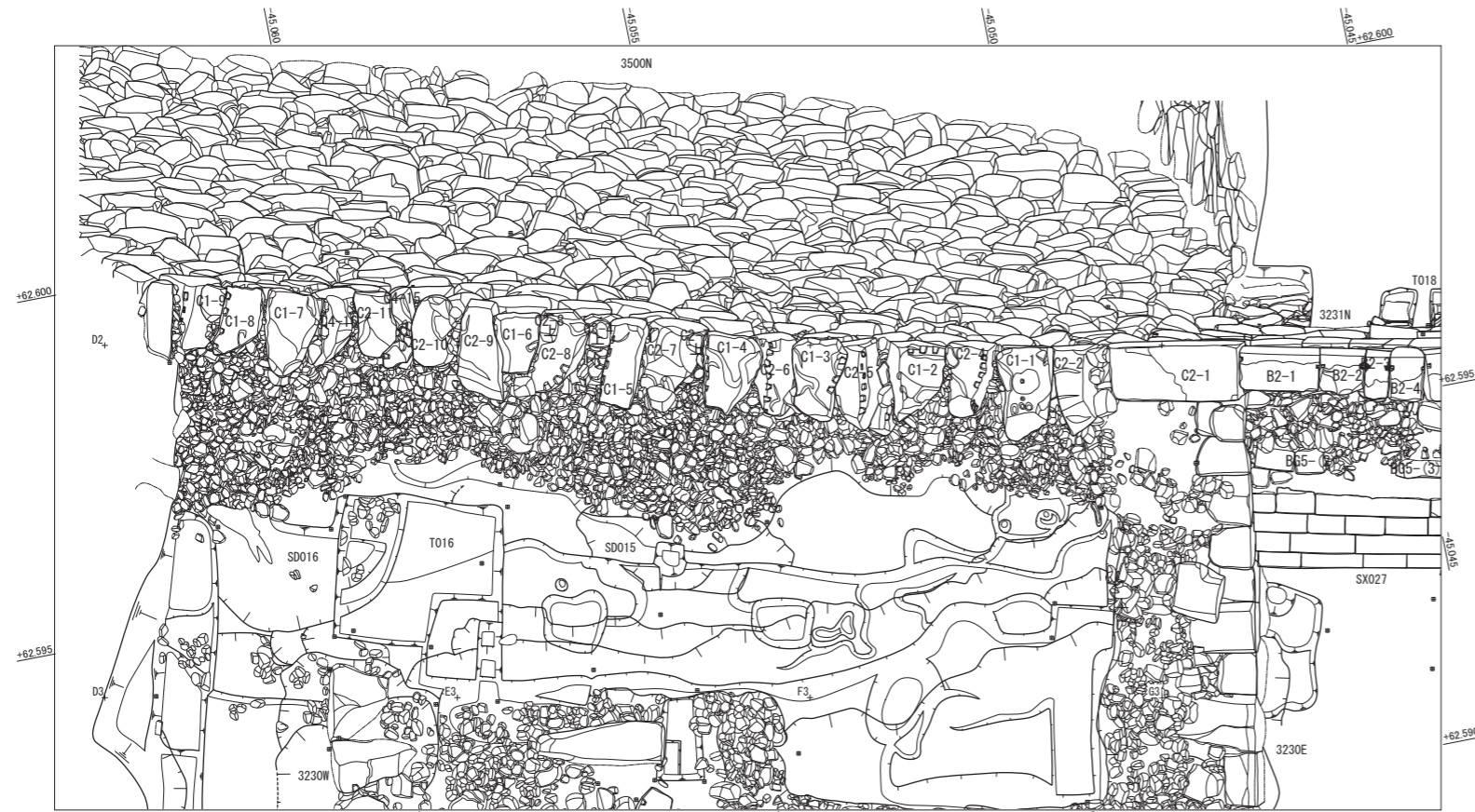
C1段 平面图
