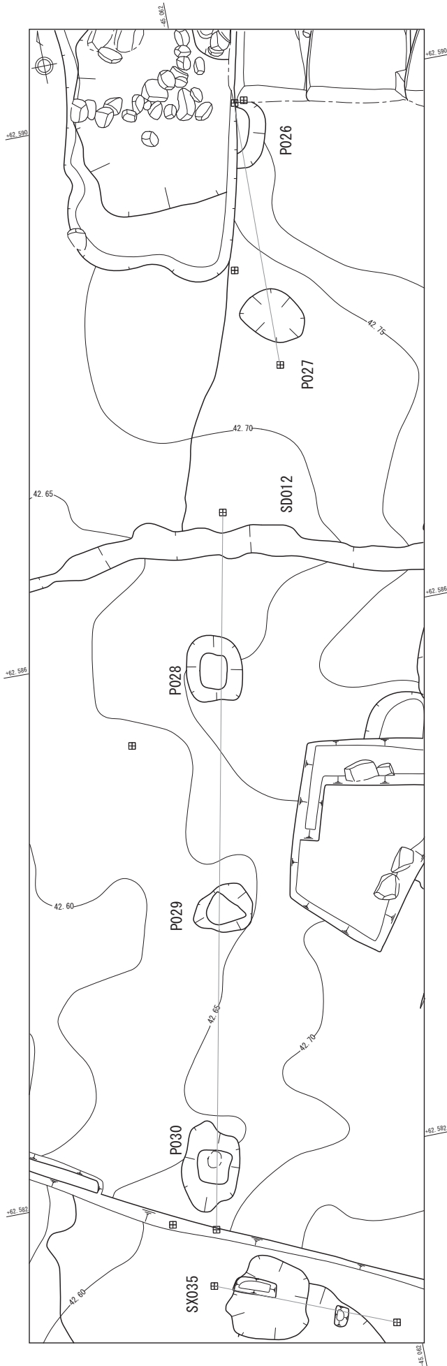
3-4-30 ~ 32 SX035・P026 ~ P030 平面図 (1/40)
