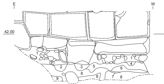
3-2-03 3241N 立面図・断面図 (1/40)
