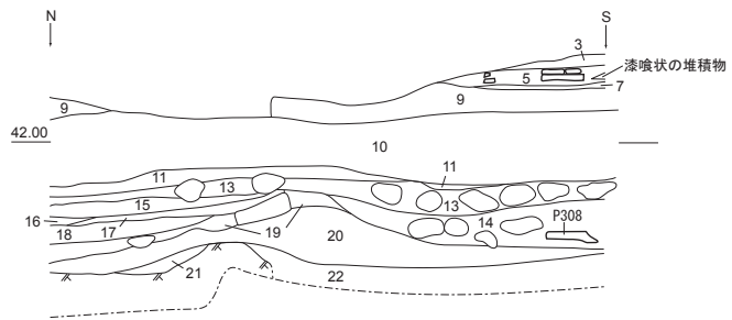
3-4-03 SD214-2 東壁 断面図③(1/30)
