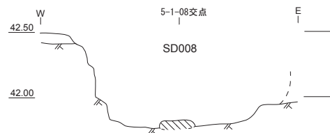
5-1-11 SD008 エレベーション④(1/40)
