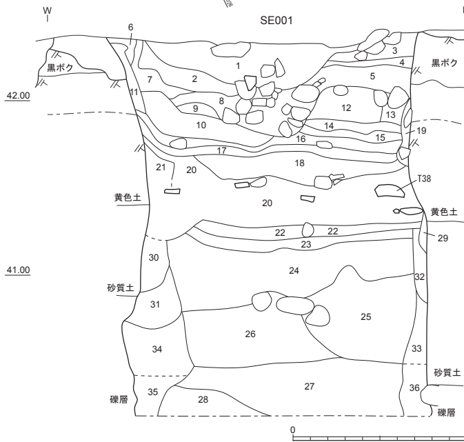
5-1-16 SE001 平面図・断面図 (1/30)
