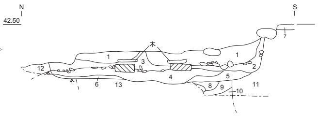
3-1-09 F7 南北断面図 (1/40)
