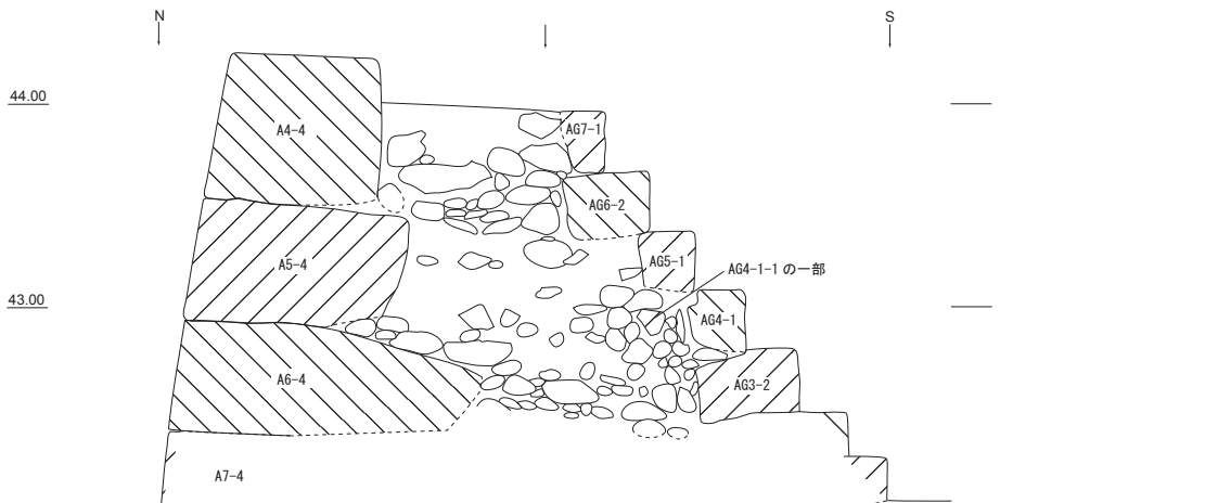
4-1-04 3241 南北断面図 (1/40)
