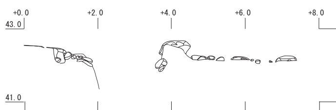
ID 3210W (二ノ門南側石垣台西面) 立面図
