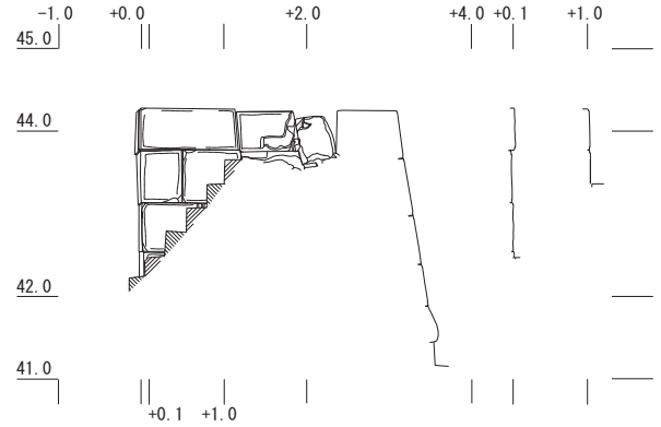
ID 3241E (一ノ門東側類当石垣東面) 立面・垂直断面図
