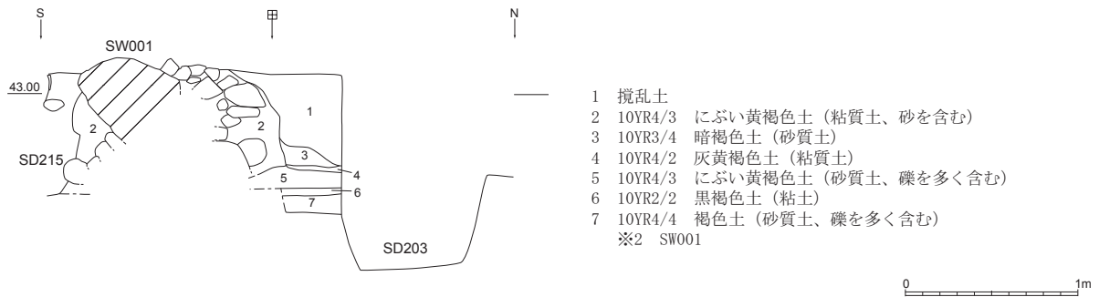
3-4-25 SW001 南北断面図 (1/40)
