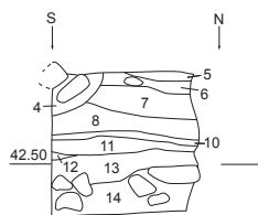
3-4-19 3220S 西壁 断面図 (1/20)
