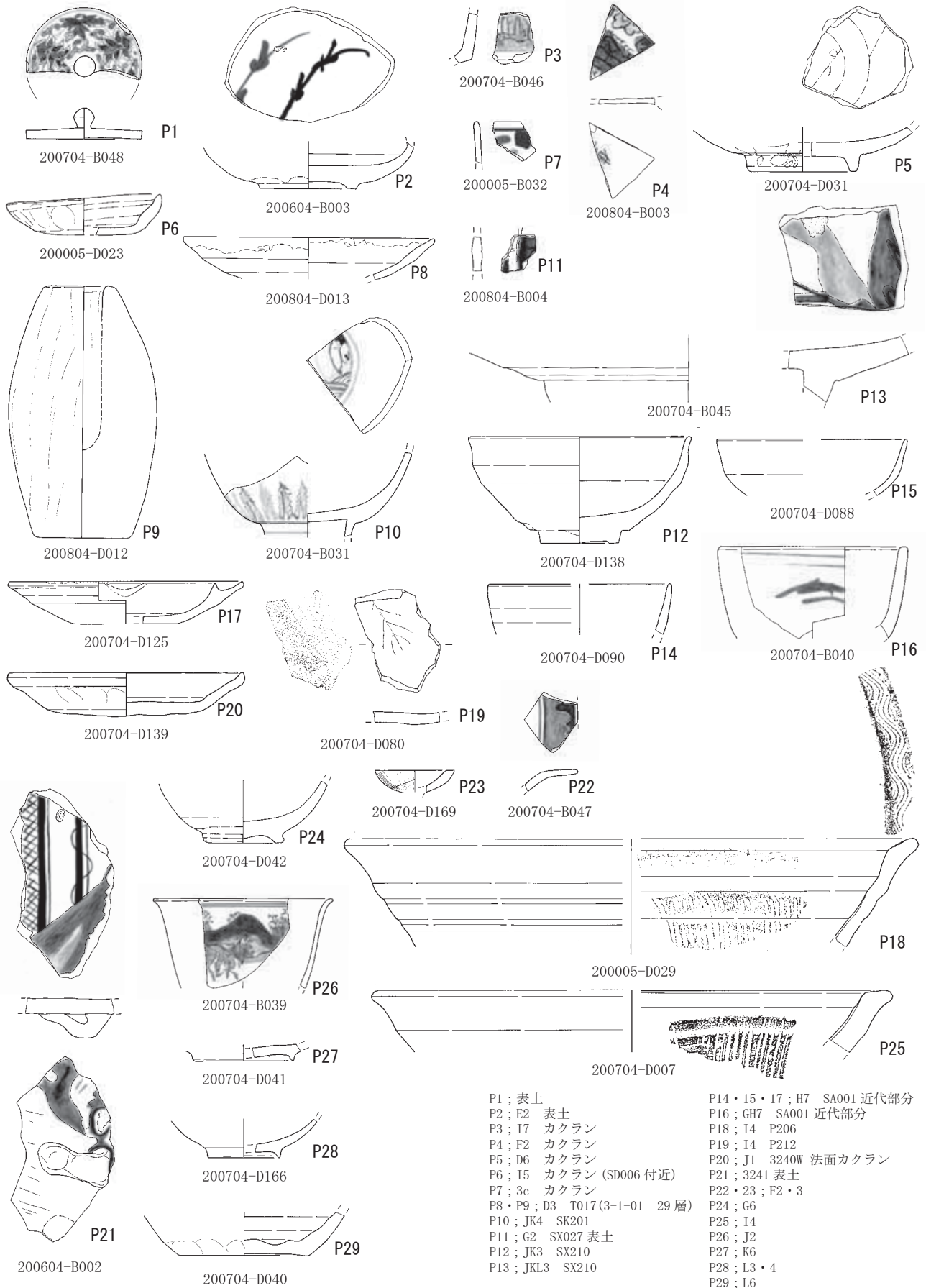
第 219 図 遺物実測図 陶磁器・土器 1 (S=1/3)
