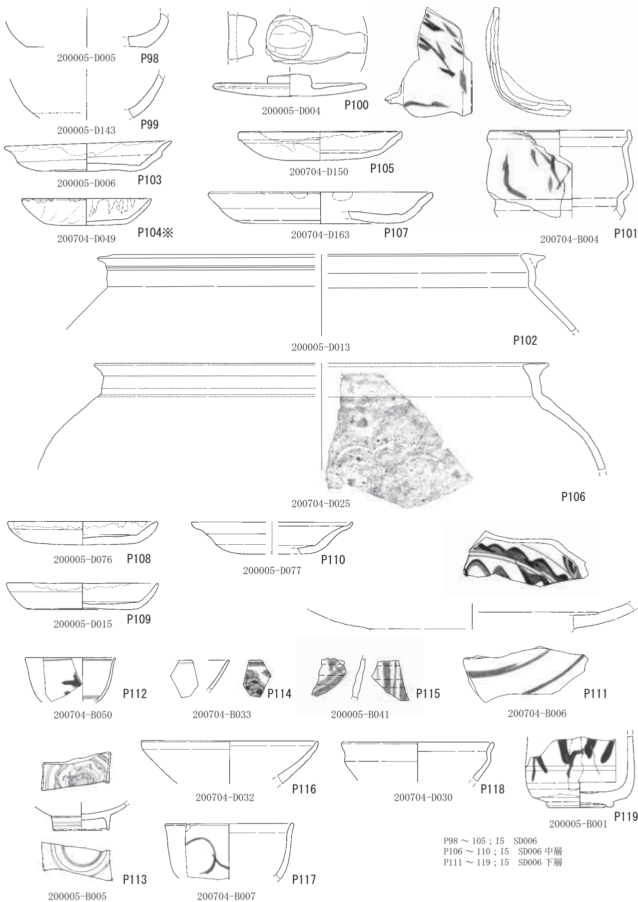
第 223 図 遺物実測図 陶磁器・土器 5 (S=1/3)
