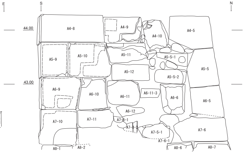
4-1-02 3241E 立面図・断面図 (1/40)
