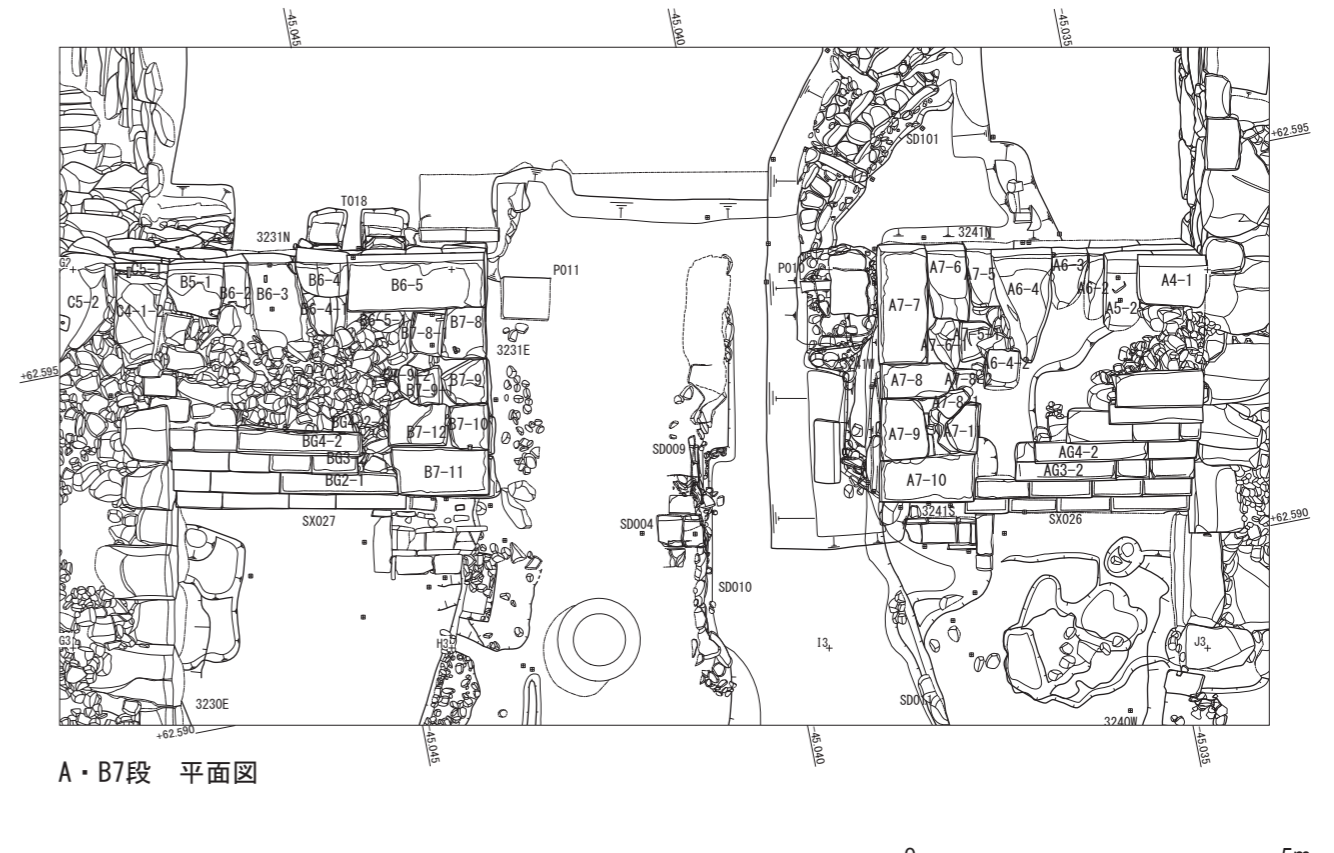
第77図 遺構図版 石垣解体測量図4 (S=1/100)
