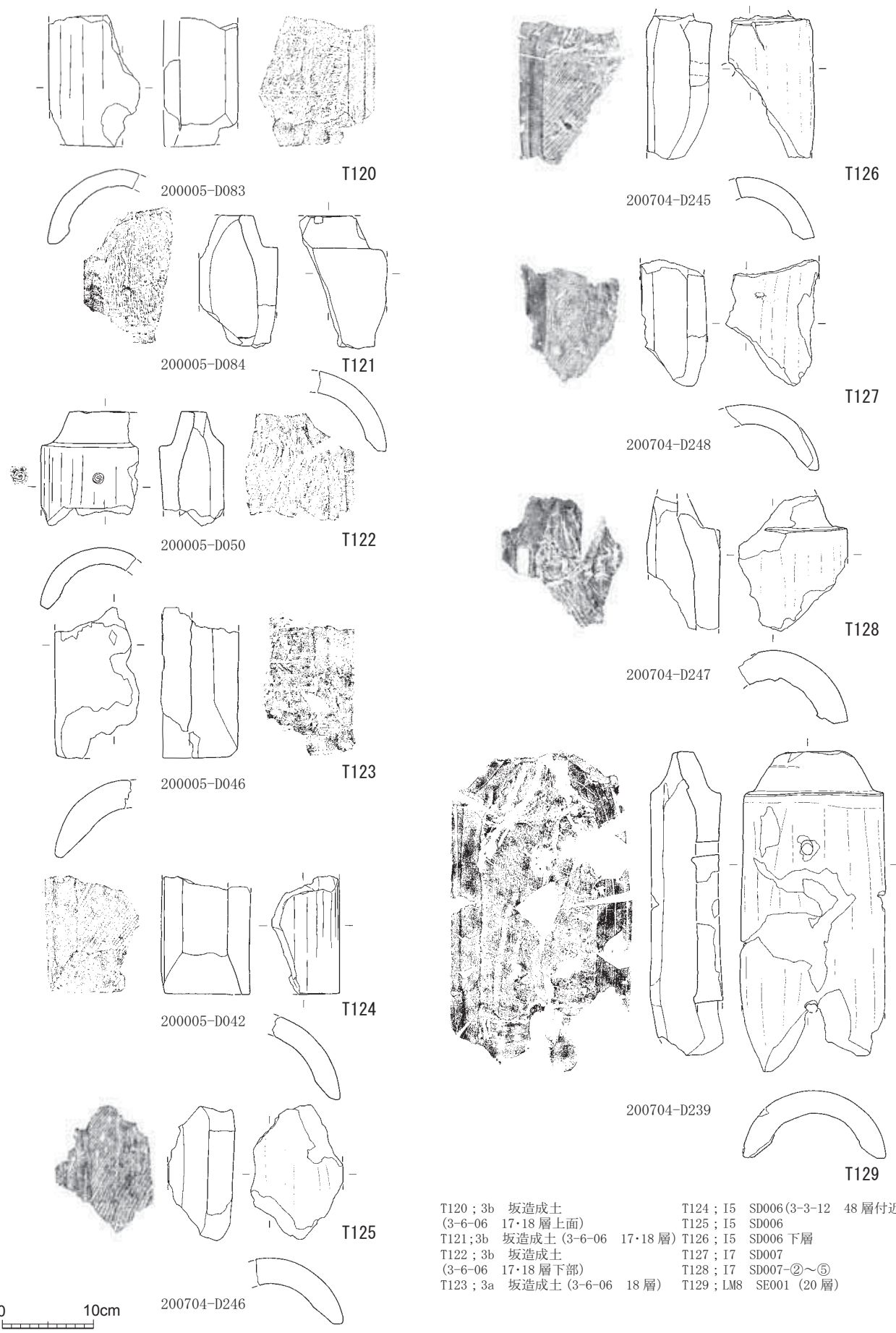
第 240 図 遺物実測図 瓦 10 (S=1/6)
