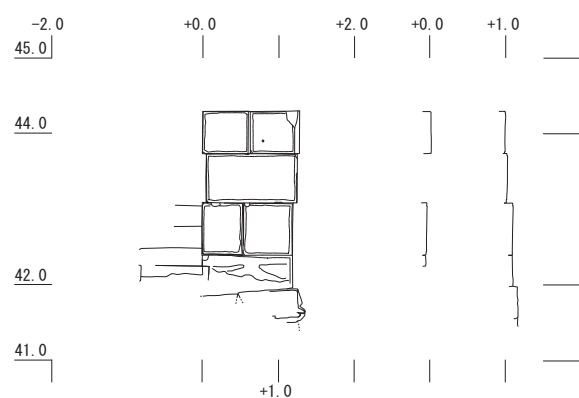
ID 3231S (一ノ門西側類当石垣南面) 立面図・垂直断面図
