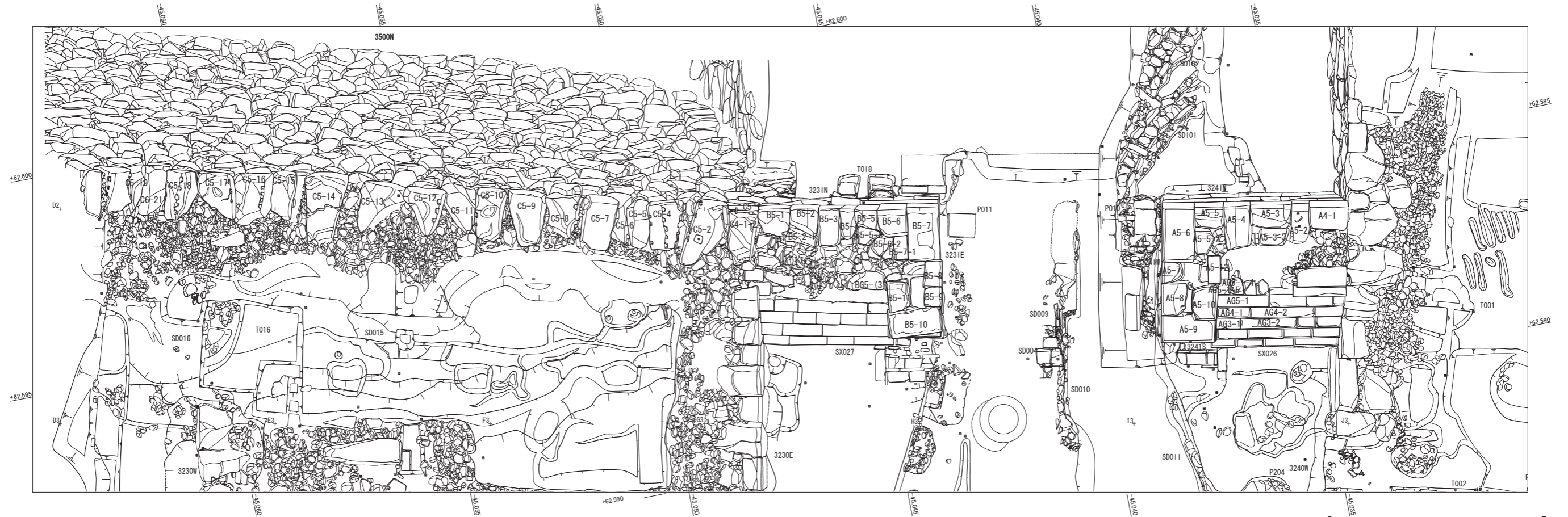
A5段下、B5段中、C5段 平面図
