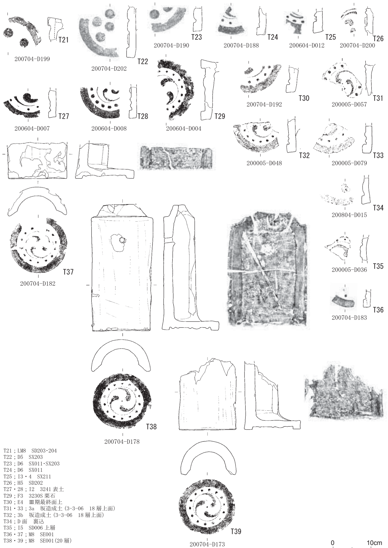
第 232 図 遺物実測図 瓦 2 (S=1/6)
