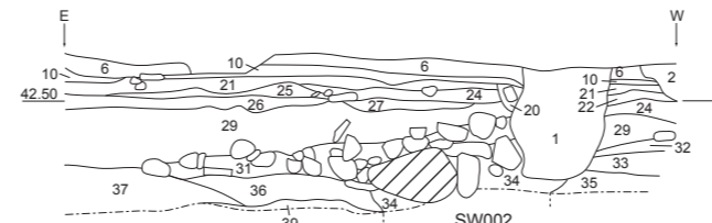
5-3-04 SD204-2 南壁 断面図 (1/30)
