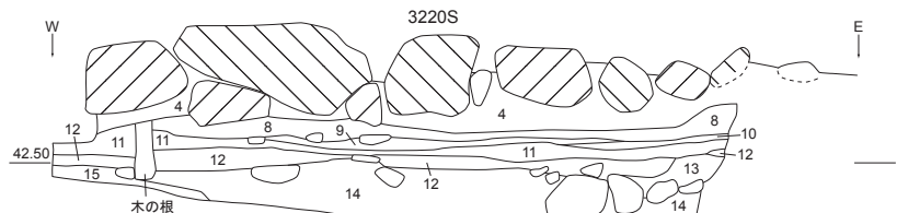
3-4-20 3220S 東西断面図②(1/20)
