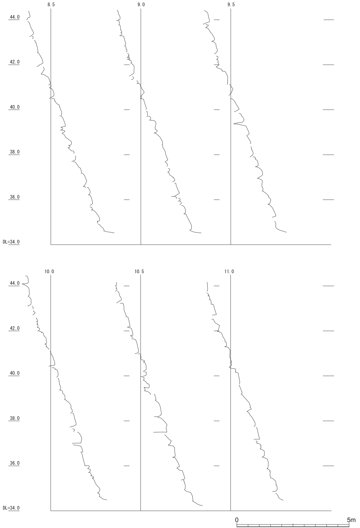
第 58 図 遺構図版 ニラミ櫓台石垣北面 (ID3500N) 垂直断面図 3 (S=1/100)
