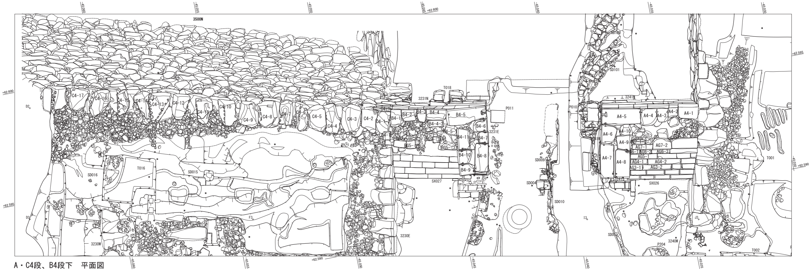
第75図 遺構図版 石垣解体測量図2 (S=1/100)
