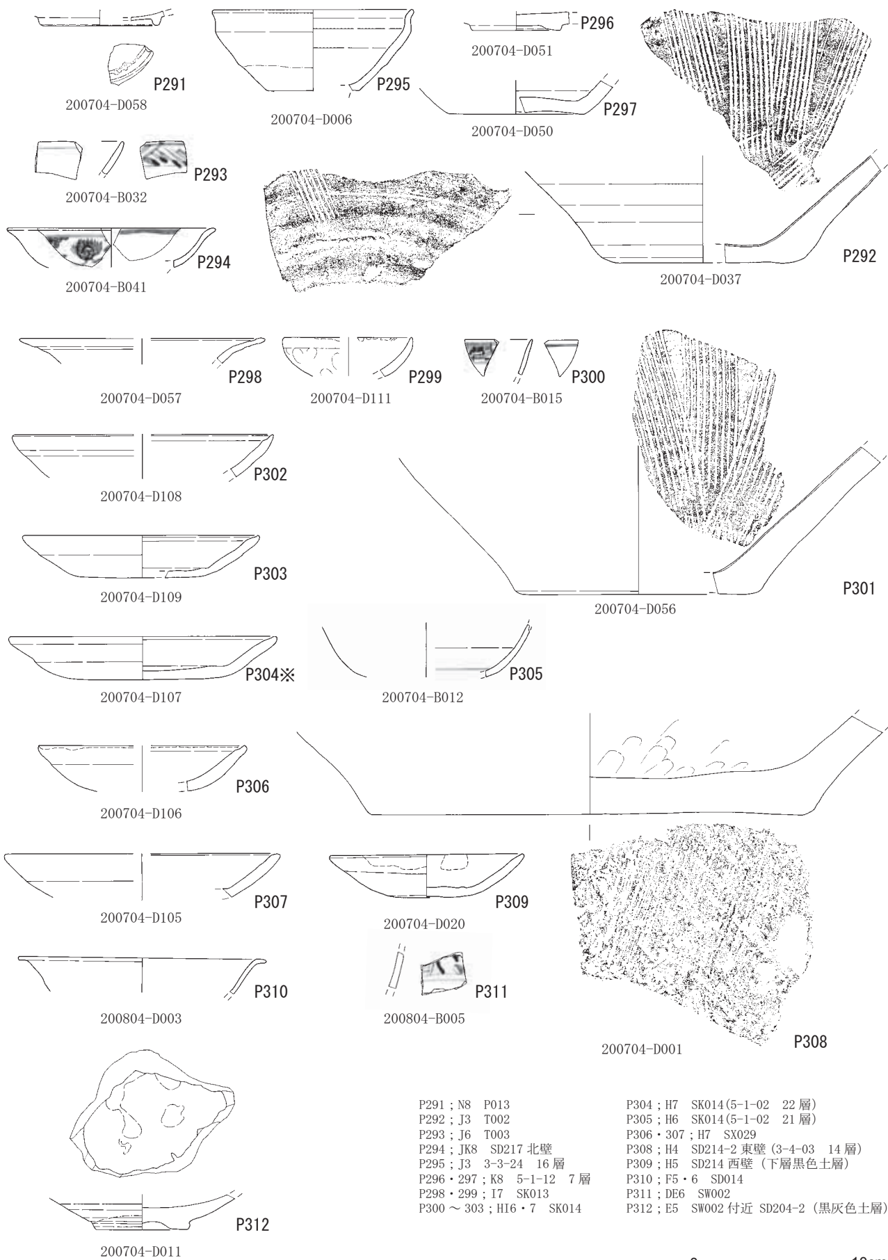
第230図 遺物実測図 陶磁器・土器 12(S=1/3)
