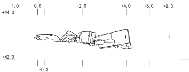
ID 3230W (ニラミ櫓台石垣西面) 立面図・垂直断面図
