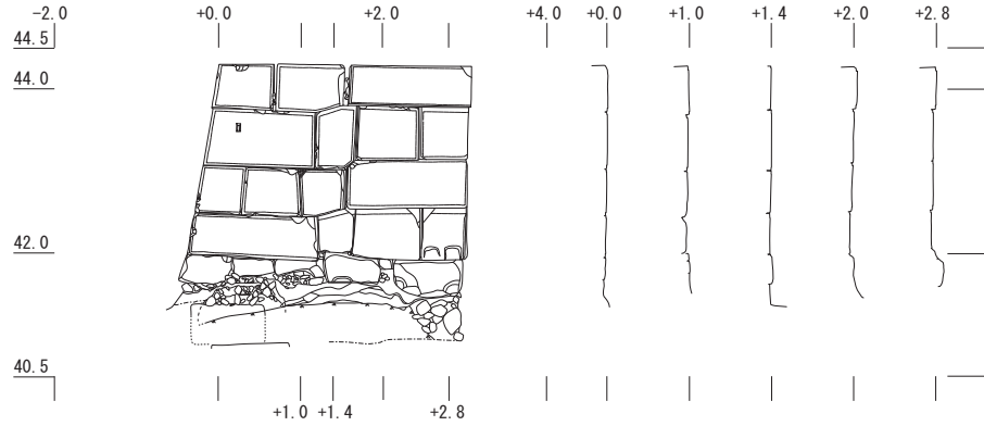
ID 3241S (東側類当石垣南面) 立面・垂直断面図
