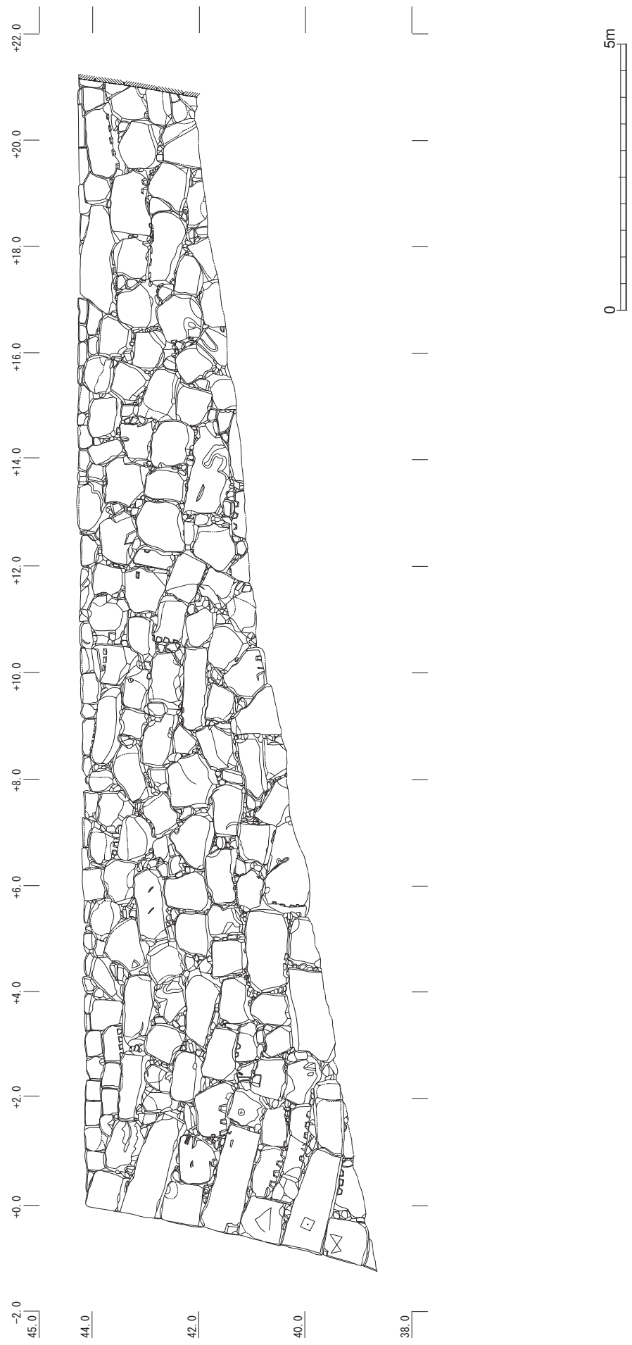
第 61 図 遺構図版 九十間長屋下石垣西面 (ID3440W) 立面図 (S=1/100)
