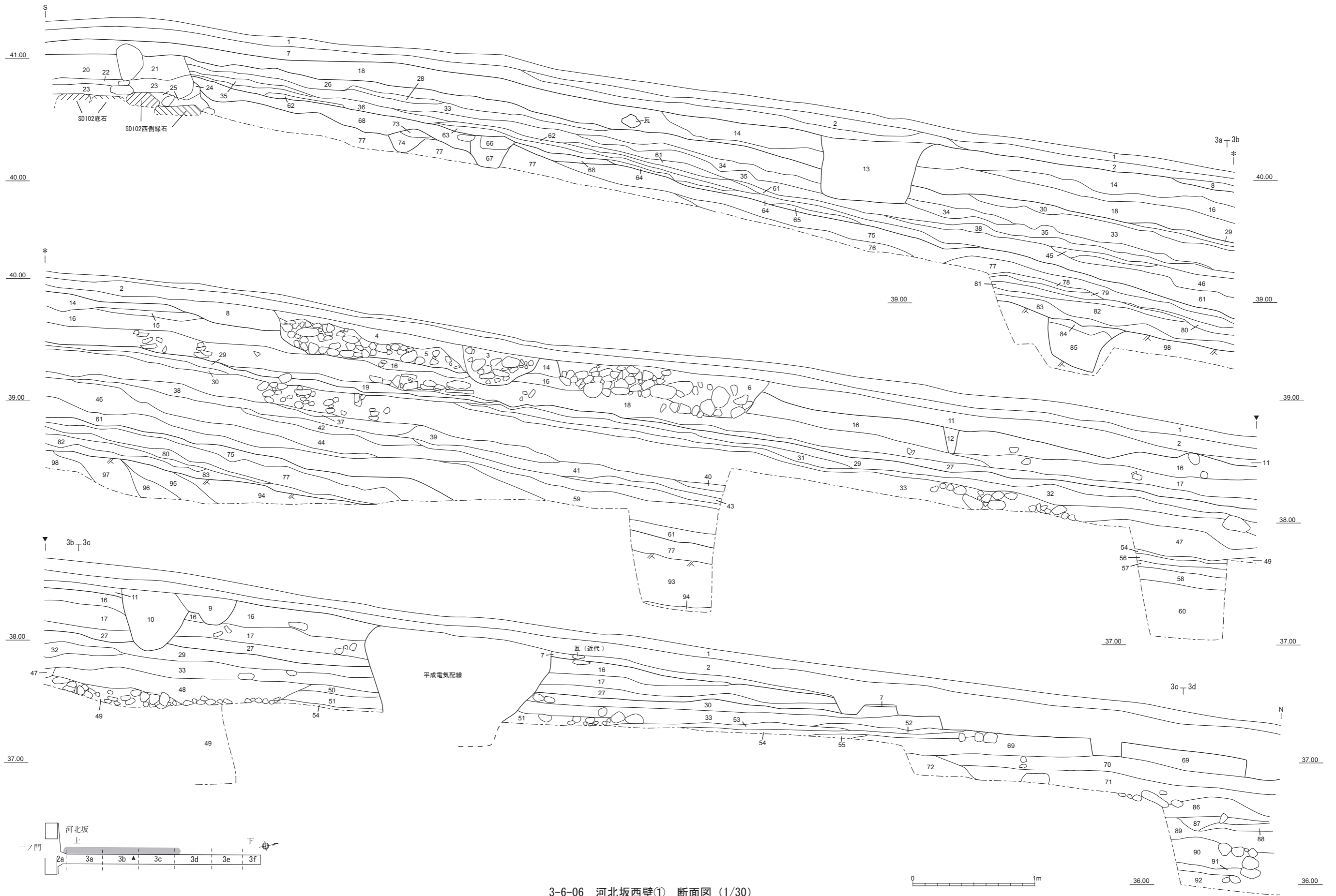
3-6-06 河北坂西壁① 断面図 (1/30) 第49図 遺構図版 河北坂3
