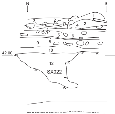
3-4-02 SD214-2 東壁 断面図②(1/30)
