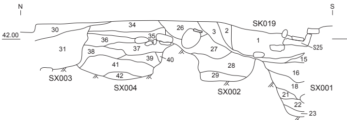
3-3-55 T019 東壁 断面図 (1/40)
