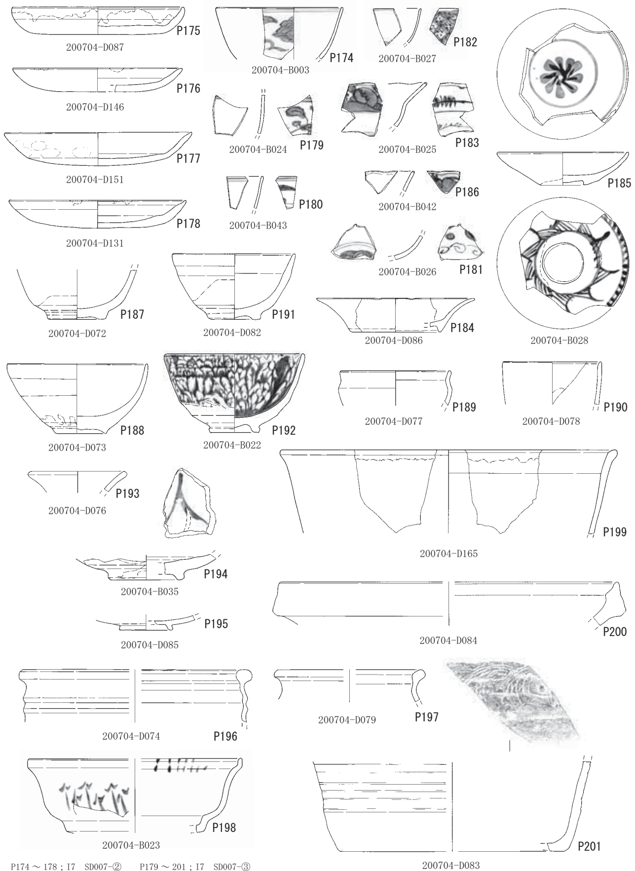
第 226 图 遺物実測図 陶磁器・土器 8 (S=1/3)
