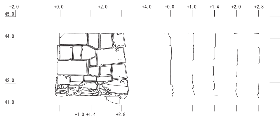
ID 3231E (一ノ門西側類当石垣東面) 立面図・垂直断面図
