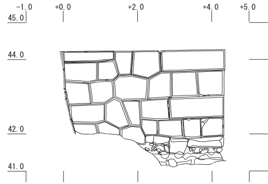
ID 3241N (一ノ門東側類当石垣北面) 立面図
