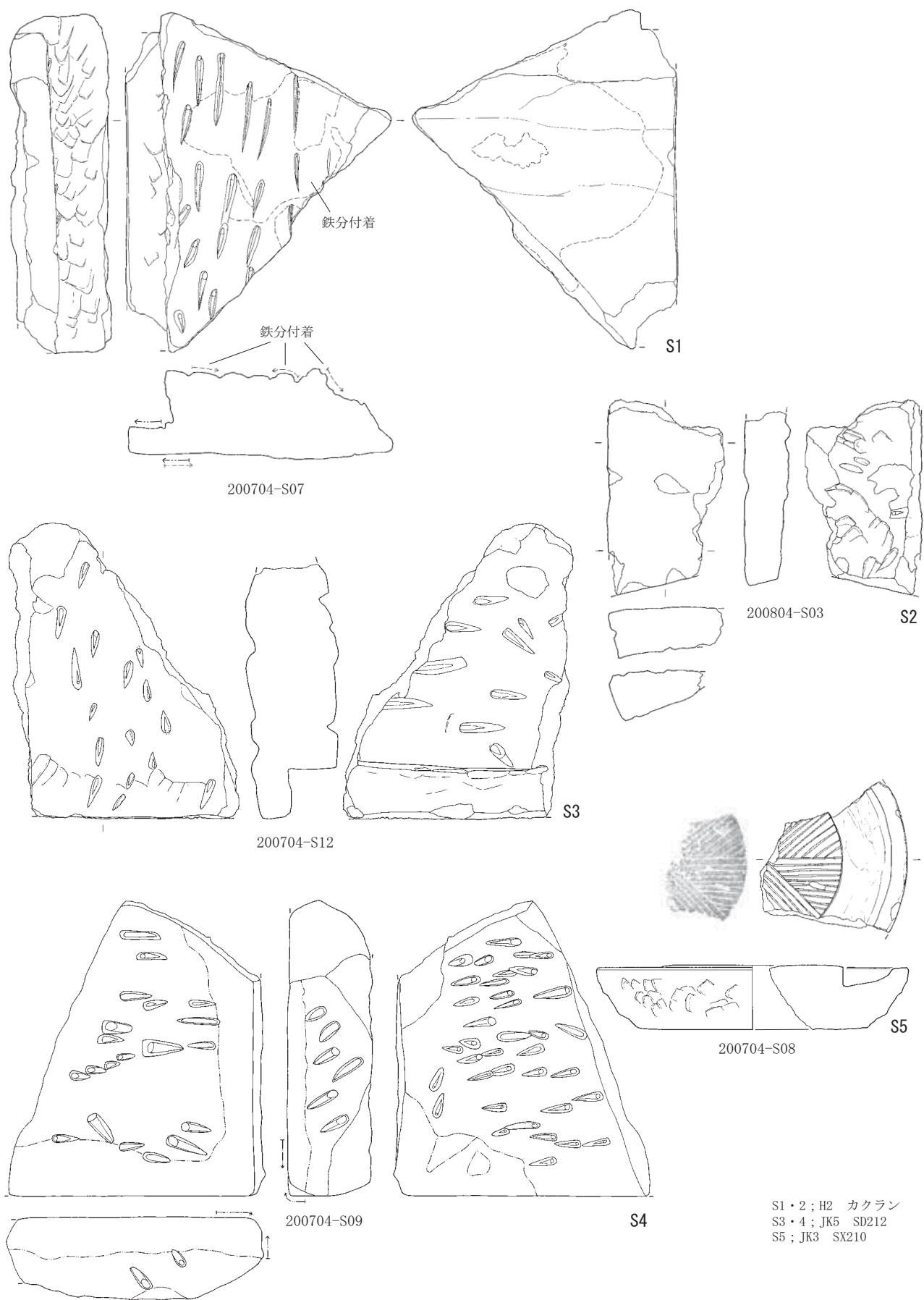
第 243 図 遺物実測図 石製品 1 (S=1/6)
