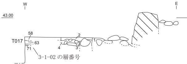
3-5-16 3230W 東西断面図① (1/40)
