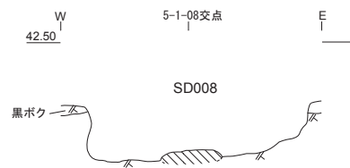
5-1-09 SD008 エレベーション②(1/40)
