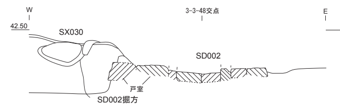
3-3-43 SD002 東西エレベーション図② (1/30)
