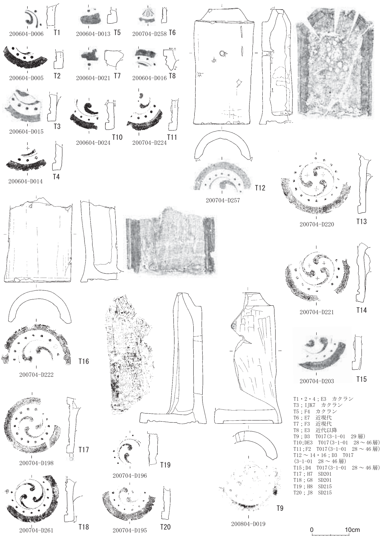
第 231 図 遺物実測図 瓦 1(S=1/6)
