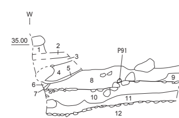
3-6-10 東西 断面図①(1/30)
