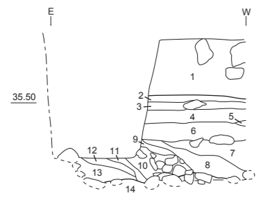
3-6-10 東西 断面図①(1/30)
