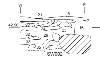
5-3-06 SD204-2 北壁② 断面図 (1/30)
