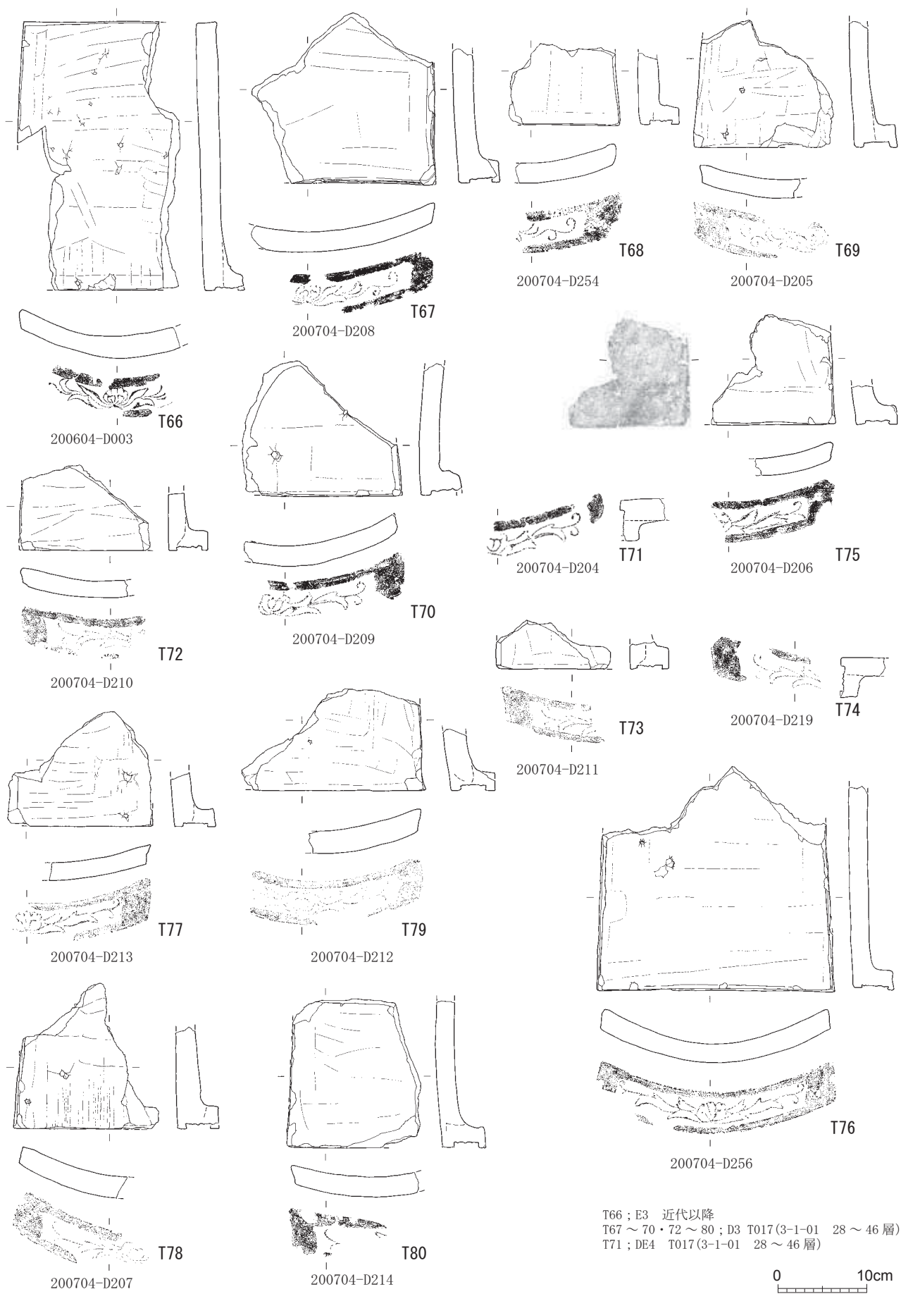
第 235 図 遺物実測図 瓦 5 (S=1/6)
