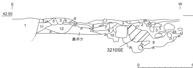
3-3-30 3210S-T004 西壁 断面図 (1/40)
