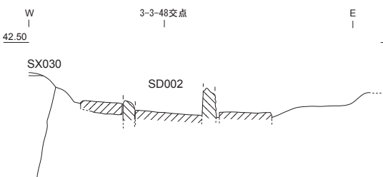
3-3-42 SD002 東西エレベーション図① (1/30)
