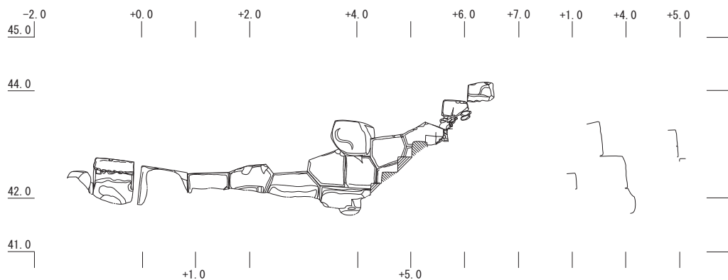
ID 3230E (ニラミ櫓台石垣東面) 立面図・垂直断面図
