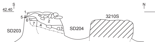
3-3-32 3210S 断面図 (1/30)
