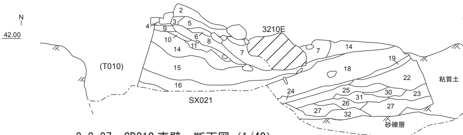
3-3-37 SD210 東壁 断面図 (1/40)
