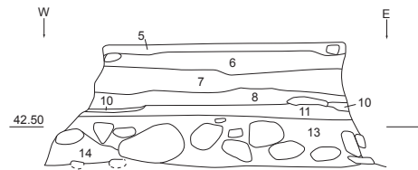
3-4-18 3220S 東西断面図①(1/20)
