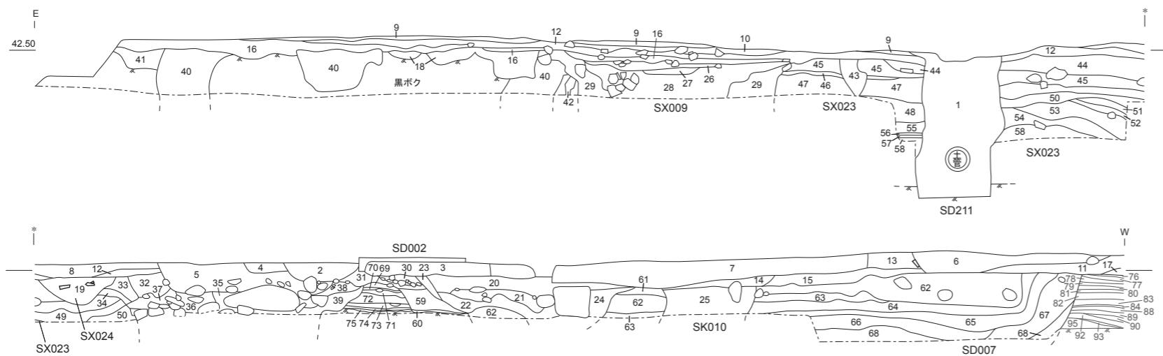
3-1-06 SD209・SX210 南壁 断面図 (1/40)
