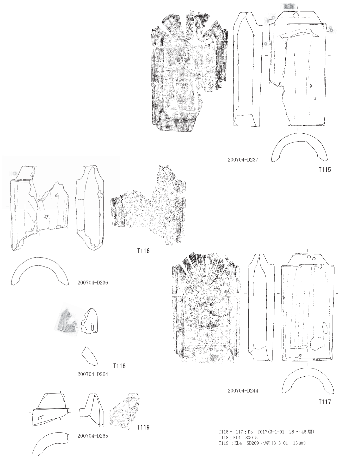
第 239 図 遺物実測図 瓦 9 (S=1/6)
