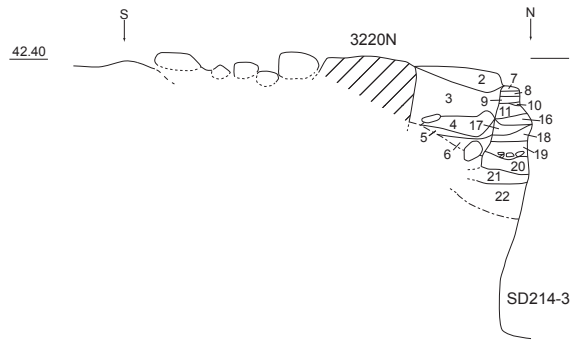
3-4-15 3220N 南北断面図 (1/30)
