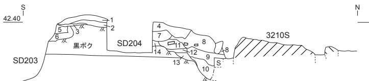
3-3-33 3210S-T009 西壁 断面図 (1/30)
