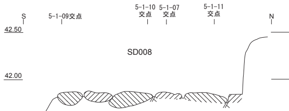
5-1-08 SD008 エレベーション①(1/40)
