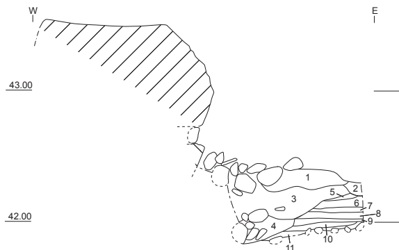
3-3-21 3240W-T001 北壁 断面図 (1/40)
