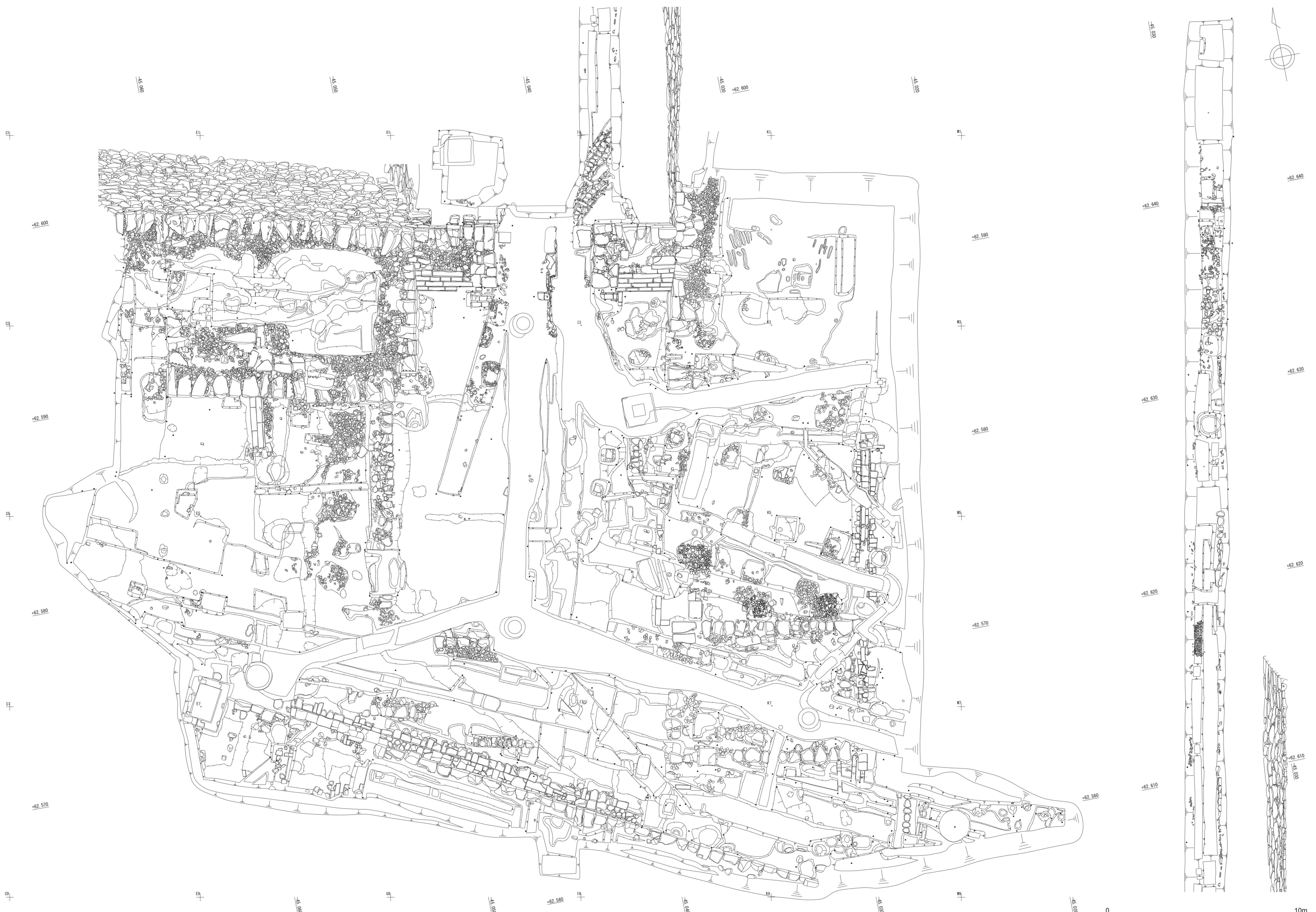
金沢城跡河北門 遺構全体図 (S=1/100)
