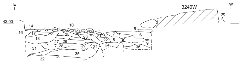
3-3-18 3240W-T002 南壁 断面図 (1/40)
