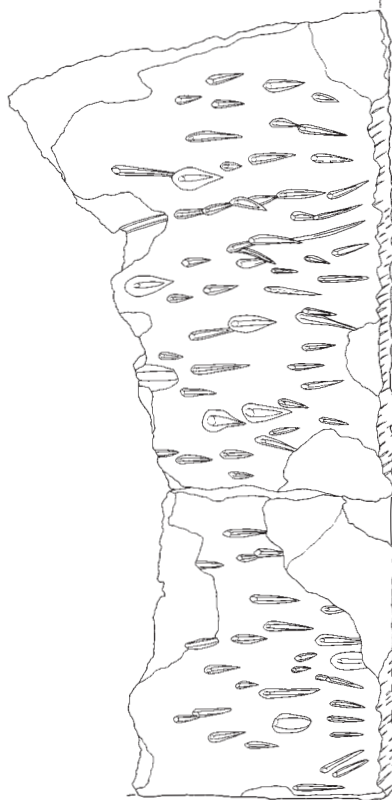
第 246 図 遺物実測図 石製品 4 (S=1/6)
