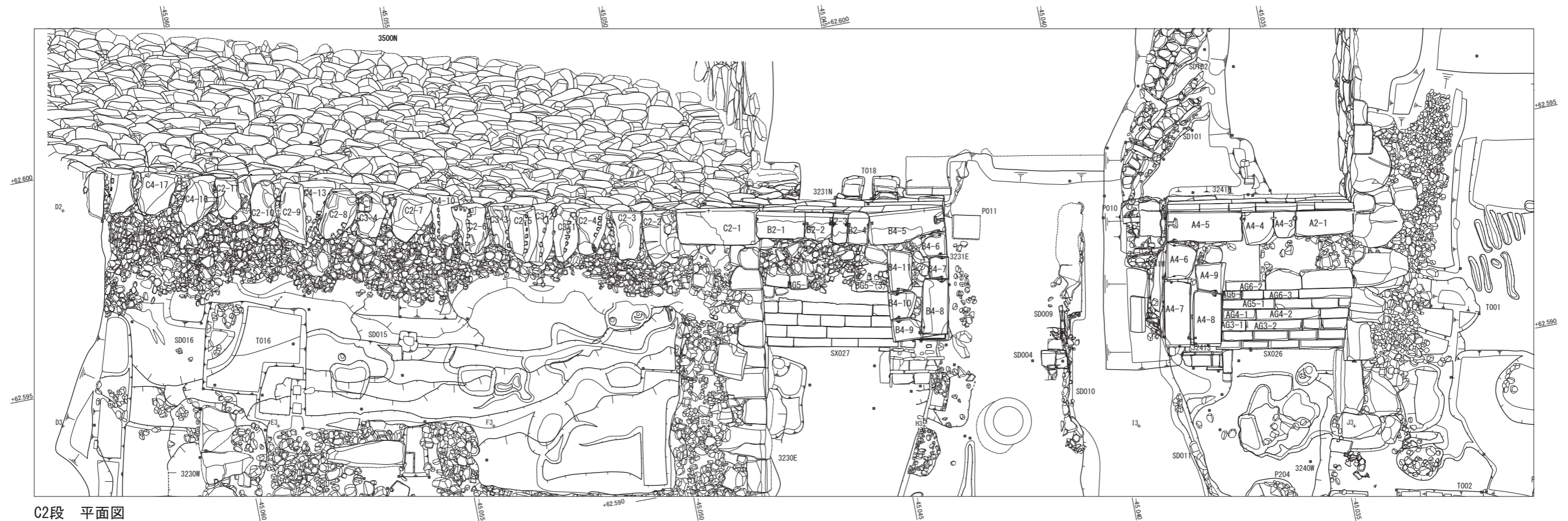
第74图 遺構図版 石垣解体測量図1 (S=1/100)
