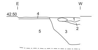
3-3-04 SX201 南壁 断面図 (1/40)
