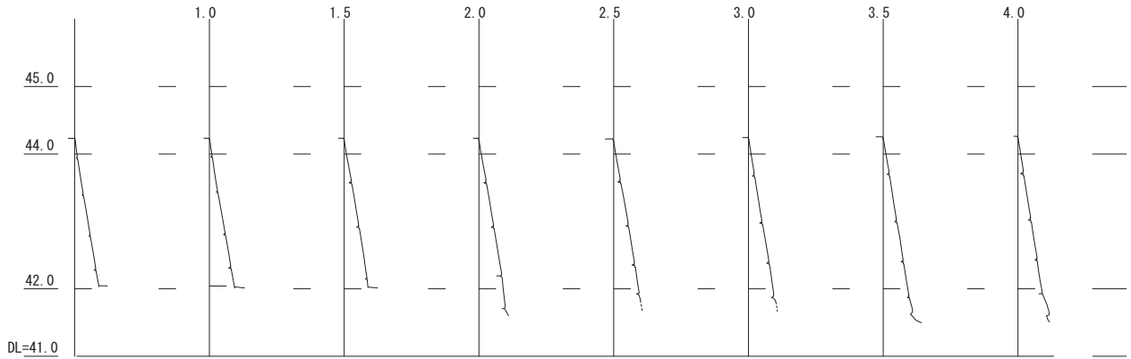
ID 3241N (一ノ門東側類当石垣北面) 垂直断面図
