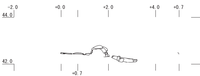
ID 3220E (土堀下石垣東面) 立面図・垂直断面図
