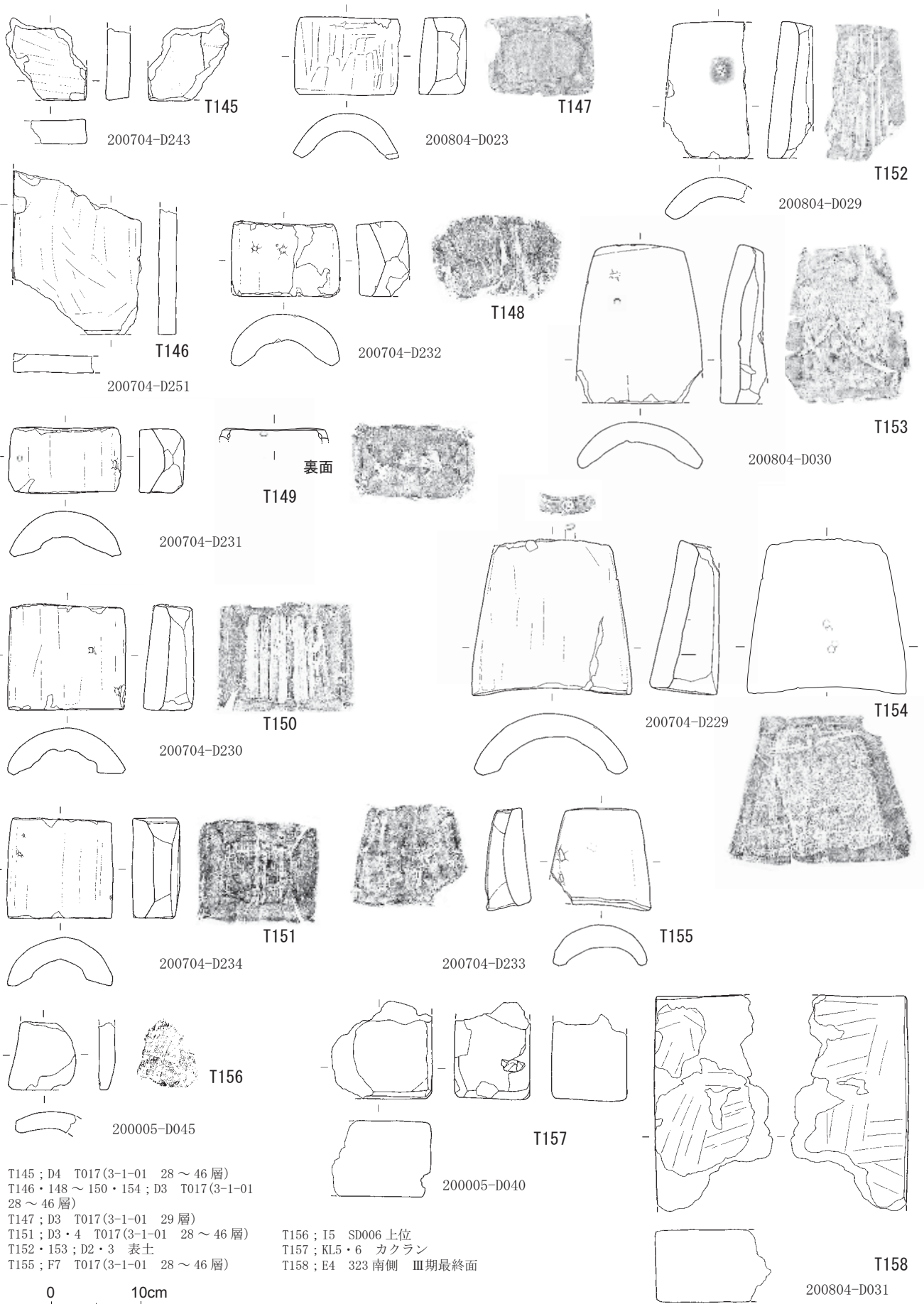
第 242 図 遺物実測図 瓦 12(S=1/6)
