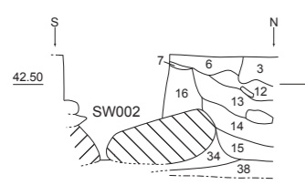
5-3-01 SD204-2 西壁① 断面図 (1/30)
