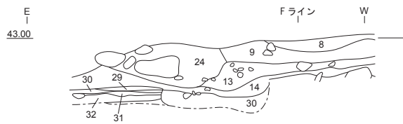
3-4-13 SA001-T014 南壁 断面図 (1/40)
