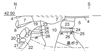
3-3-03 SX201 東壁 断面図 (1/40)
