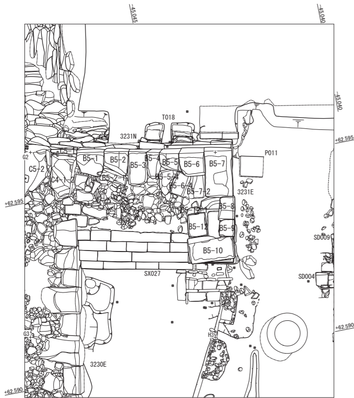
B5段下 平面図
