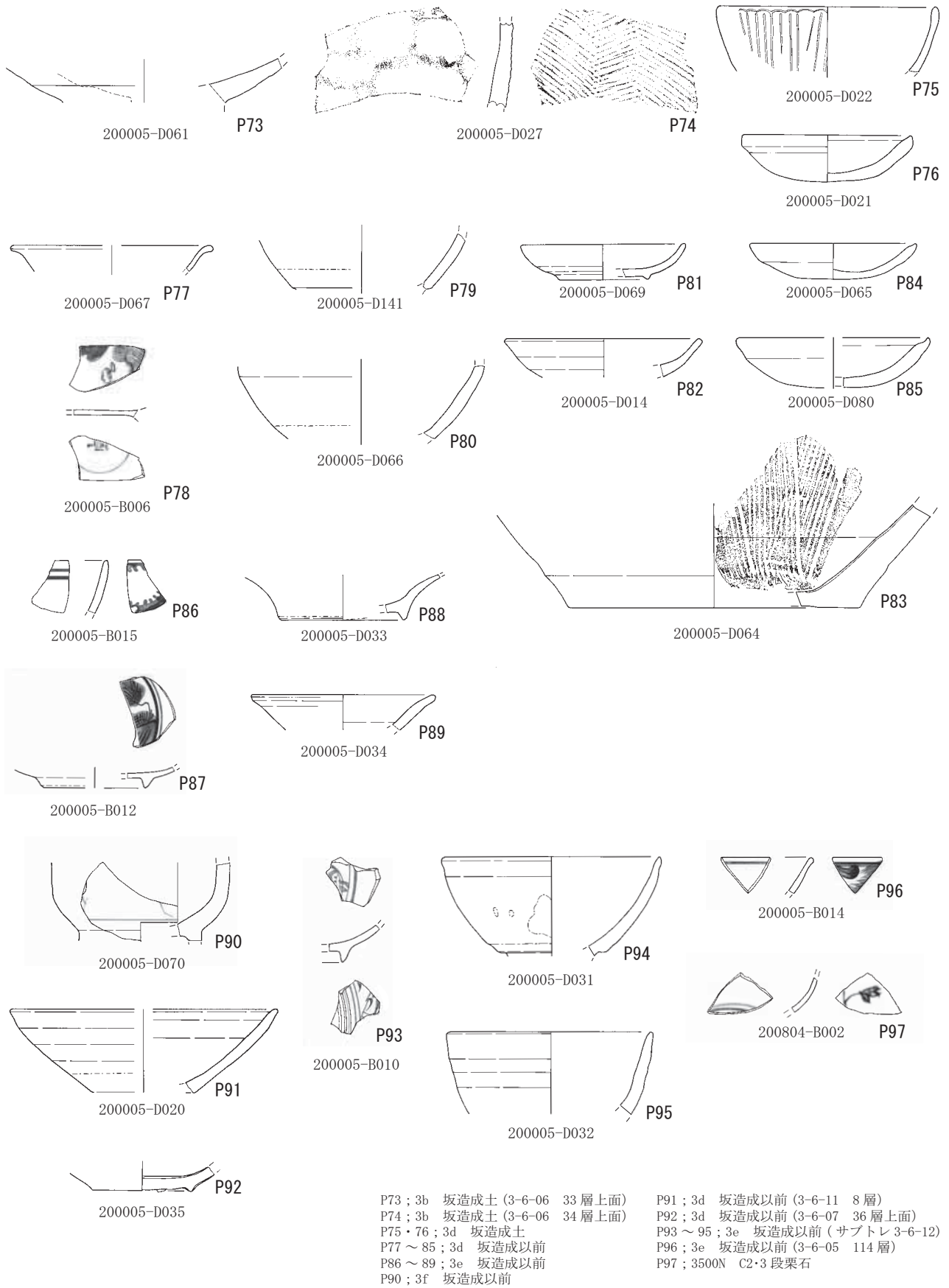
第 222 図 遺物実測図 陶磁器・土器 4 (S=1/3)
