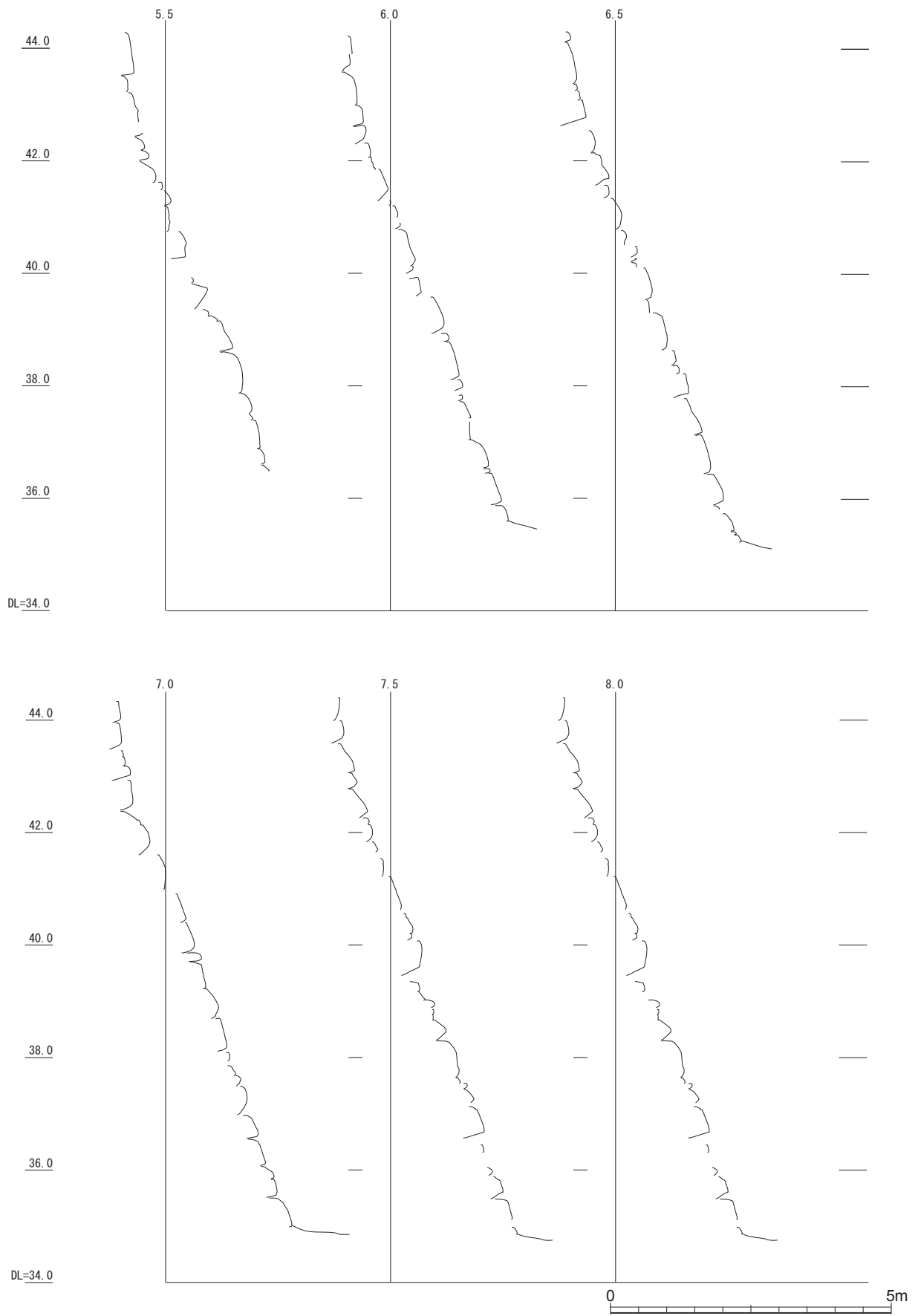
第 57 図 遺構図版 ニラミ 檜台石垣北面 (ID3500N) 垂直断面図 2 (S=1/100)
