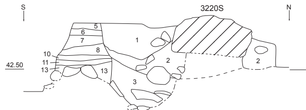
3-4-17 3220S 西壁 断面図 (1/20)
