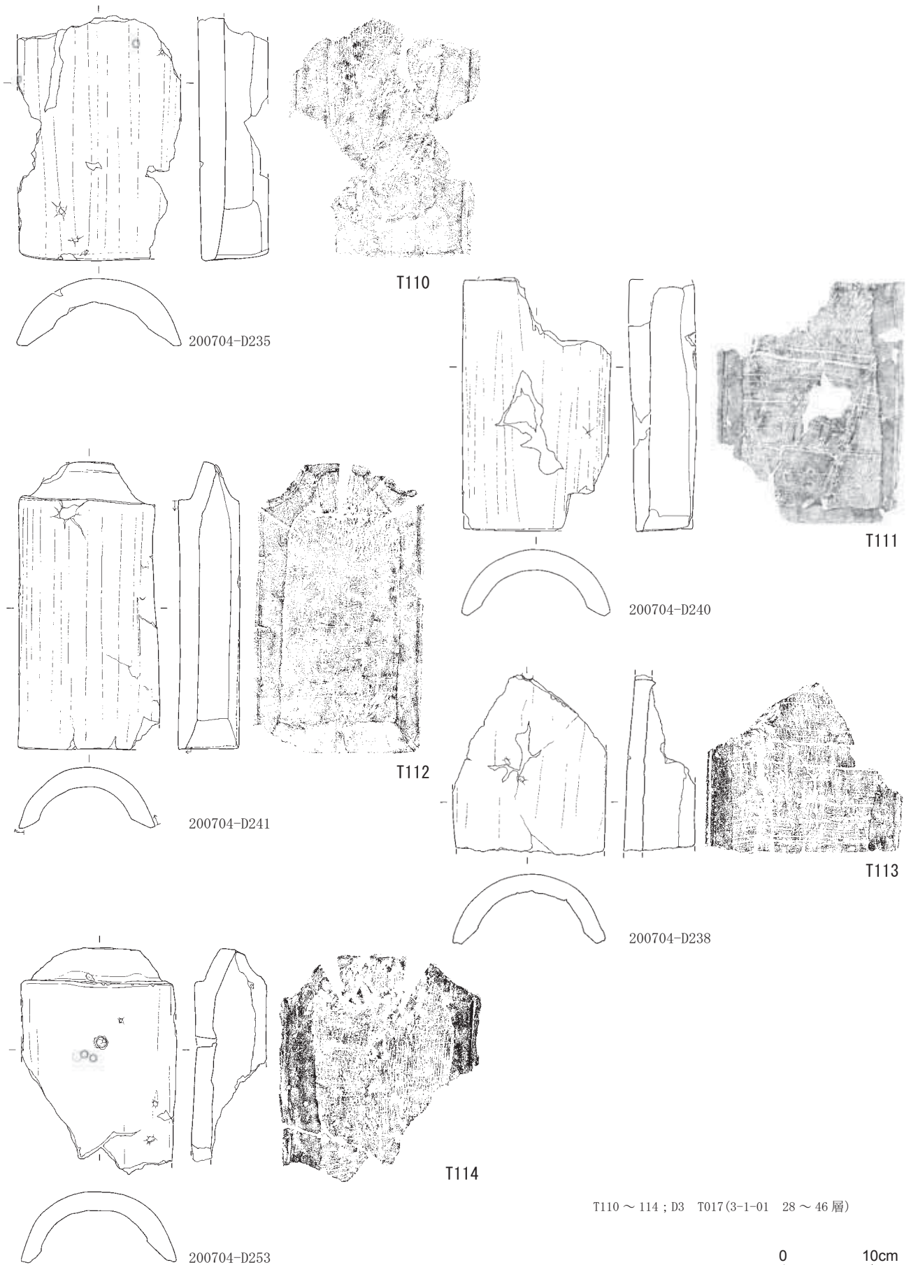
第 238 図 遺物実測図 瓦 8 (S=1/6)
