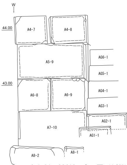
4-1-01 3241S 立面図 (1/40)
