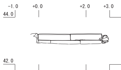
SX028 (ニラミ櫓台南側階段) 立面図
