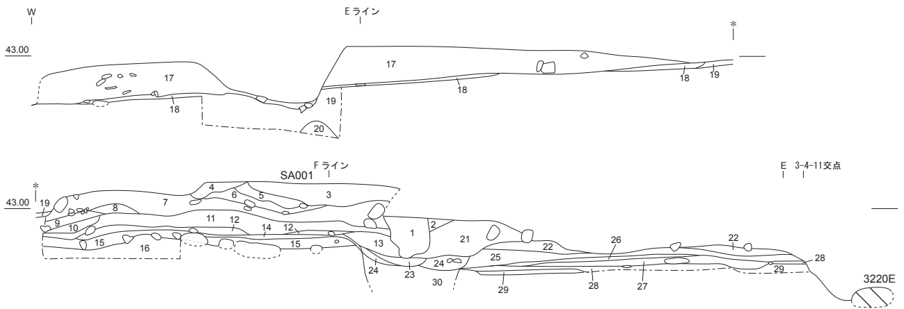
3-4-12 SA001-T014 北壁 断面図 (1/40)
