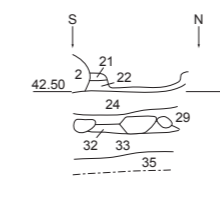
5-3-05 SD204-2 西壁② 断面図 (1/30)
