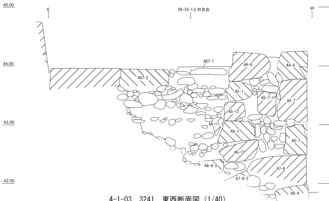
4-1-03 3241 東西断面図 (1/40)
