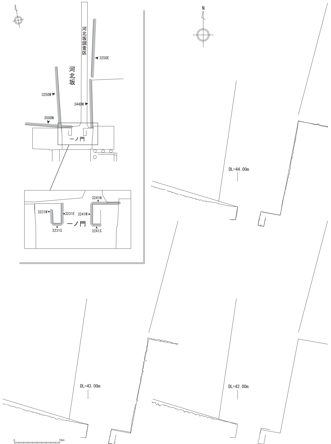
第 52 図 遺構図版 石垣水平断面図 1 (S=1/400)
