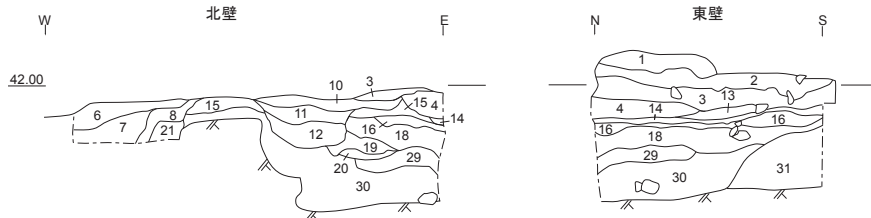
3-3-19 324-T002 北・東壁 断面図 (1/40)
