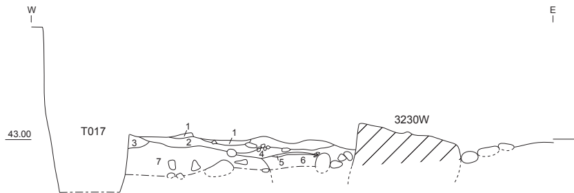
3-5-16 3230W 東西断面図① (1/40)
