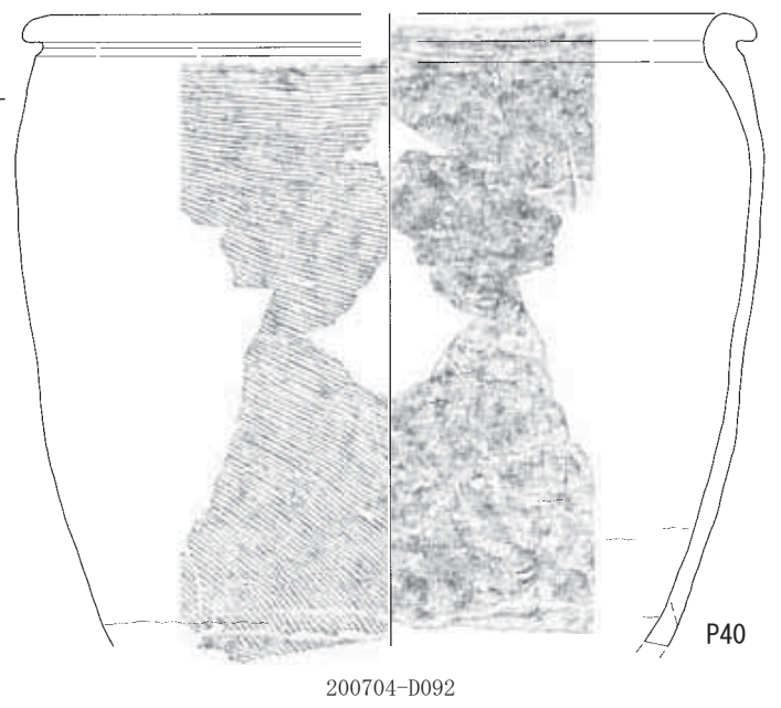
第220図 遺物実測図 陶磁器・土器2 (S=1/3・S=1/6)
