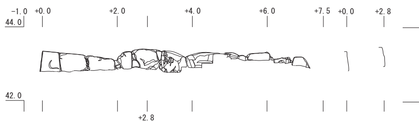
ID 3230S (ニラミ櫓台石垣南面) 立面図・垂直断面図
