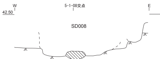
5-1-10 SD008 エレベーション③(1/40)
