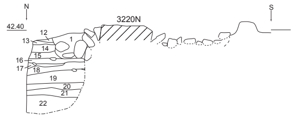
3-4-16 3220N 南北断面図 (1/30)
