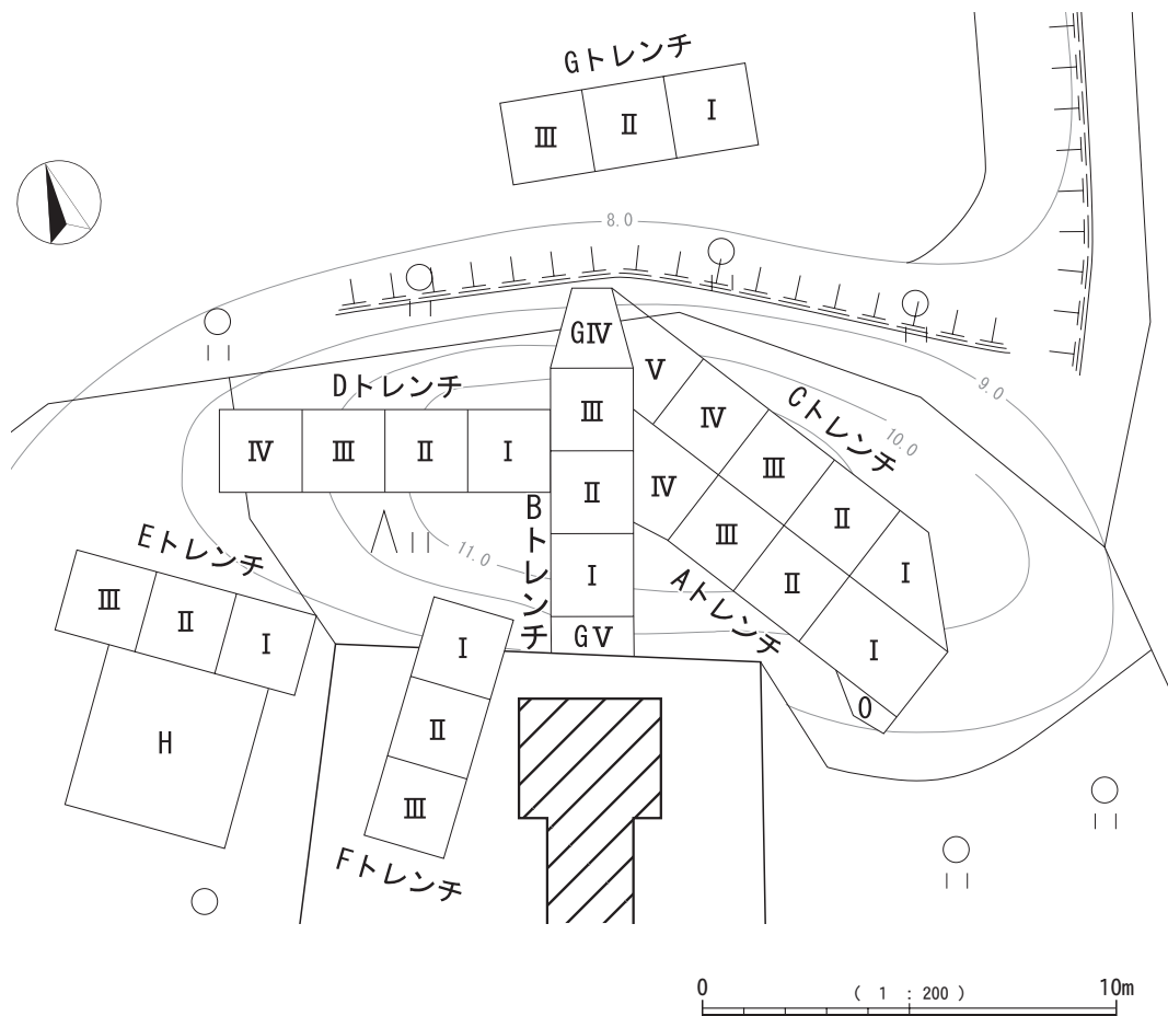
第2図 高橋貝塚 トレンチ配置図
