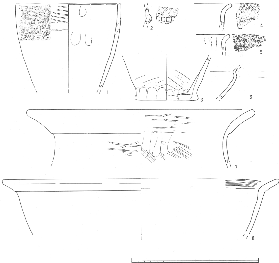
第5図 溝2出土土器実測図 (1/3)
