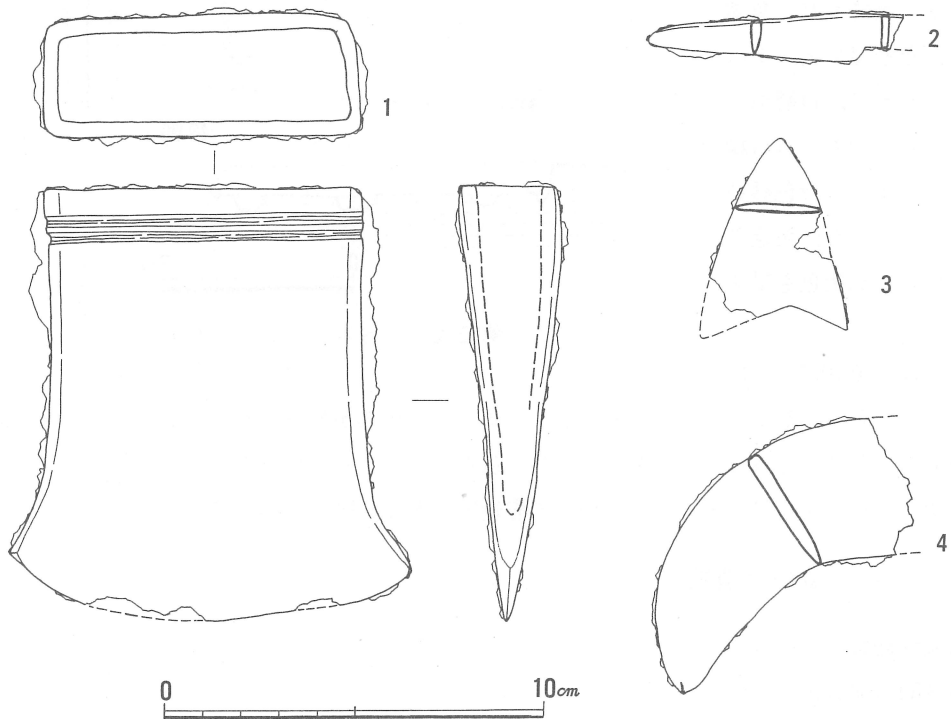
第 11 図 出土鉄器実測図 (1/2)
