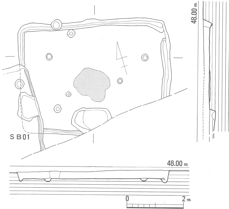
第 13 図 SB02実測図 (1/80)
