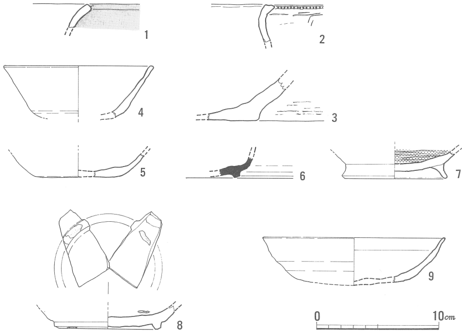
第 18 図 第 3 層出土土器実測図 (1/3)
