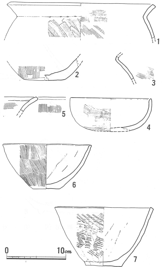
第16図 SB02出土土器実測図(1/4)
