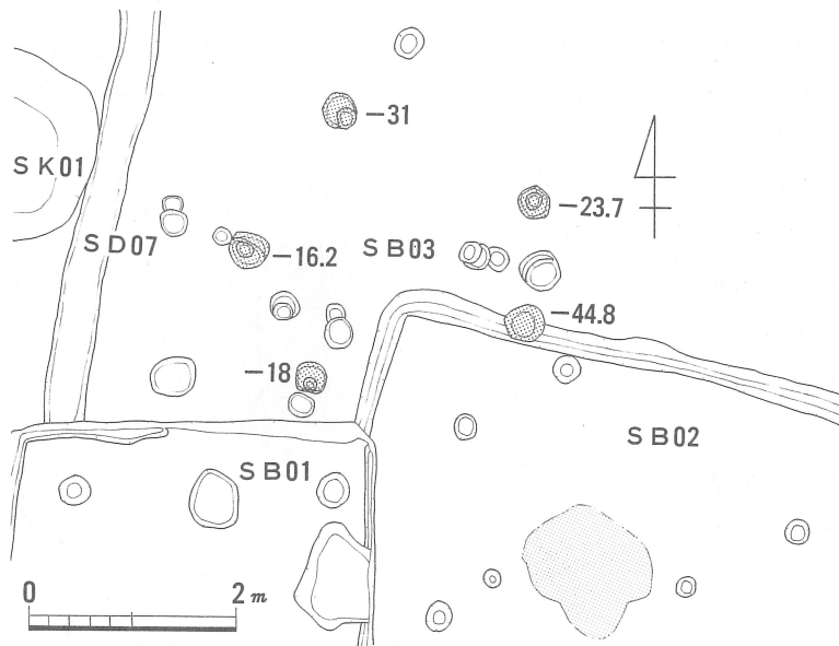
第 14 図 SB03実測図 (1/80)
