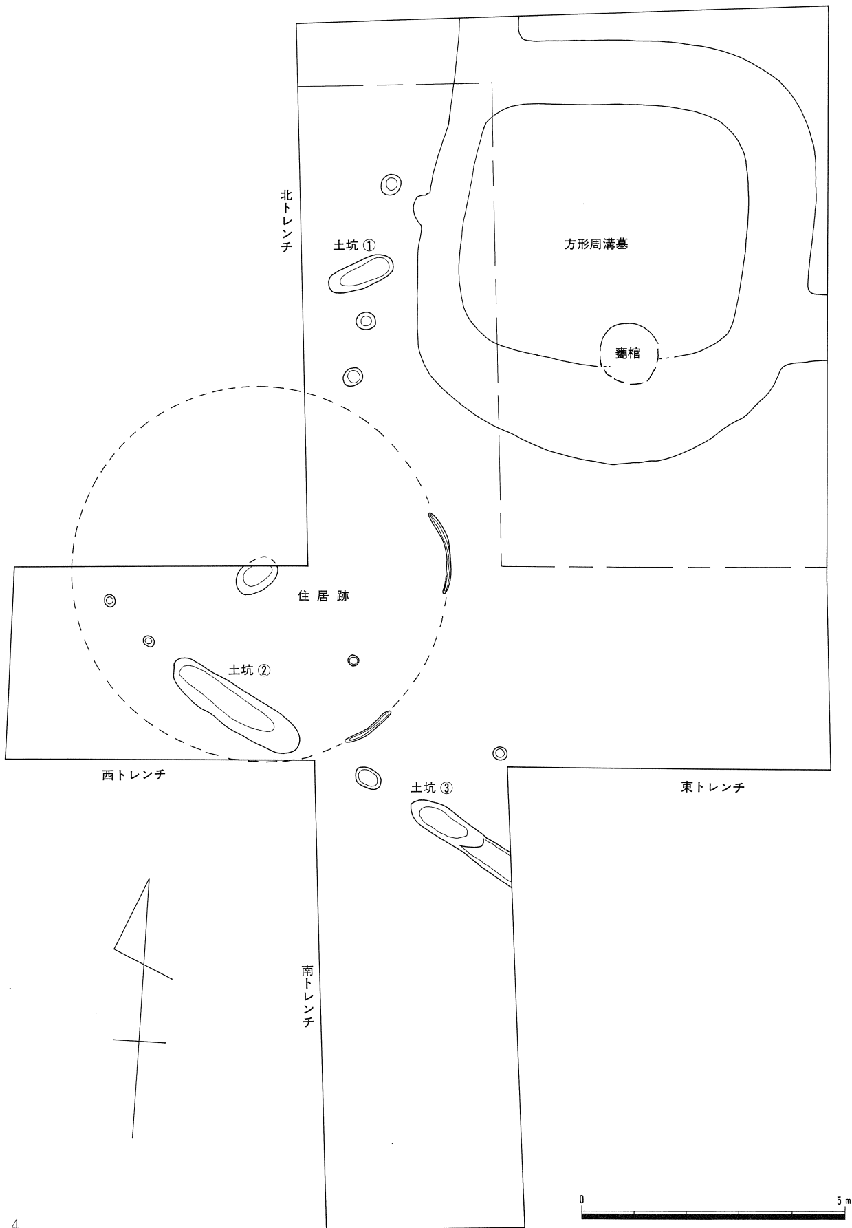
Fig. 4 調査区内遺構配置図 (1/100)
