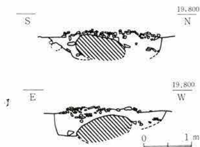
Fig. 3 No.25掘り方断面図
