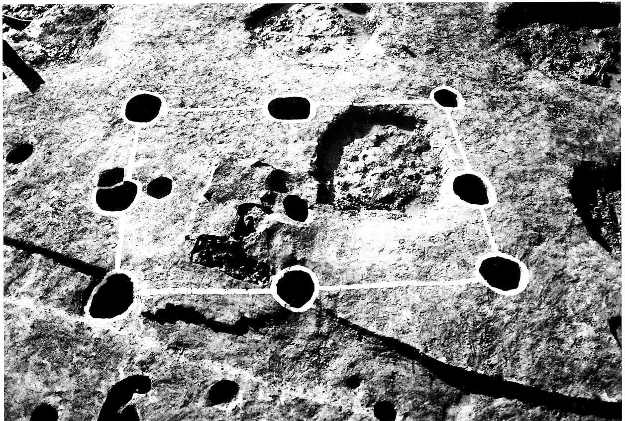
2 第51号掘立柱建物跡
