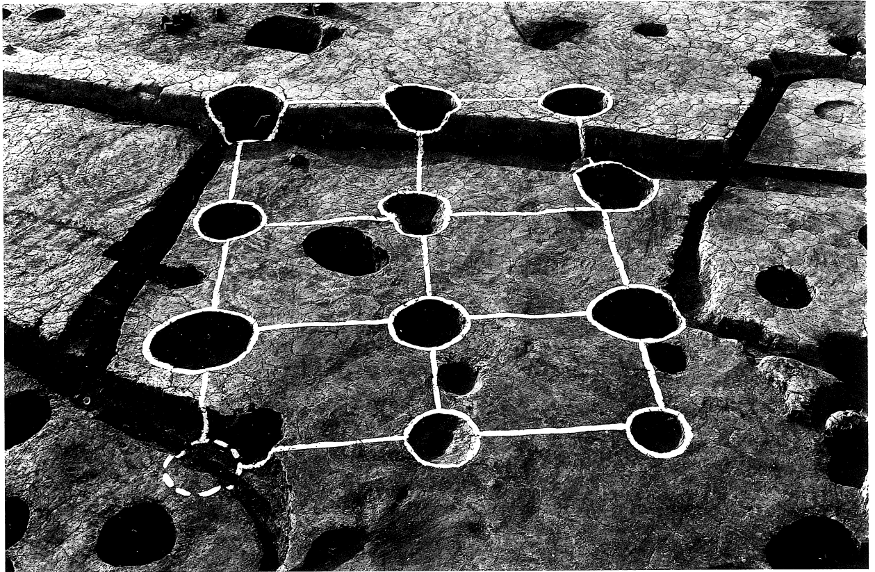
1 第50号掘立柱建物跡
