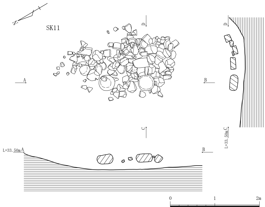
第 12 図 集石遺構 A 実測図
