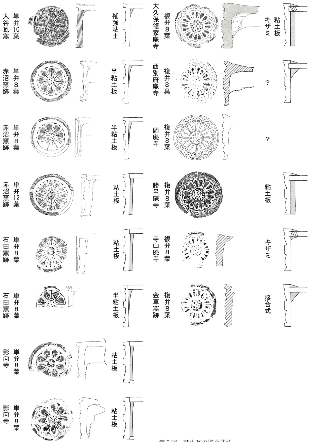
第5図 軒先瓦の接合技法
