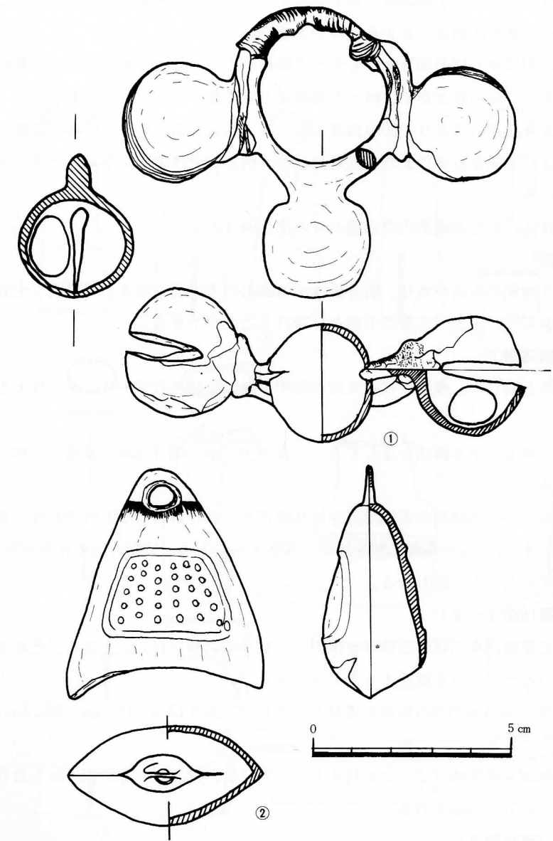
第14図 馬具実測図(II) 〔三環鈴①、馬鐸②〕
