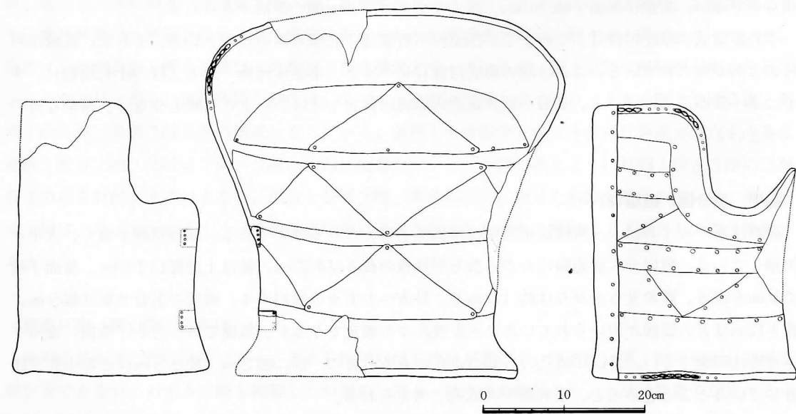
第 11 図 武具実測図 (III)〔三角板鉄留短甲〕
