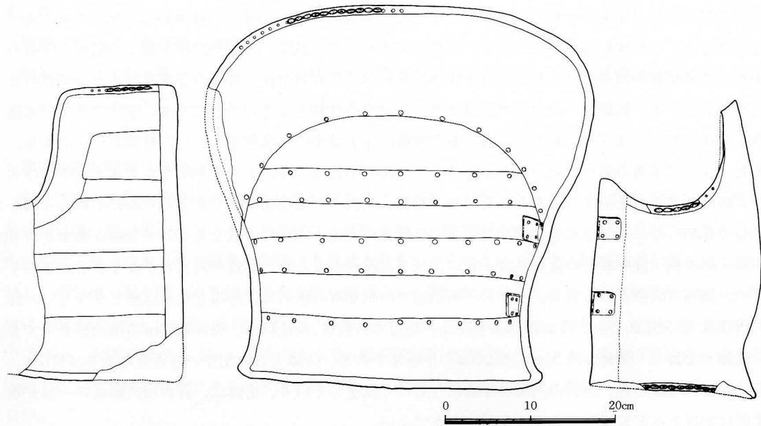
第 10 図 武具実測図 (II)〔横板板鉄留短甲〕
