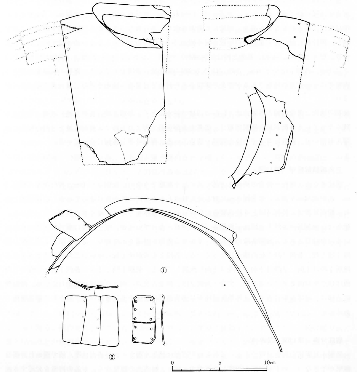
第 9 図 武具実測図 (I) [ 頸甲①、小札② ]
