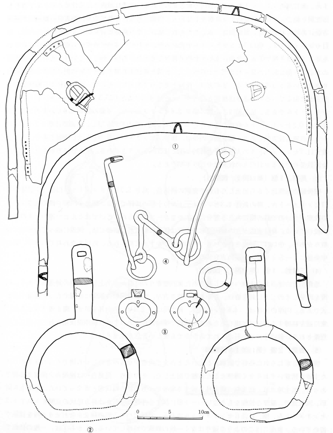
第13図 馬具実測図 (I)
