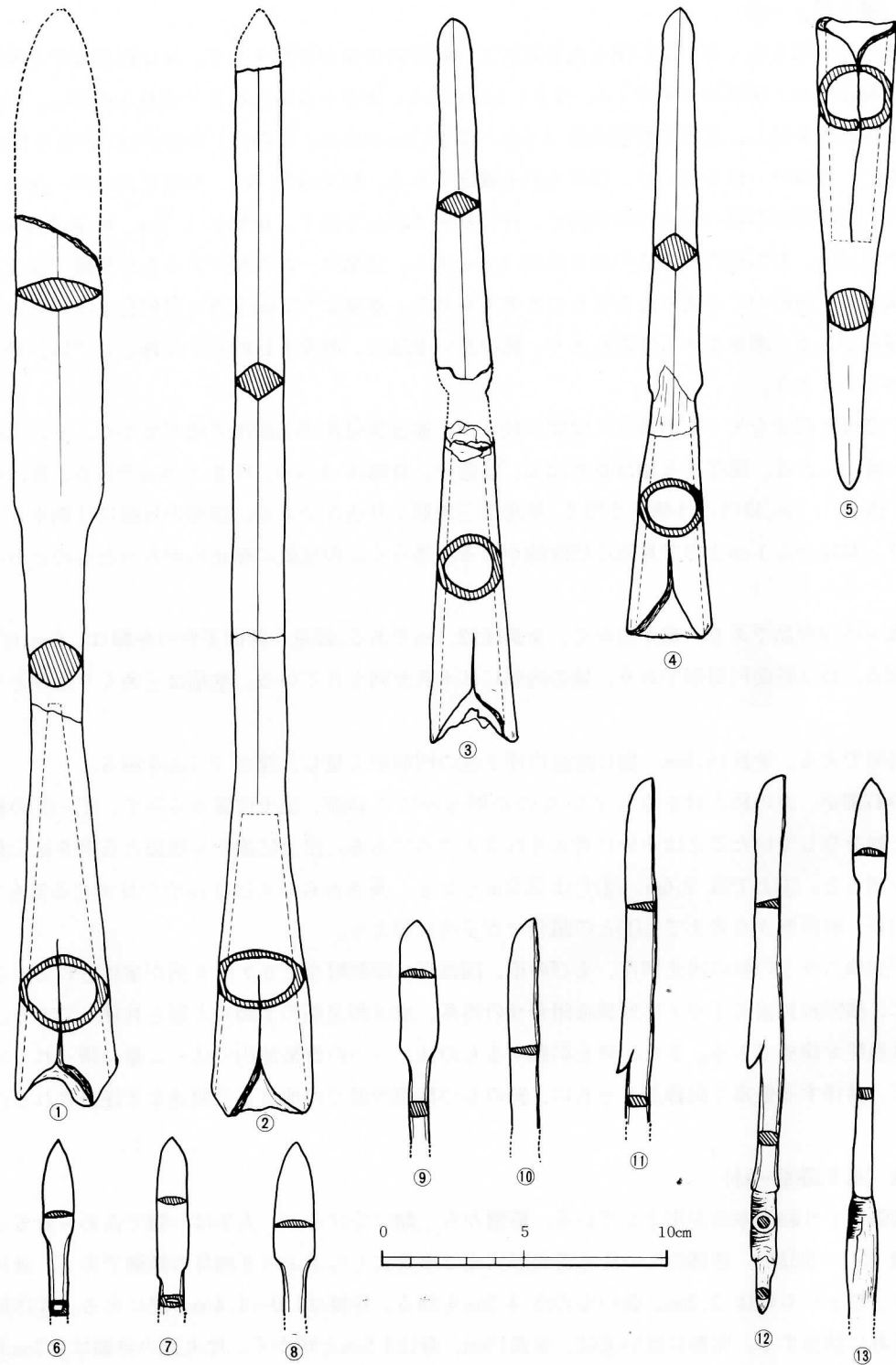
第 8 図 武器実測図 (II) [ 鉾①~⑤、鉄剣⑥~⑬ ]
